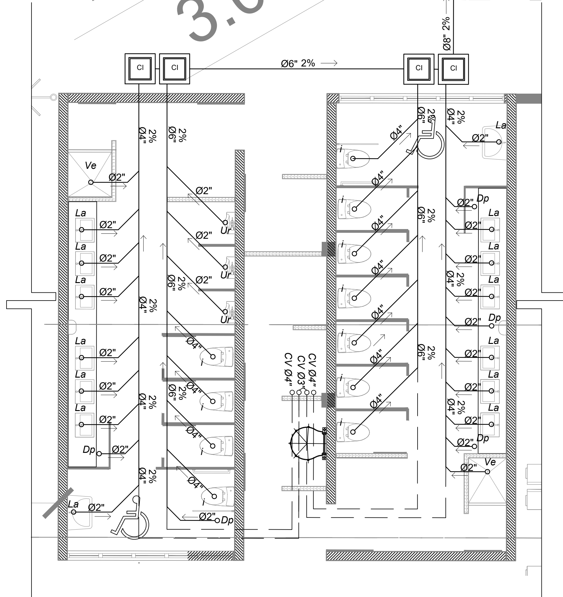
2 D-2 Baños Hombres y Mujeres Esc. 1:50
