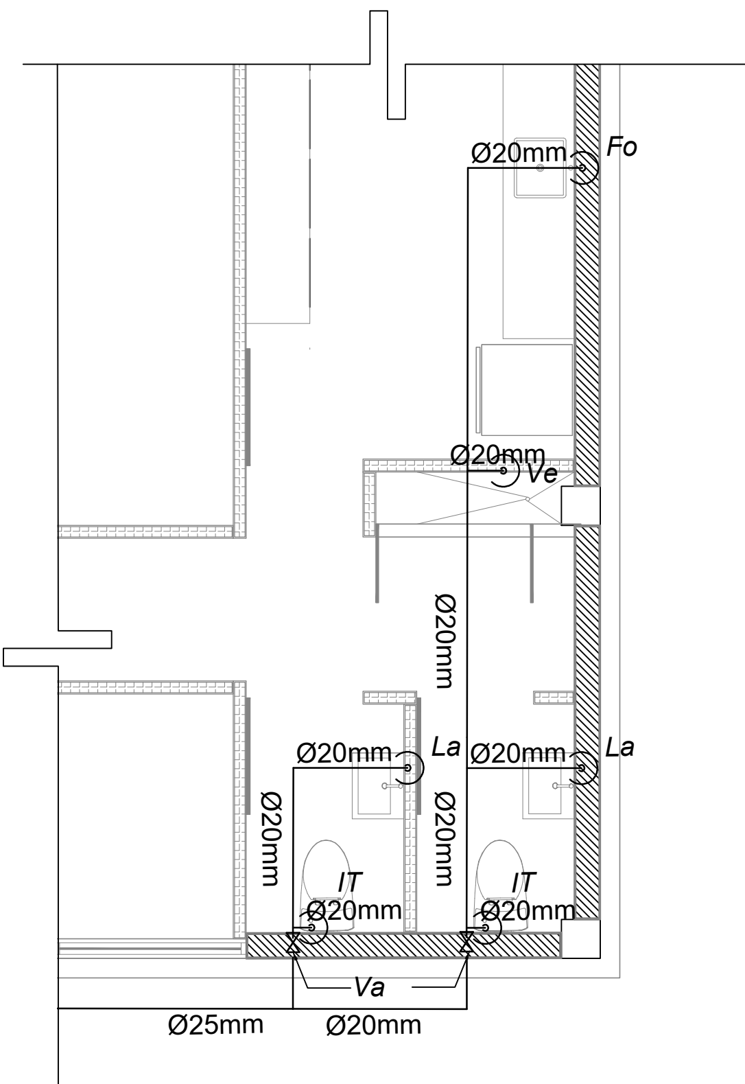
5 D-11 Baños Módulo Administrativo Esc. 1:40
