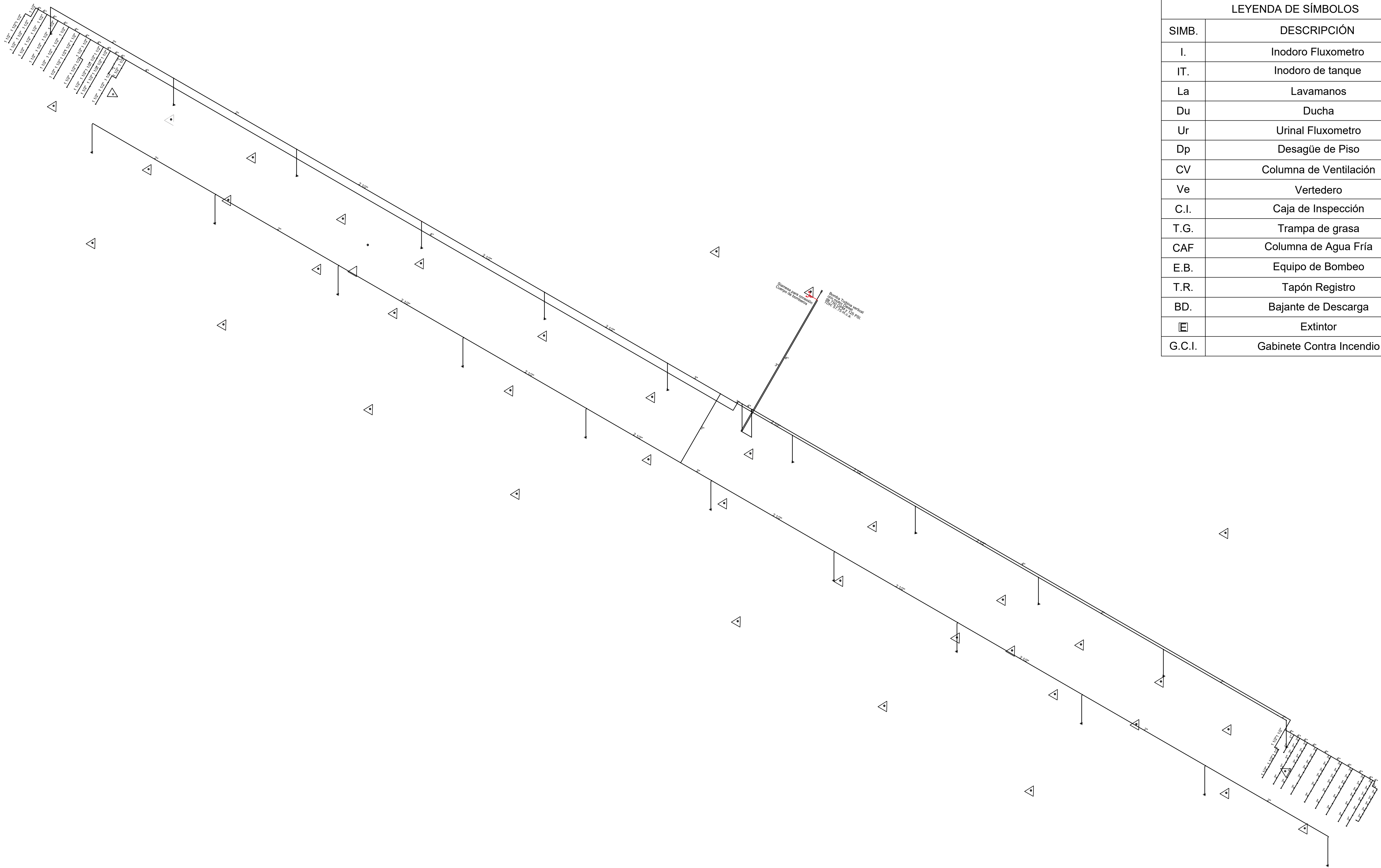
1 Proyección Isométrica Contra Incendios No Esc.
