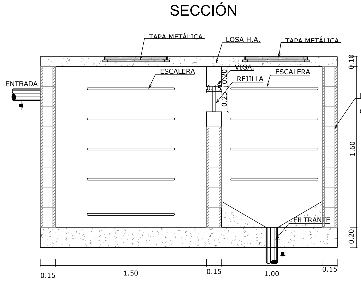
5 DETALLE DESARENADOR. Esc. 1:20
