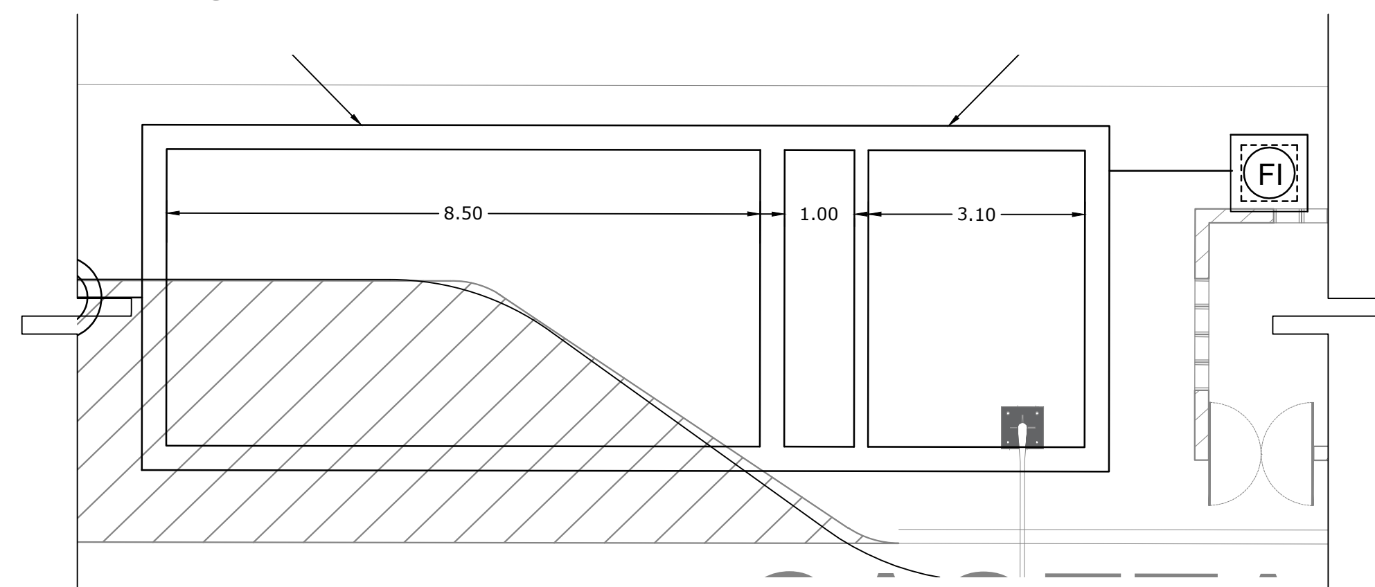
6 D-6 Reactor Anaerobio de Flujo Ascendente Esc. 1:75
