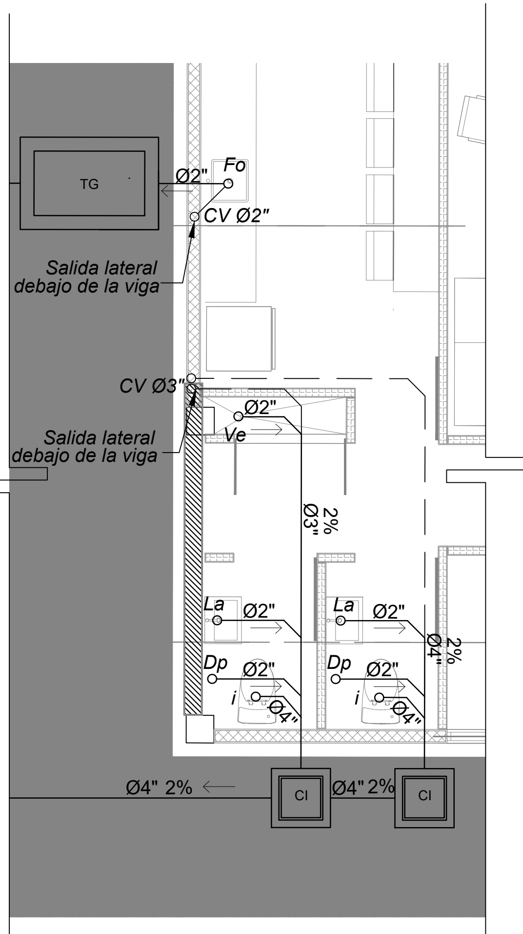
1 D-1 Baños Módulo Administrativo Esc. 1:40
