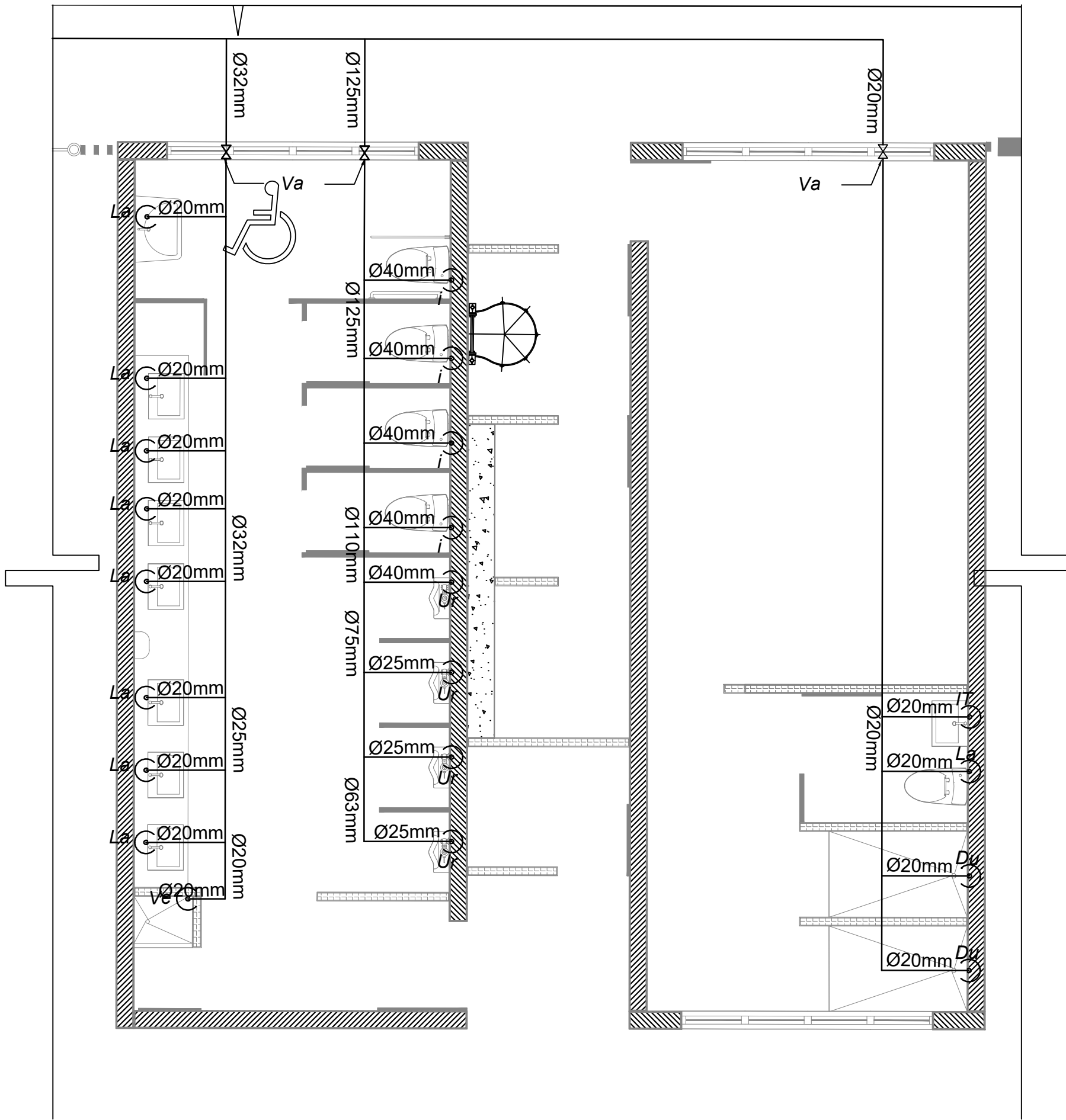
2 D-8 Baños Hombres Esc. 1:50
