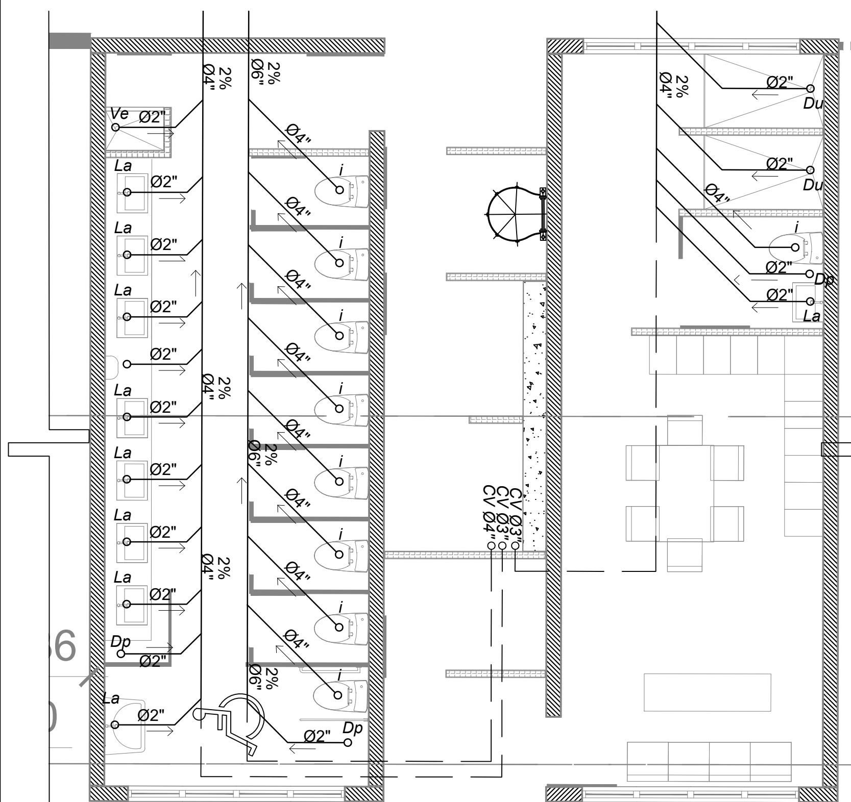
4 D-4 Baños Mujeres Esc. 1:50
