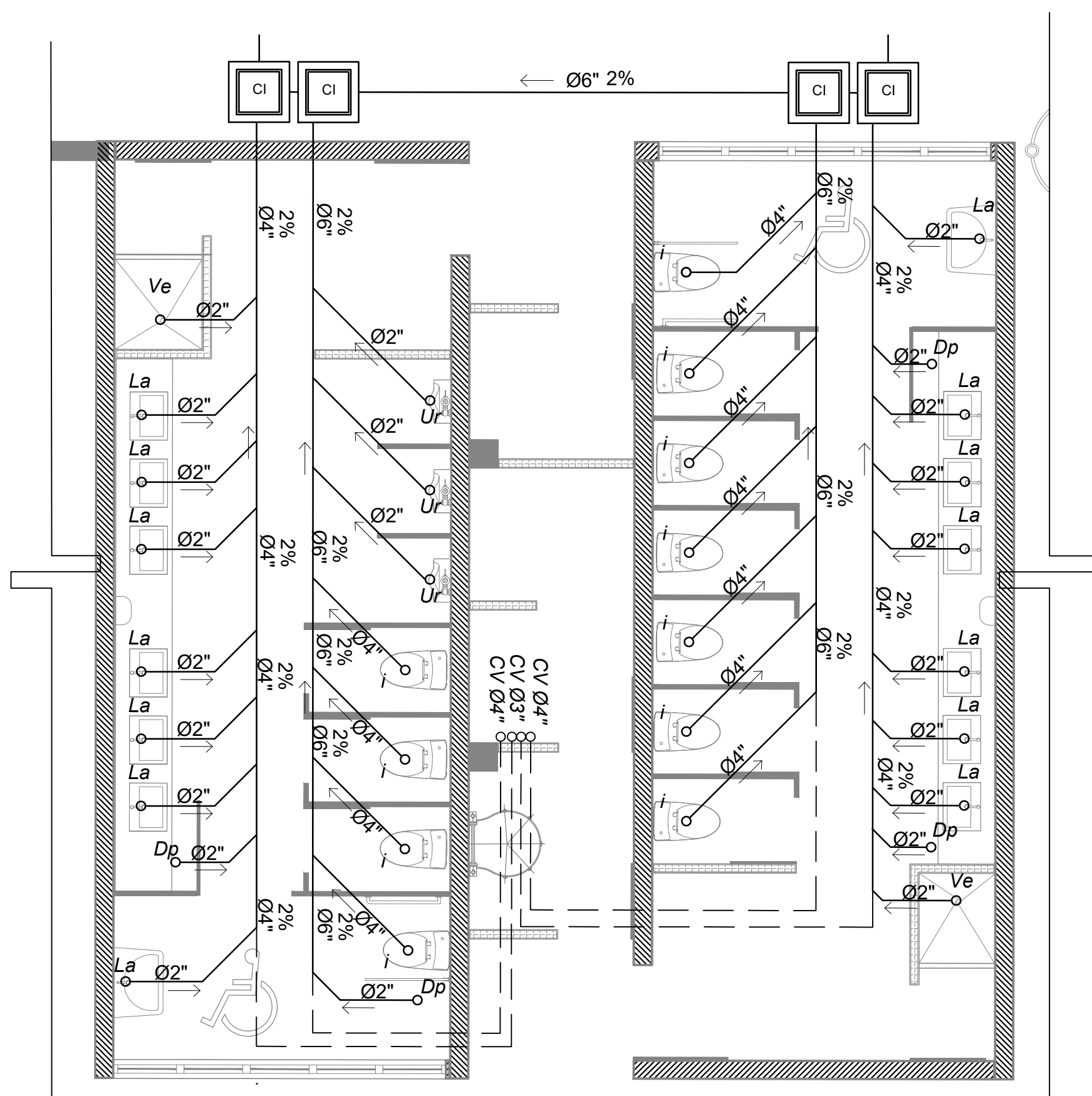
4 D-10 Baño Hombres y Mujeres Esc. 1:50
