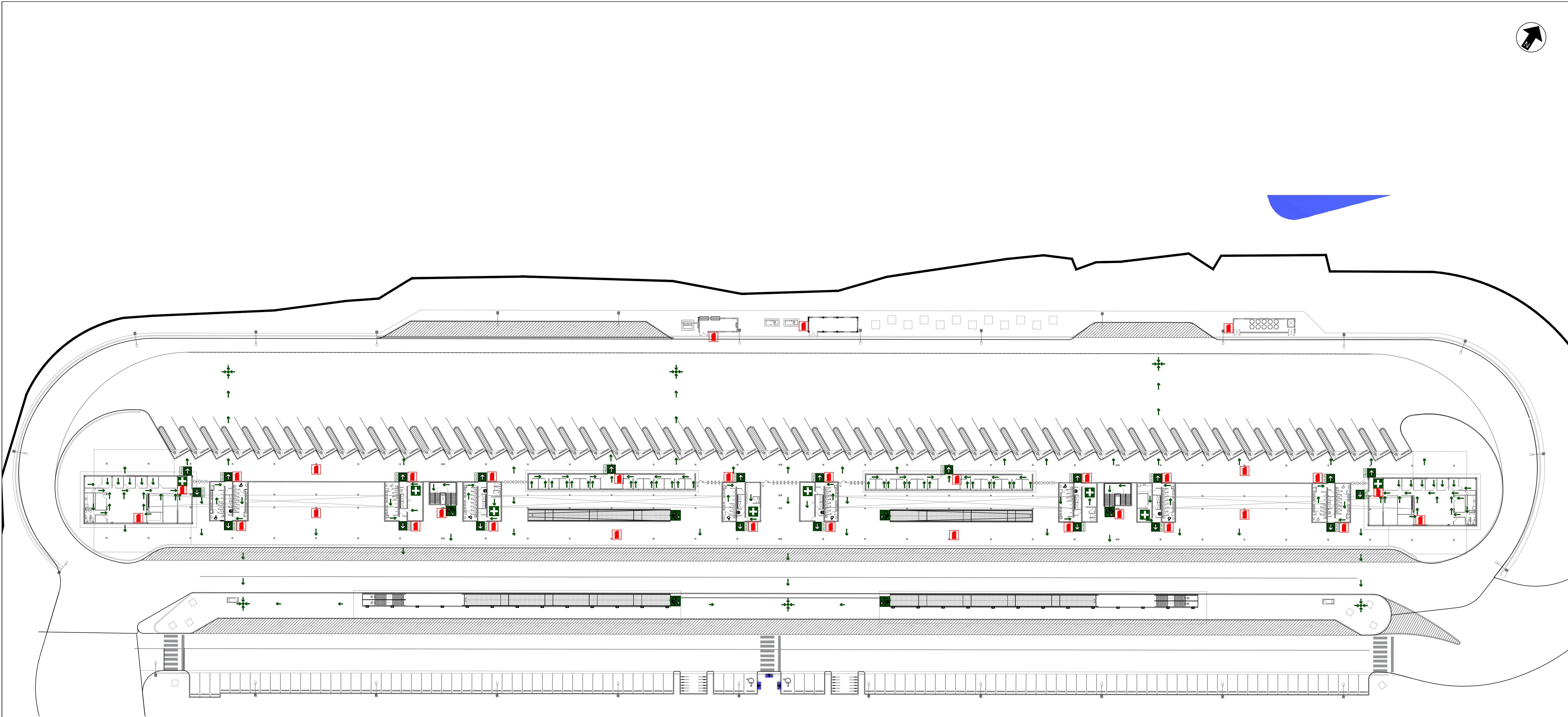
1 Planta de Señalización y Ruta de Evacuación, Nivel 1 Esc. 1:500
