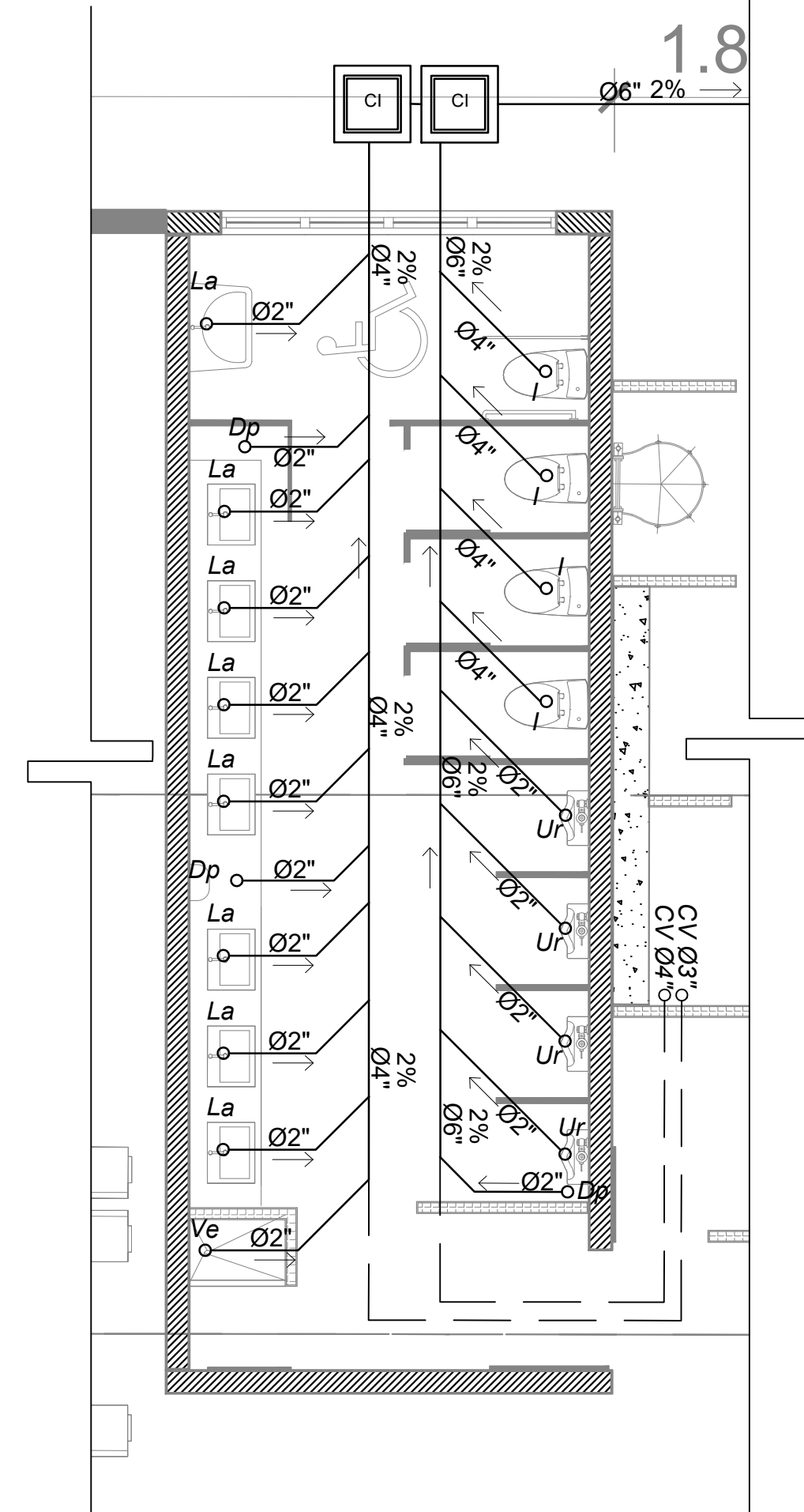
3 D-3 Baños Mujeres Esc. 1:50
