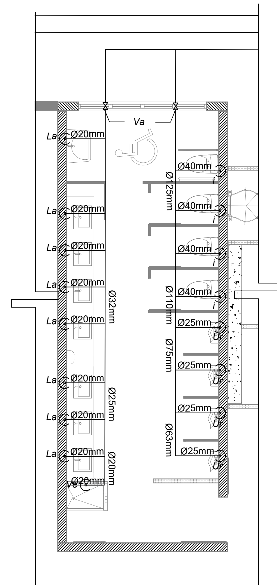
3 D-3 Baños Mujeres Esc. 1:50
