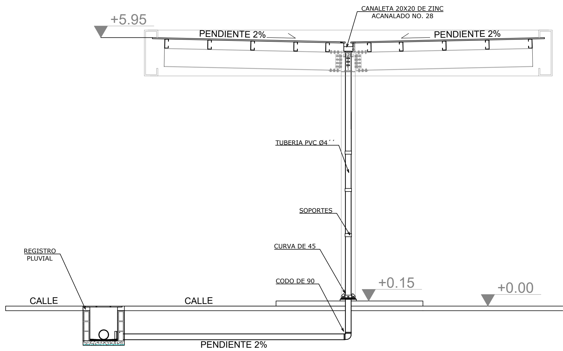
4 DETALLE SECCIÓN A-A. Esc. 1:40
