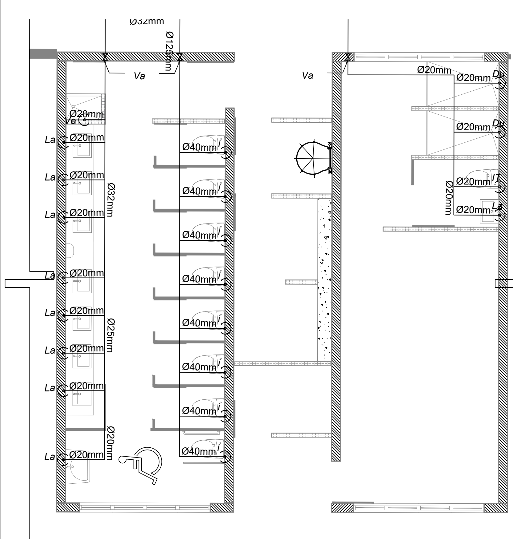
4 D-4 Baños Mujeres Esc. 1:50
