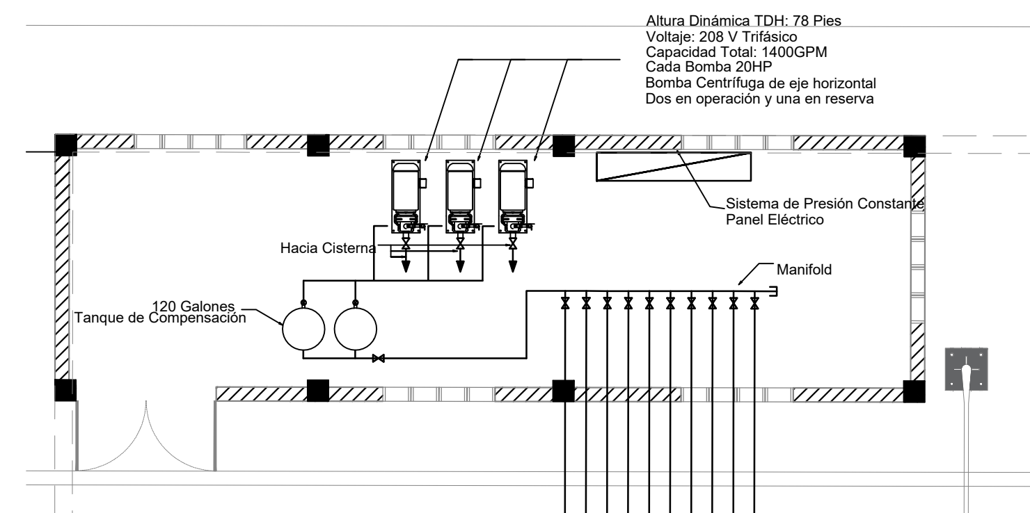
6 D-6 Cuarto de Bombas Esc. 1:75
