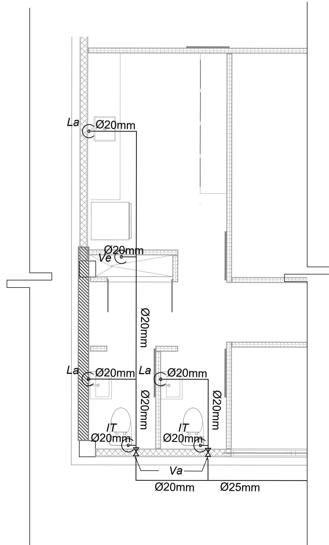
1 D-1 Baños Módulo Administrativo Esc. 1:40
