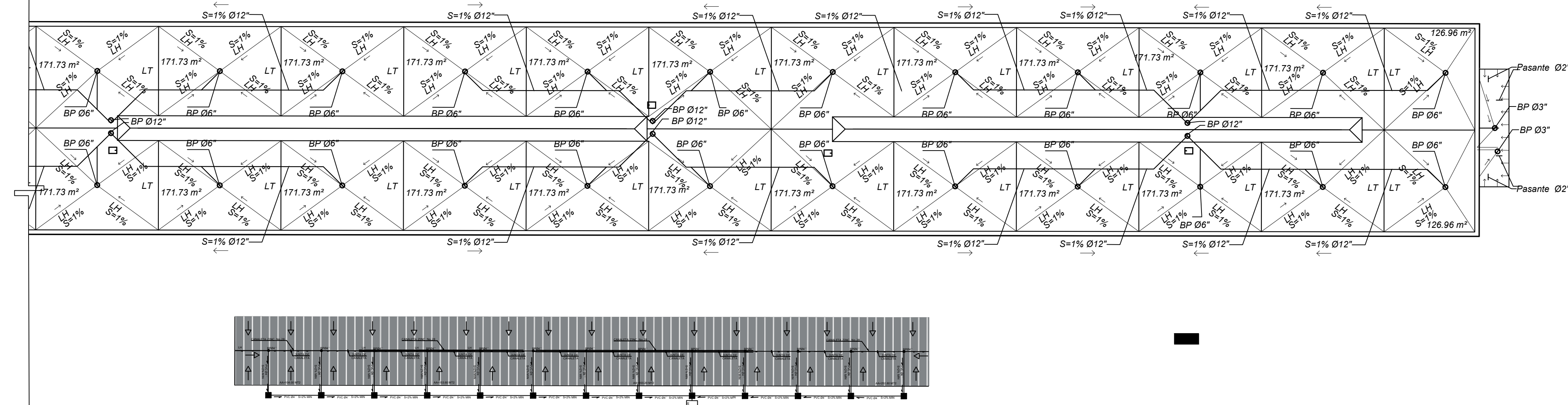
3 D-2 Planta Drenaje Pluvial Esc. 1:400
