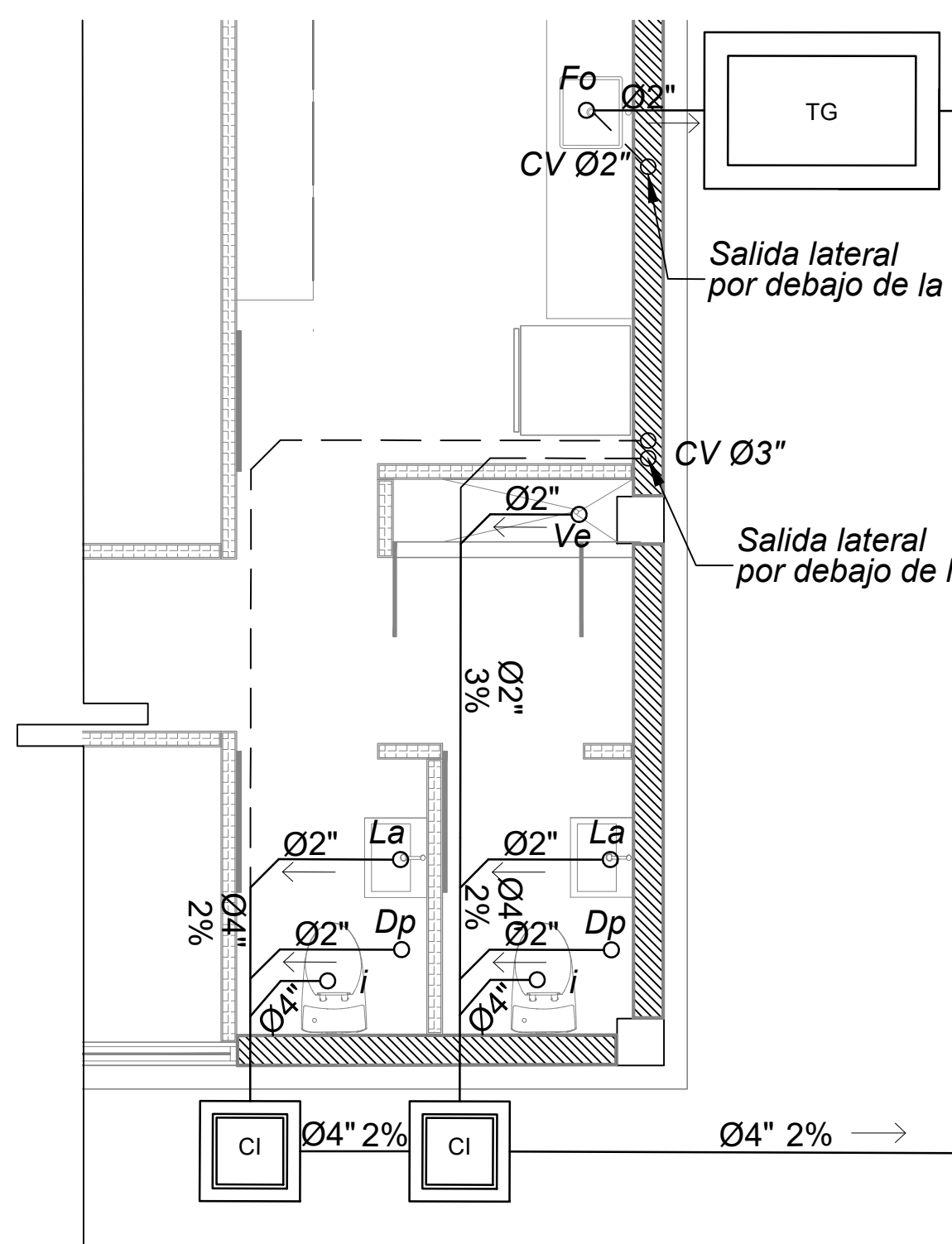
5 D-11 Baños Módulo Administrativo Esc. 1:40
