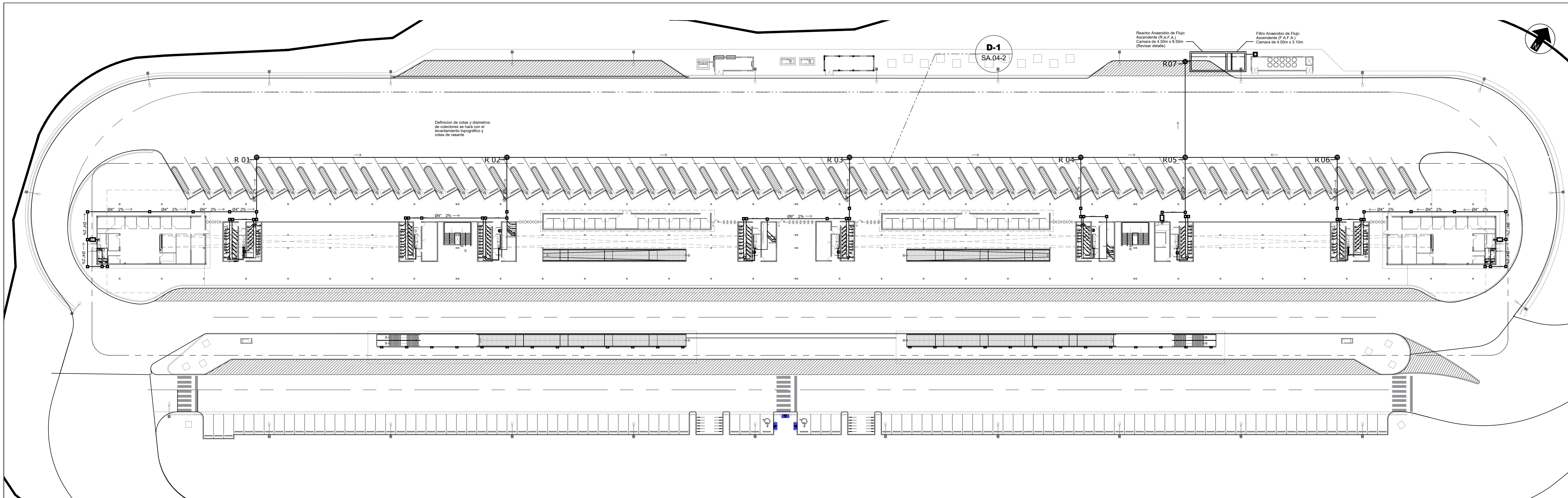
1 Sistema de Evacuación Aguas Negras Esc. 1:500
