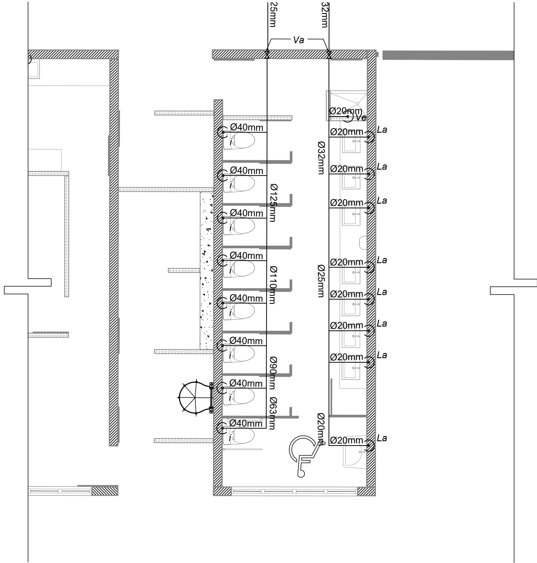
3 D-9 Baño Mujeres Esc. 1:50
