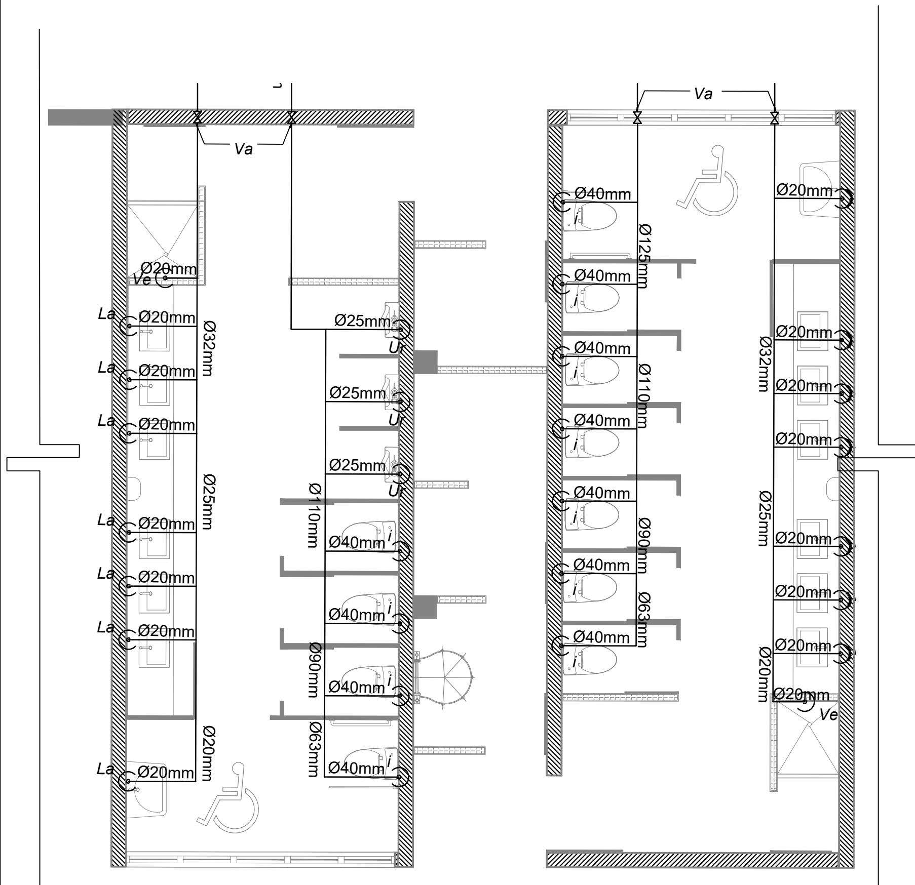
4 D-10 Baño Hombres y Mujeres Esc. 1:50
