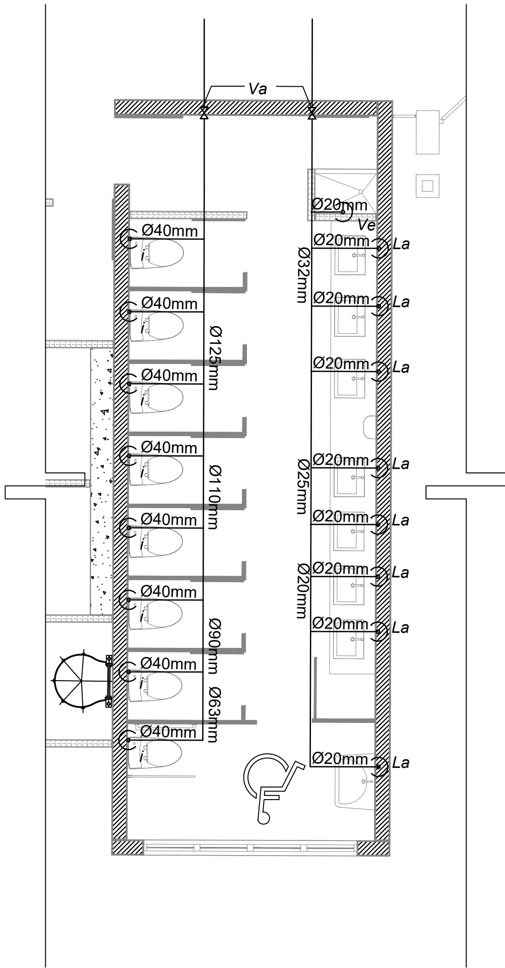
1 D-7 Baño Mujeres Esc. 1:50
