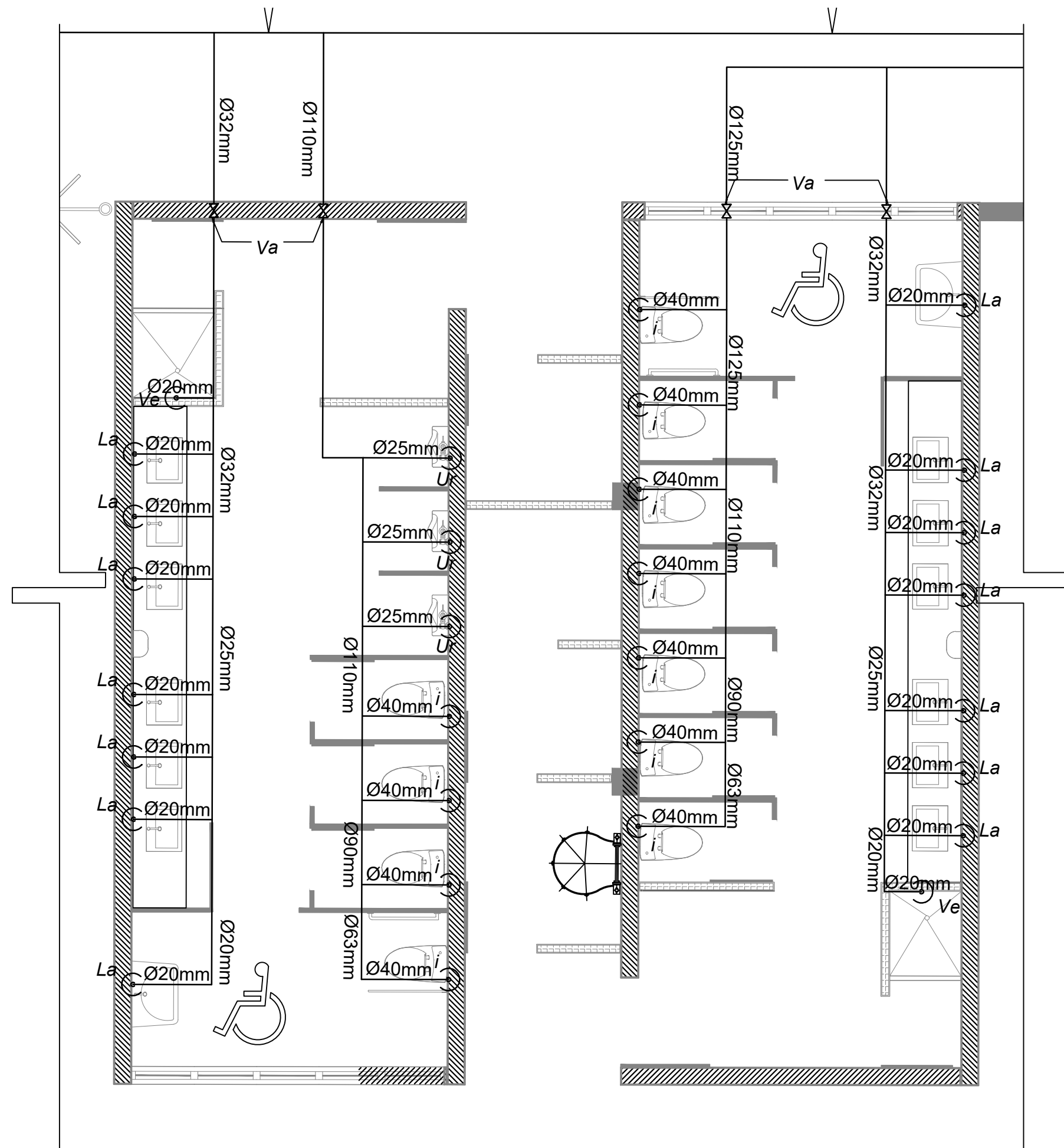
2 D-2 Baños Hombres y Mujeres Esc. 1:50
