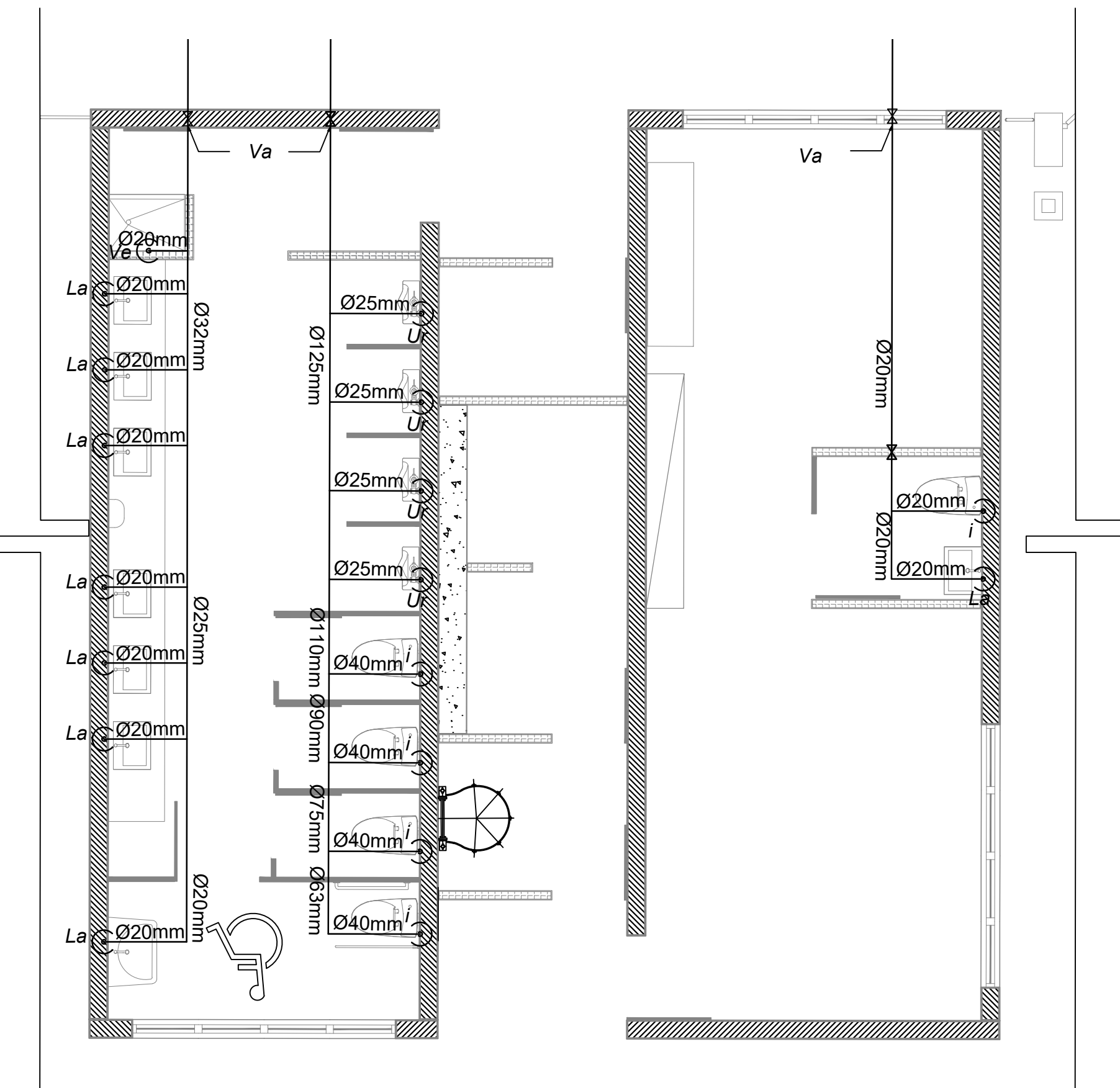
5 D-5 Baño Mujeres Esc. 1:50
