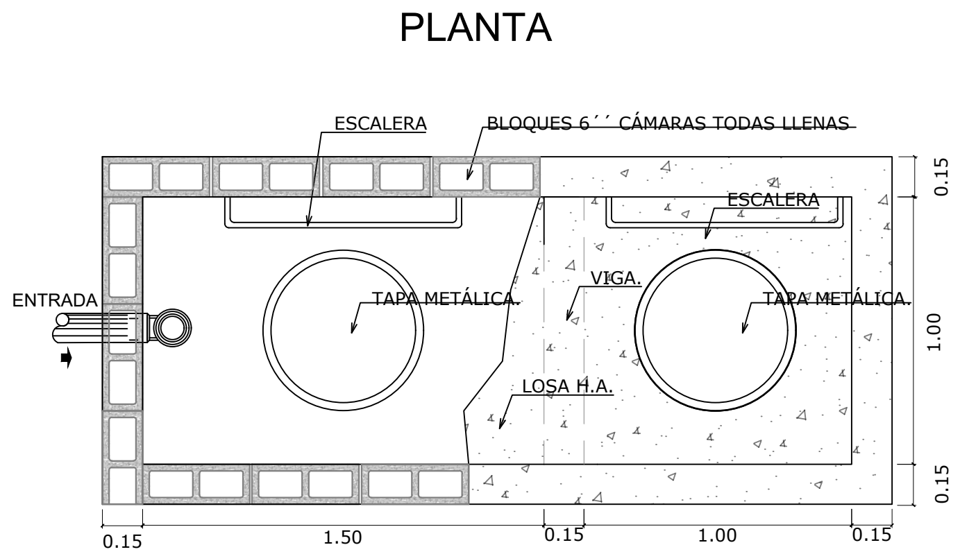
5 DETALLE DESARENADOR. Esc. 1:20
