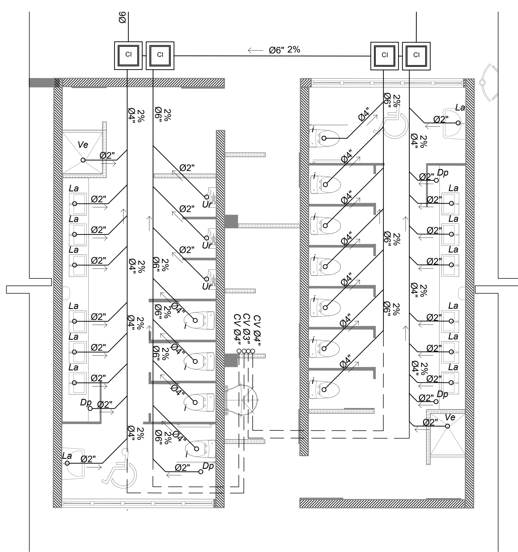
2 D-8 Baños Hombres Esc. 1:50
