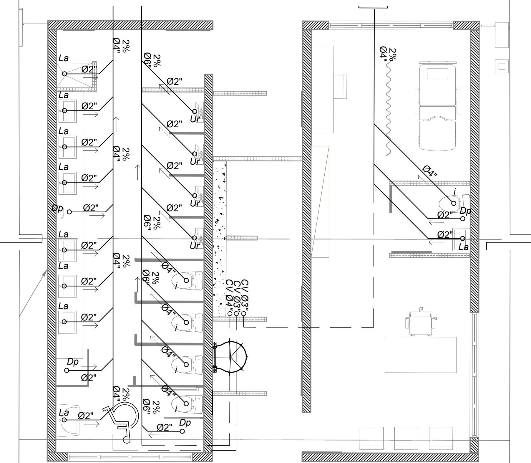
5 D-5 Baño Mujeres Esc. 1:50
