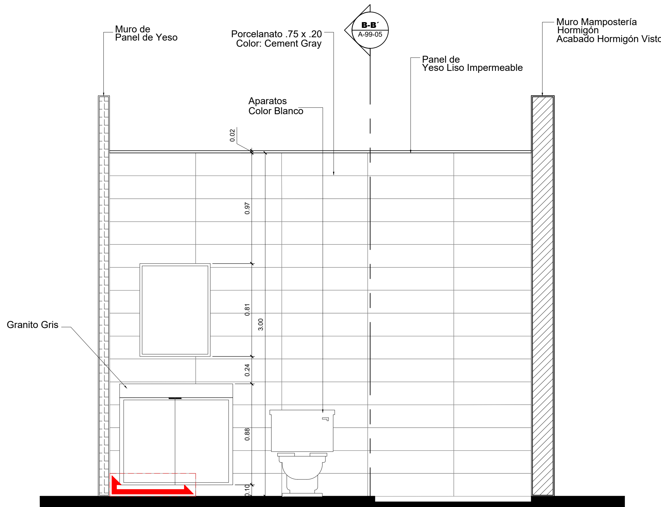
4 Sección A-A' Esc. 1: 20
