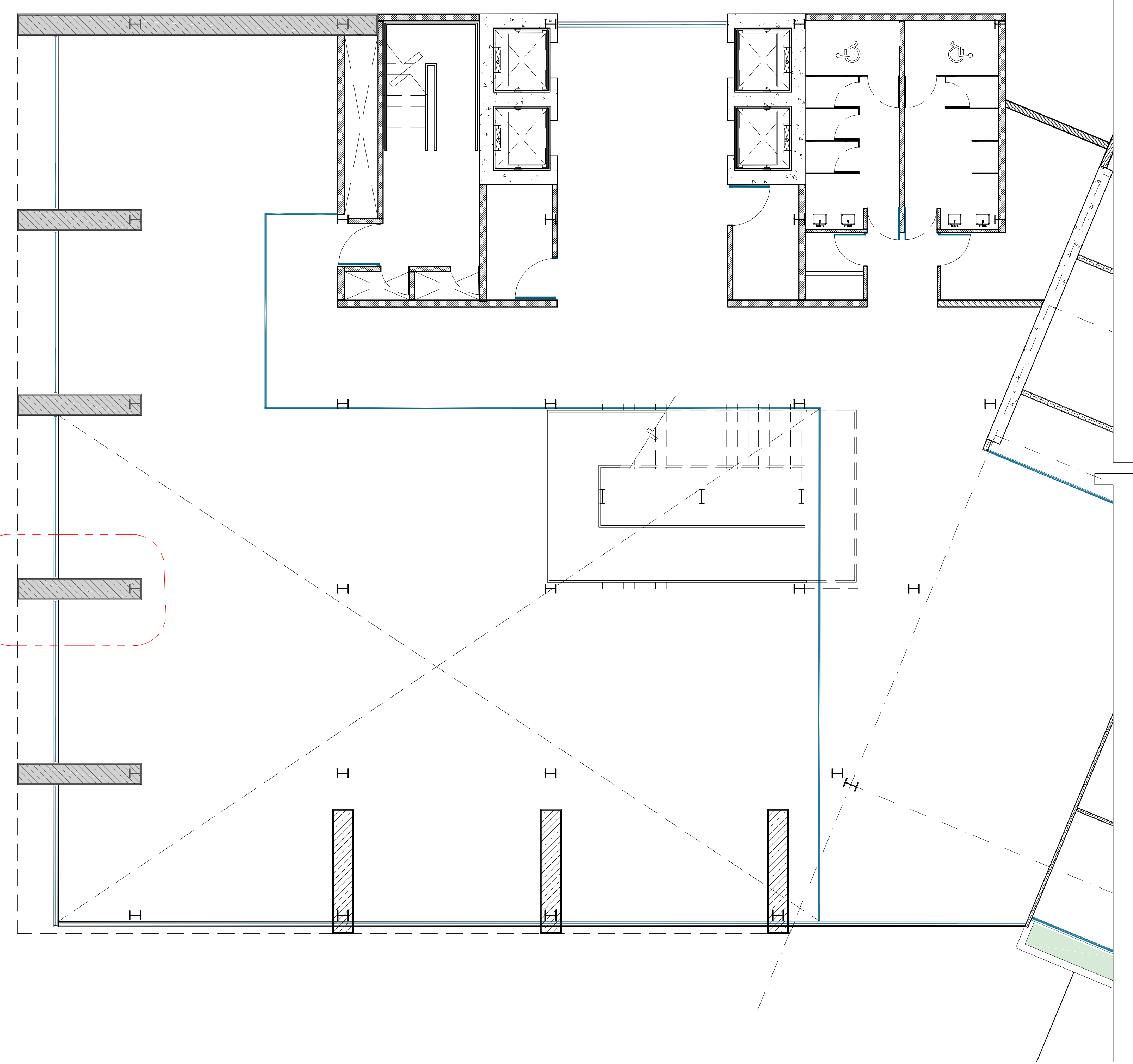
1 Planta Muros Bloque 1- Nivel 4 Esc. 1:75
