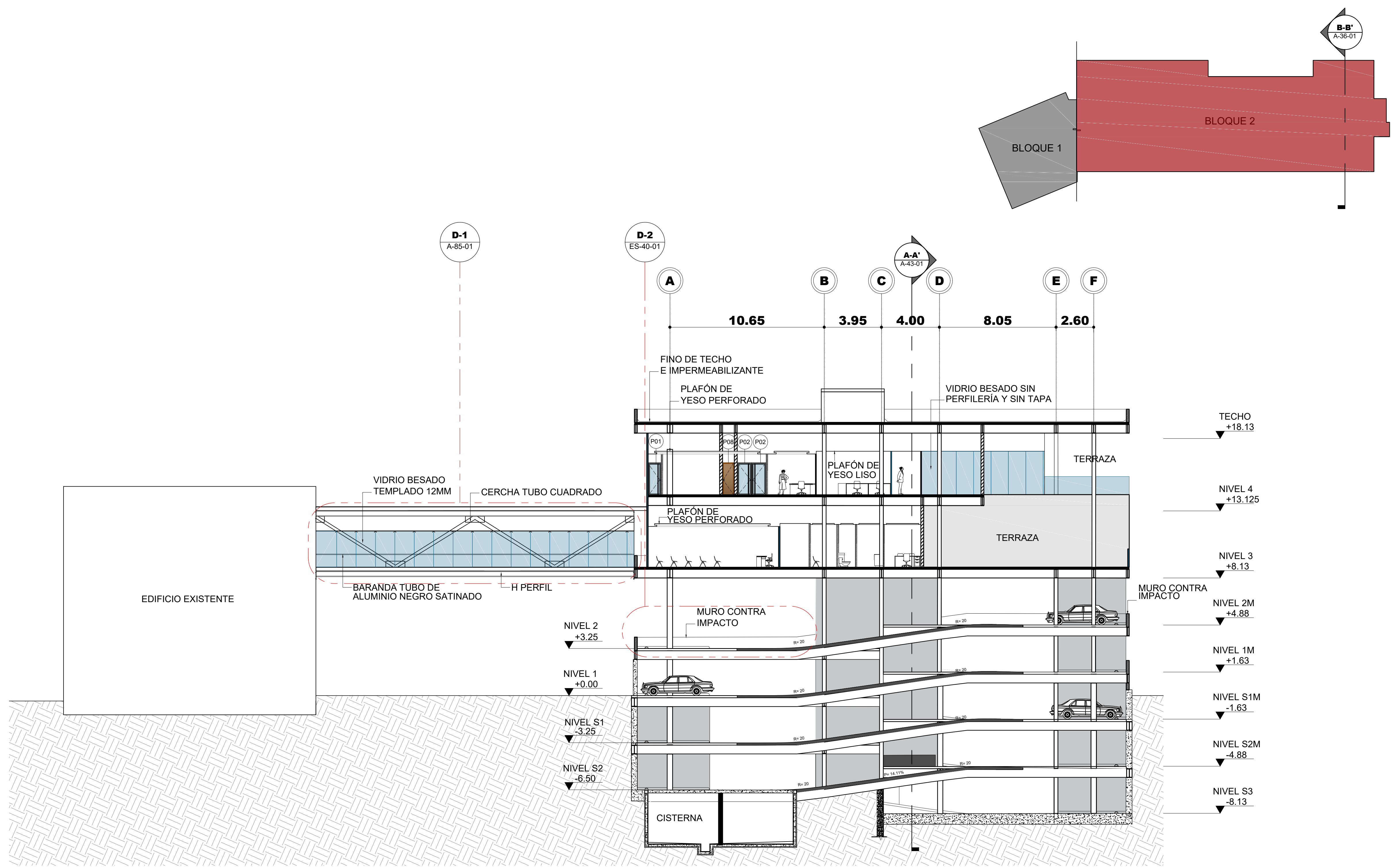
1 Sección Transversal B-B' Esc. 1:150
