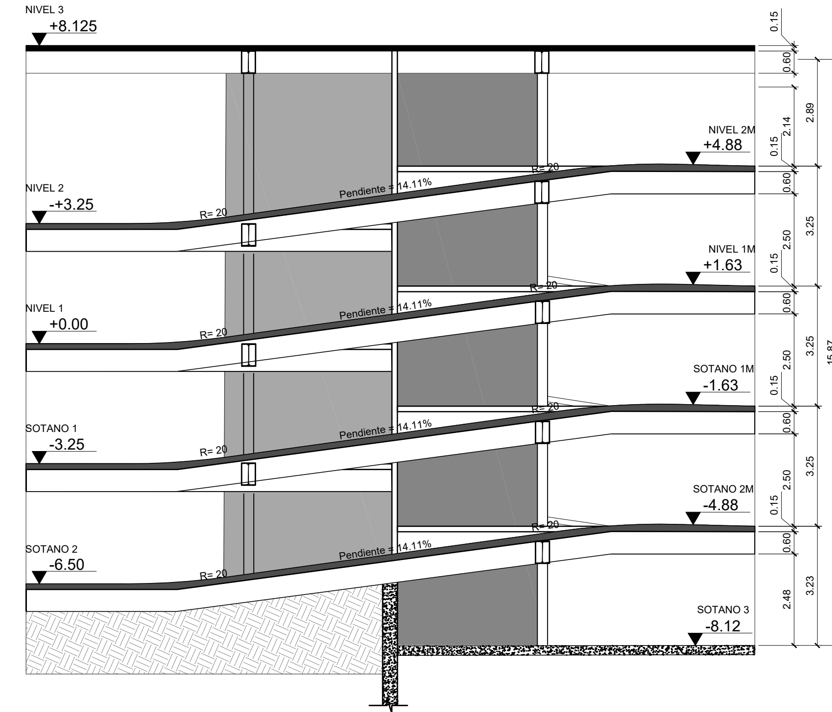
3 Sección de Detalle Rampa 3 - Bloque 2 Esc. 1:100
