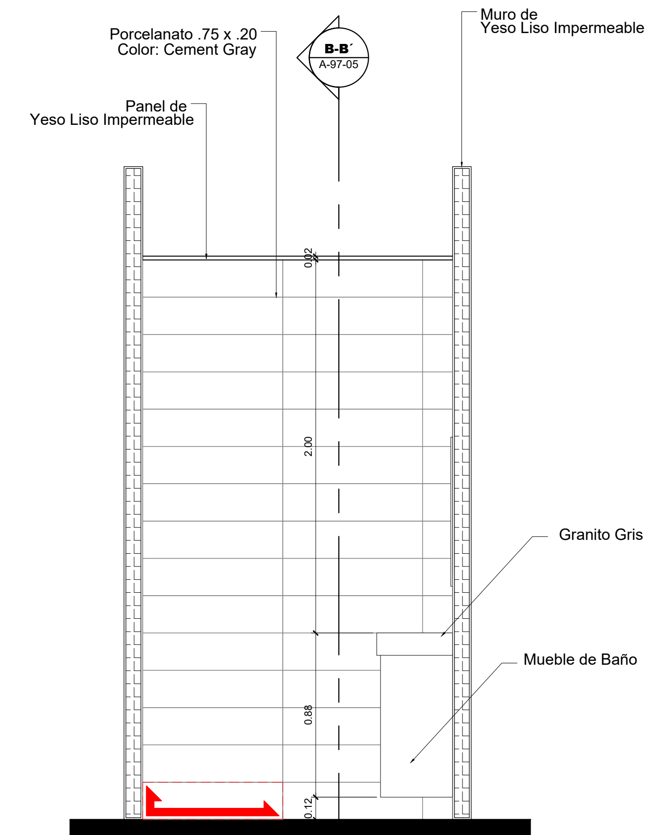
6 Sección C-C' Esc. 1: 20
