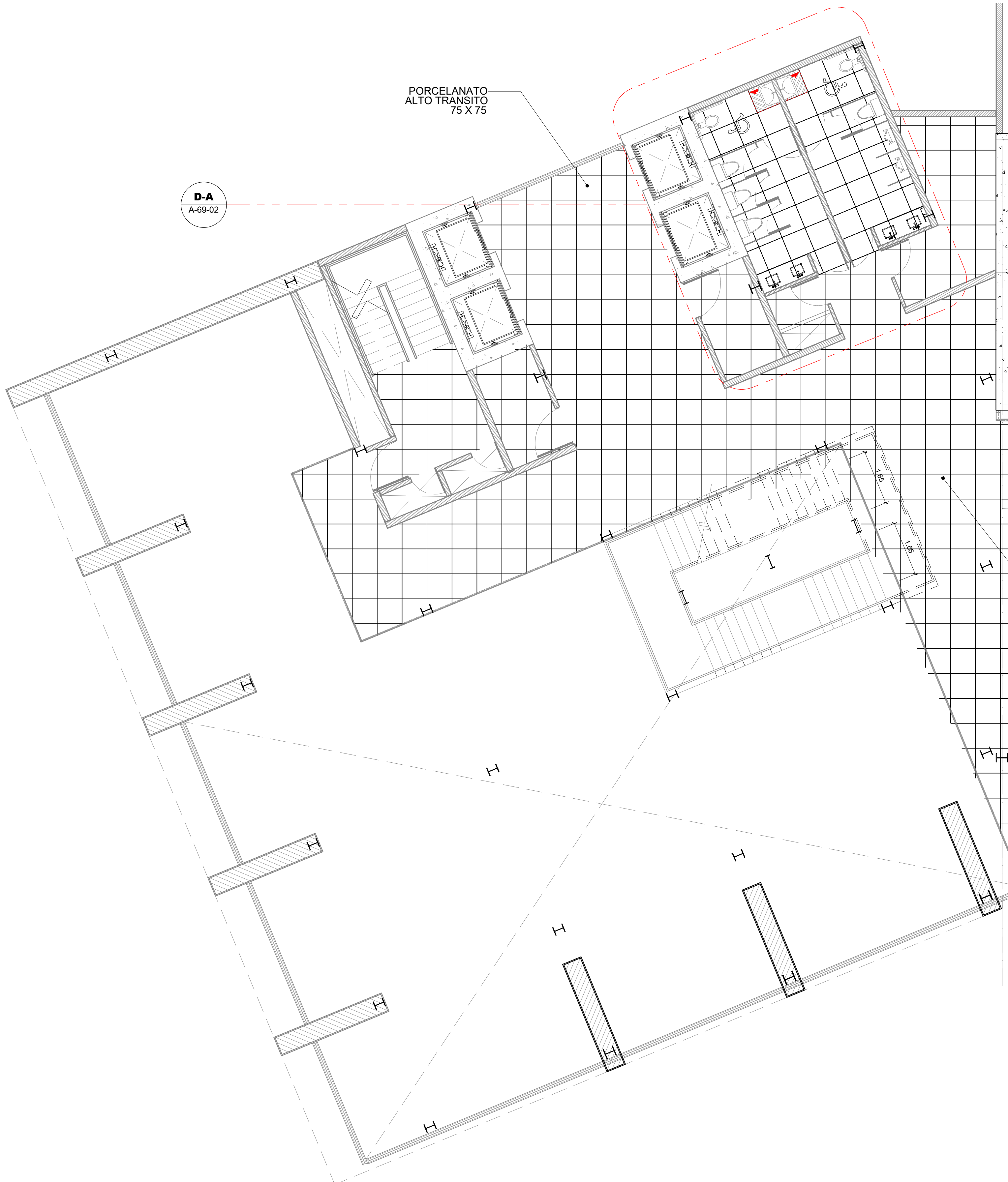
1 Planta Pisos - Bloque 1 - Nivel 4 Esc. 1:200
