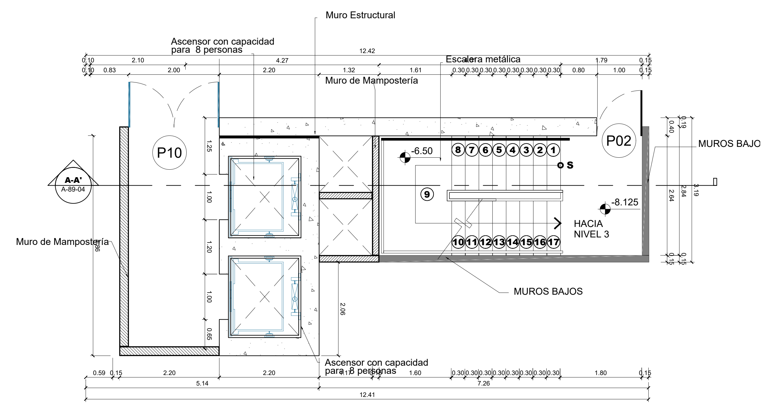
1 Planta Núcleo C - Sótano 3M a N3 Escalera metálica Esc. 1:50
