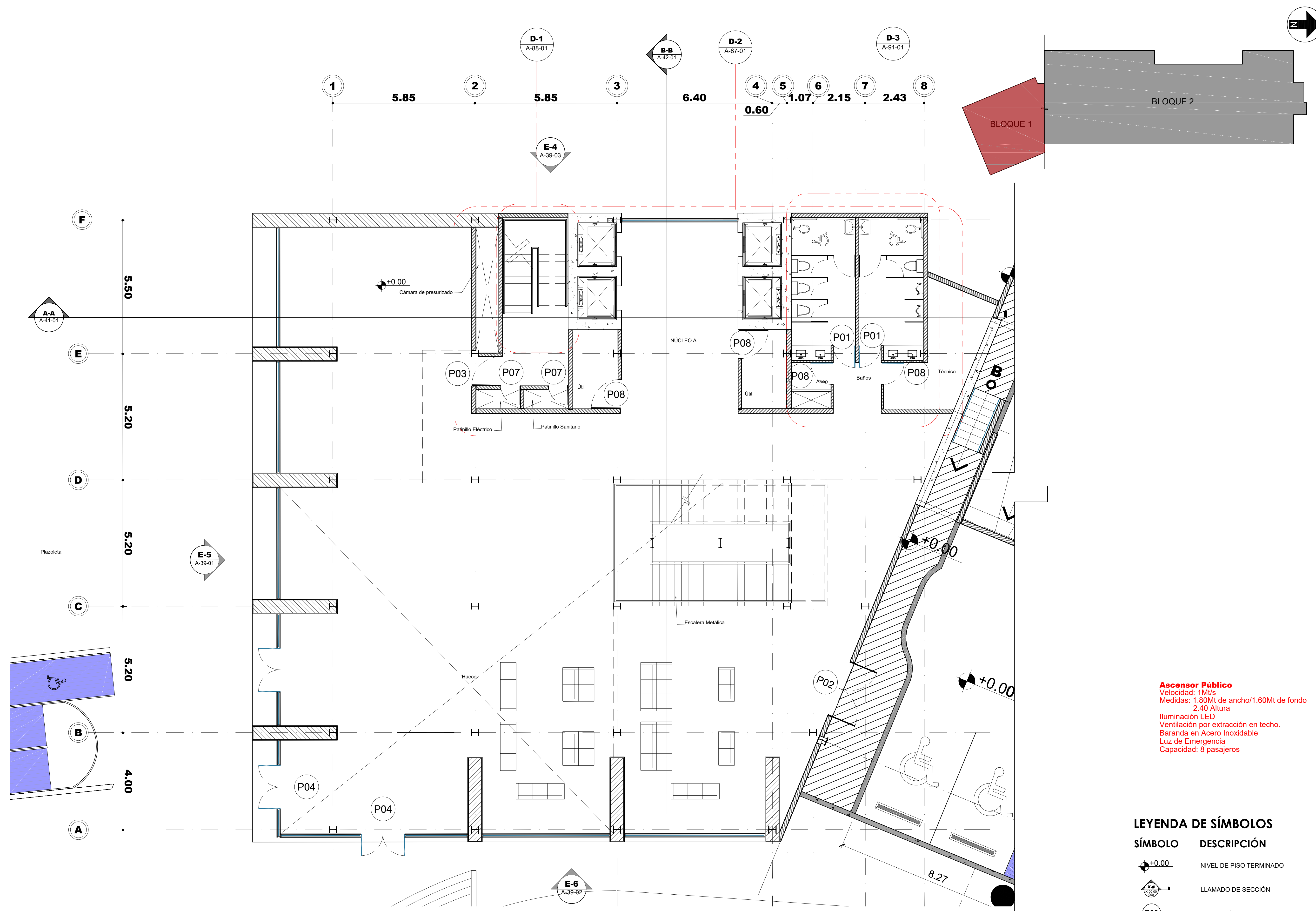
1 Planta Amueblada - Nivel 1 - Bloque 1 Esc. 1:75
