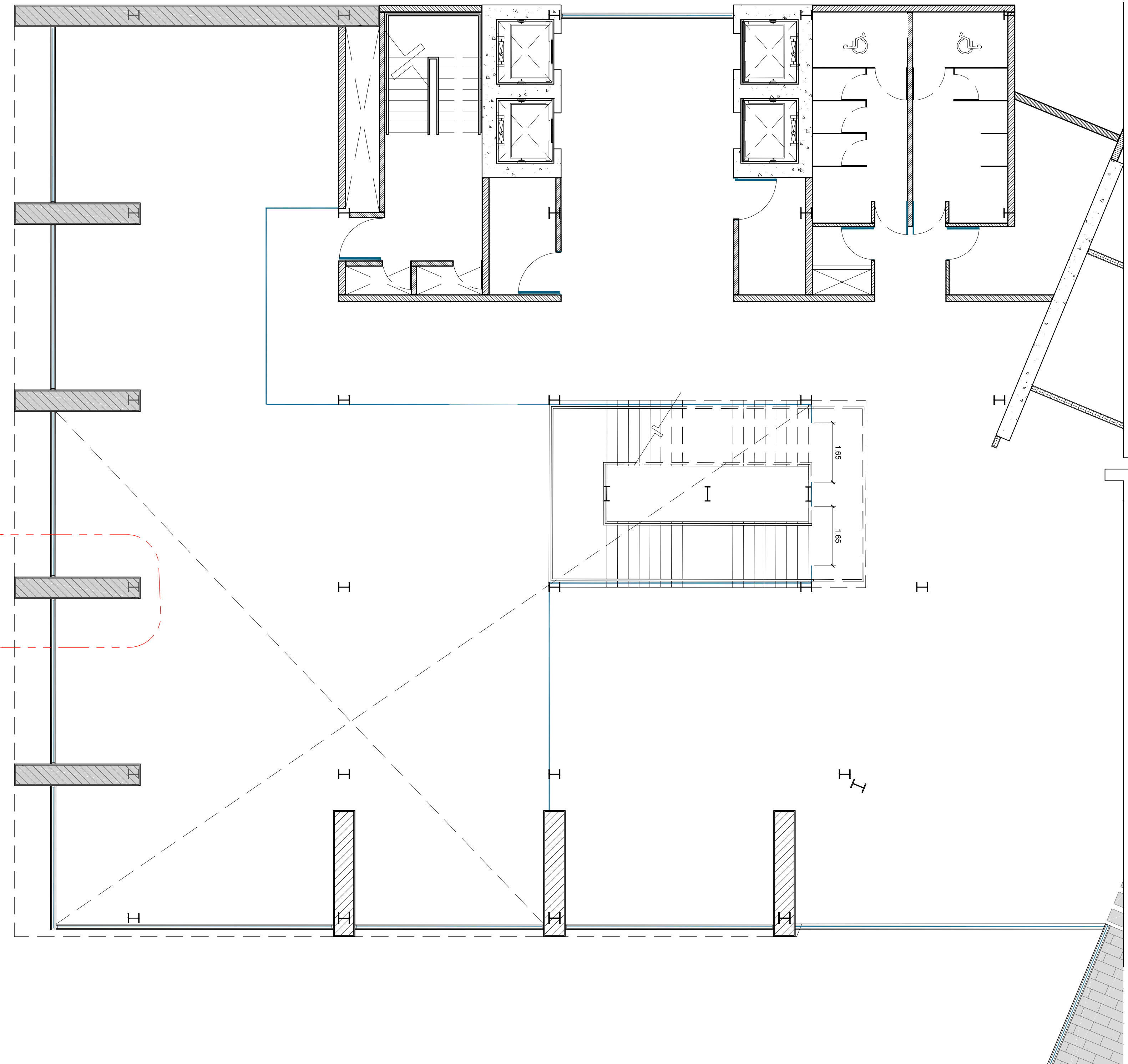
1 Planta Muros Bloque 1 - Nivel 3 Esc. 1:75
