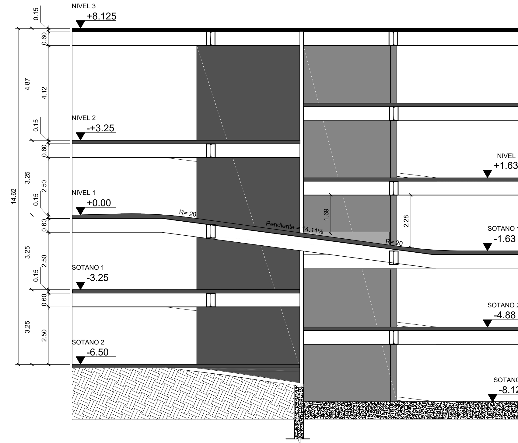
2 Sección de Detalle Rampa 2 - Bloque 2 Esc. 1:100
