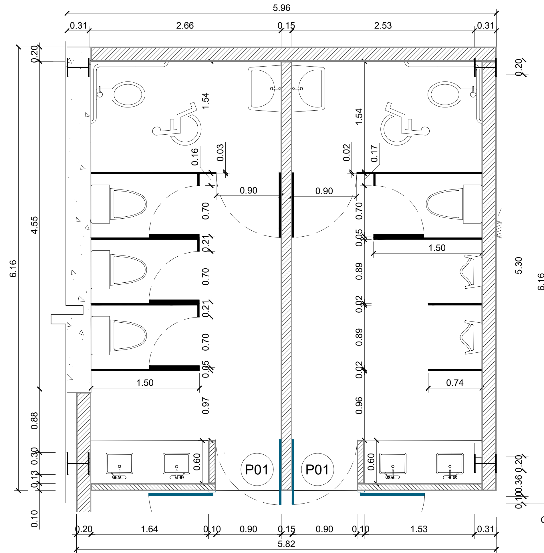
3 Planta Dimensionada - Baños Esc. 1: 30
