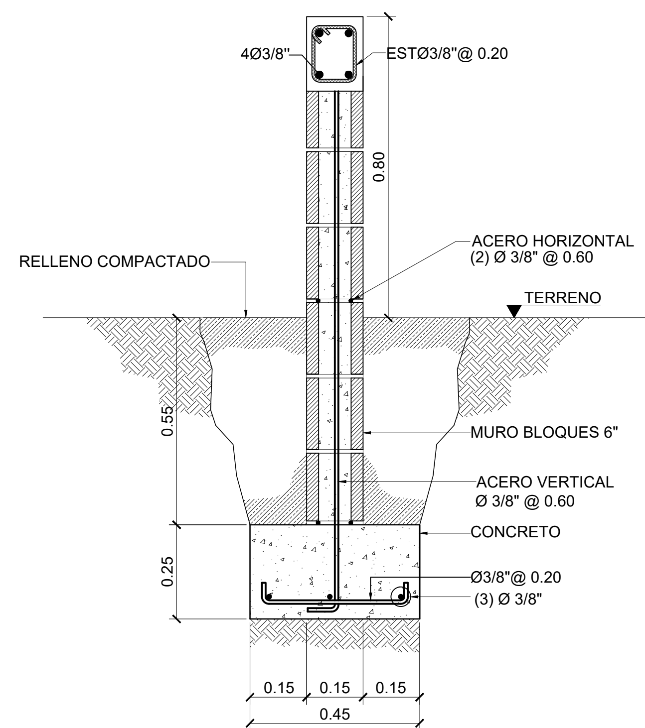
3 Detalle de Muro Perimetral Esc. 1:10
