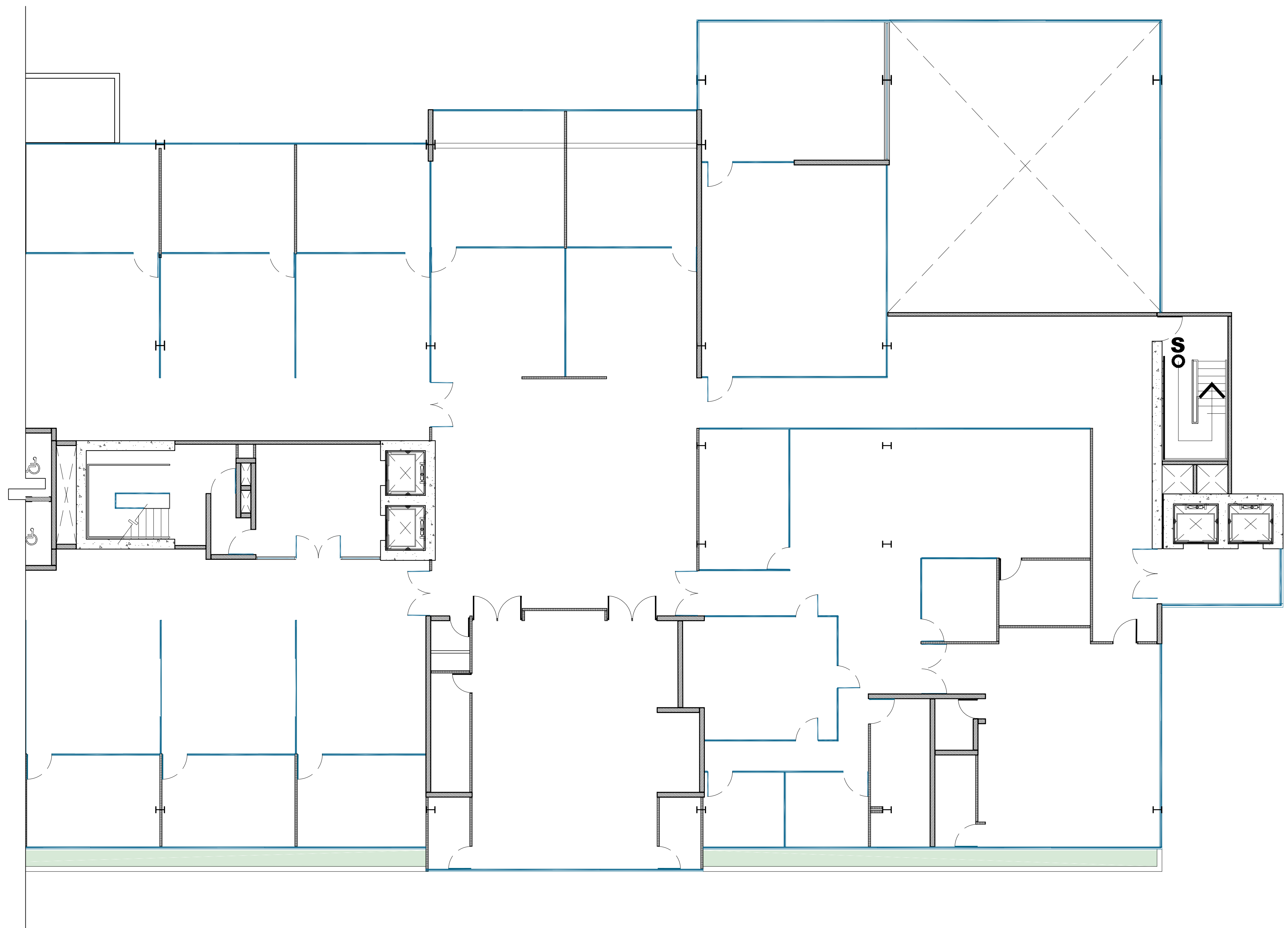
1 Planta Muros Bloque 2B - Nivel 4 Esc. 1:100
