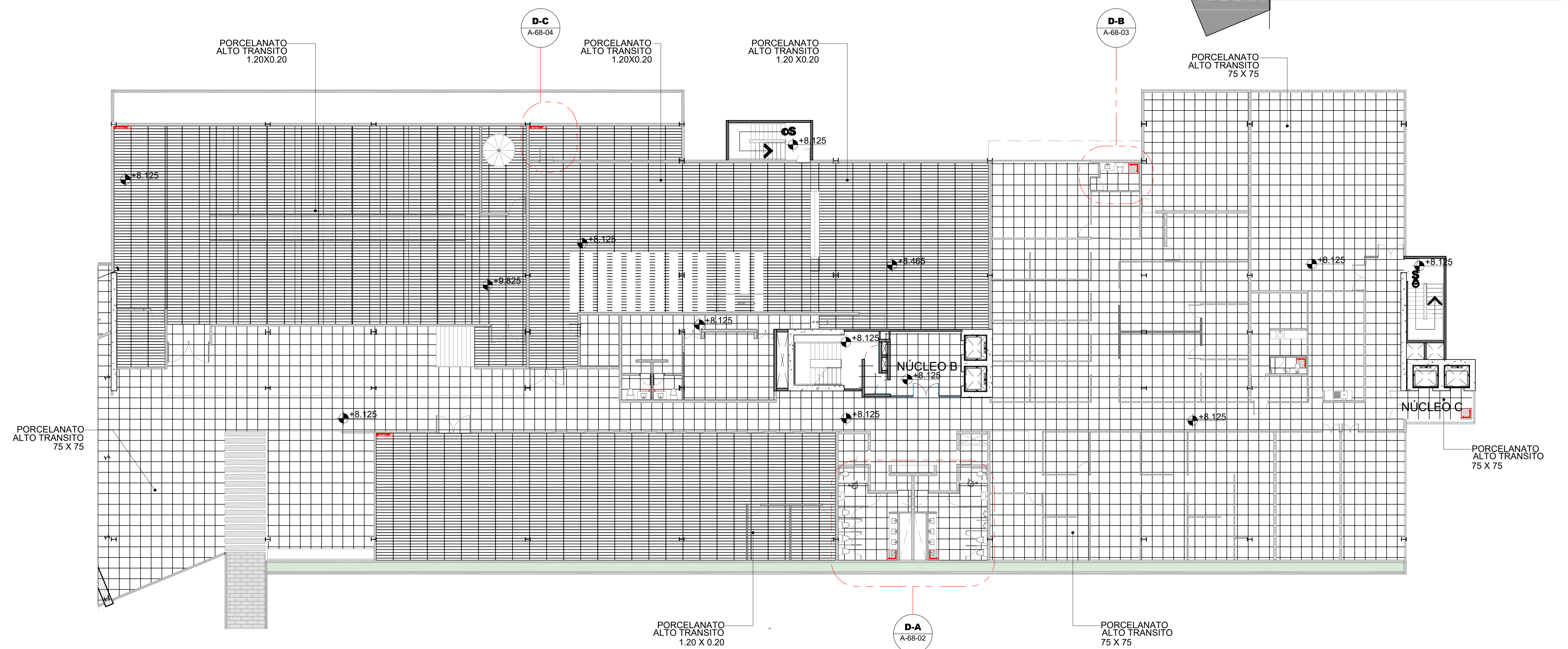
1 Planta Pisos - Bloque 2 - Nivel 3 Esc. 1:150
