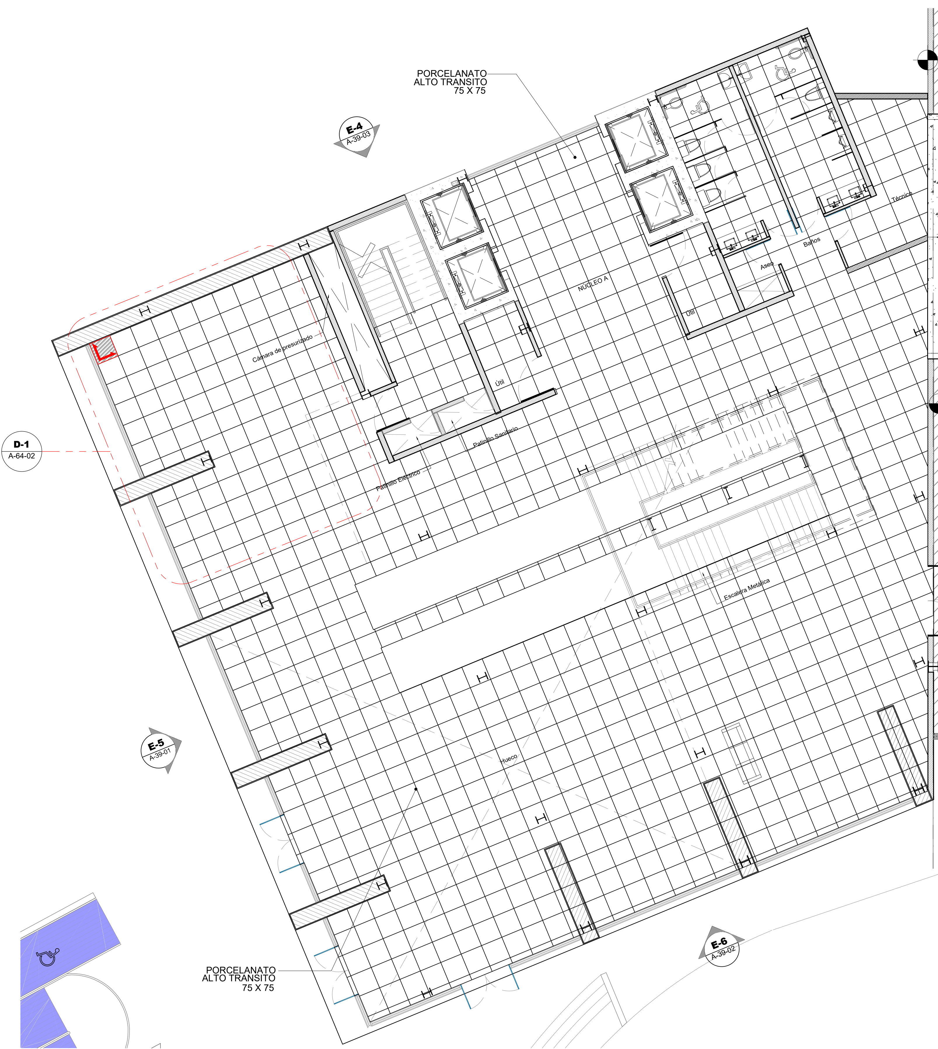
1 Planta Pisos - Bloque 1 - Nivel 1 Esc. 1:75
