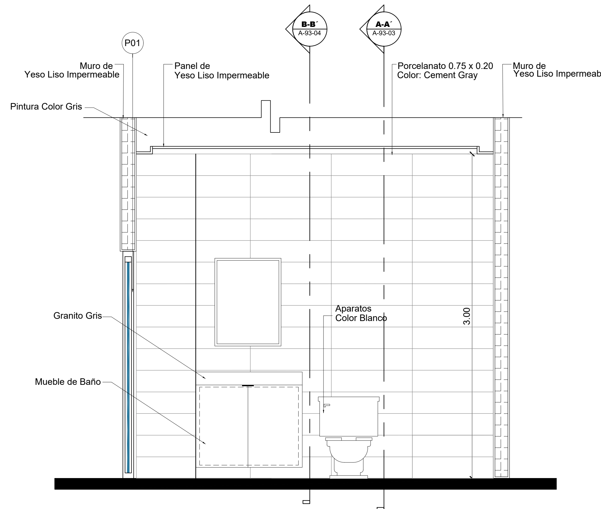
5 Sección C-C' Esc. 1: 20
