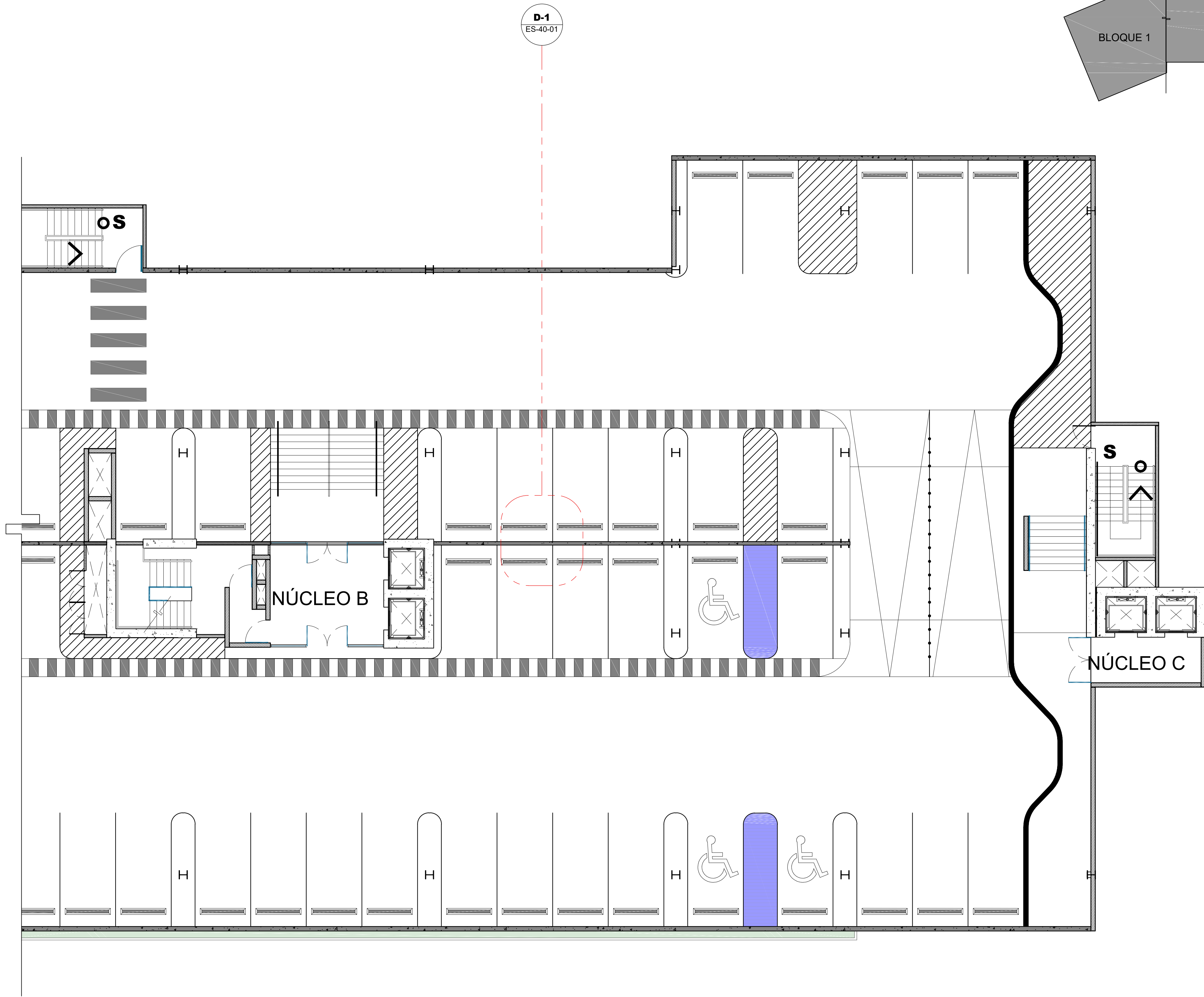
1 Planta Muros Bloque 2B - Nivel 2 Esc. 1:100
