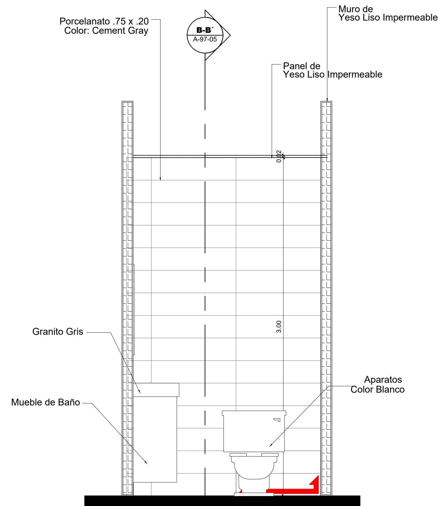
4 Sección A-A' Esc. 1: 20
