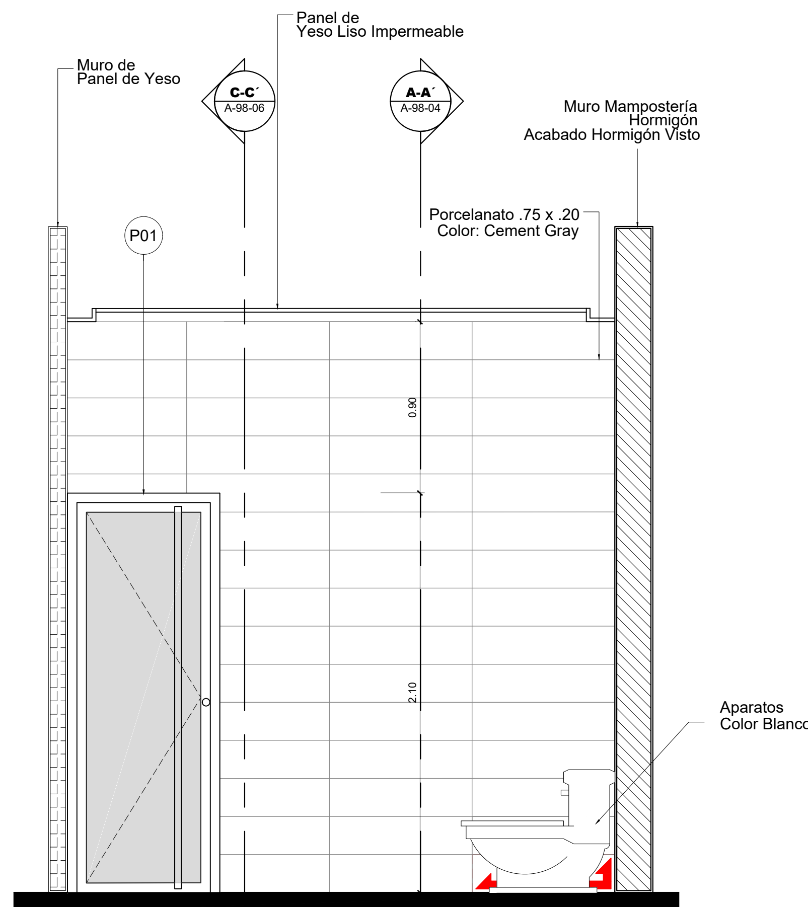
5 Sección B-B' Esc. 1: 20
