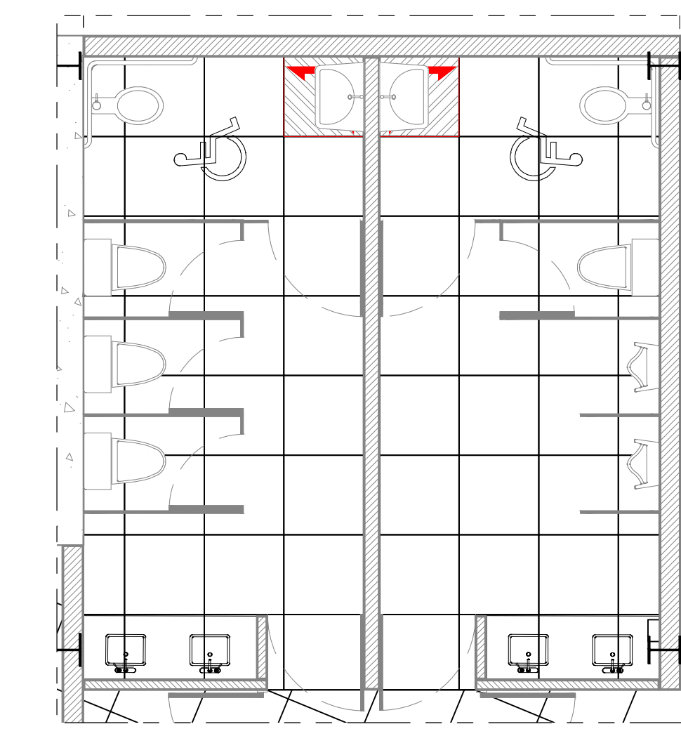
2 Detalle A Esc. 1:50
