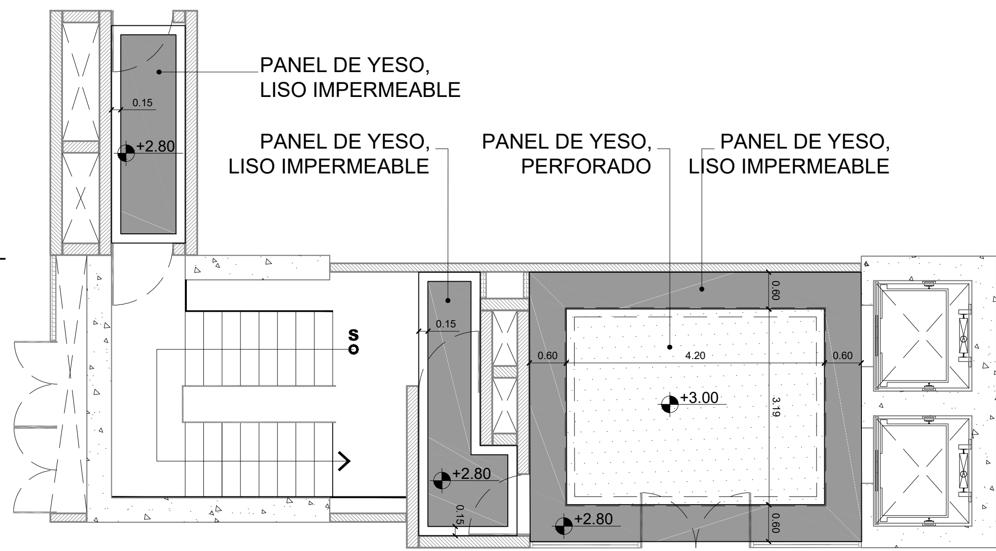
3 Detalle 2, Planta de Plafón, Nucleo B Esc. 1:60
