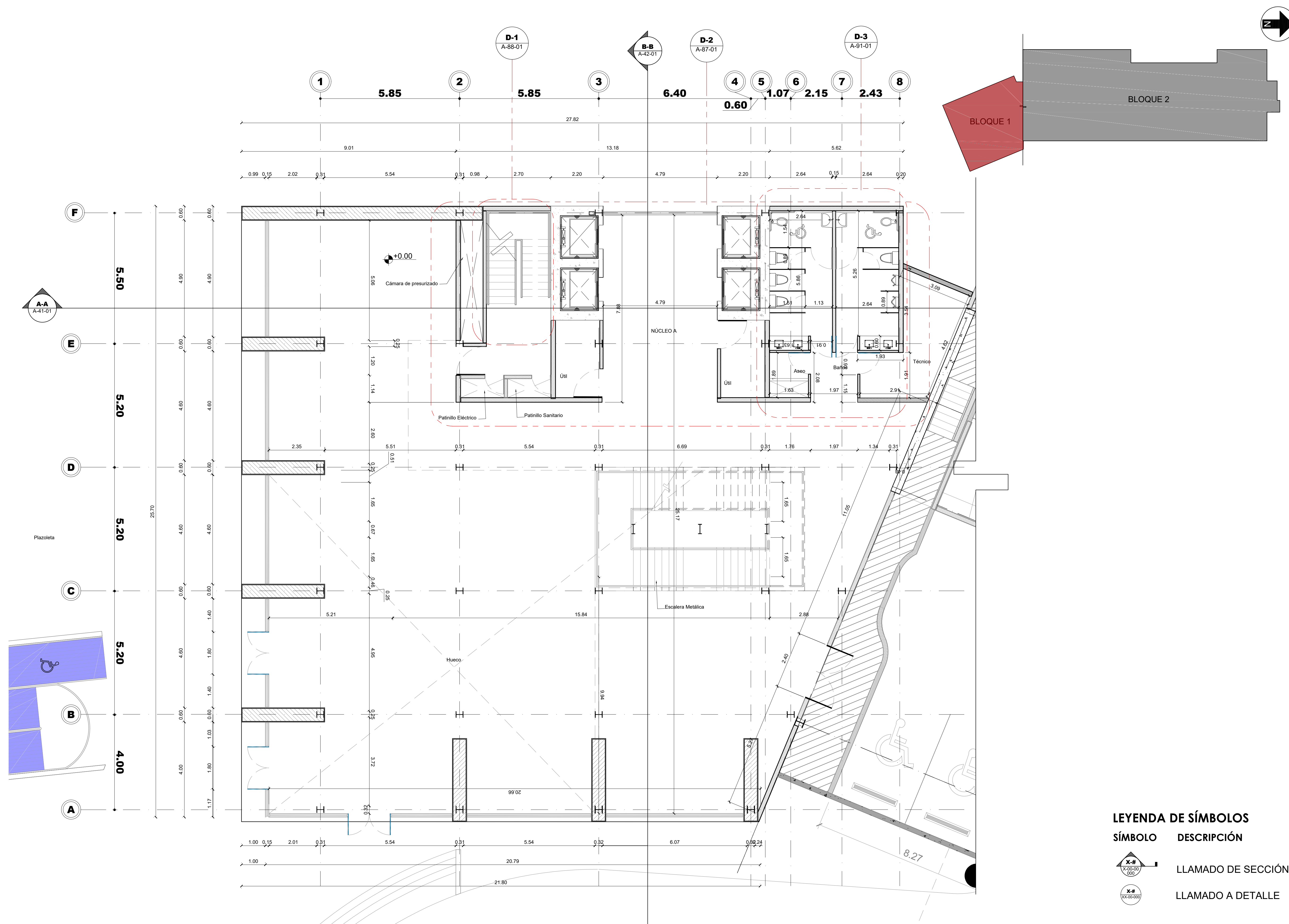
1 Planta Dimensionada - Bloque 1- Nivel 1 Esc. 1:75
