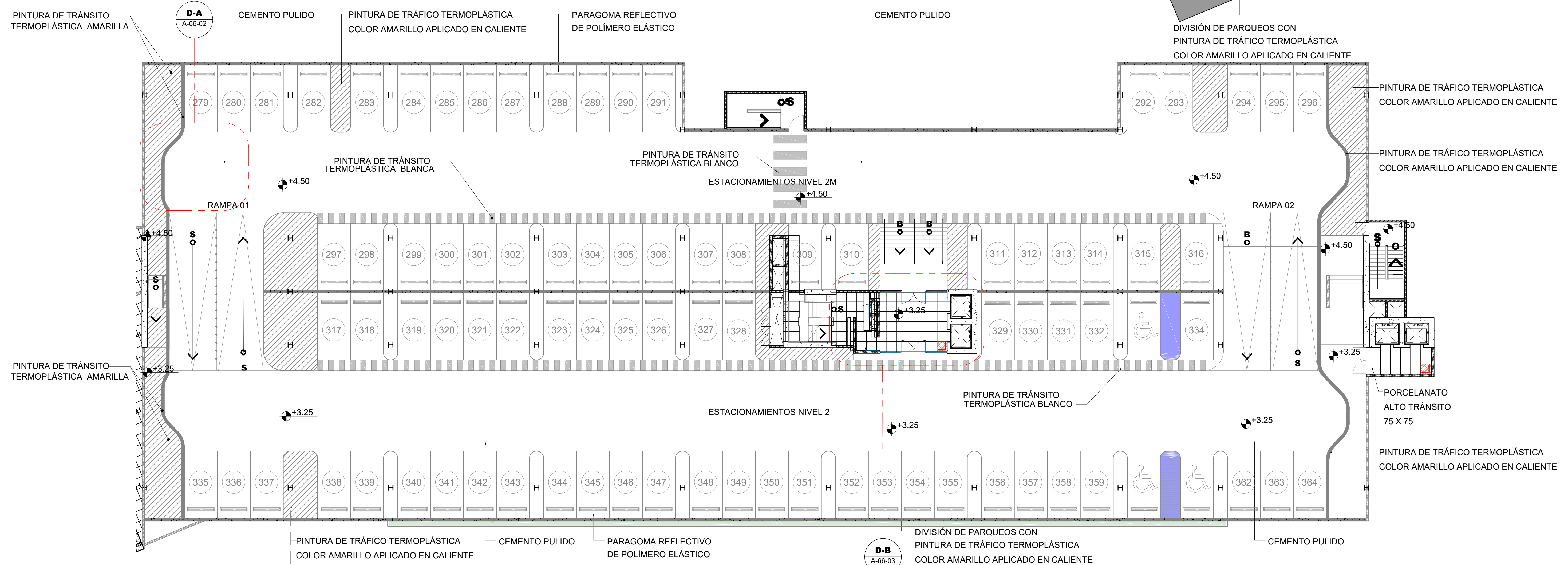
1 Planta Pisos - Bloque 2 - Nivel 2 Esc. 1:150
