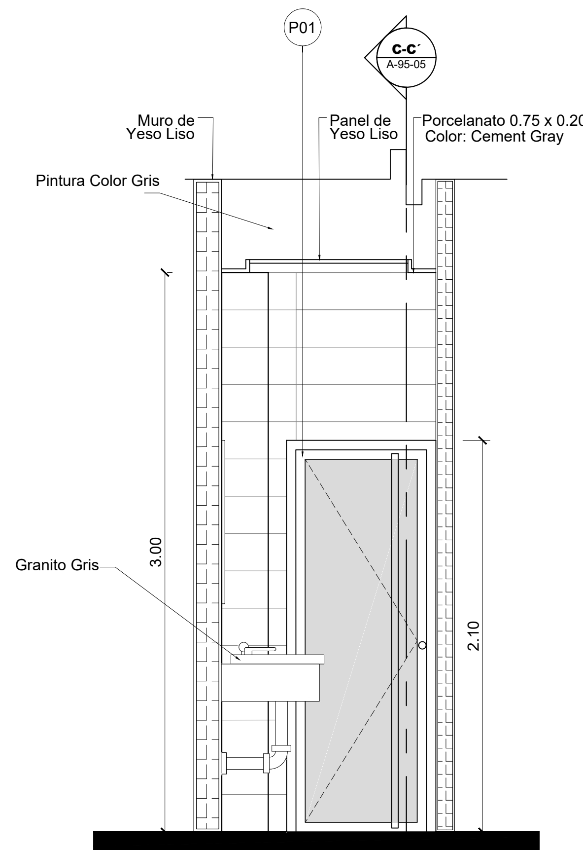
4 Sección B-B' Esc. 1: 20
