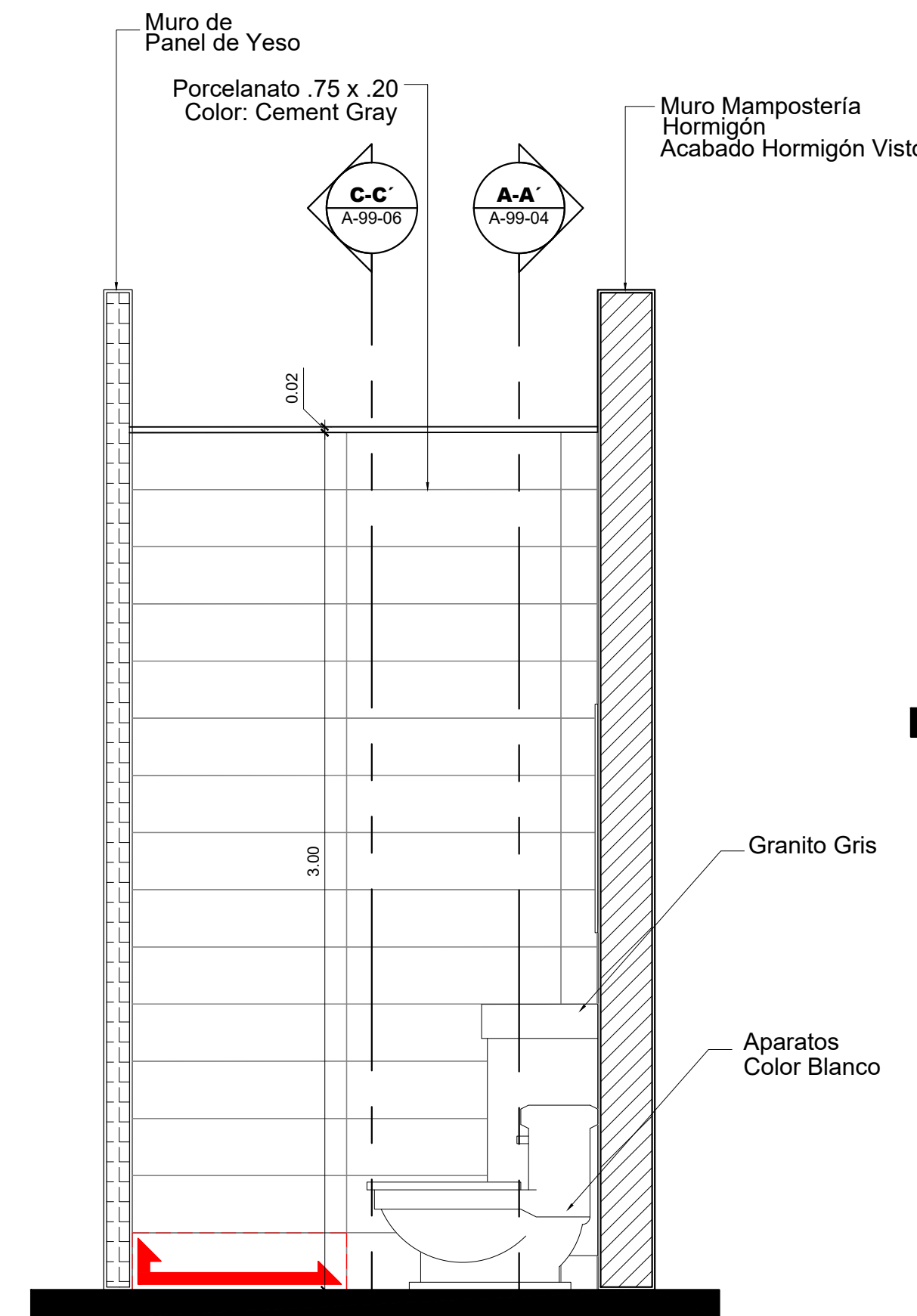
5 Sección B-B' Esc. 1: 20
