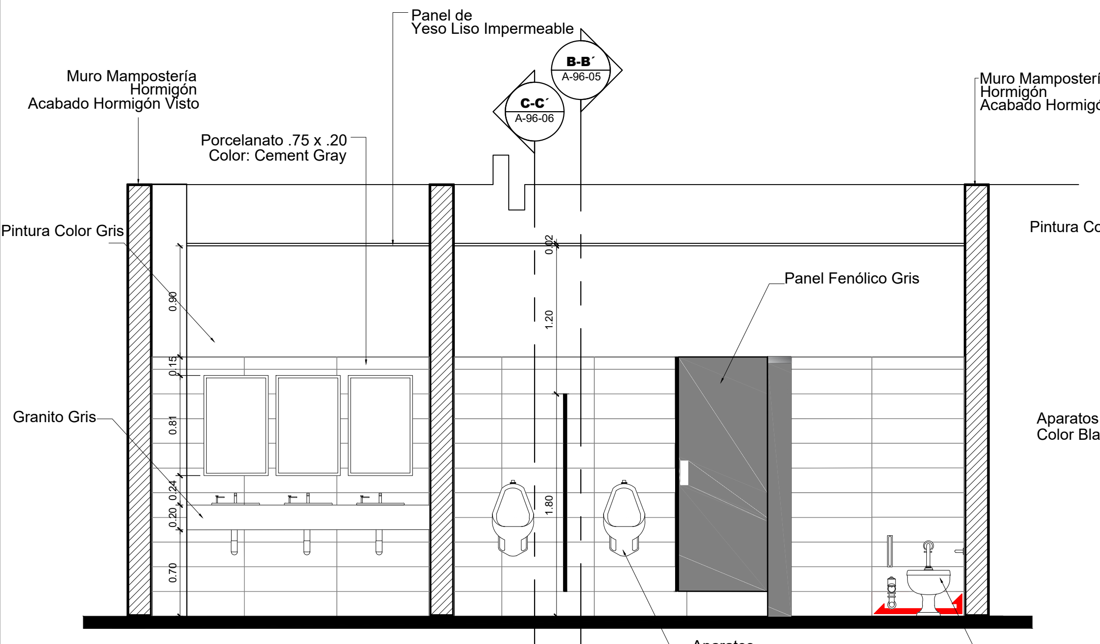
4 Sección A-A' Esc. 1: 30
