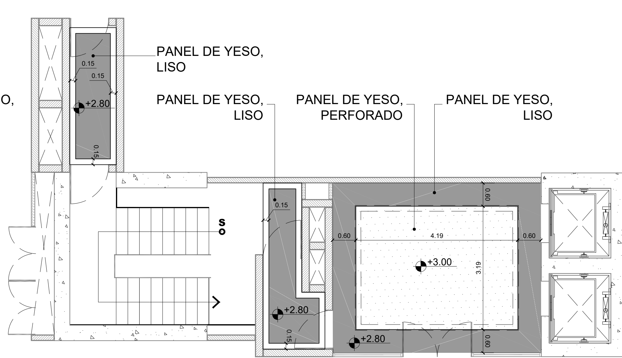
3 Detalle 2, Planta de Plafón, Nucleo B Esc. 1:60
