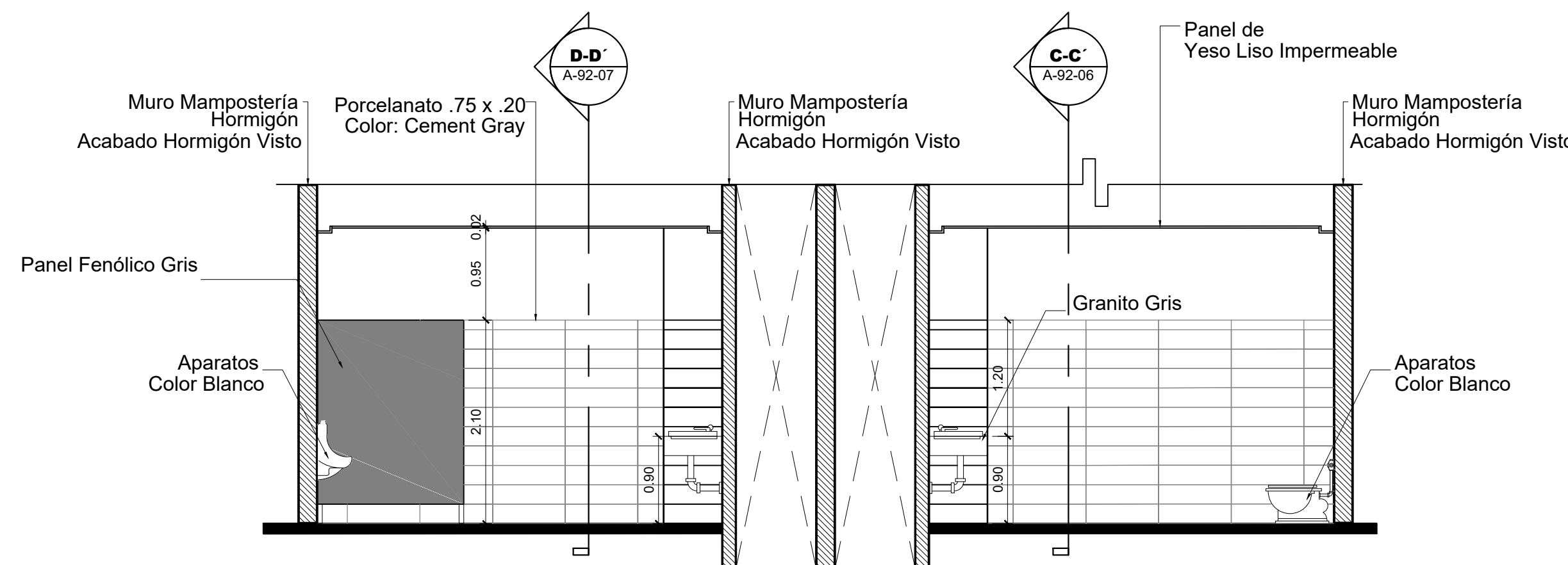
5 Sección B-B' Esc. 1: 50
