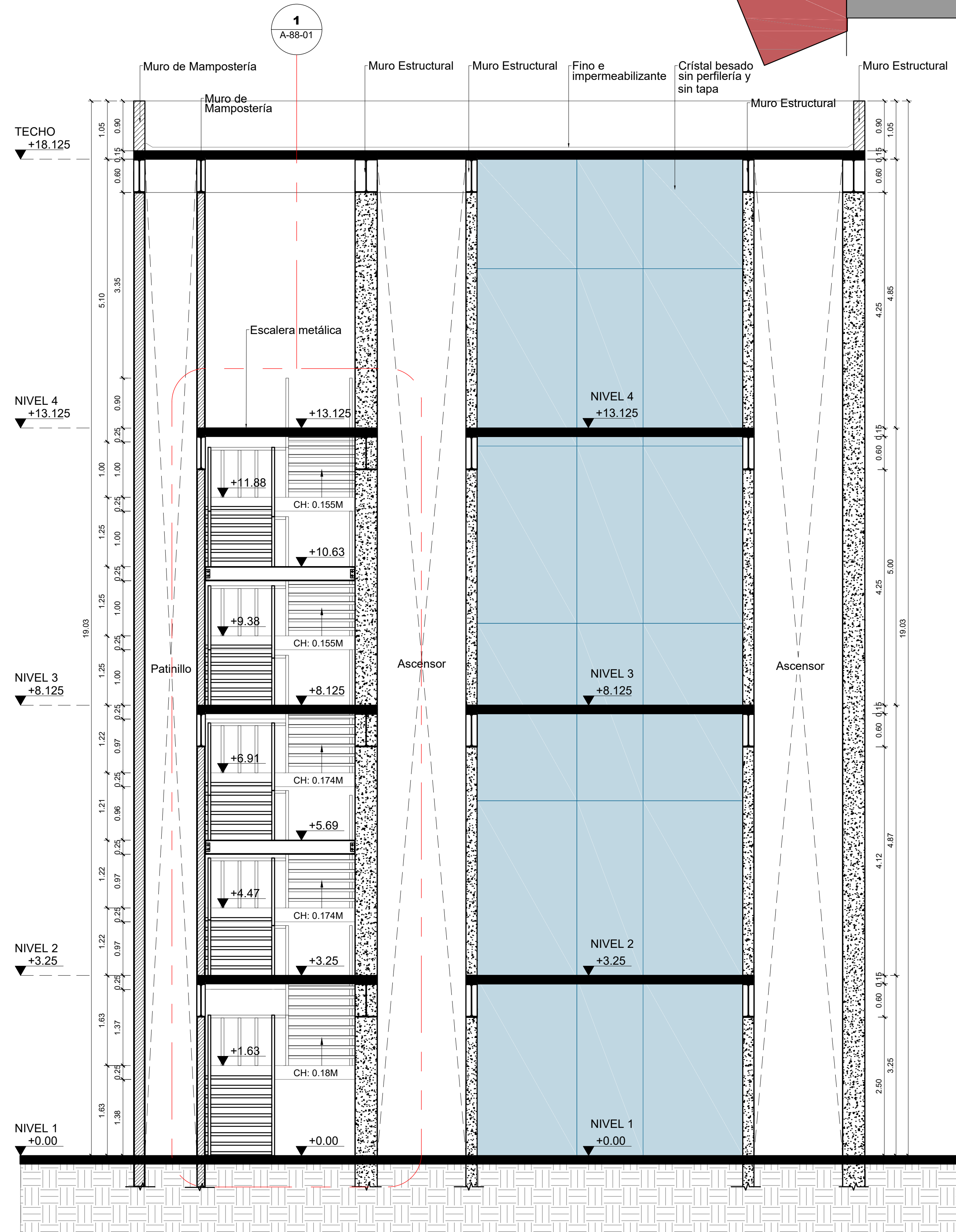
4 Sección A-A' Núcleo A - N1 a N4 Esc. 1:50
