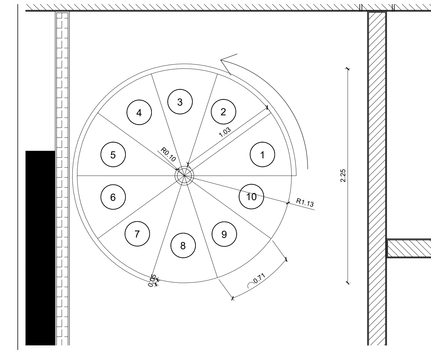
7 Detalle Escalera Metálica en Auditorio, N3-N4 Esc. 1:25
