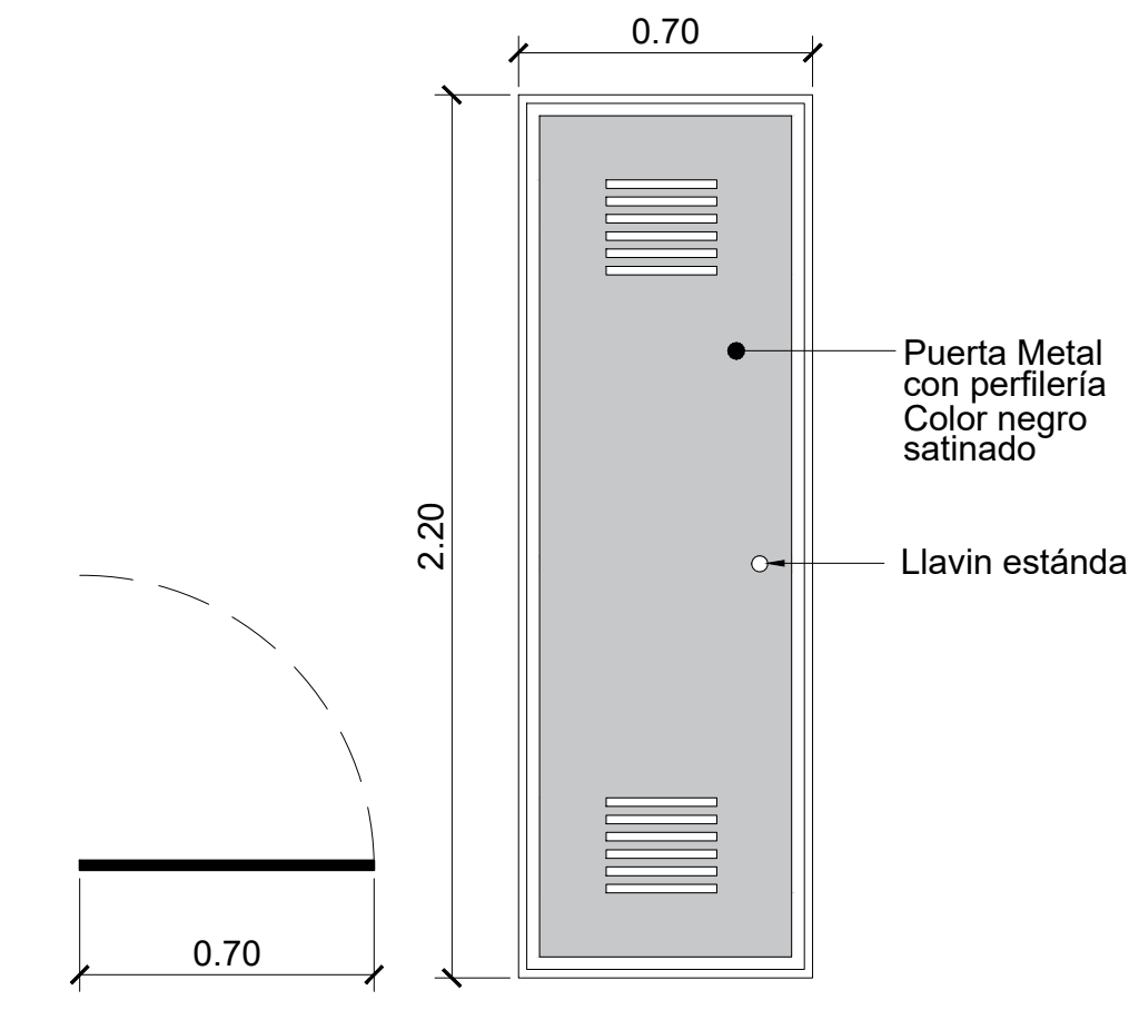
8 Puerta P07 ESCALA 1:20
