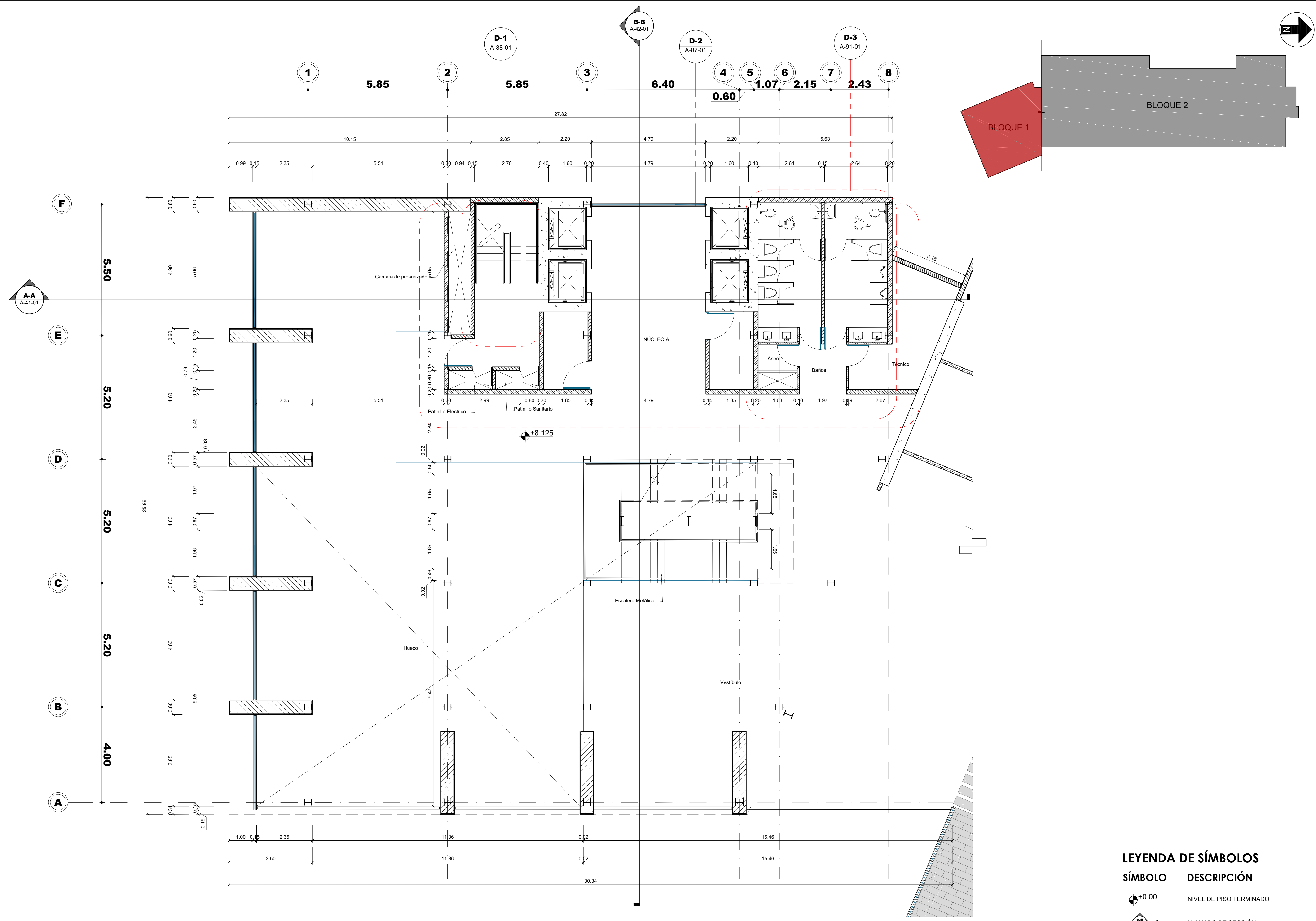
1 Planta Dimensionada - Bloque 1 - Nivel 3 Esc. 1:75
