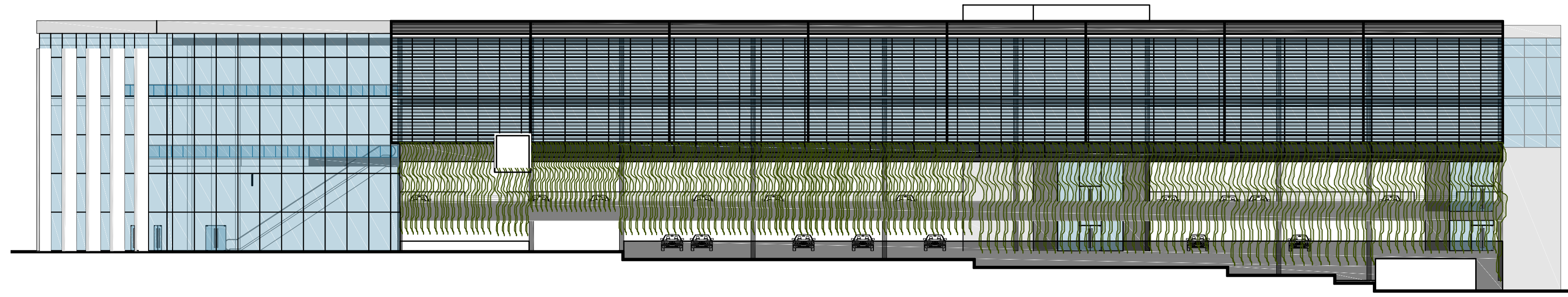
1 Elevación Bloque 2 Esc. 1:300
