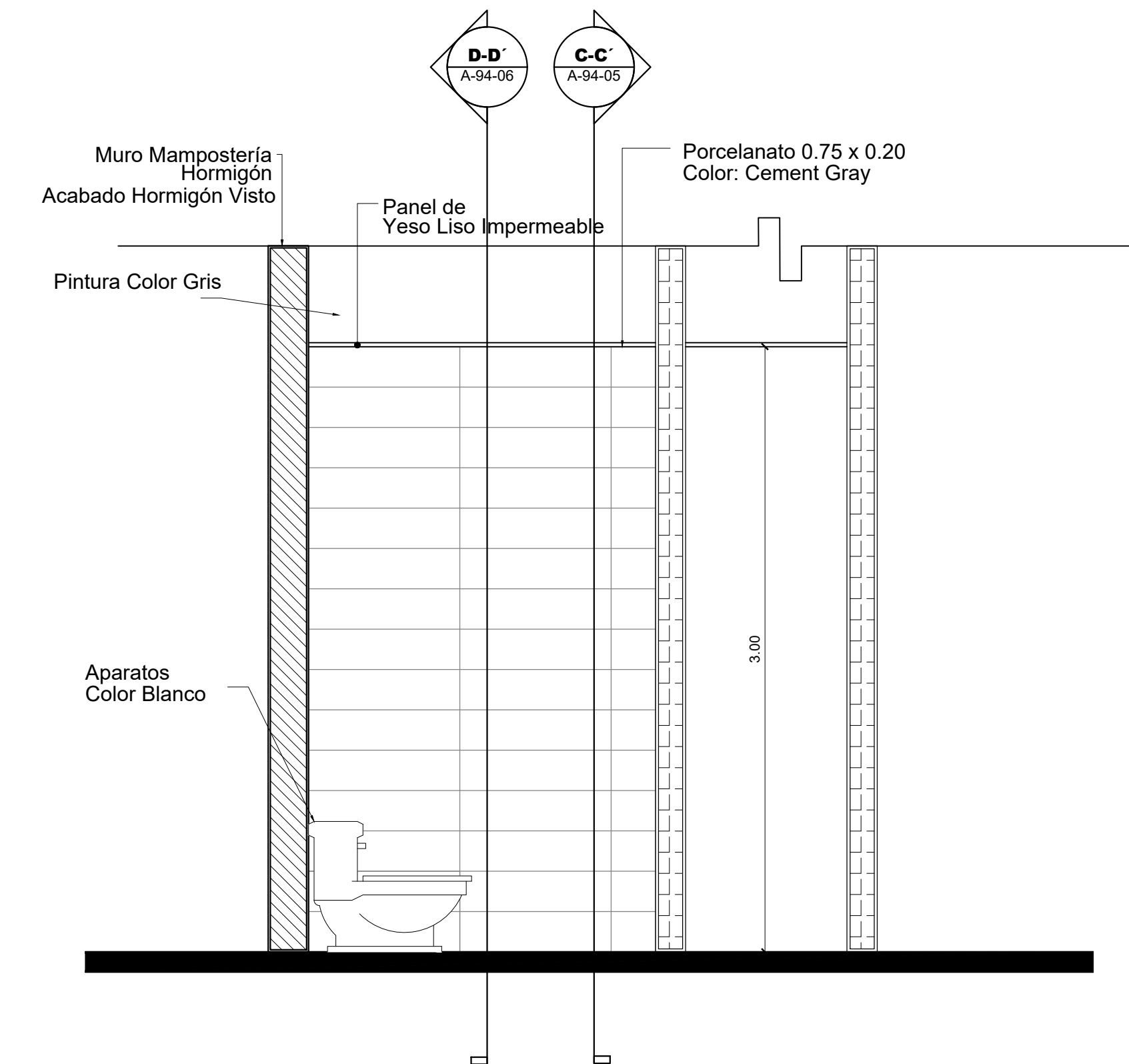
3 Sección A-A' Esc. 1: 25
