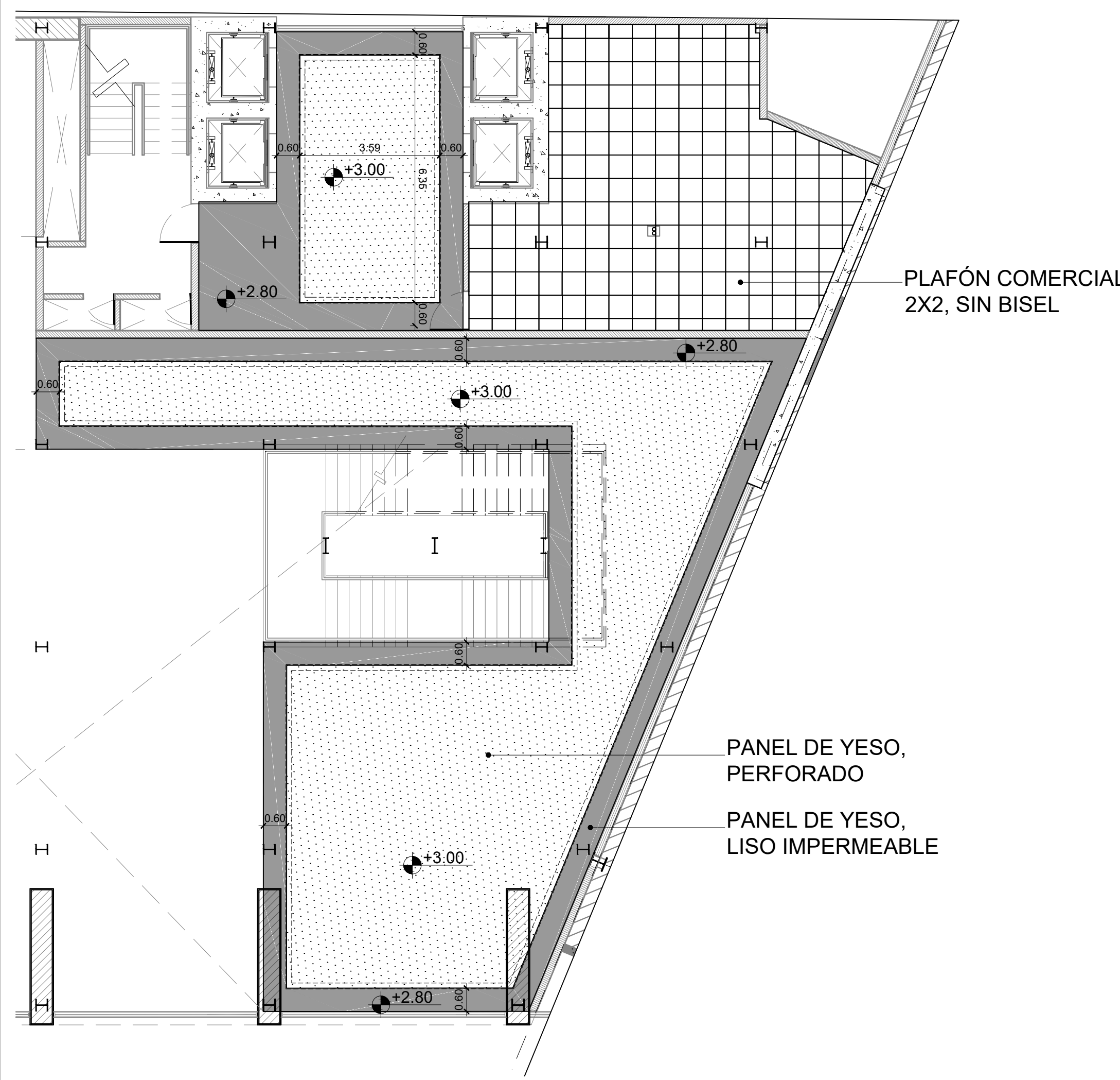
2 Detalle 1, Planta de Plafón, Nucleo A Esc. 1:100
