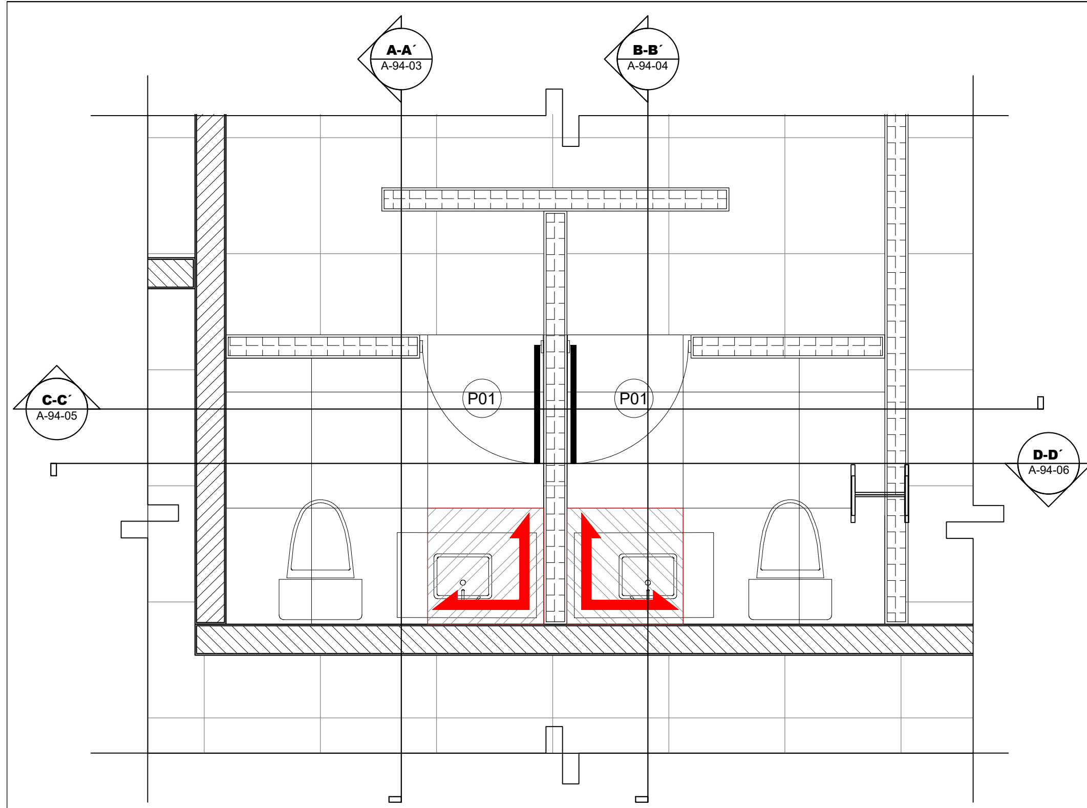
1 Planta Amueblada - Baños Esc. 1: 25
