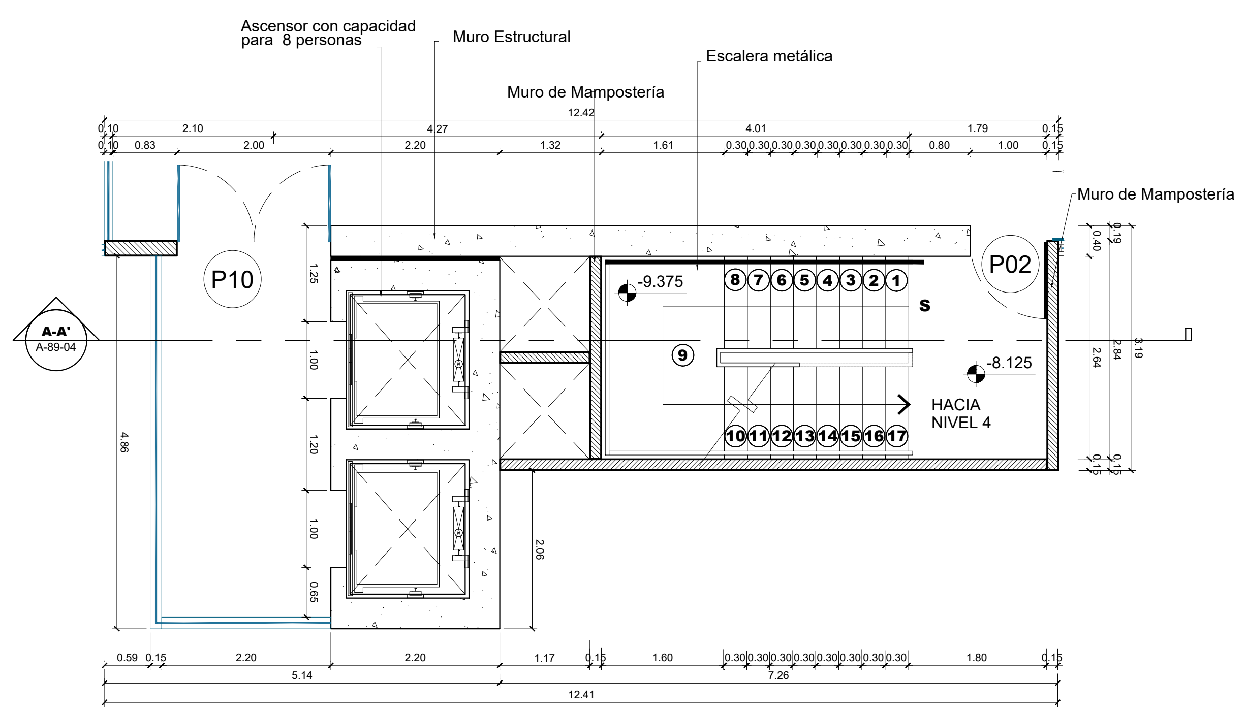
2 Planta Núcleo C - Nivel 3 a Nivel 4 Esc. 1:50
