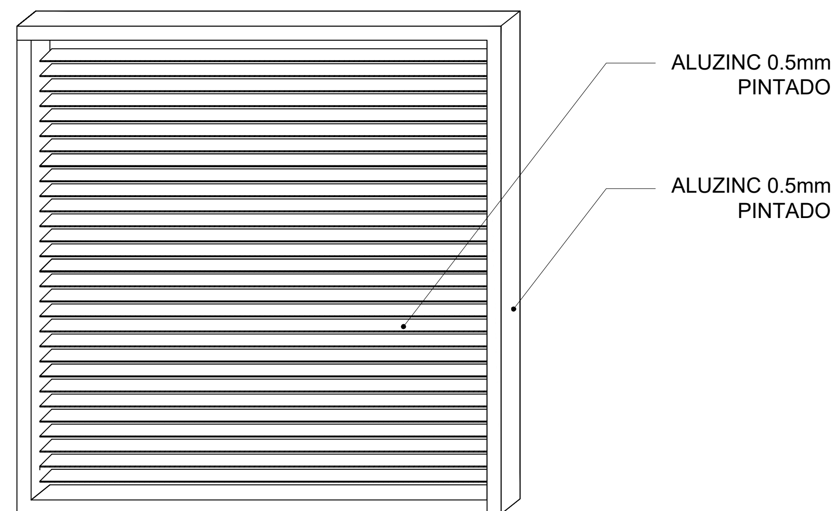
3 Detalle Típico Louvers Esc. 1:40
