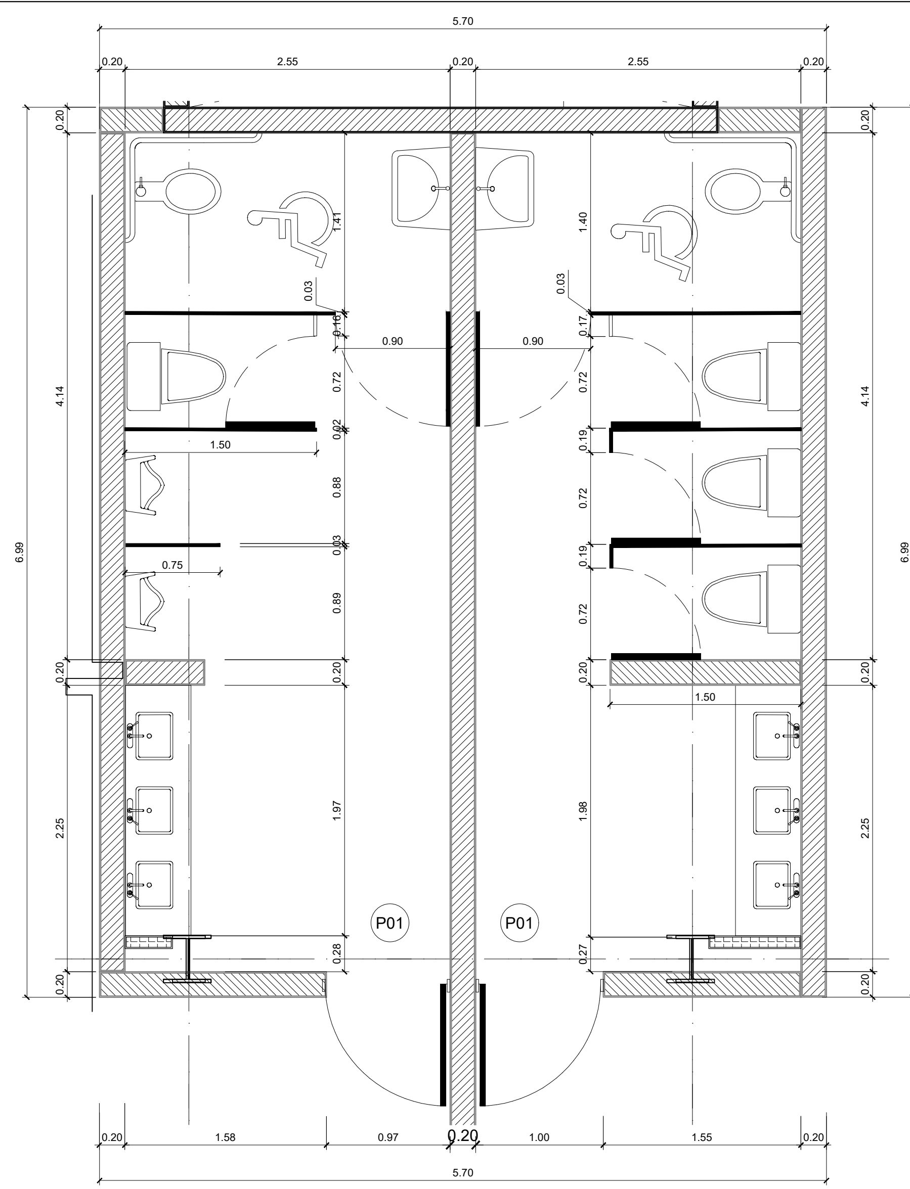
3 Planta Dimensionada - Baños Esc. 1: 30
