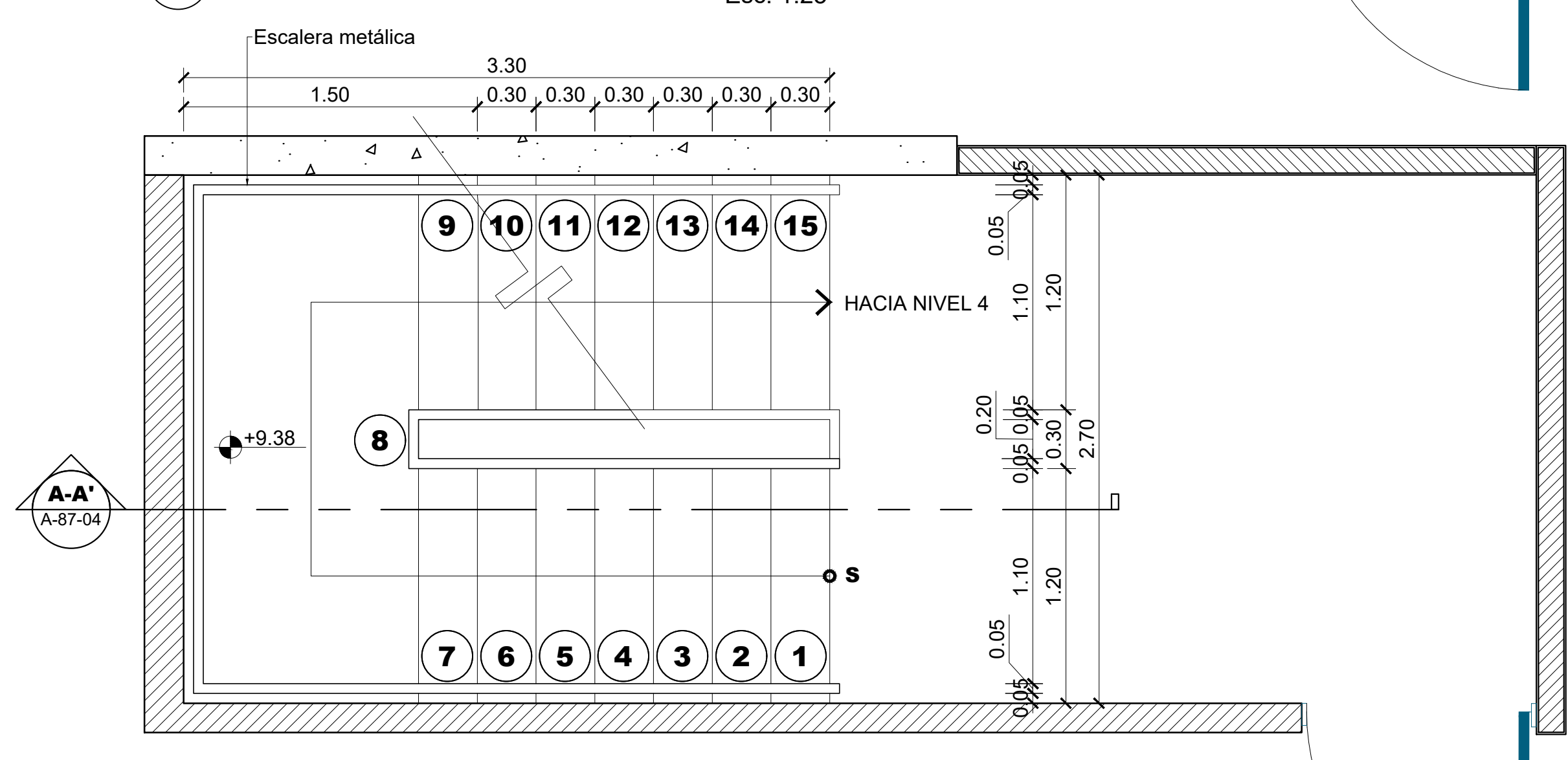
3 Planta Escalera A - Núcleo A - N3 a N4 Esc. 1:25
