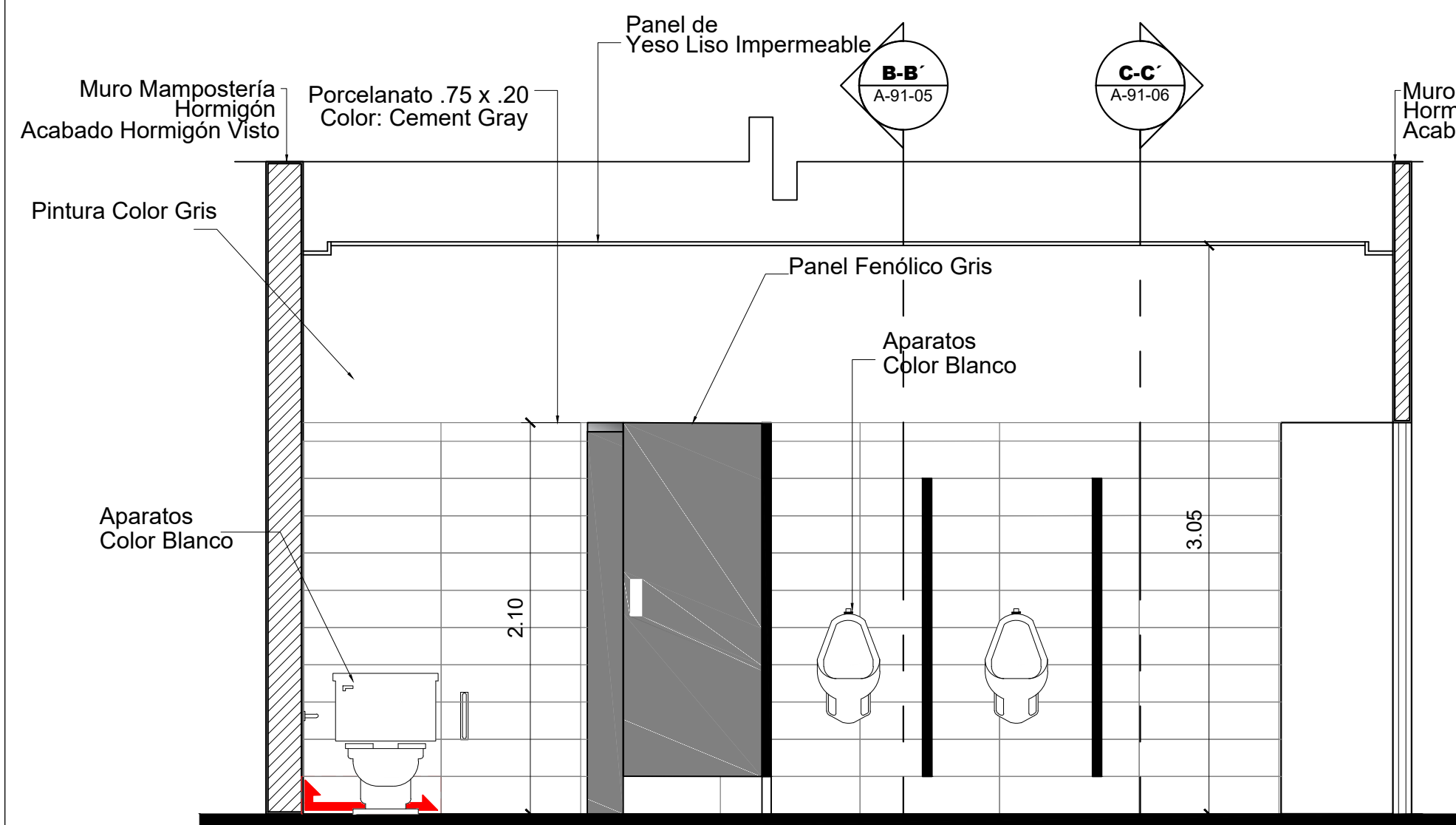
4 Sección A-A' Esc. 1: 30
