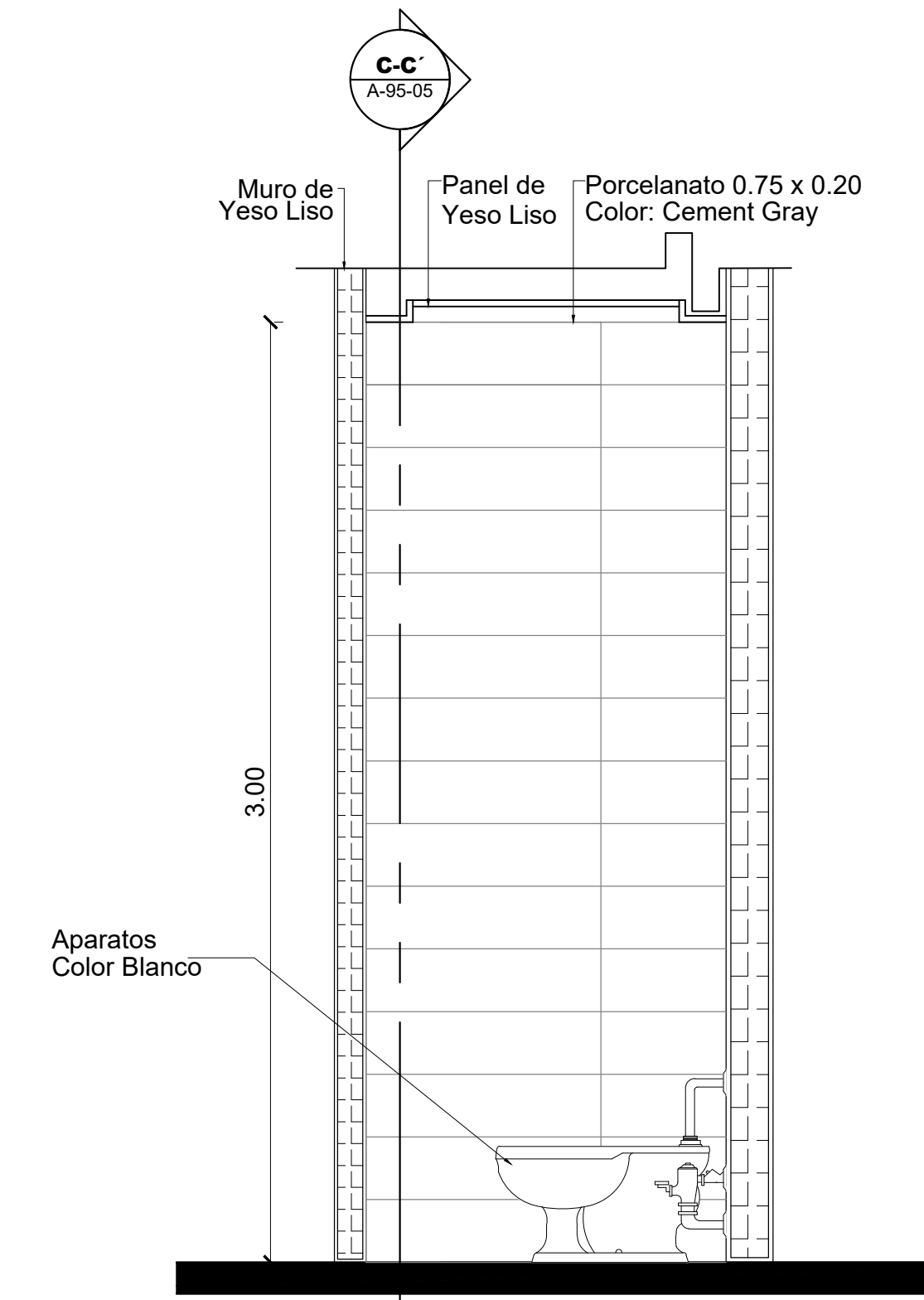
3 Sección A-A' Esc. 1: 20
