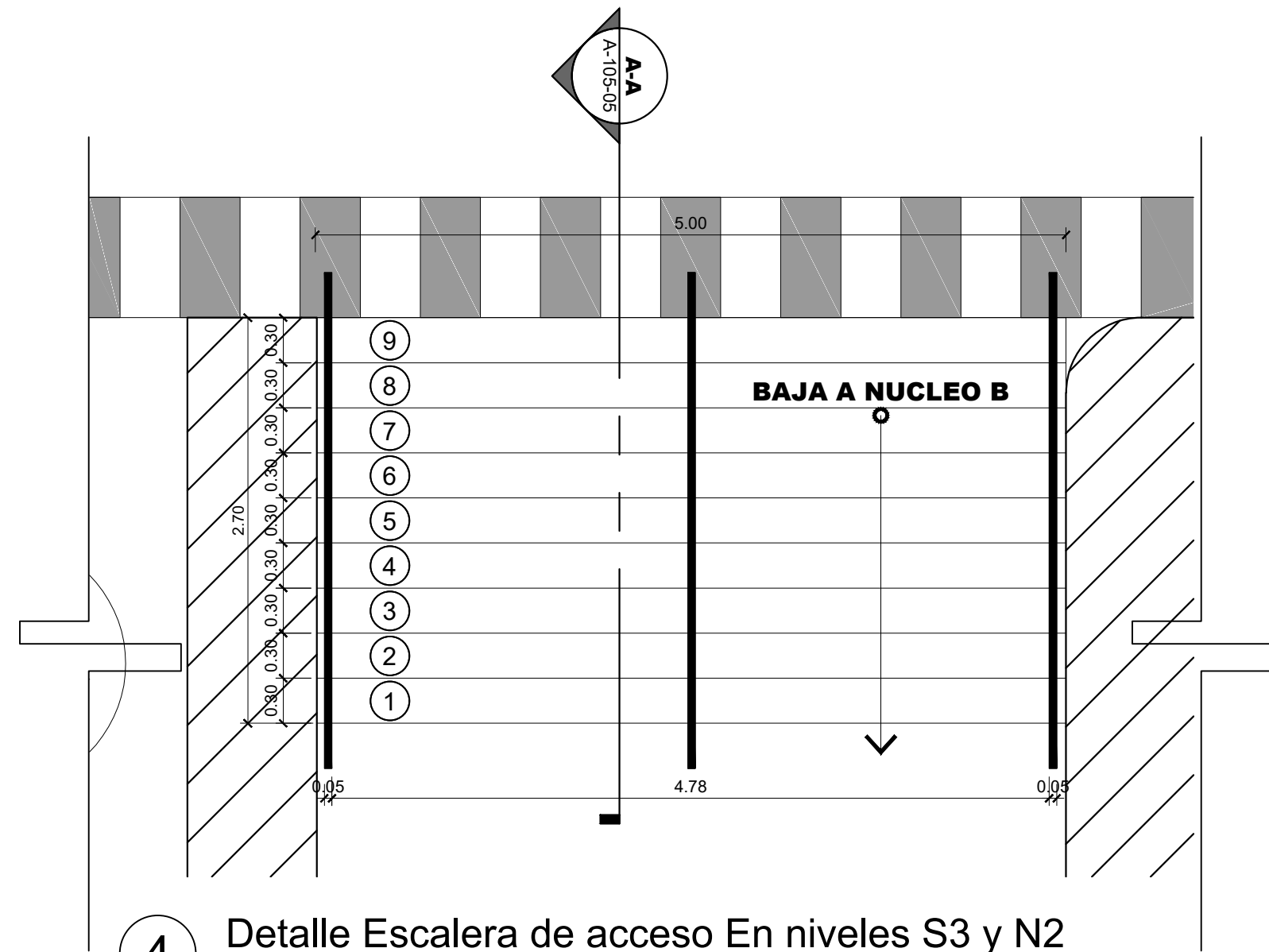
4 Detalle Escalera de acceso En niveles S3 y N2 Esc. 1:40
