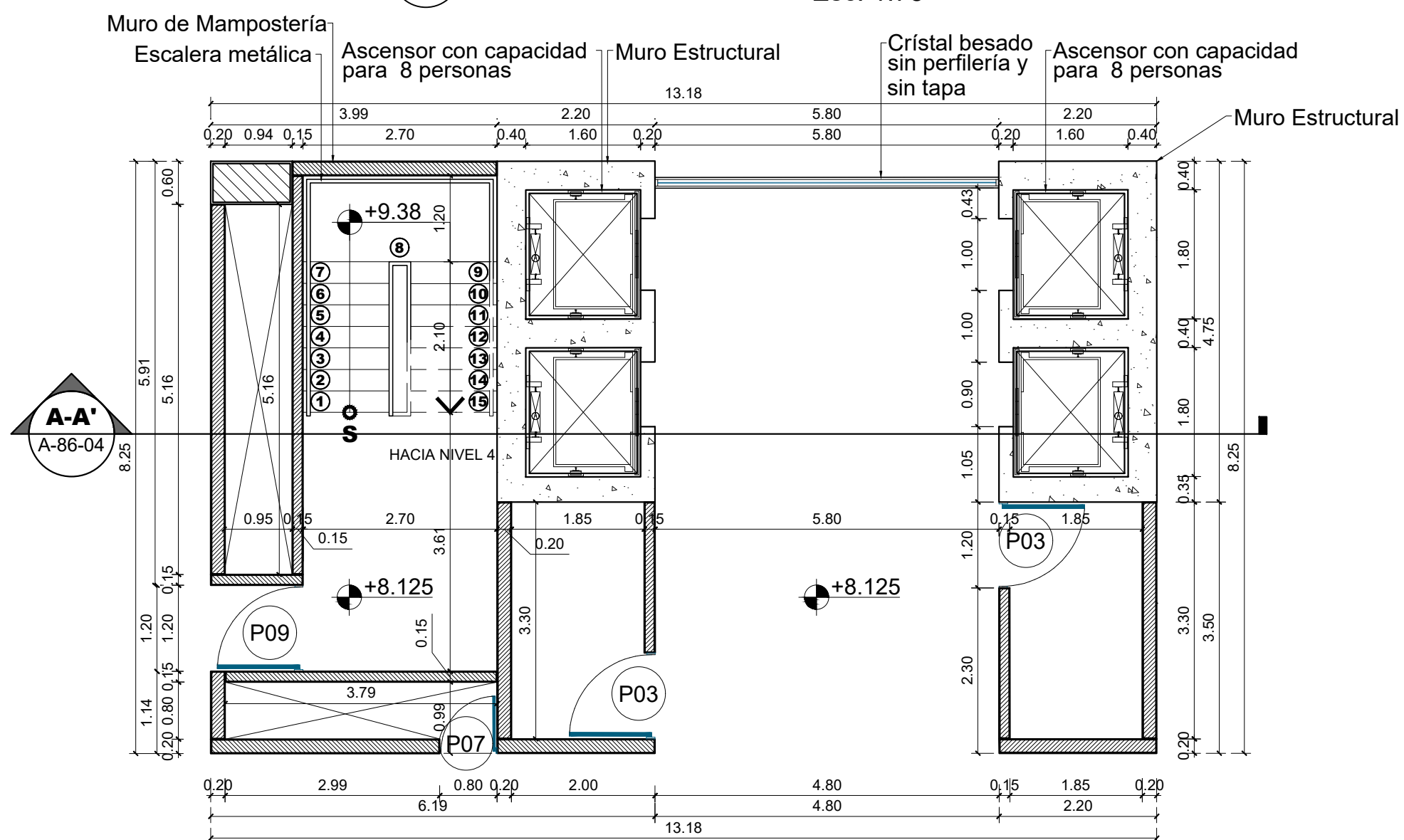
3 Planta Núcleo A - N3 a N4 Esc. 1:75
