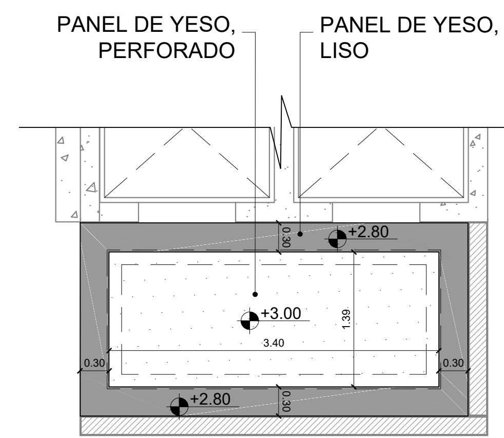
4 Detalle 3, Planta de Plafón, Nucleo C Esc. 1:40
