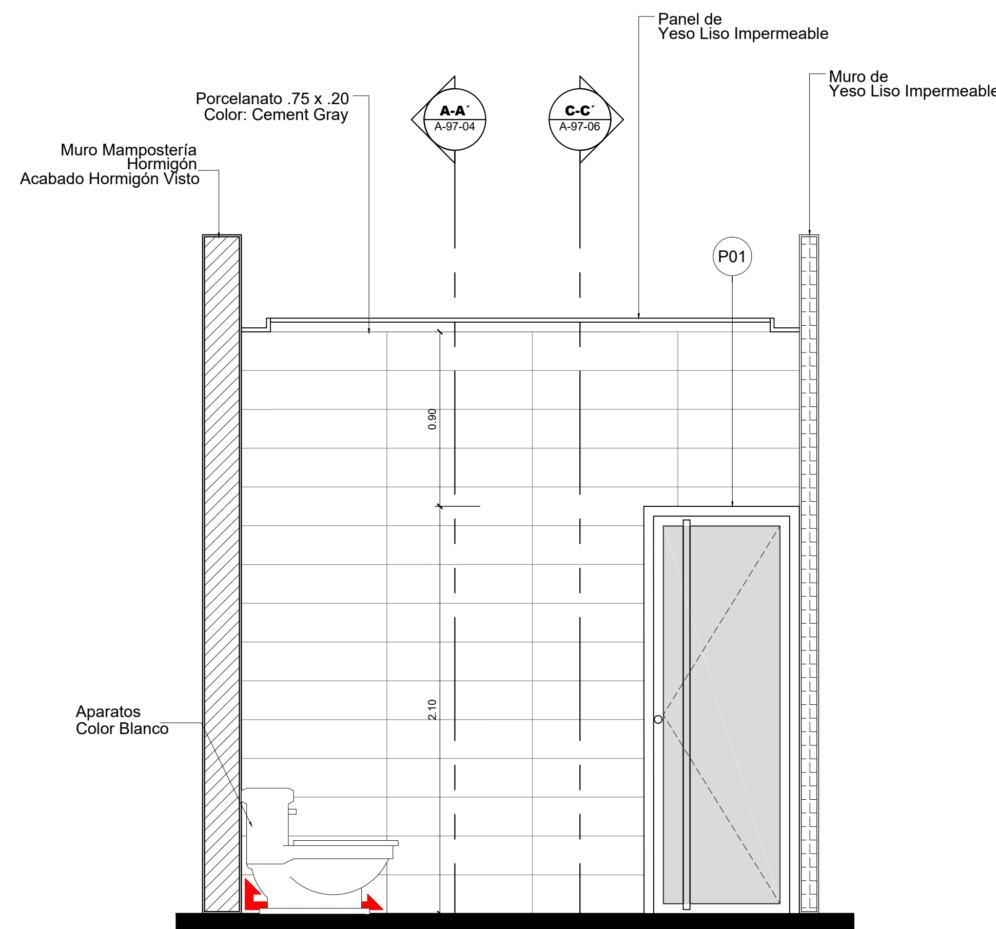
5 Sección B-B' Esc. 1: 20
