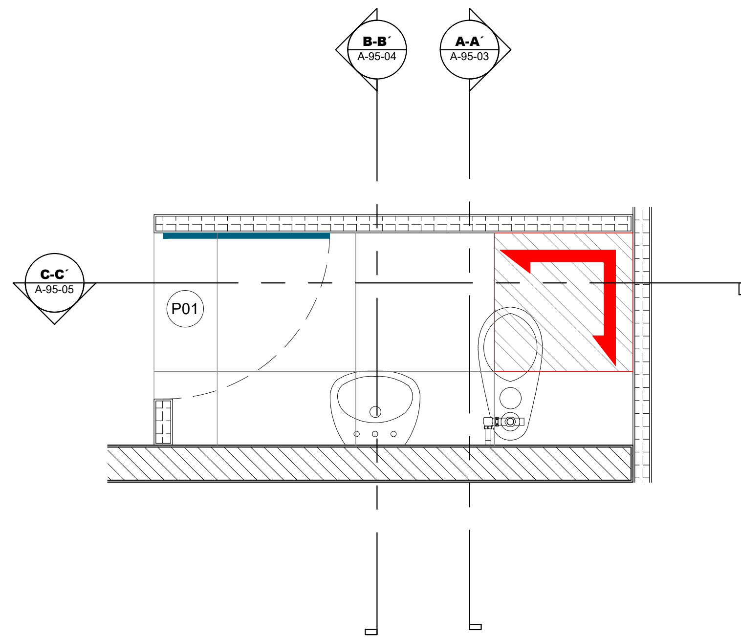
1 Planta Amueblada - Baños Esc. 1: 20
