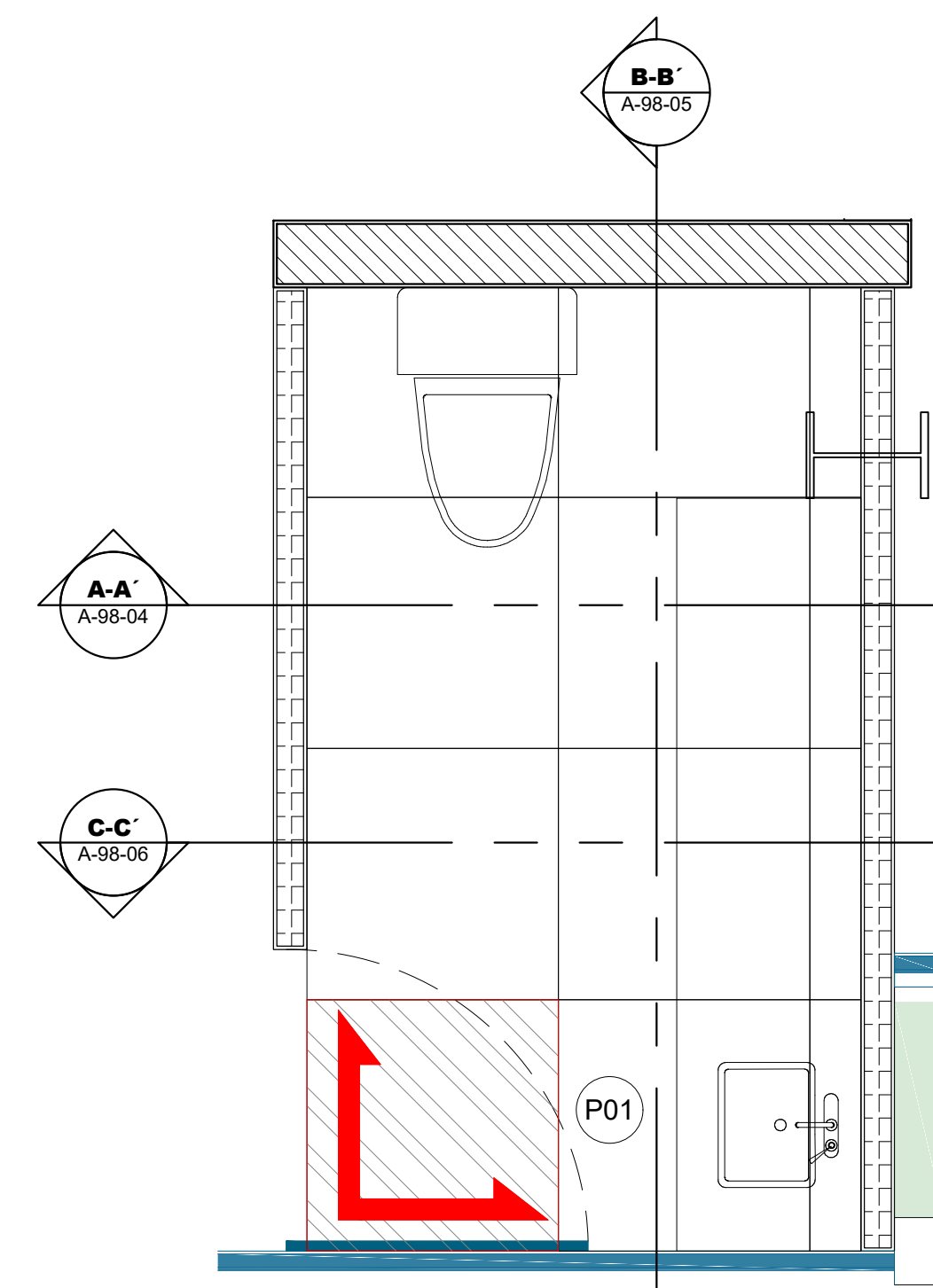
2 Planta Amueblada - Baños Esc. 1: 20
