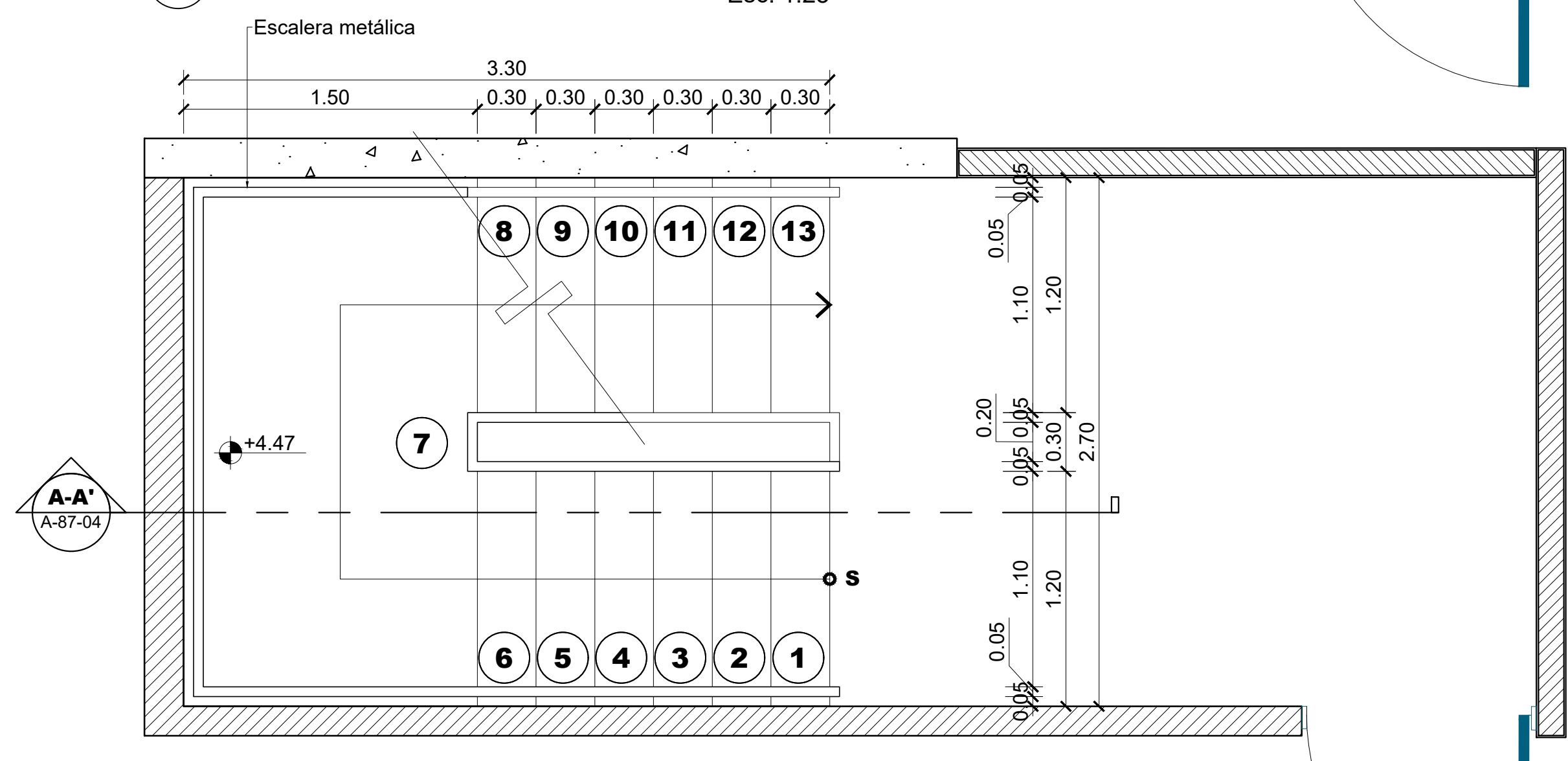
2 Planta Escalera A - Núcleo A - N2 a N3 Esc. 1:25
