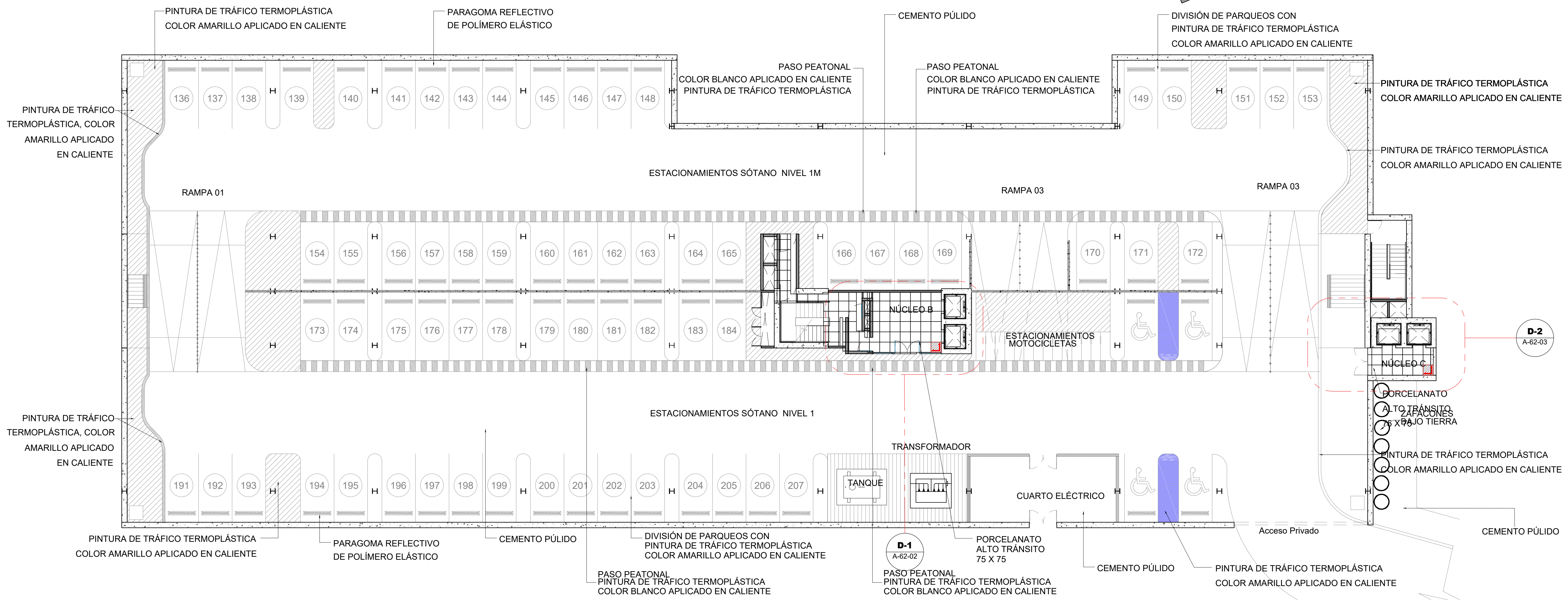
1 Planta Pisos - Sótano 1 Esc. 1:150
