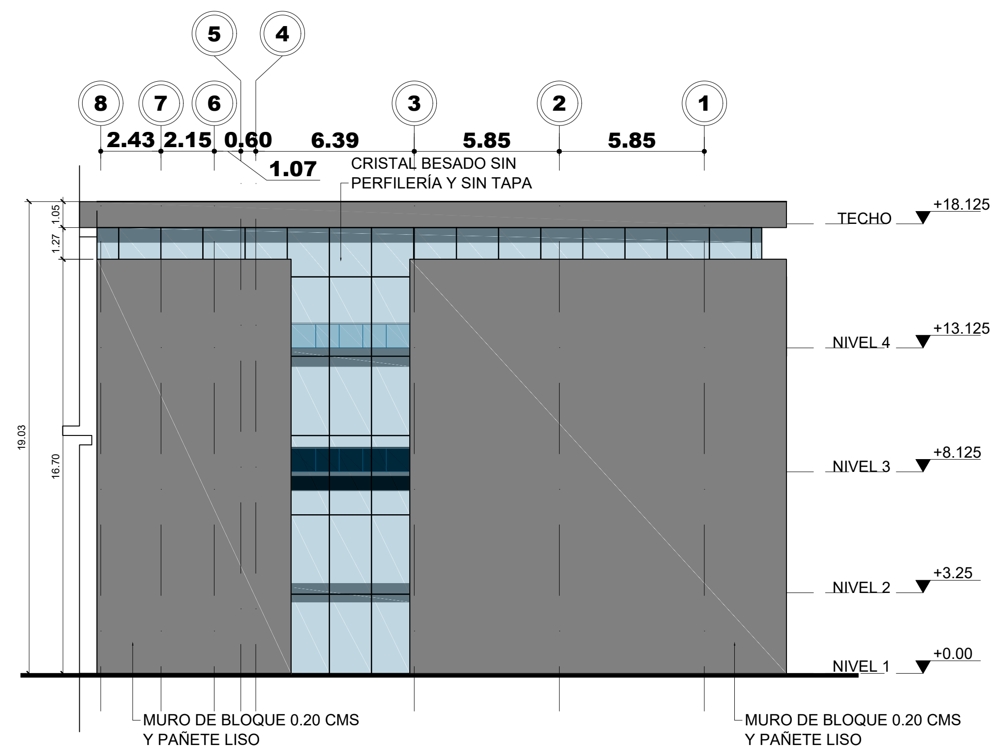
3 Elevación Lateral Izquierda bloque 1 Esc. 1:150
