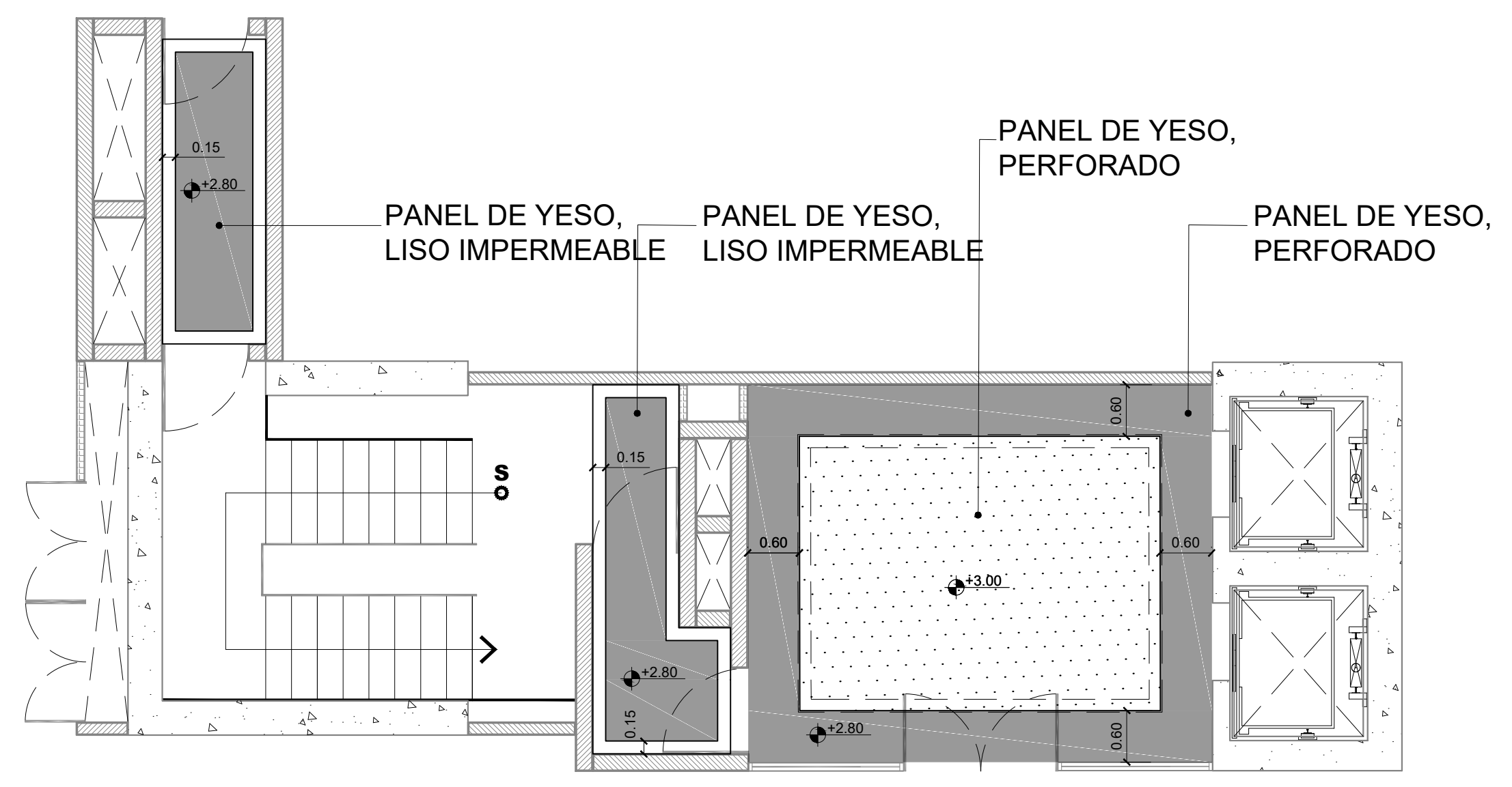
2 Detalle 1, Planta de Plafón, Nucleo B Esc. 1:60
