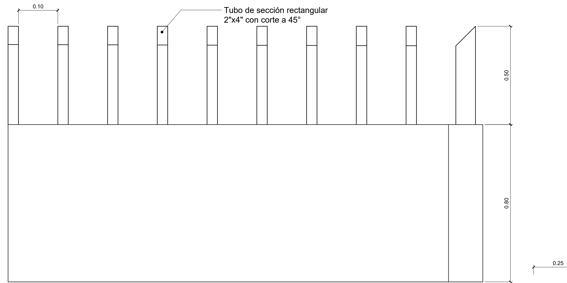
1 Detalle de Muro Perimetral Esc. 1:10
