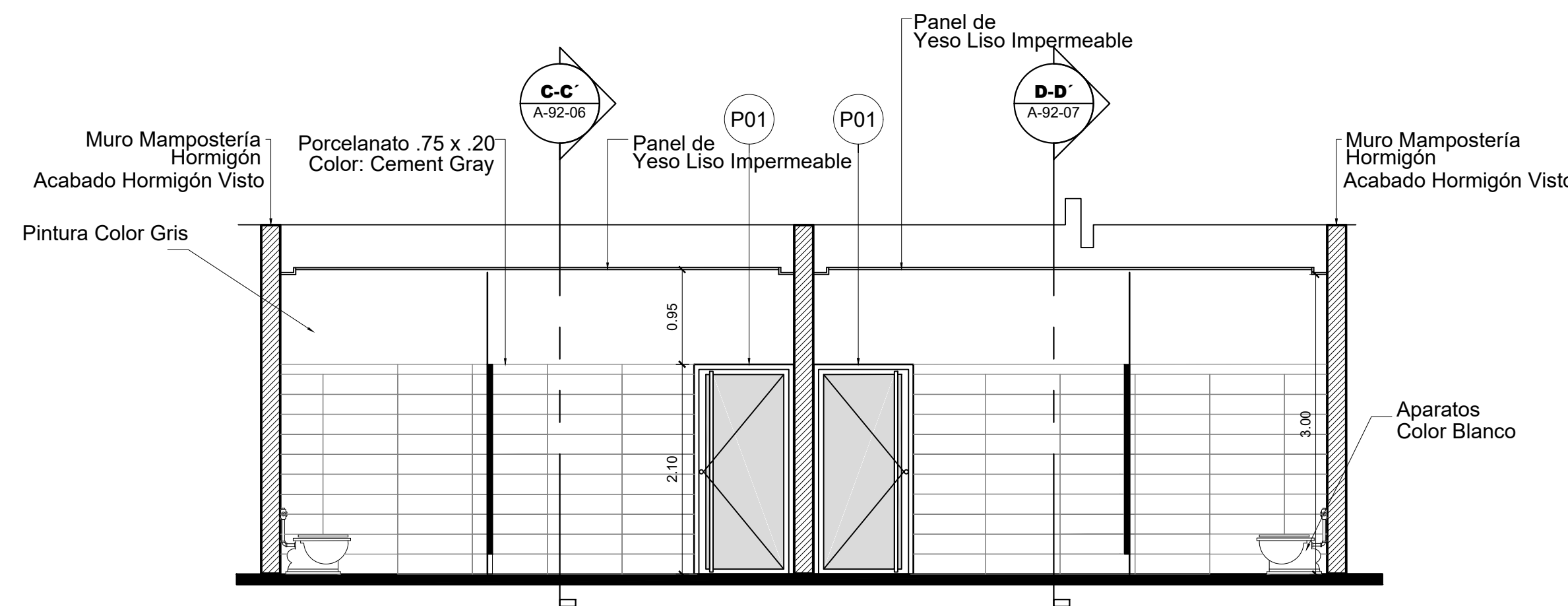
4 Sección A-A' Esc. 1: 50
