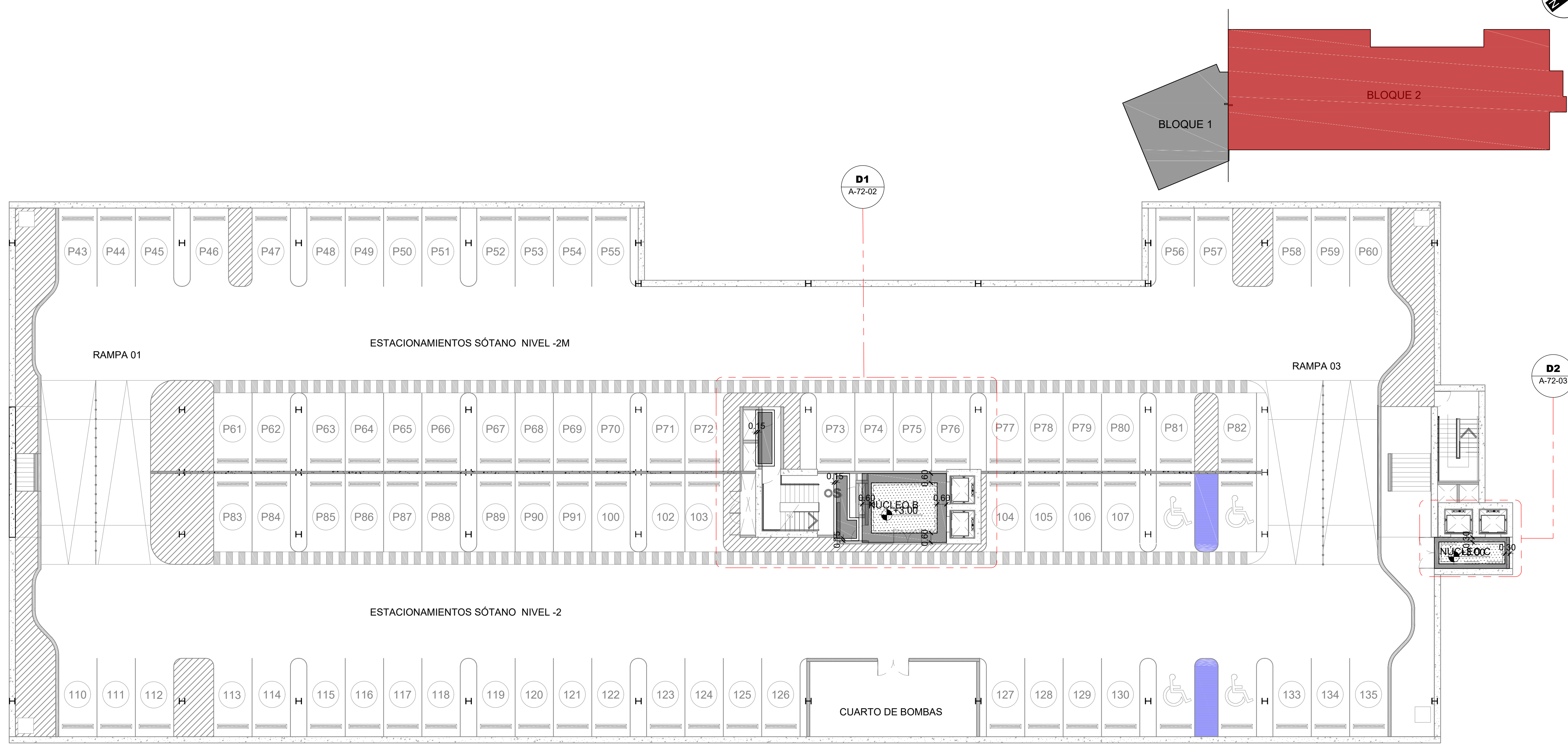
1 Planta Plafones - Sótano 2 Esc. 1:150
