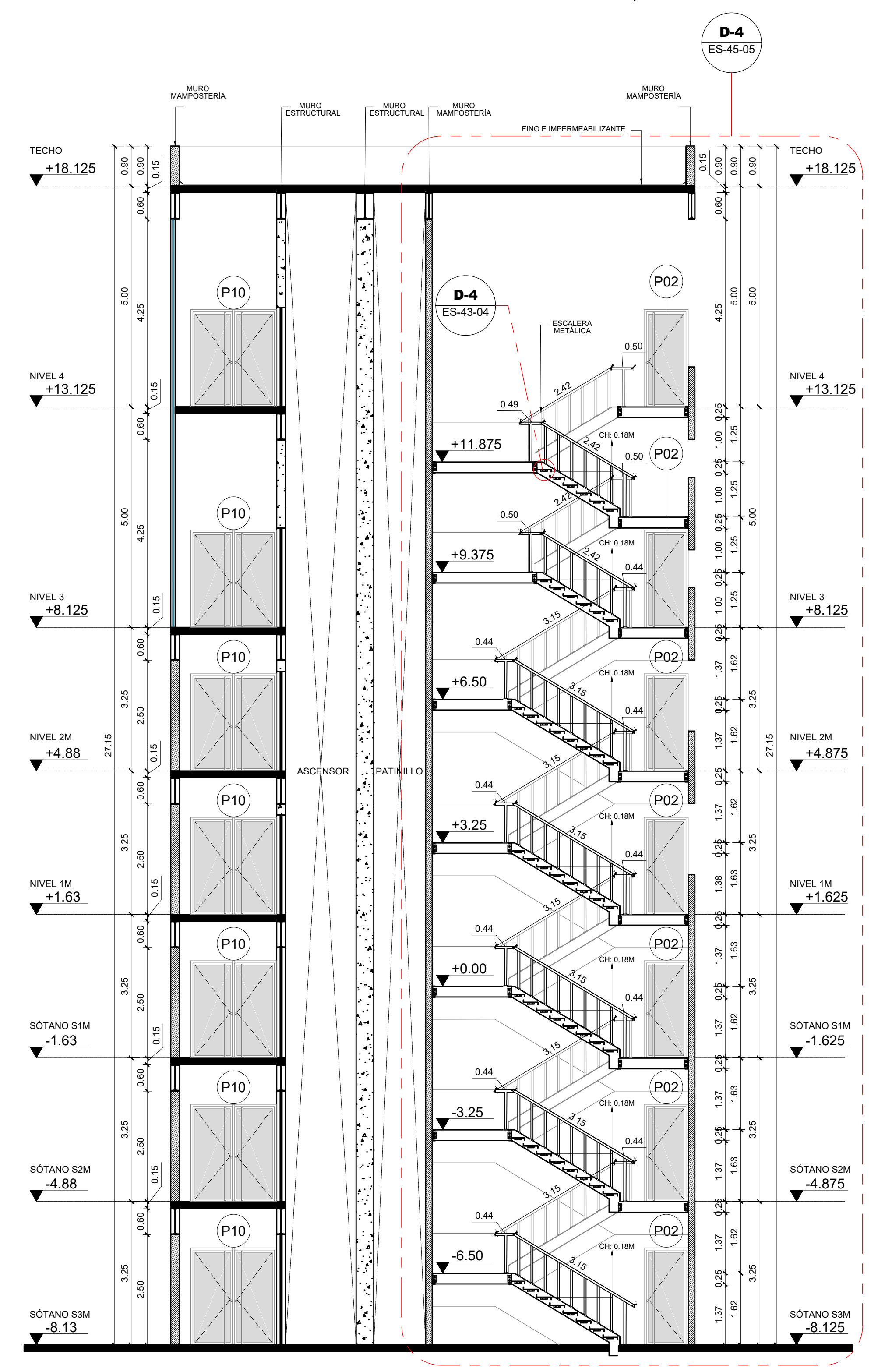
3 Sección A-A' Núcleo C - Sótano 3M a Nivel 4 Esc. 1:75
