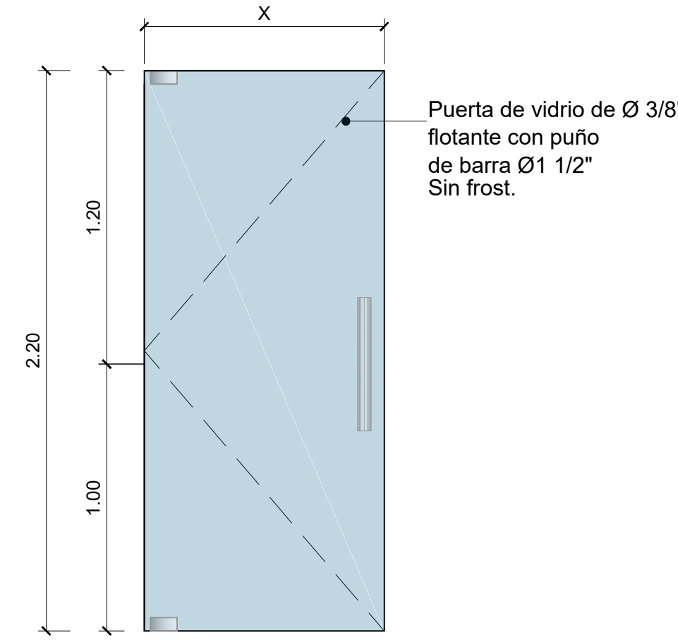
2 Puerta P02 ESCALA 1:20
