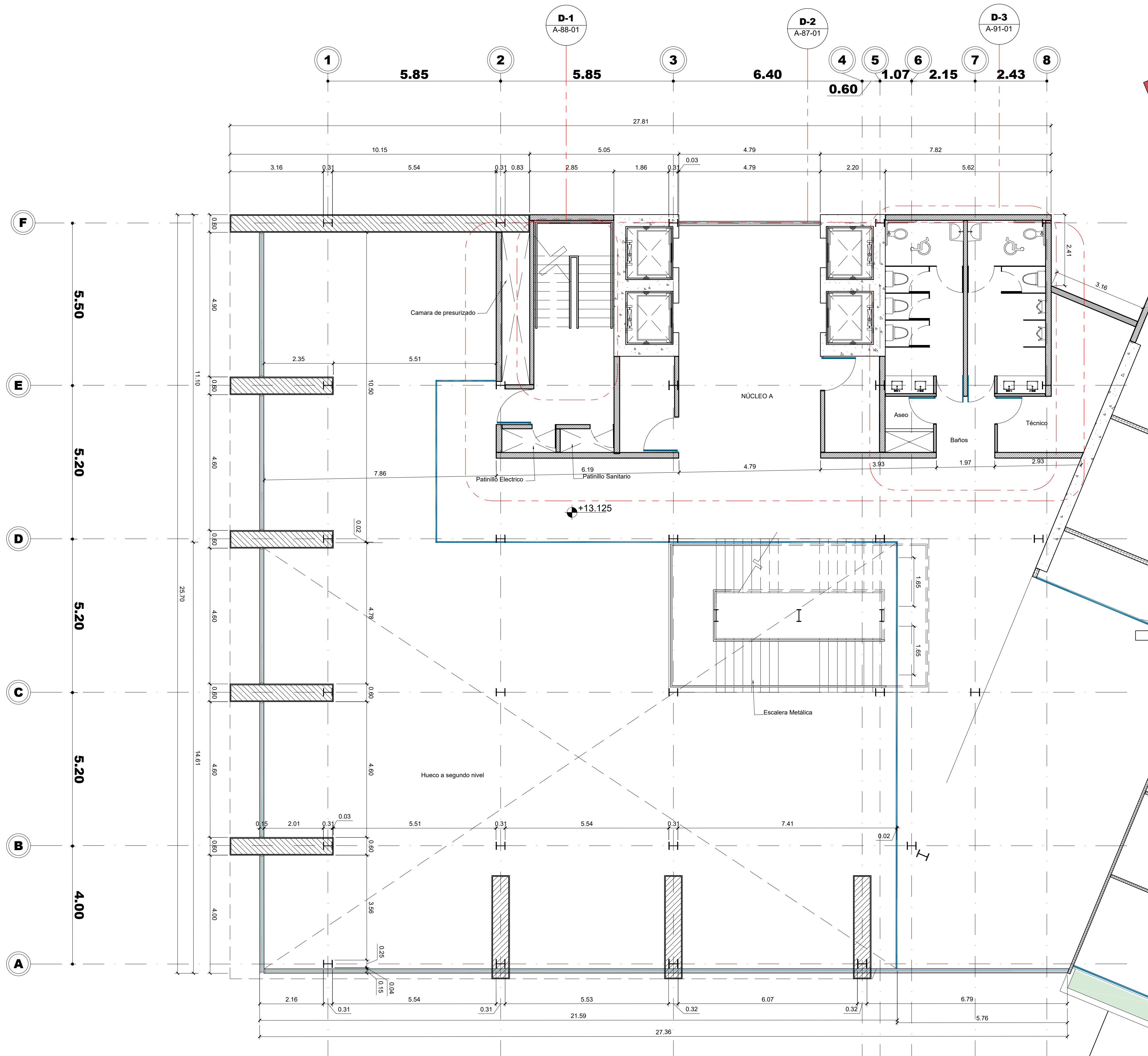
1 Planta Dimensionada - Bloque 1 - Nivel 4 Esc. 1:75
