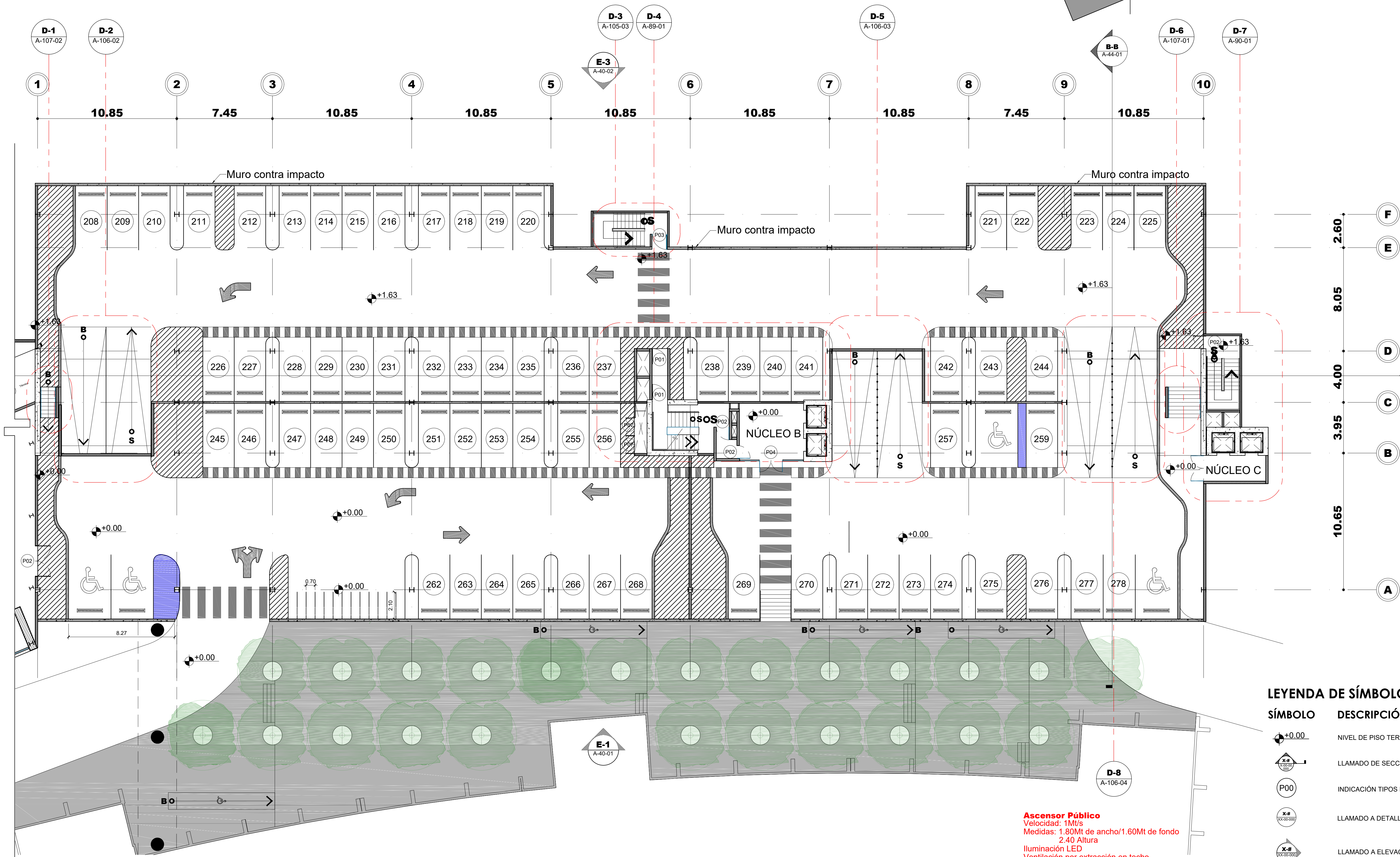
1 Planta Amueblada - Nivel 1 - Bloque 2 Esc. 1:150
