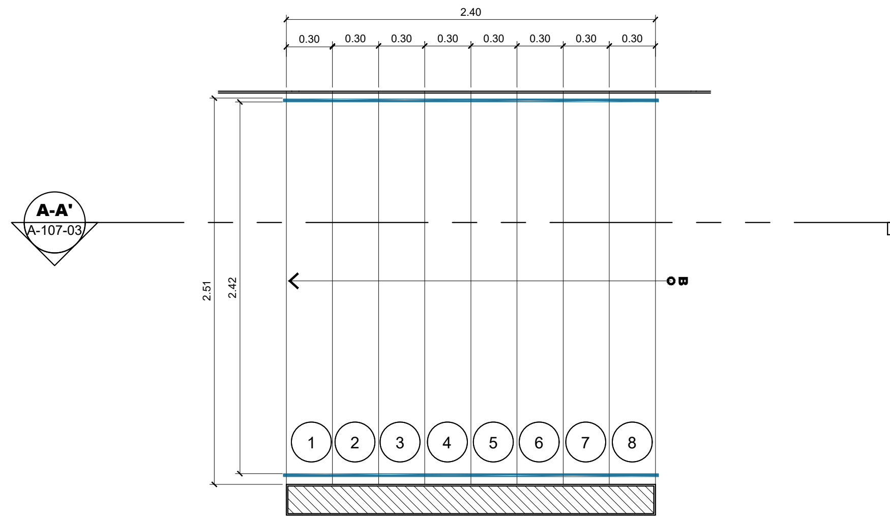
1 Detalle Escalera Lateral derecha S3-N2M Esc. 1:25
