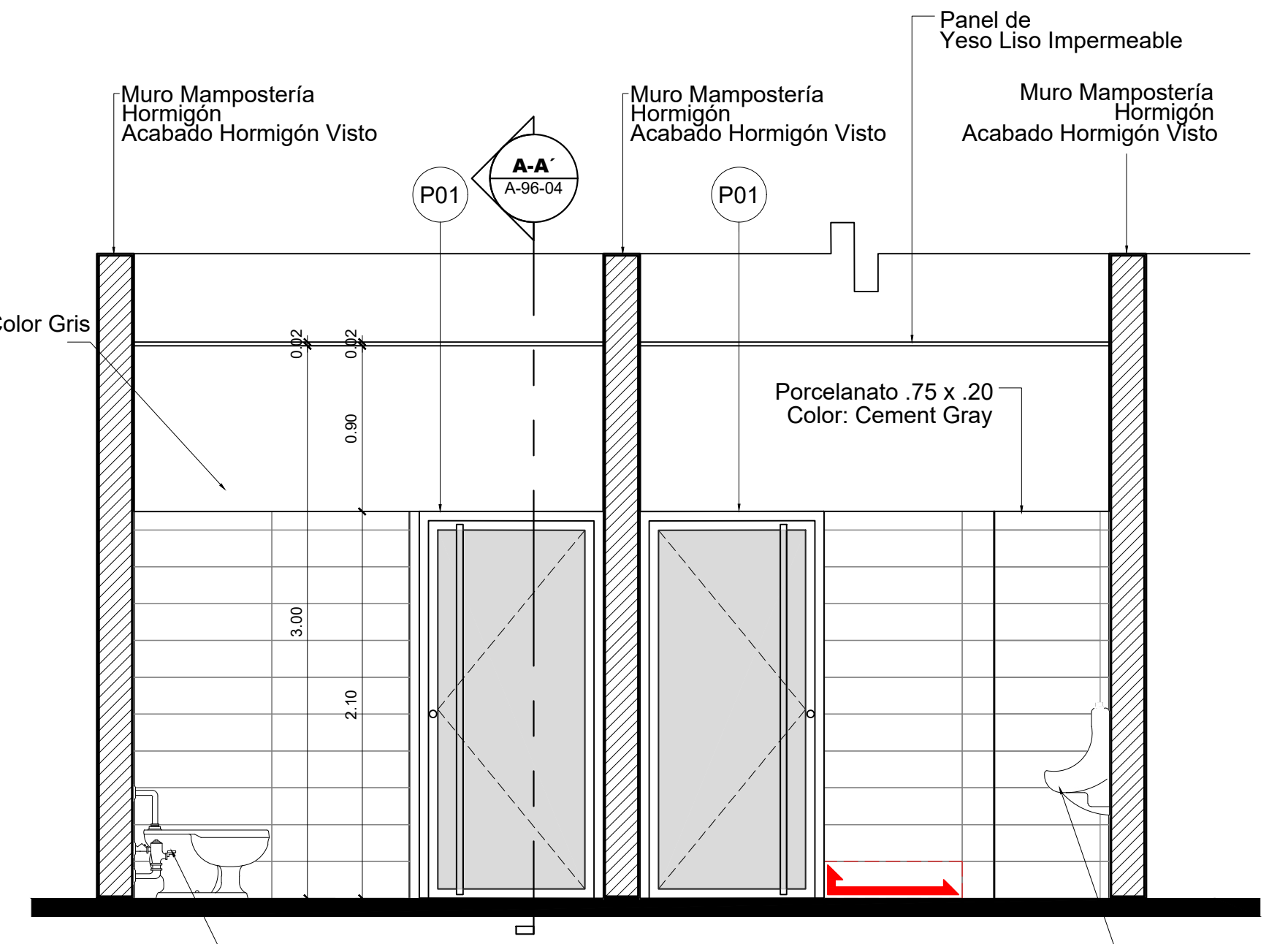
6 Sección C-C' Esc. 1: 30
