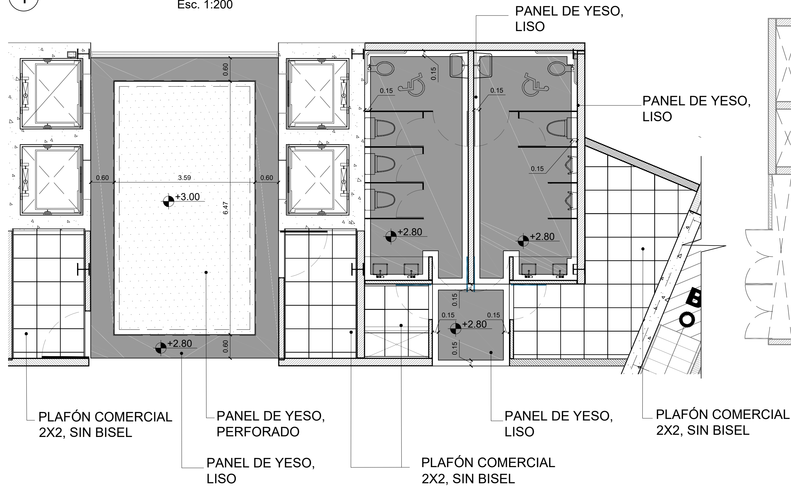
2 Detalle 1, Planta de Plafón, Nucleo Bloque A Esc. 1:60
