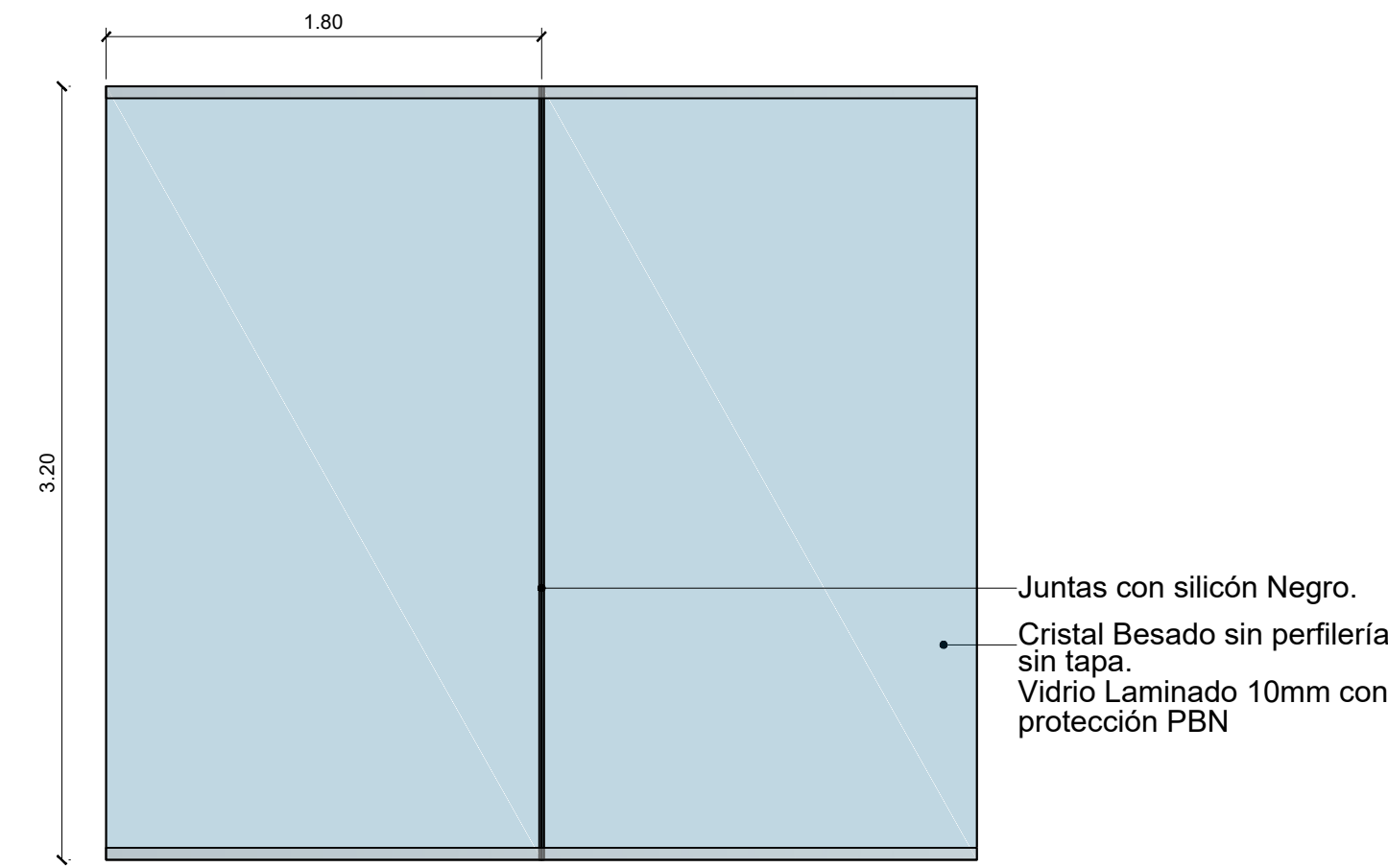
11 Cristal en Fachada ESCALA 1:30
