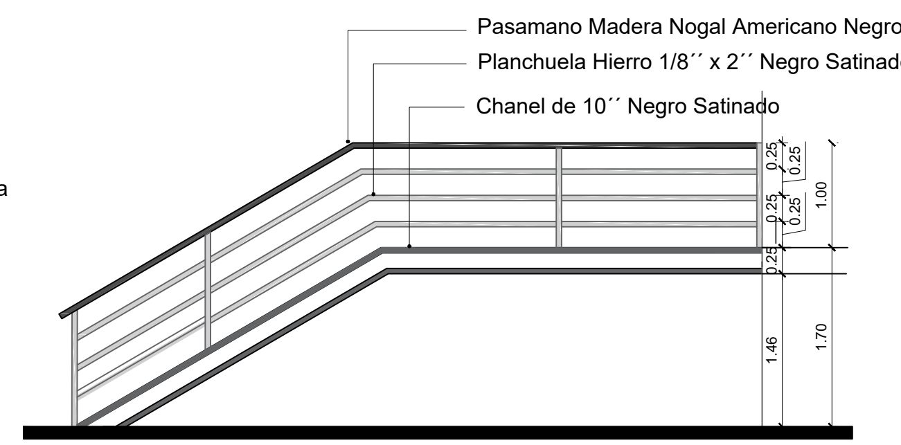
10 Baranda Auditorio ESCALA 1:50
