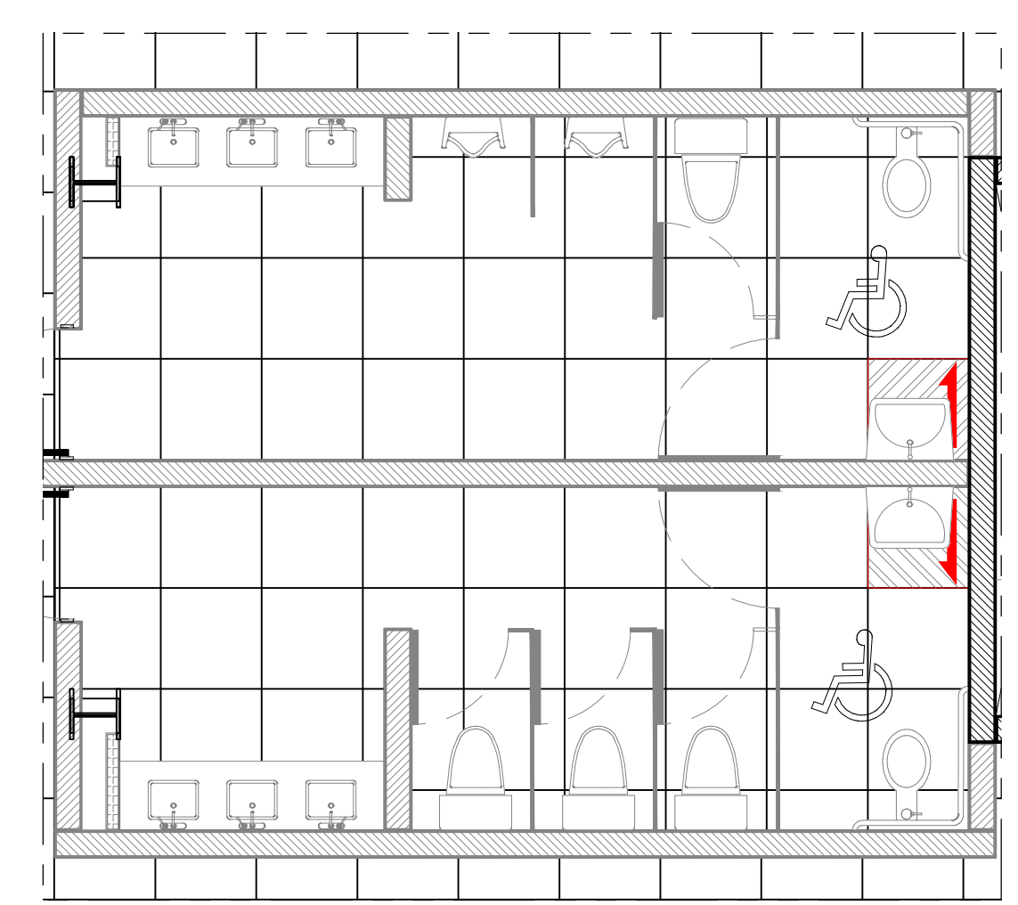
2 Detalle A Esc. 1:50
