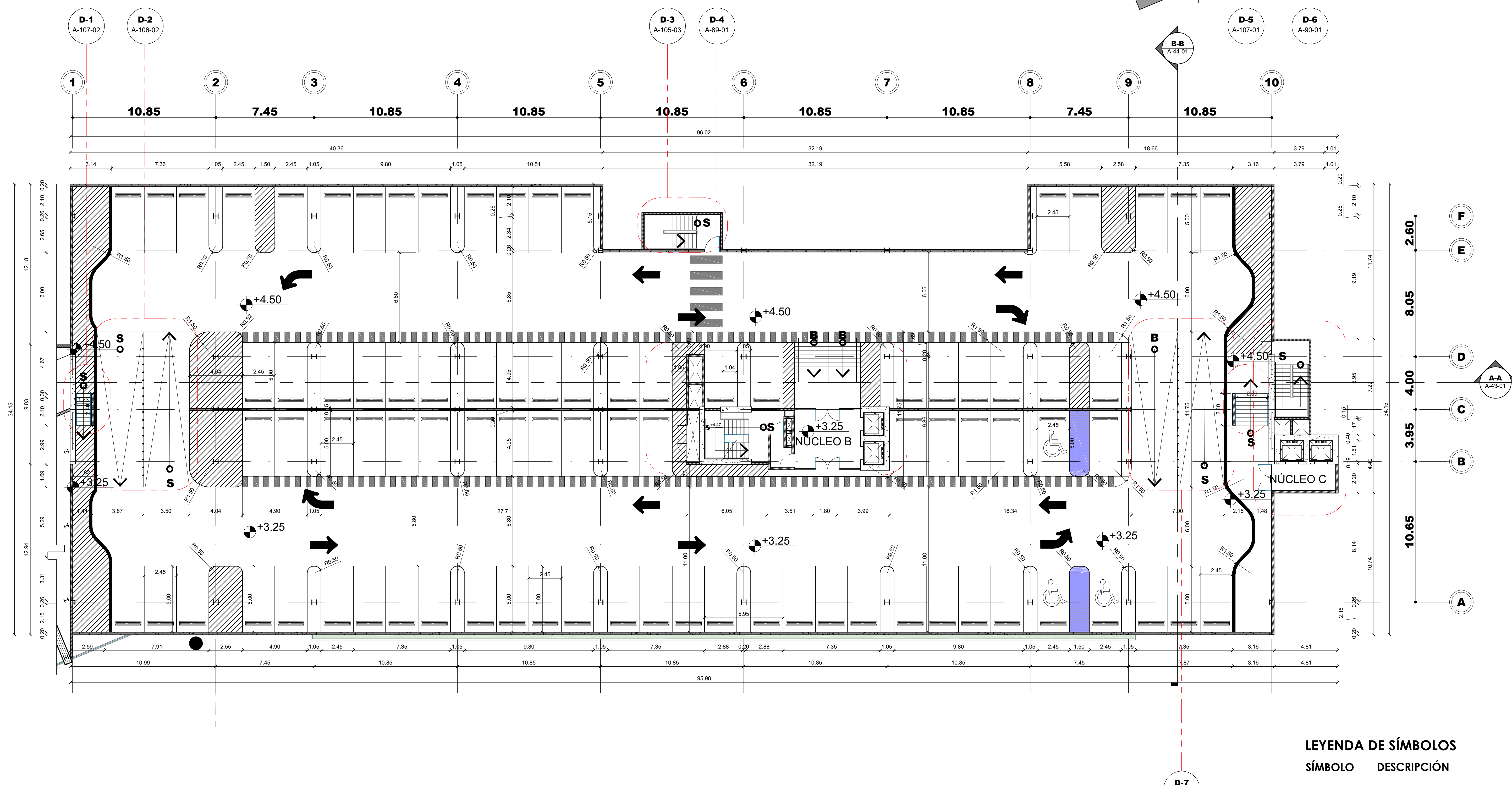
1 Planta Dimensionada Nivel 2 - BLOQUE 2 Esc. 1:150
