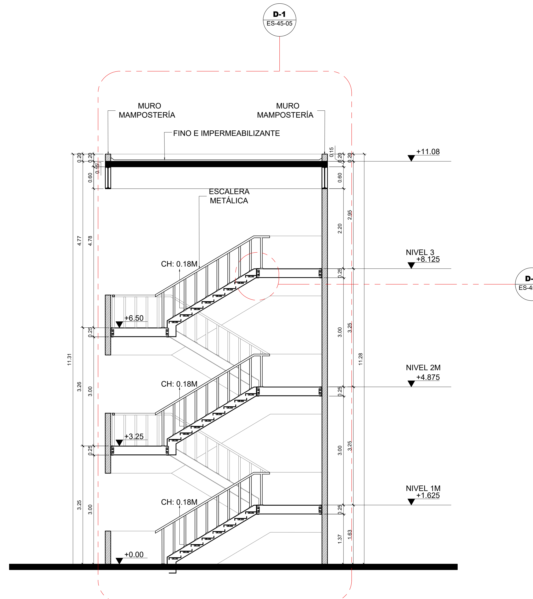
2 Sección A-A' Escalera Sala de Audiencia Esc. 1:50
