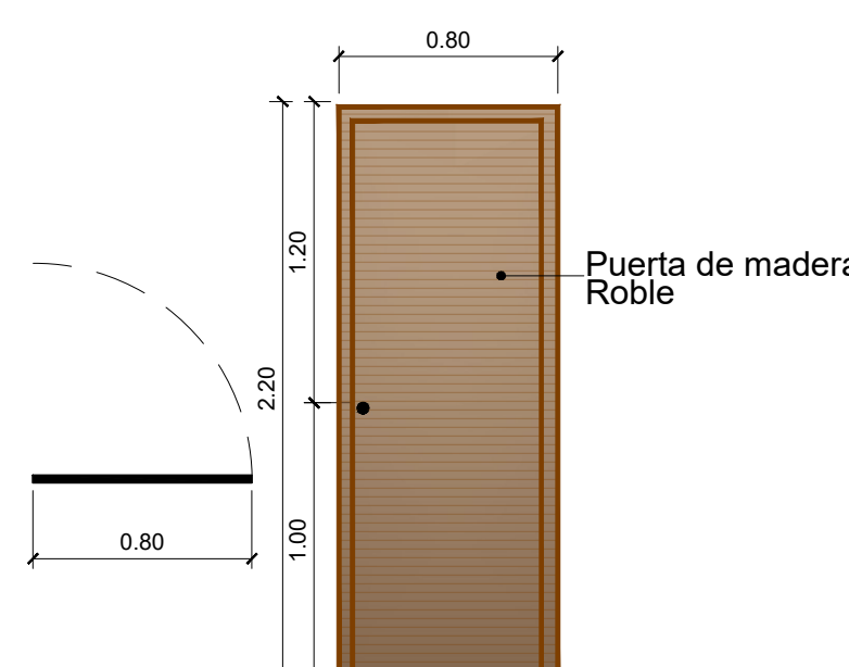
9 Puerta P08 ESCALA 1:30
