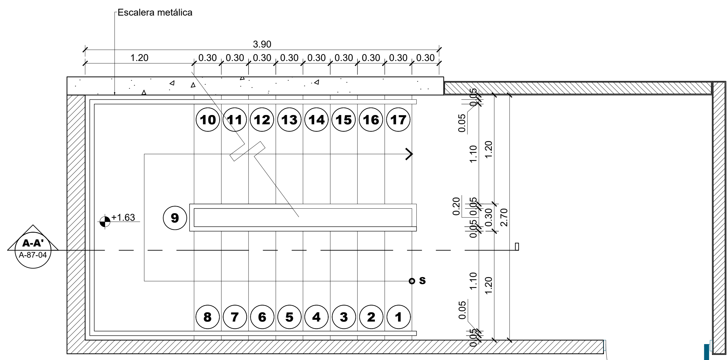
1 Planta Escalera A - Núcleo A - N1 a N2 Esc. 1:25
