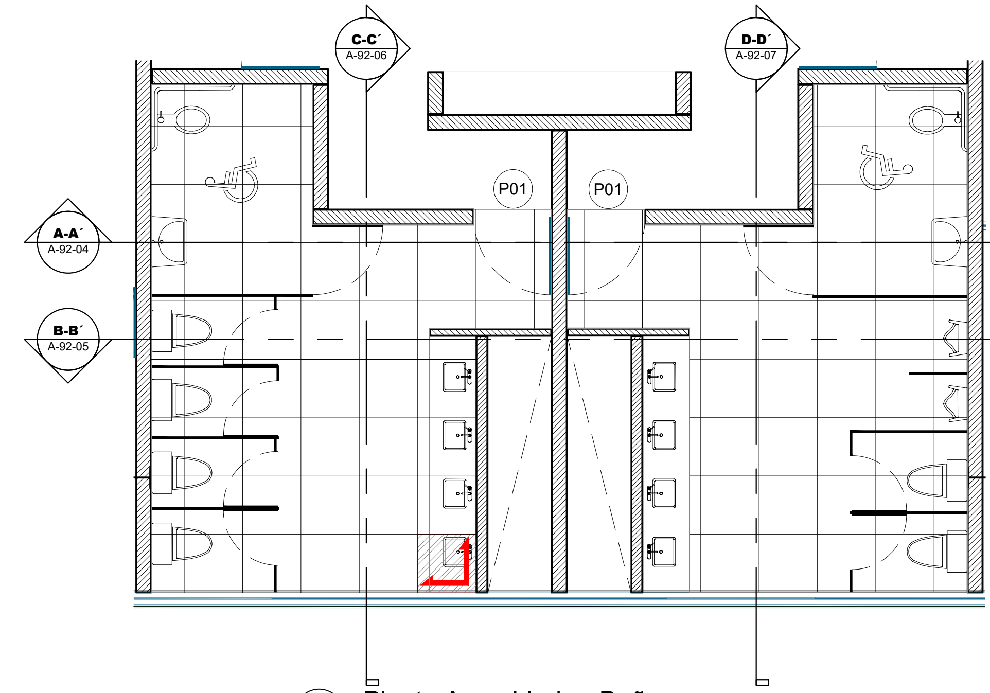
3 Planta Amueblada - Baños Esc. 1: 50
