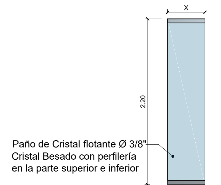
4 Detalle de Paneles Cristal Fijo ESCALA 1:30
