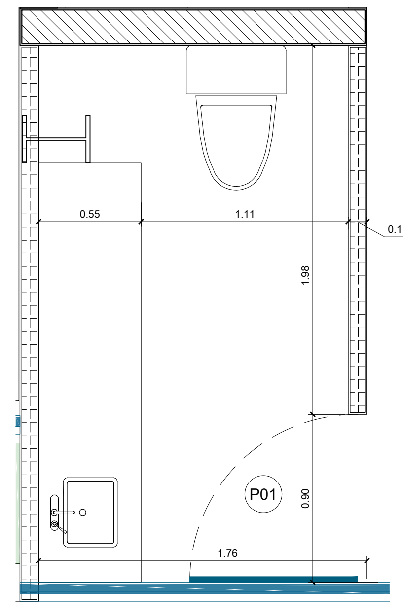
3 Planta Dimensionada - Baños Esc. 1: 20
