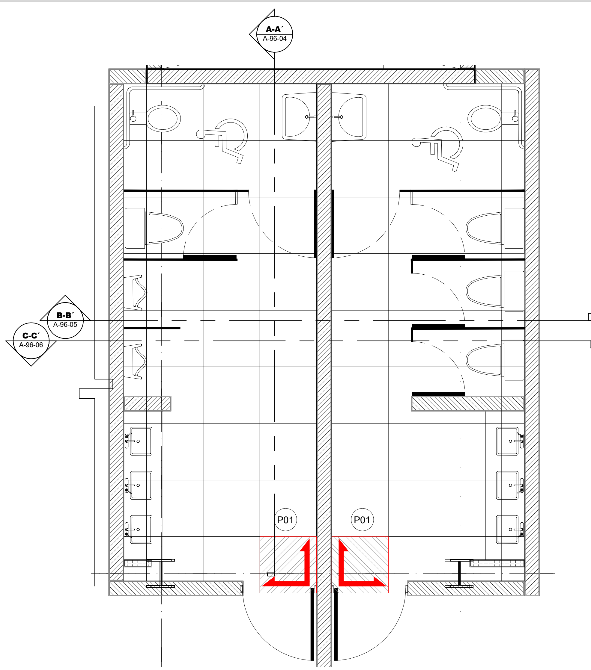
2 Planta Amueblada - Baños Esc. 1: 30
