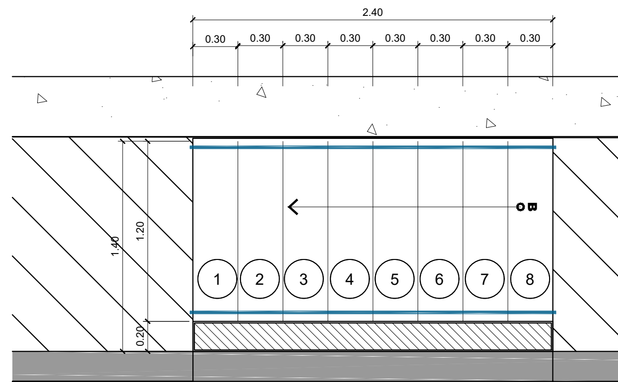
2 Detalle Escalera Lateral izquierda S3-N2M Esc. 1:25
