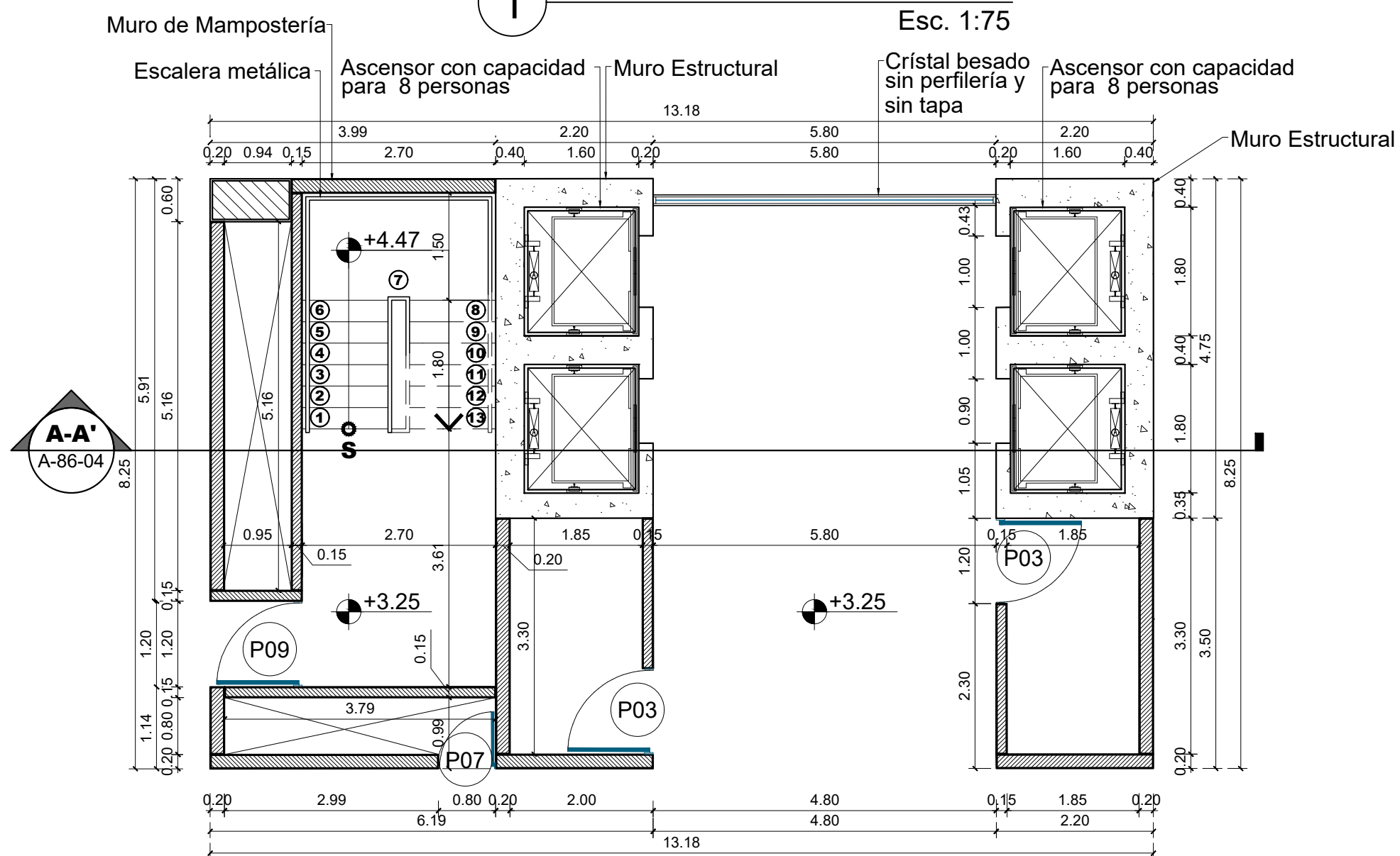
2 Planta Núcleo A - N2 a N3 Esc. 1:75
