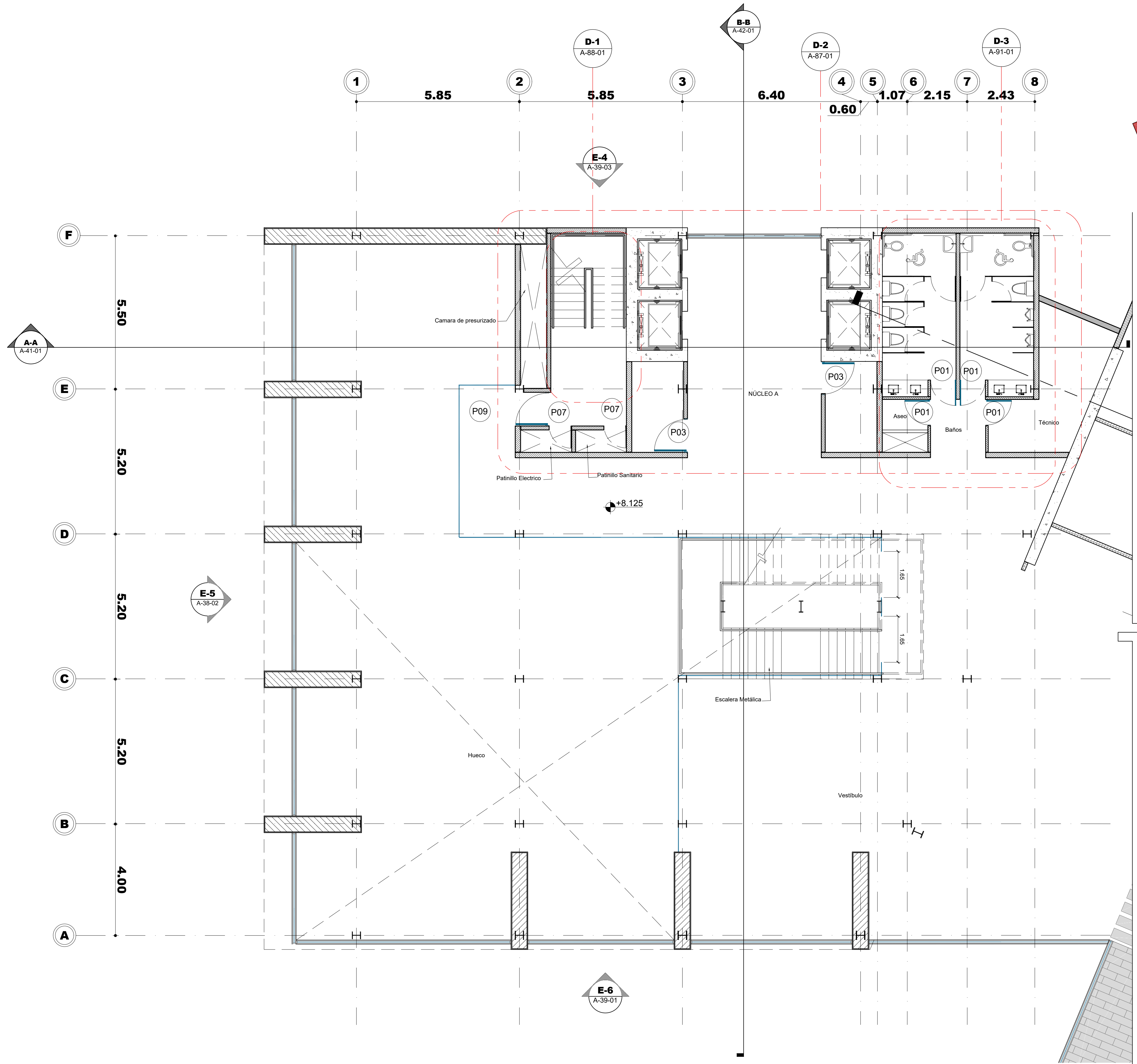
1 Planta Amueblada - Bloque 1 Nivel 3 Esc. 1:75
