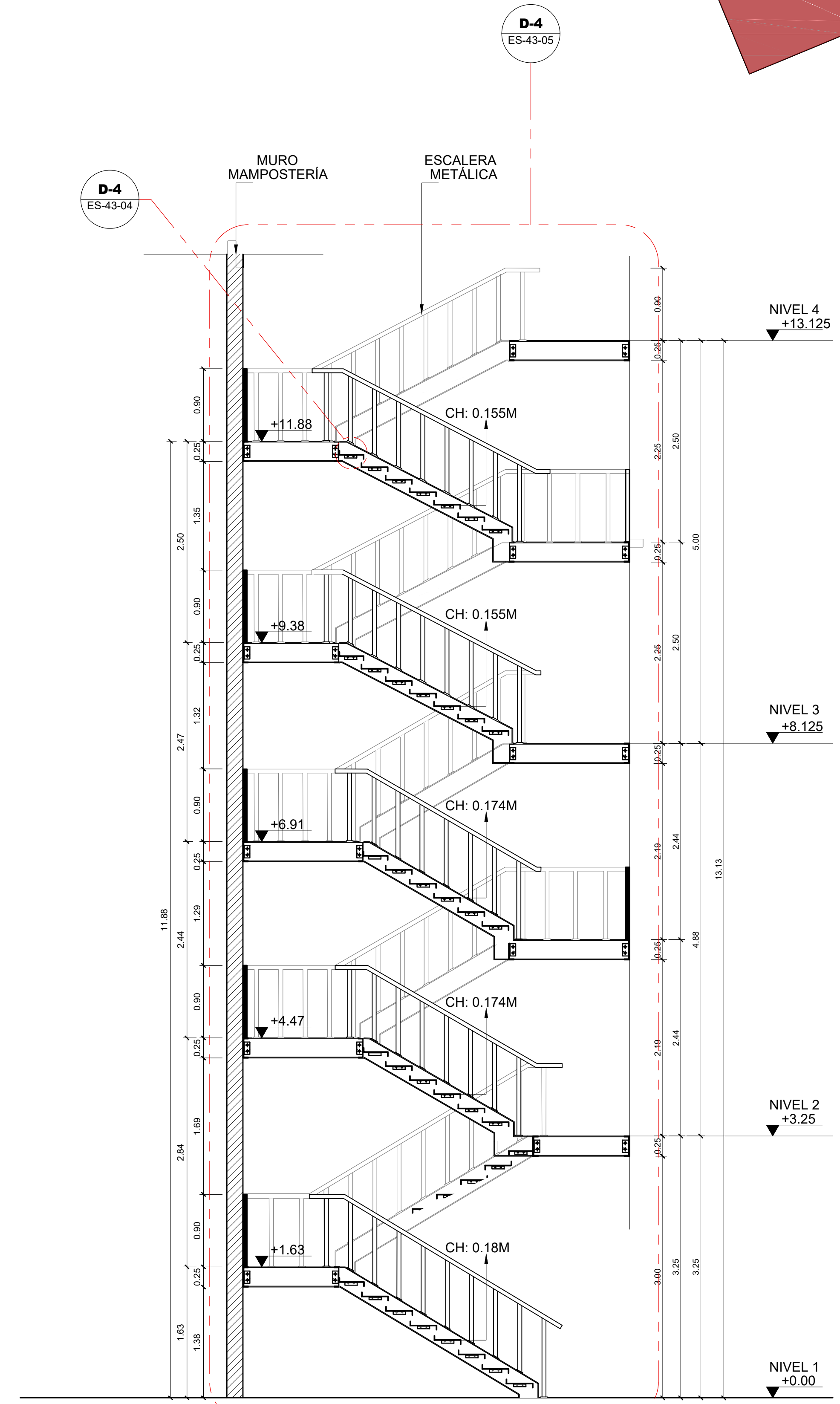
4 Sección A-A' Escalera A - Núcleo A - N1 a N4 Esc. 1:40
