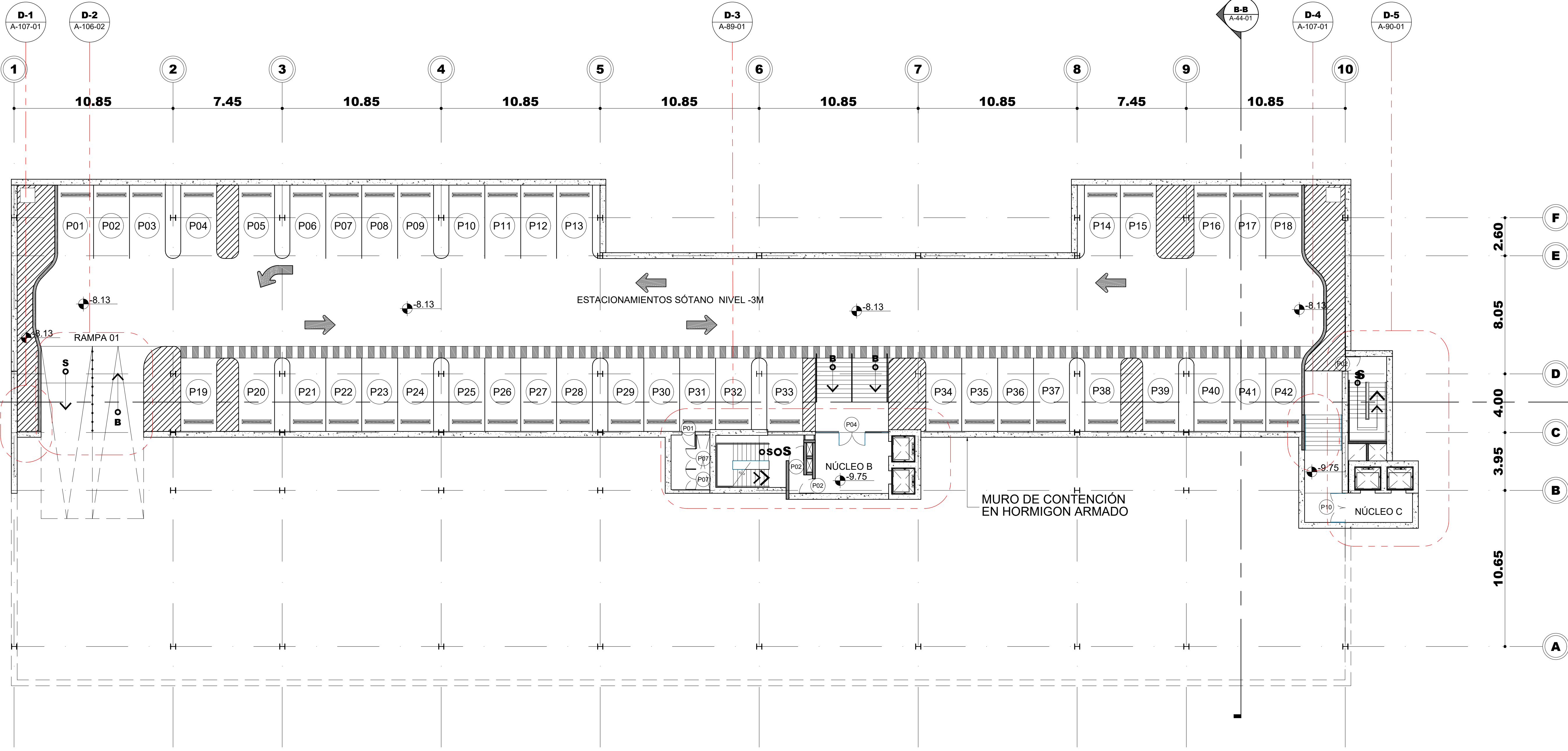
1 Planta Amueblada - Sótano 3 - Bloque 2 Esc. 1:150
