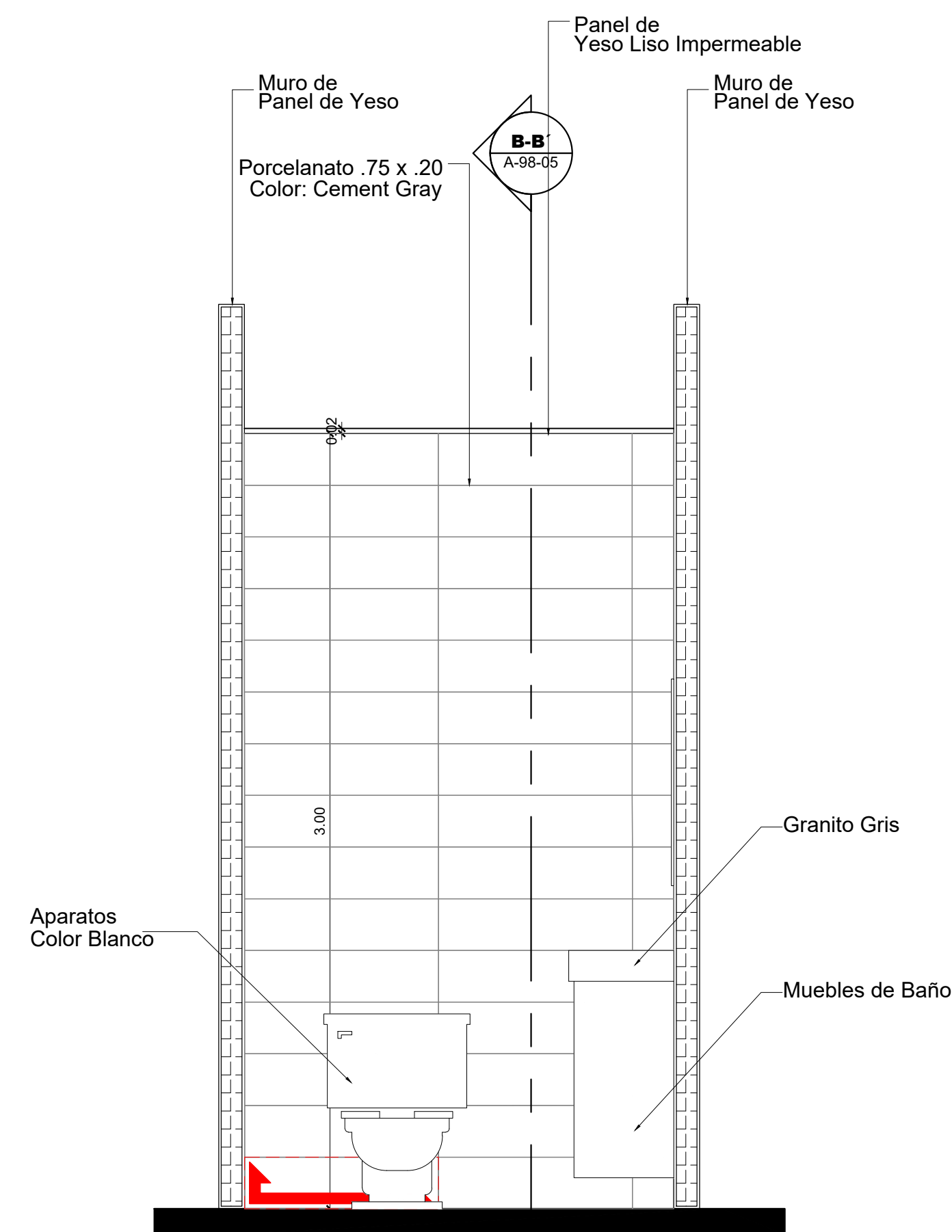
4 Sección A-A' Esc. 1: 20
