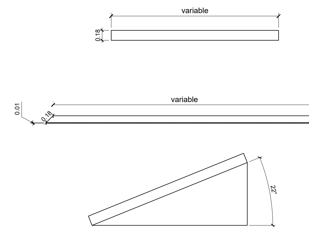
4 Detalle Típico Paneles de Louvers Esc. 1:40
