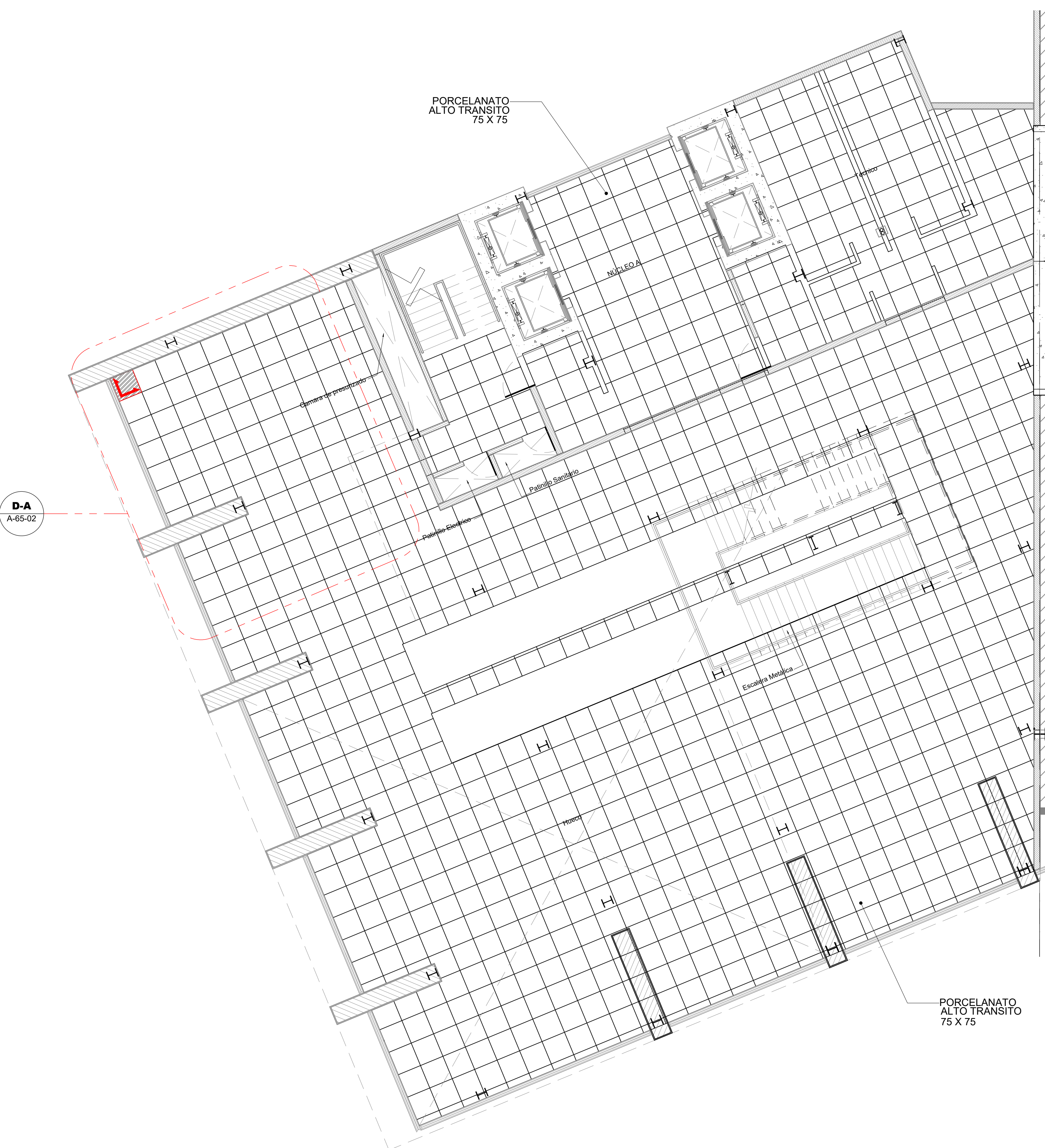
1 Planta Pisos - Bloque 1 - Nivel 2 Esc. 1:75
