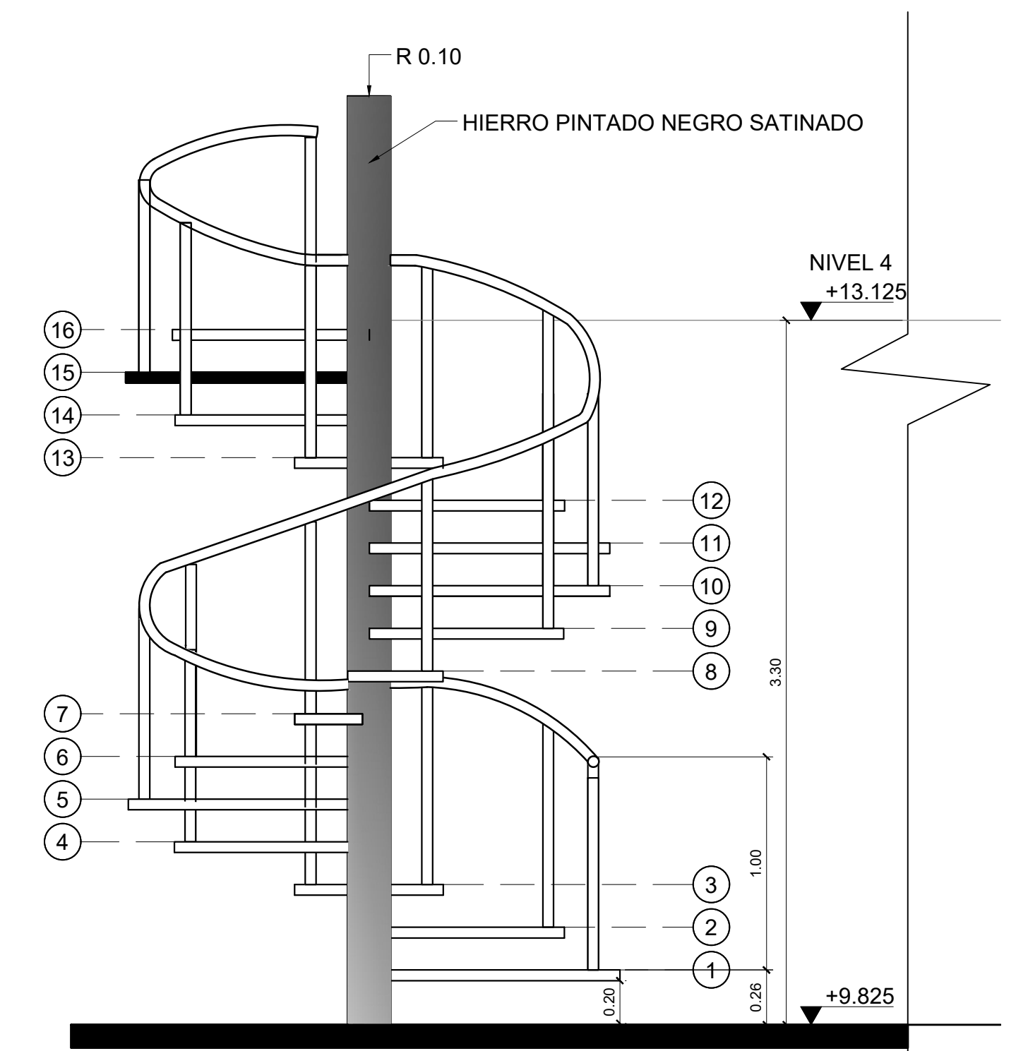
8 Elevación Escalera de Auditorio, N3 y N4 Esc. 1:25
