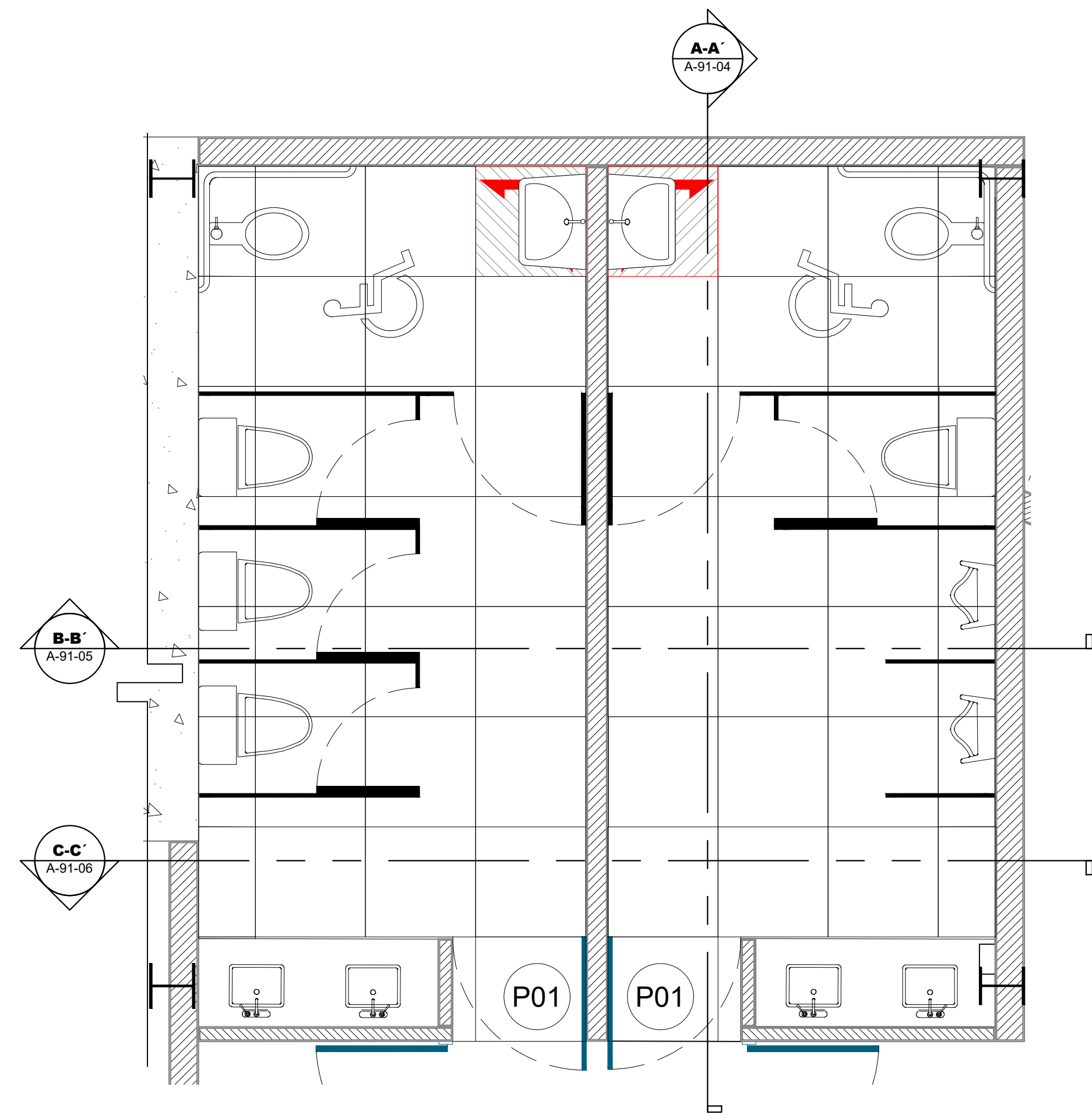
2 Planta Amueblada - Baños Esc. 1: 30
