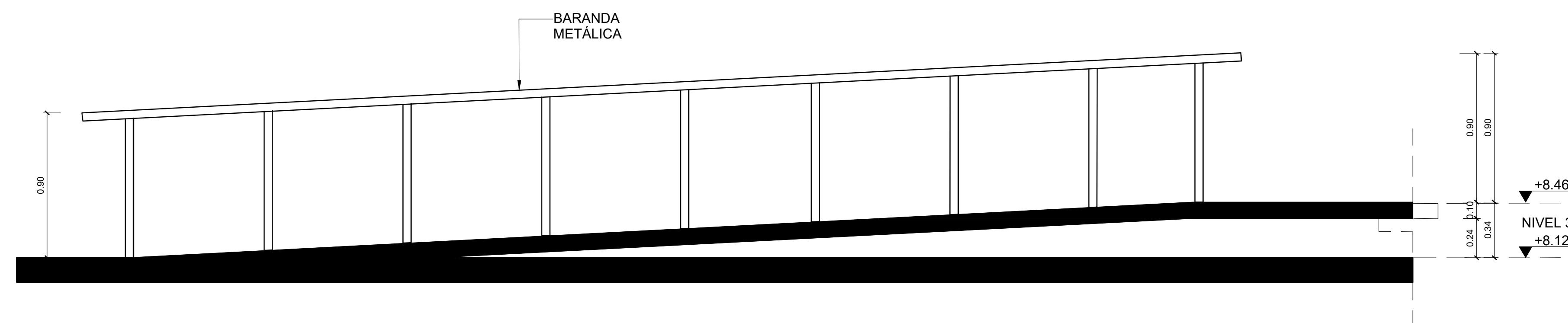
2 Sección A-A' Rampa Sala de Audiencia - N3 Esc. 1:20
