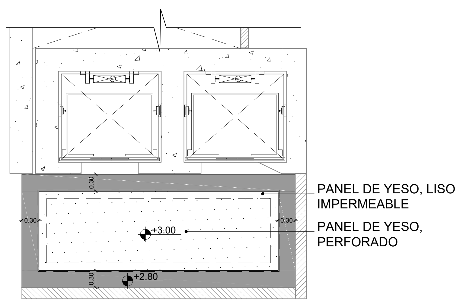
3 Detalle 2, Planta de Plafón, Nucleo C Esc. 1:40
