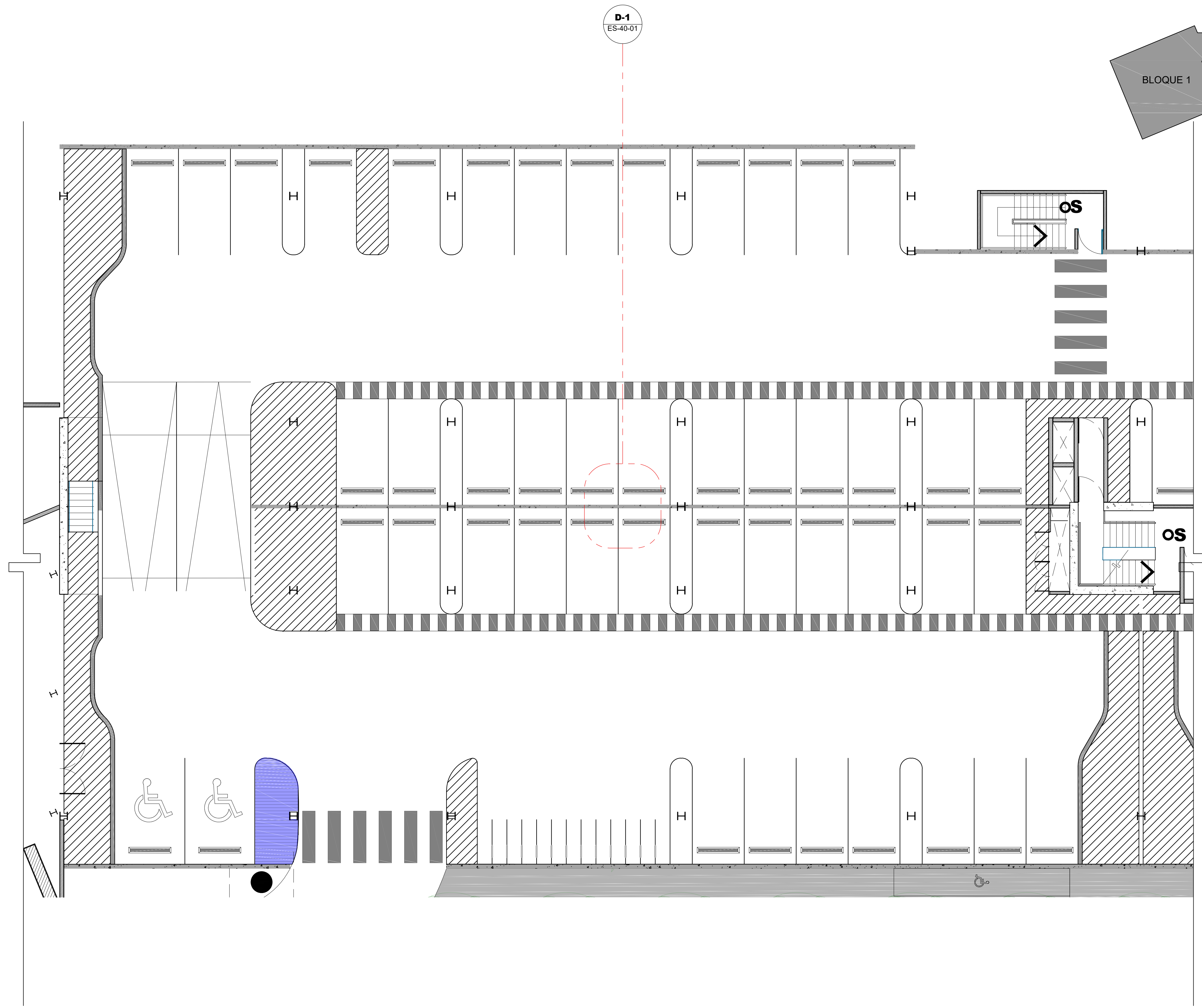
1 Planta Muros Bloque 2A- Nivel 1 Esc. 1:100
