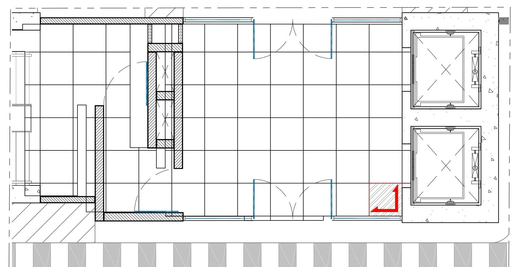
3 Detalle B Esc. 1:50
