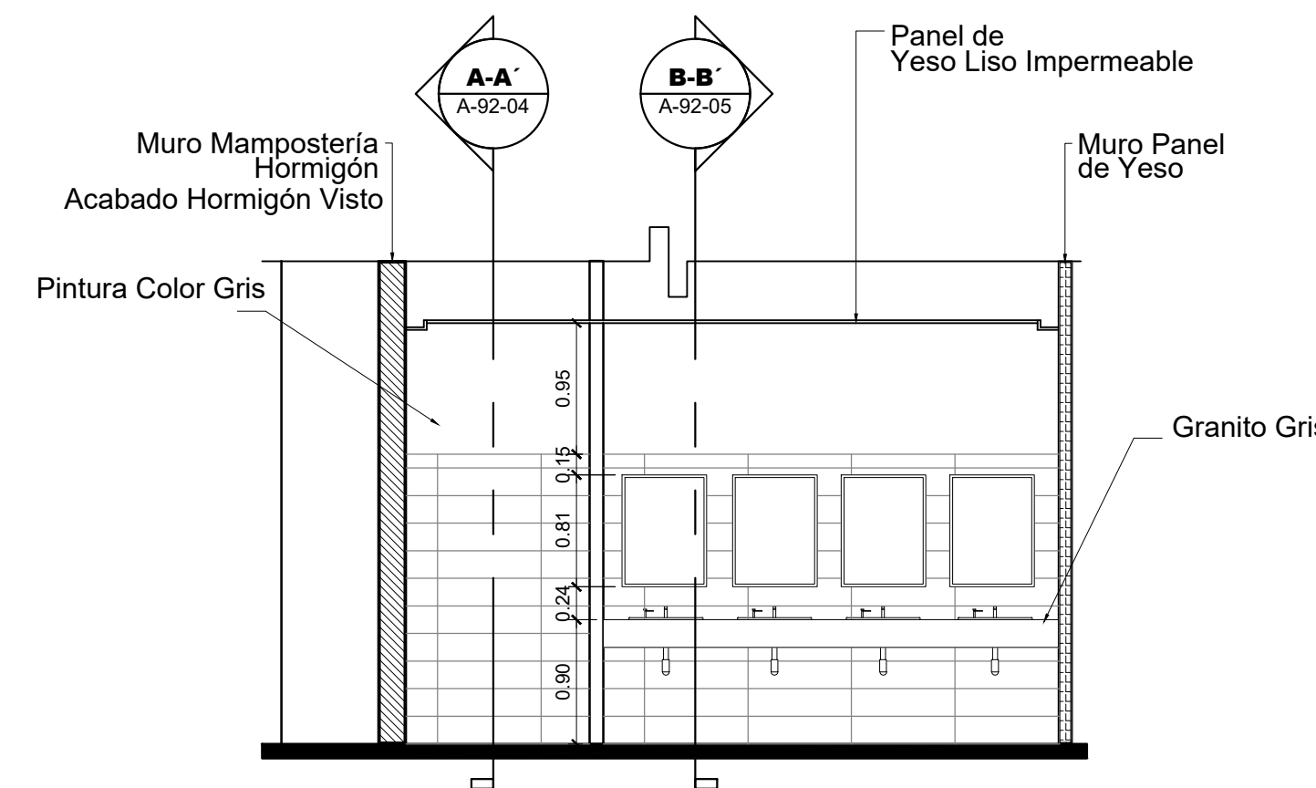
6 Sección C-C' Esc. 1: 50
