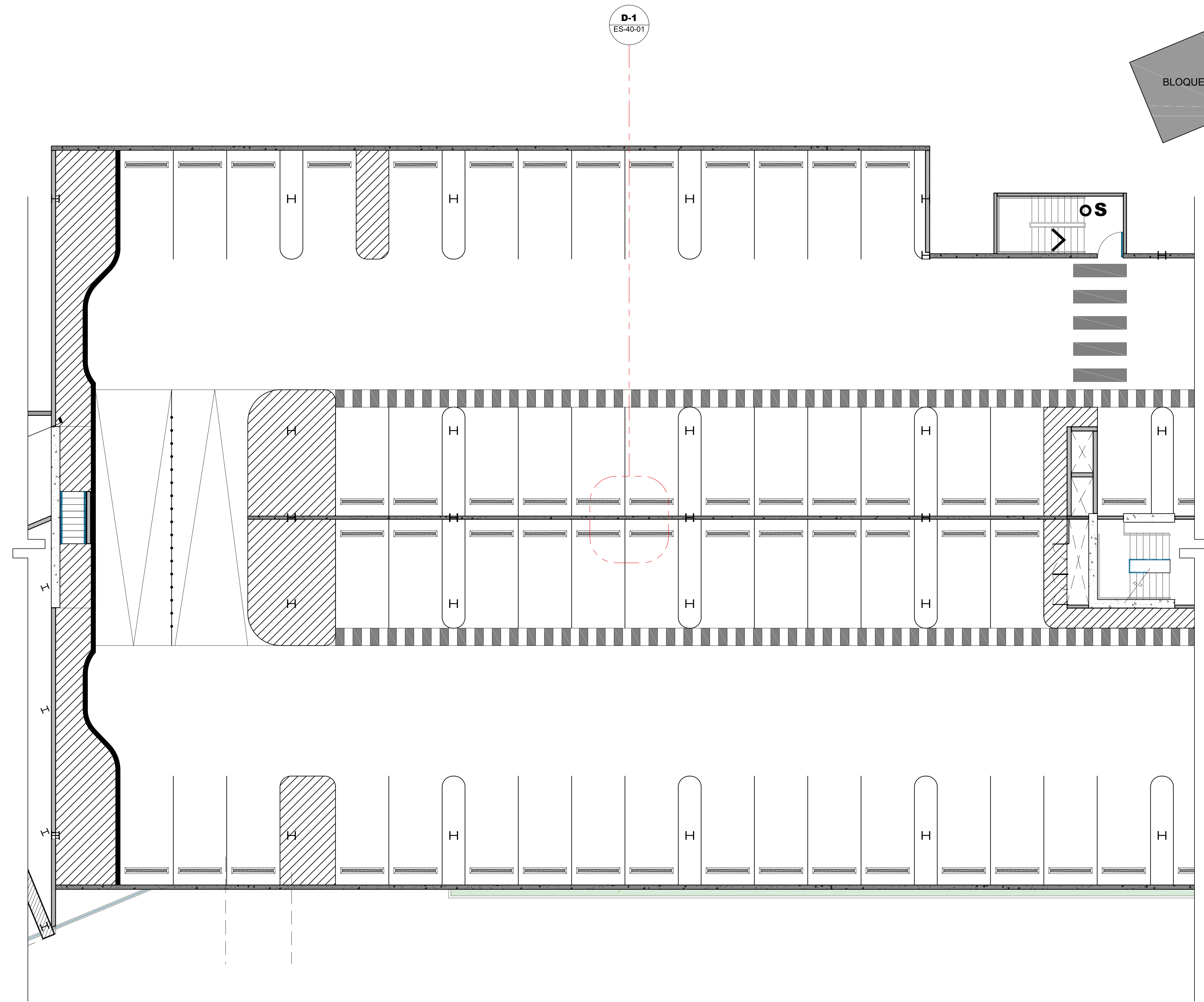
1 Planta Muros Bloque 2A - Nivel 2 Esc. 1:100
