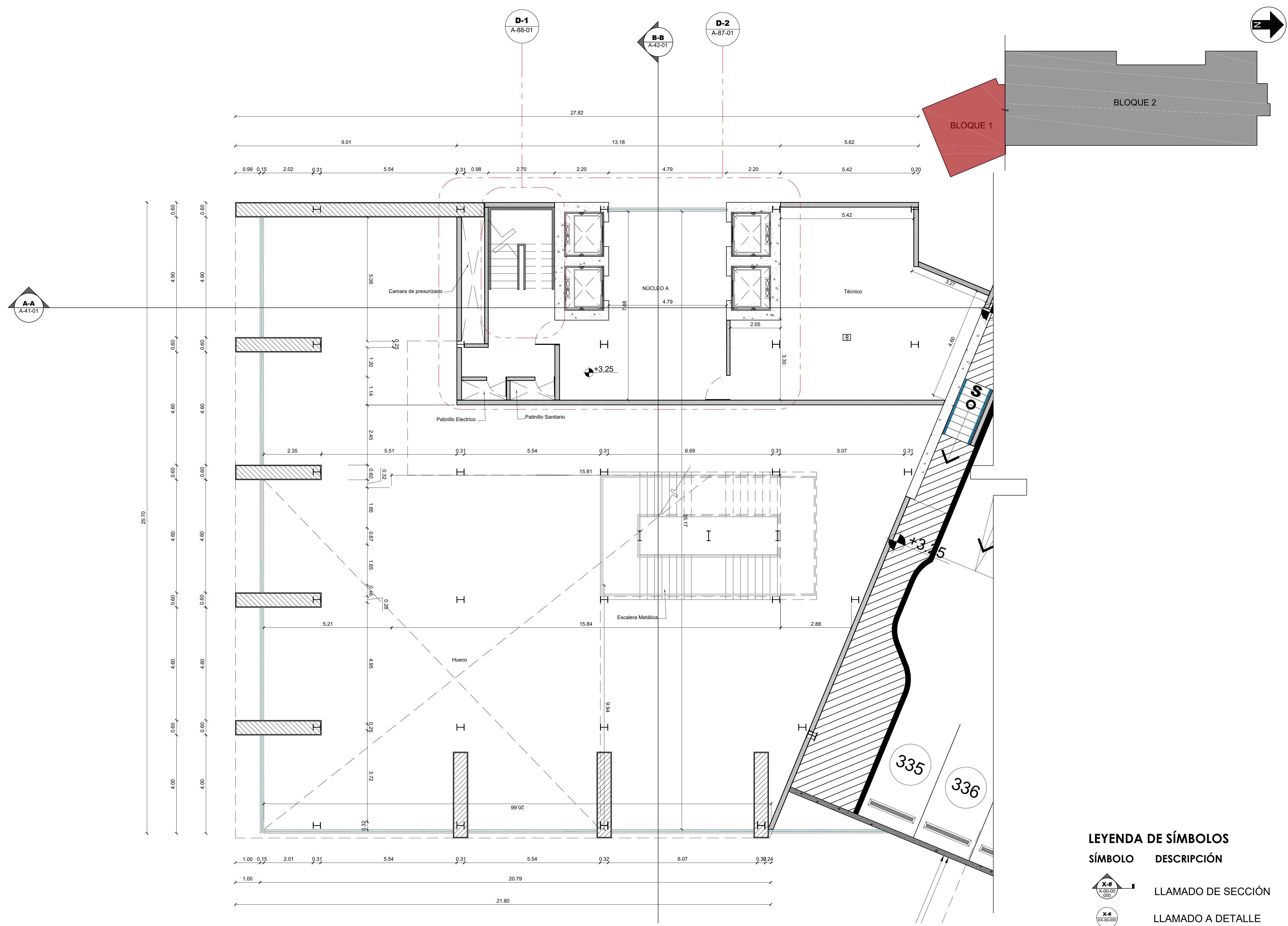
1 Planta Dimensionada Nivel 2 - BLOQUE 1 Esc. 1:75
