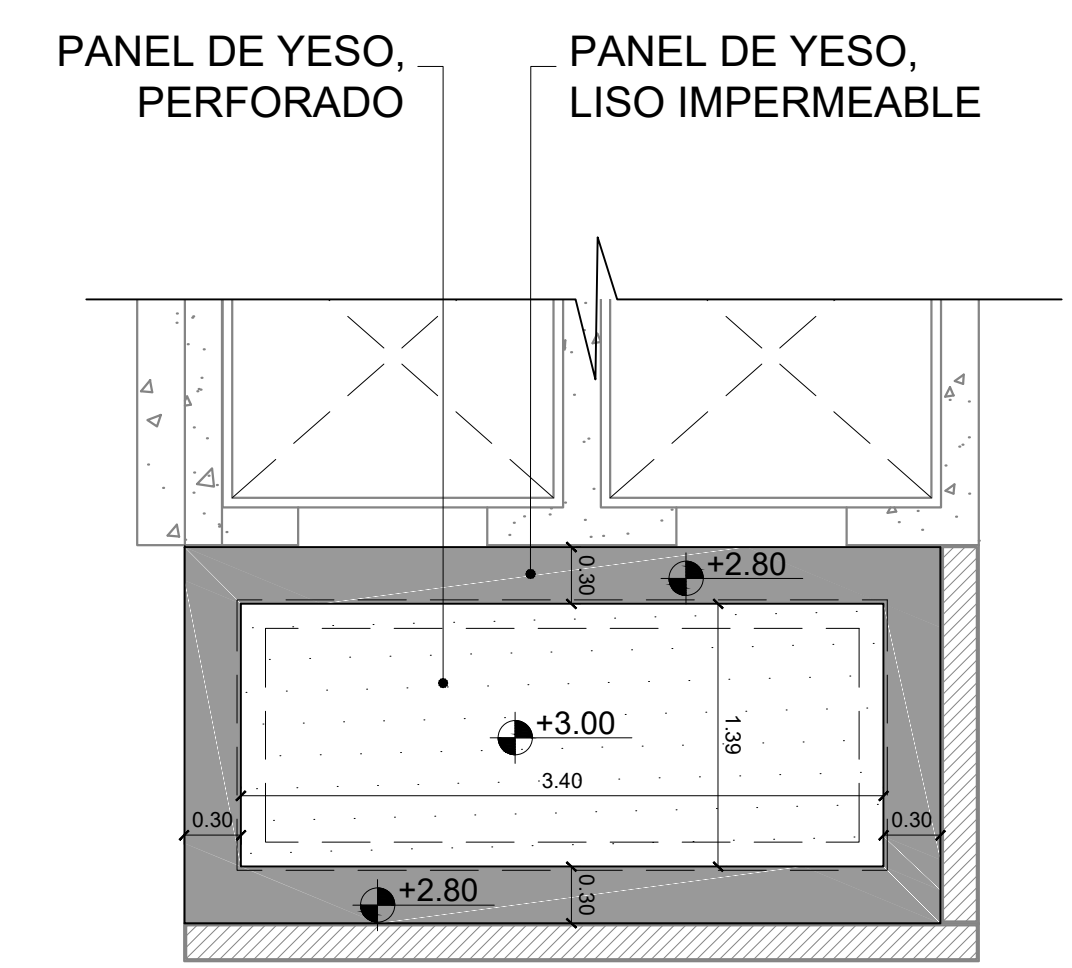
4 Detalle 3, Planta de Plafón, Nucleo C Esc. 1:40
