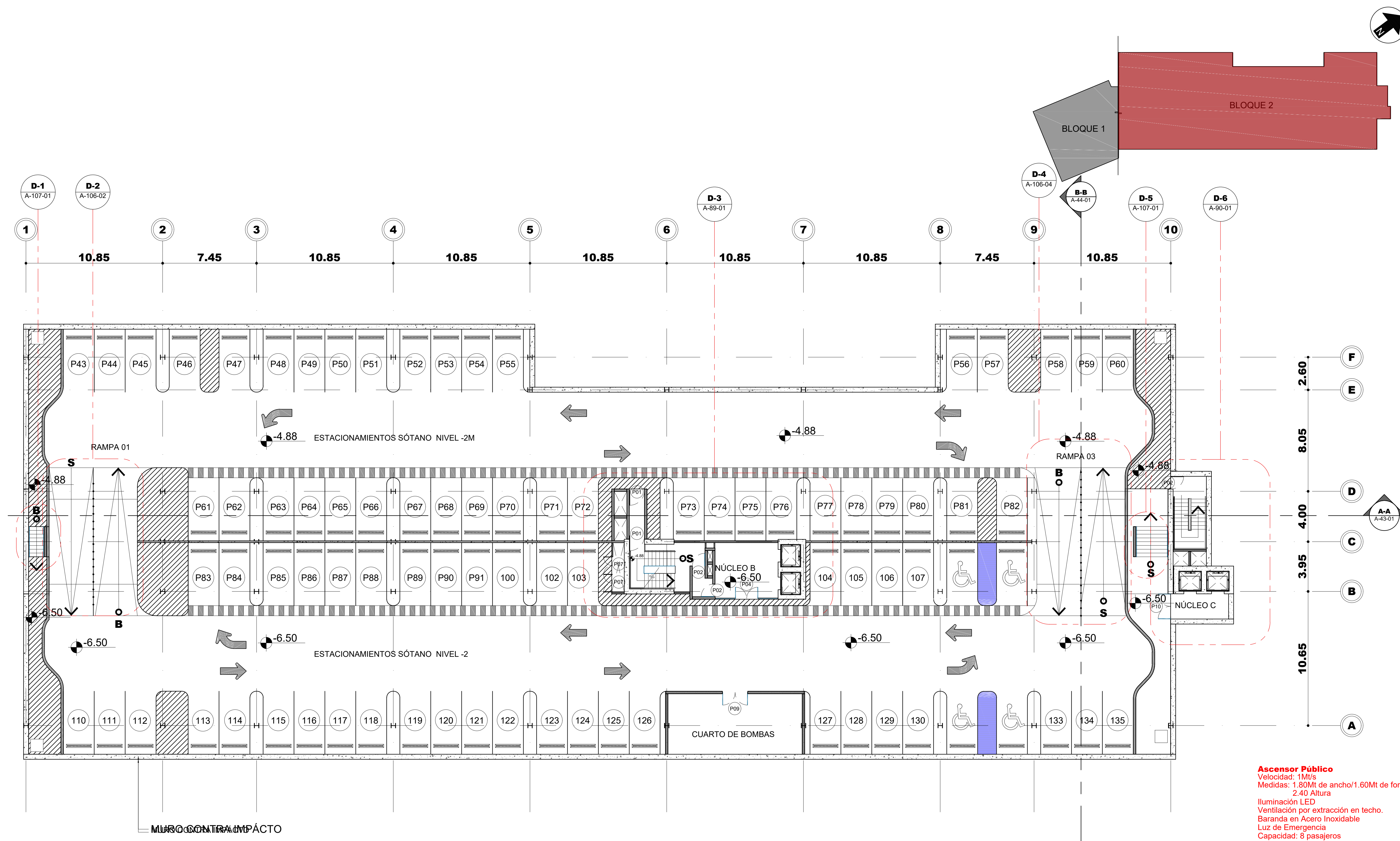
1 Planta Amueblada - Sótano 2 - Bloque 2 Esc. 1:150
