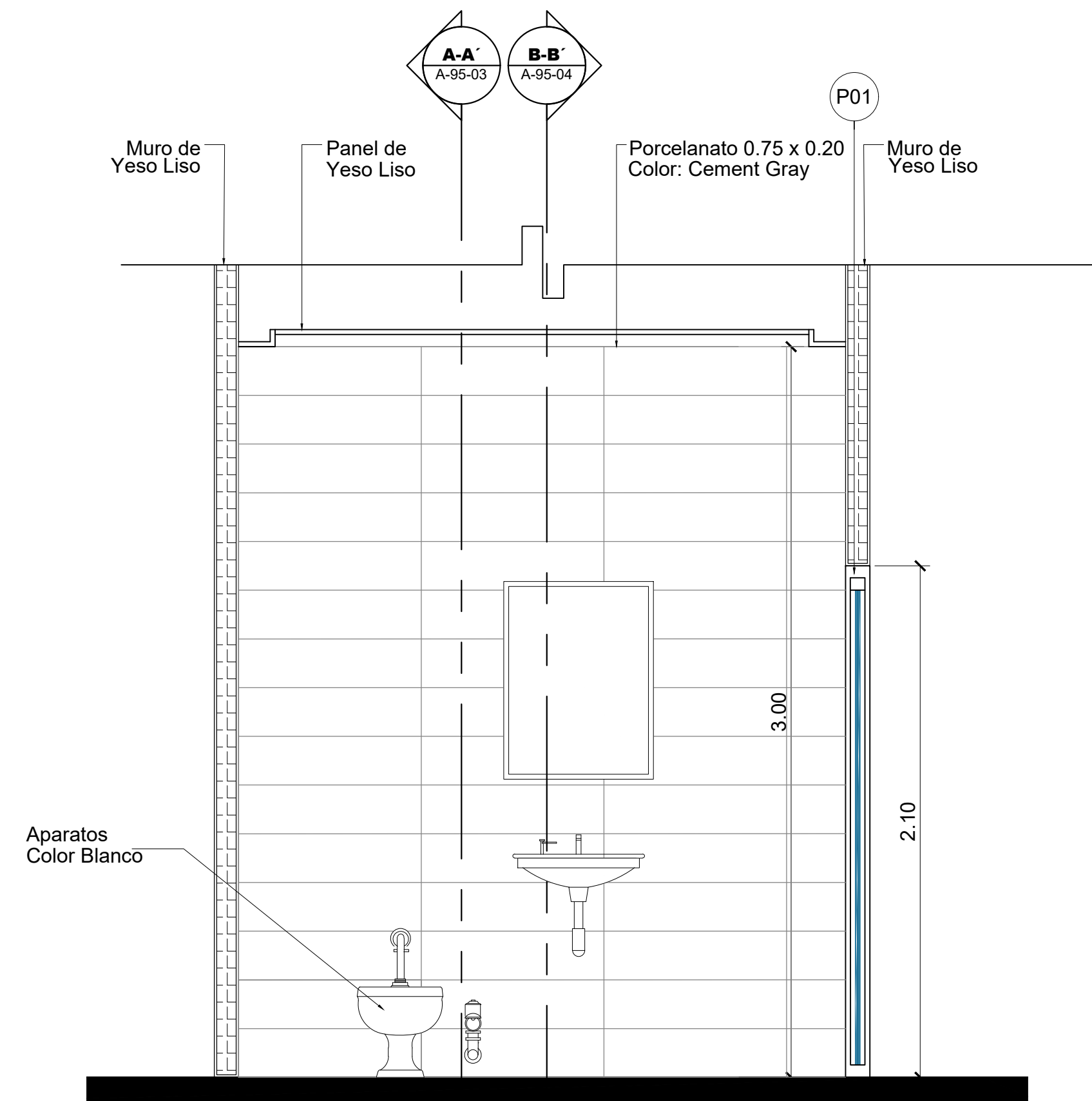
5 Sección C-C' Esc. 1: 20
