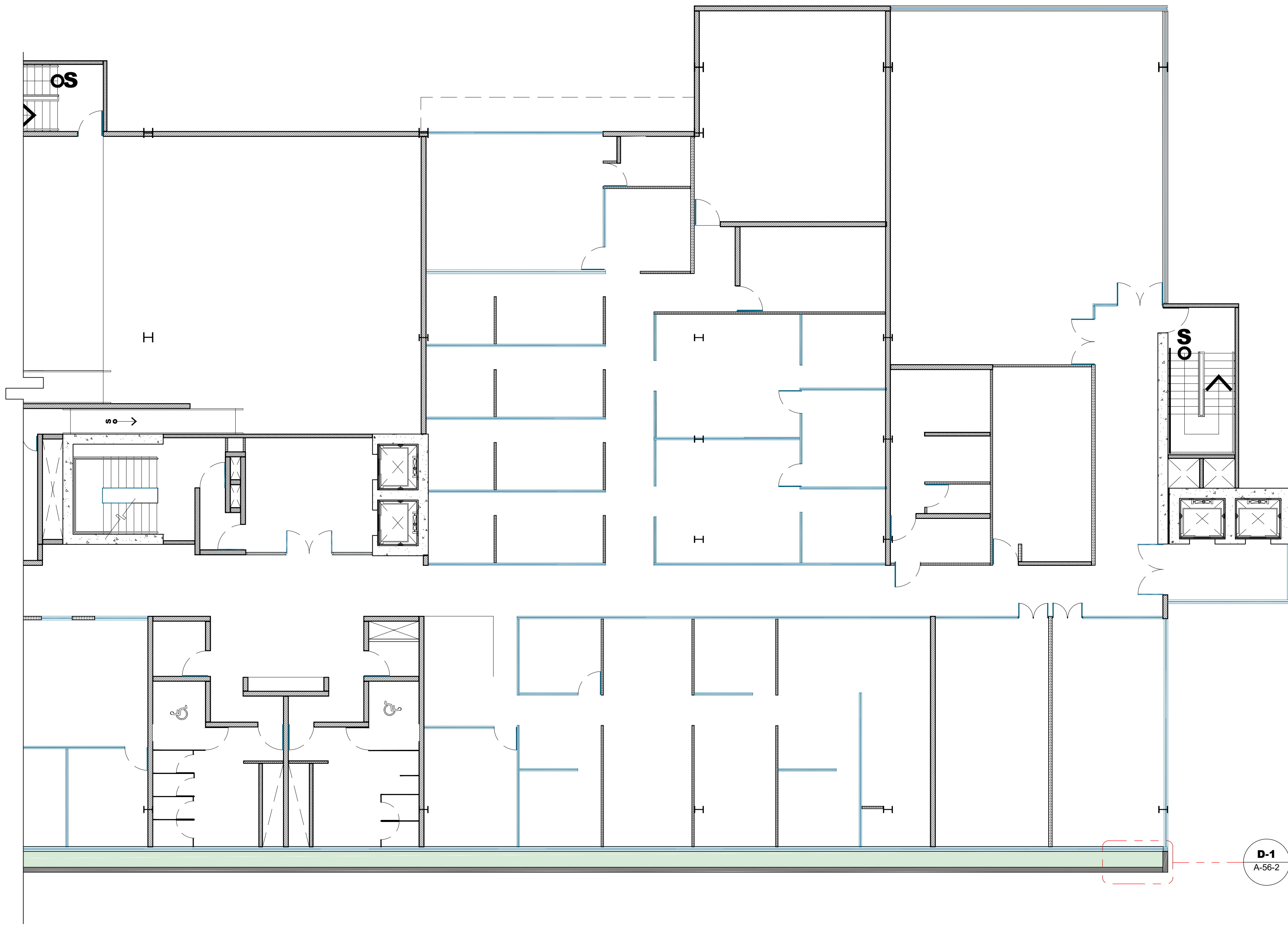
1 Planta Muros Bloque 2B - Nivel 3 Esc. 1:100
