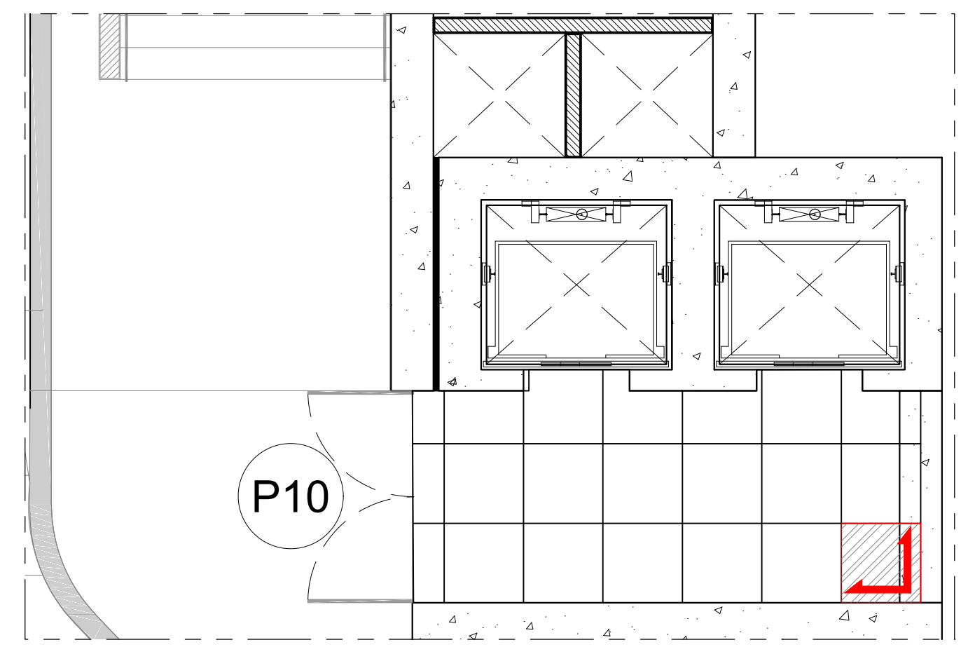
3 Detalle B Esc. 1:50
