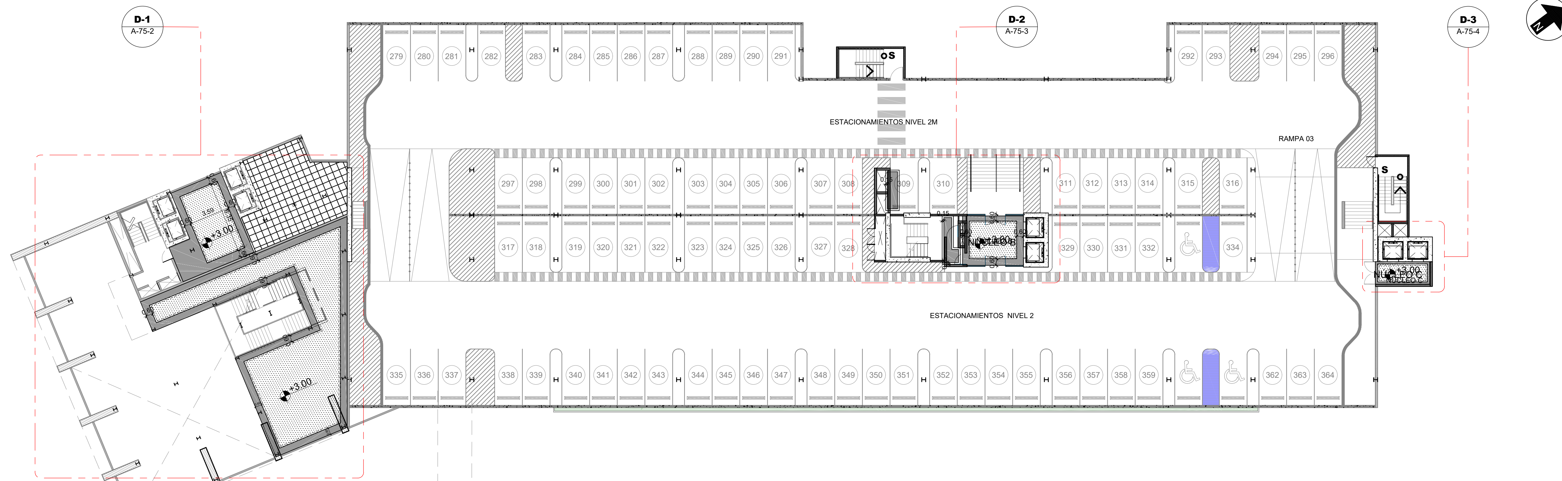
1 Planta Plafones - Nivel 2 Esc. 1:200
