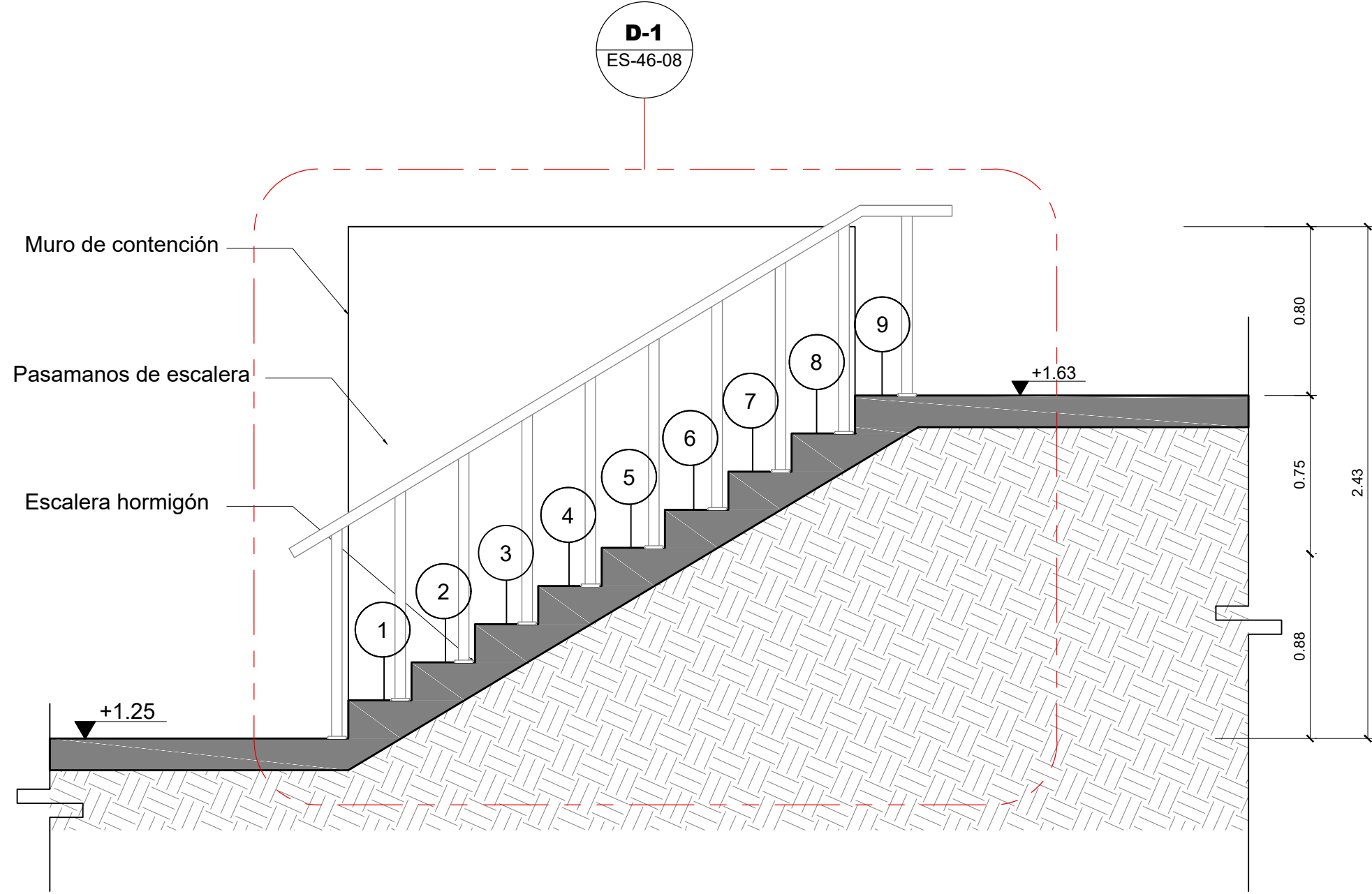
3 Sección Escalera en Parquesos S3-N2M Esc. 1:25
