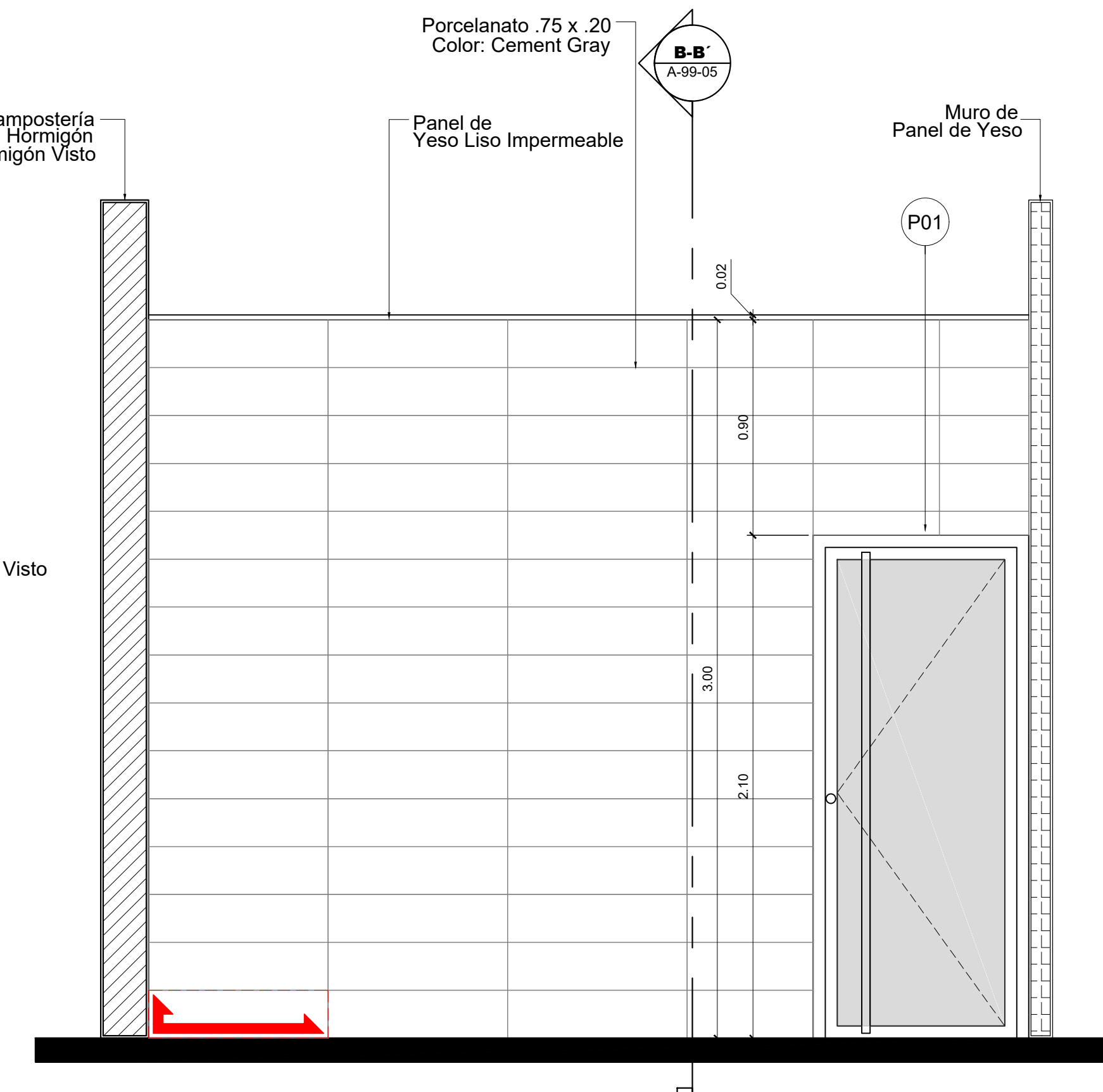
6 Sección C-C' Esc. 1: 20
