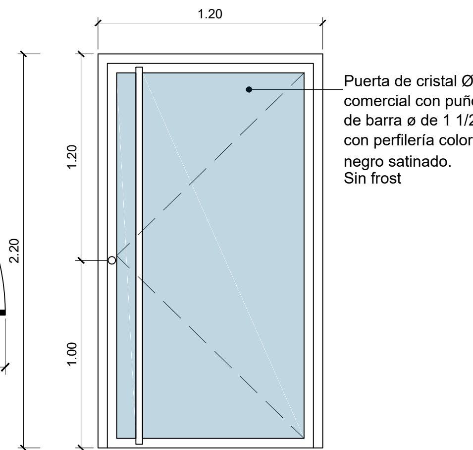
3 Puerta P03 ESCALA 1:20
