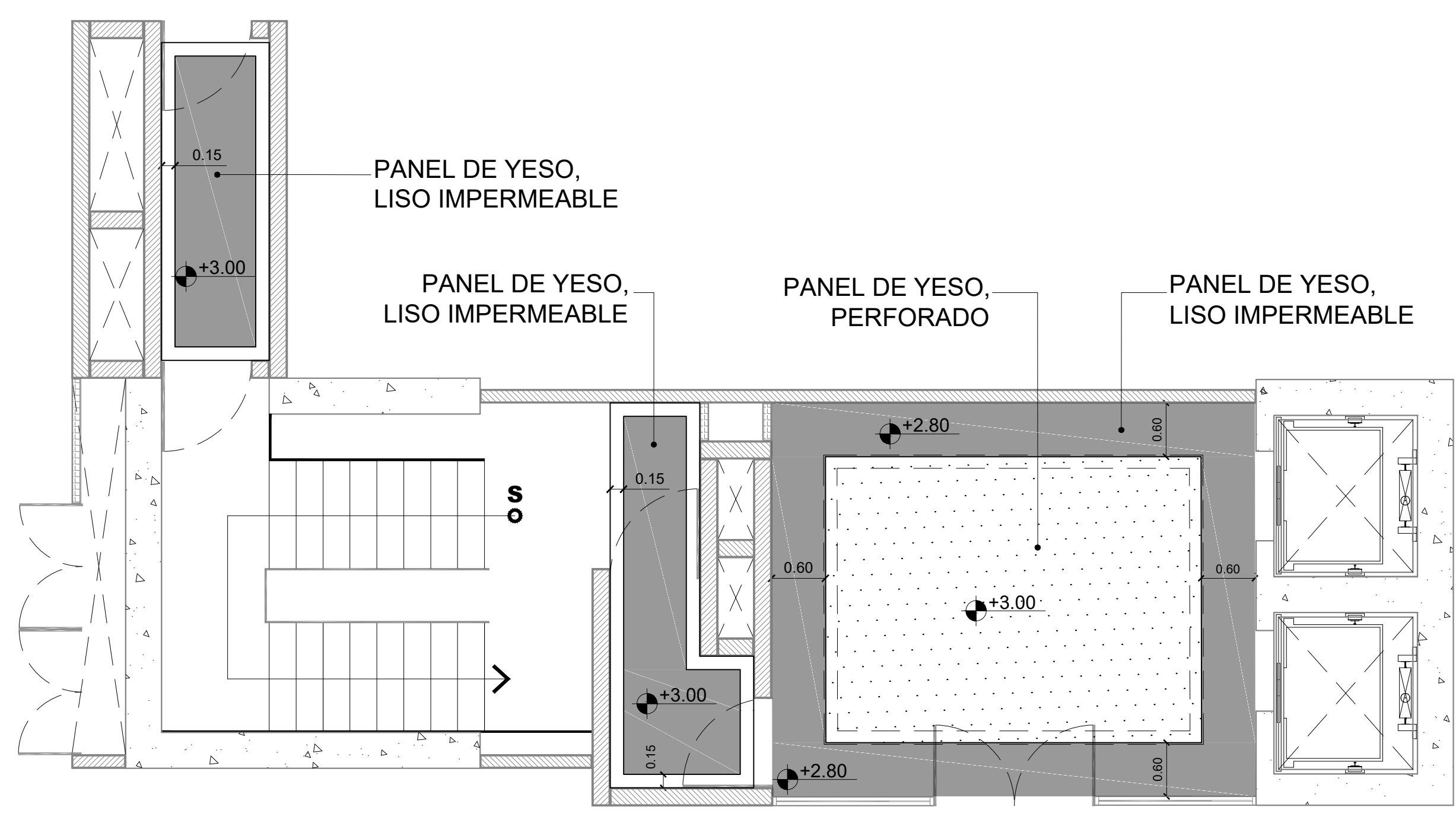
2 Detalle 2, Planta de Plafón, Nucleo B Esc. 1:50
