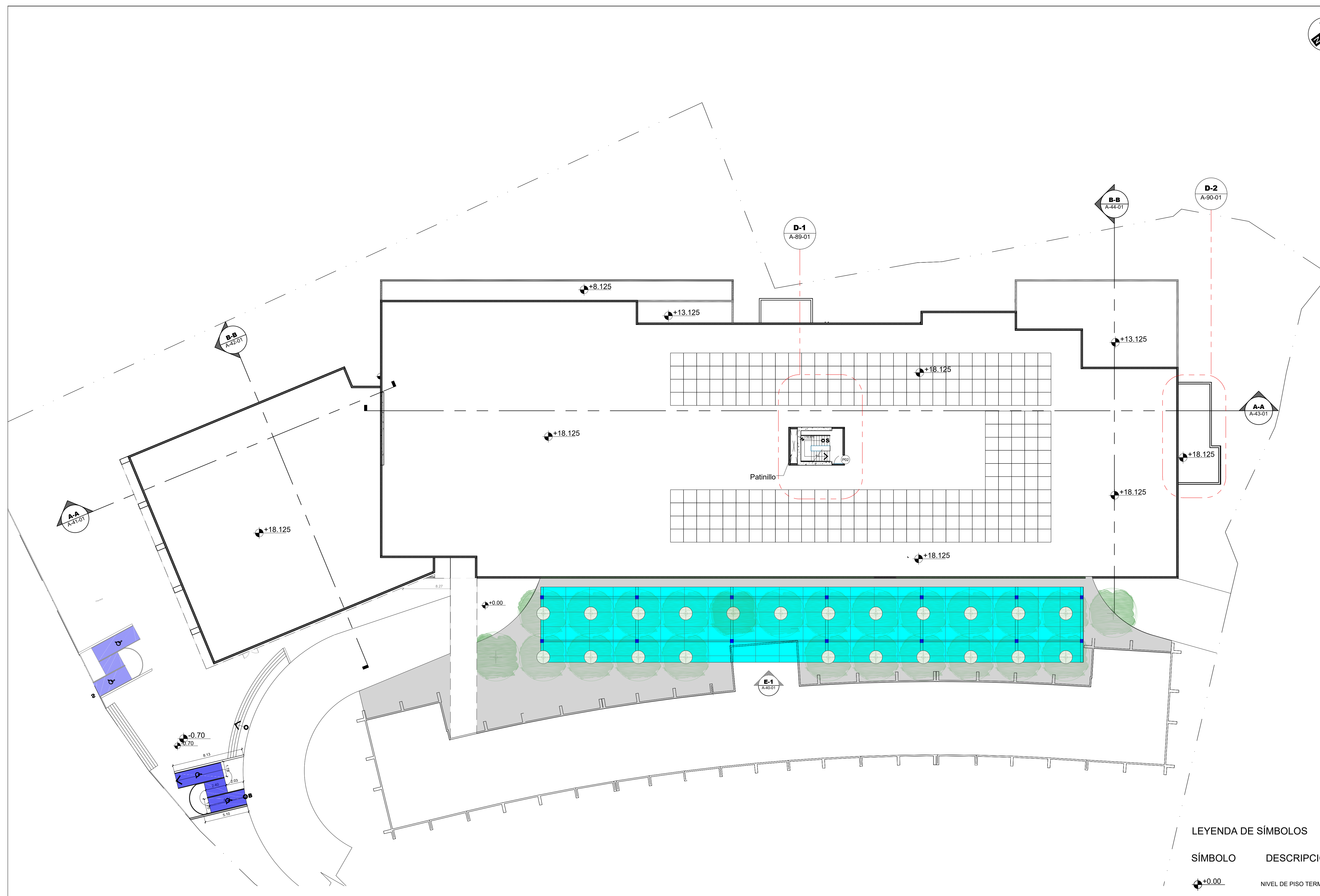
1 Planta de Azotea Esc. 1:200
