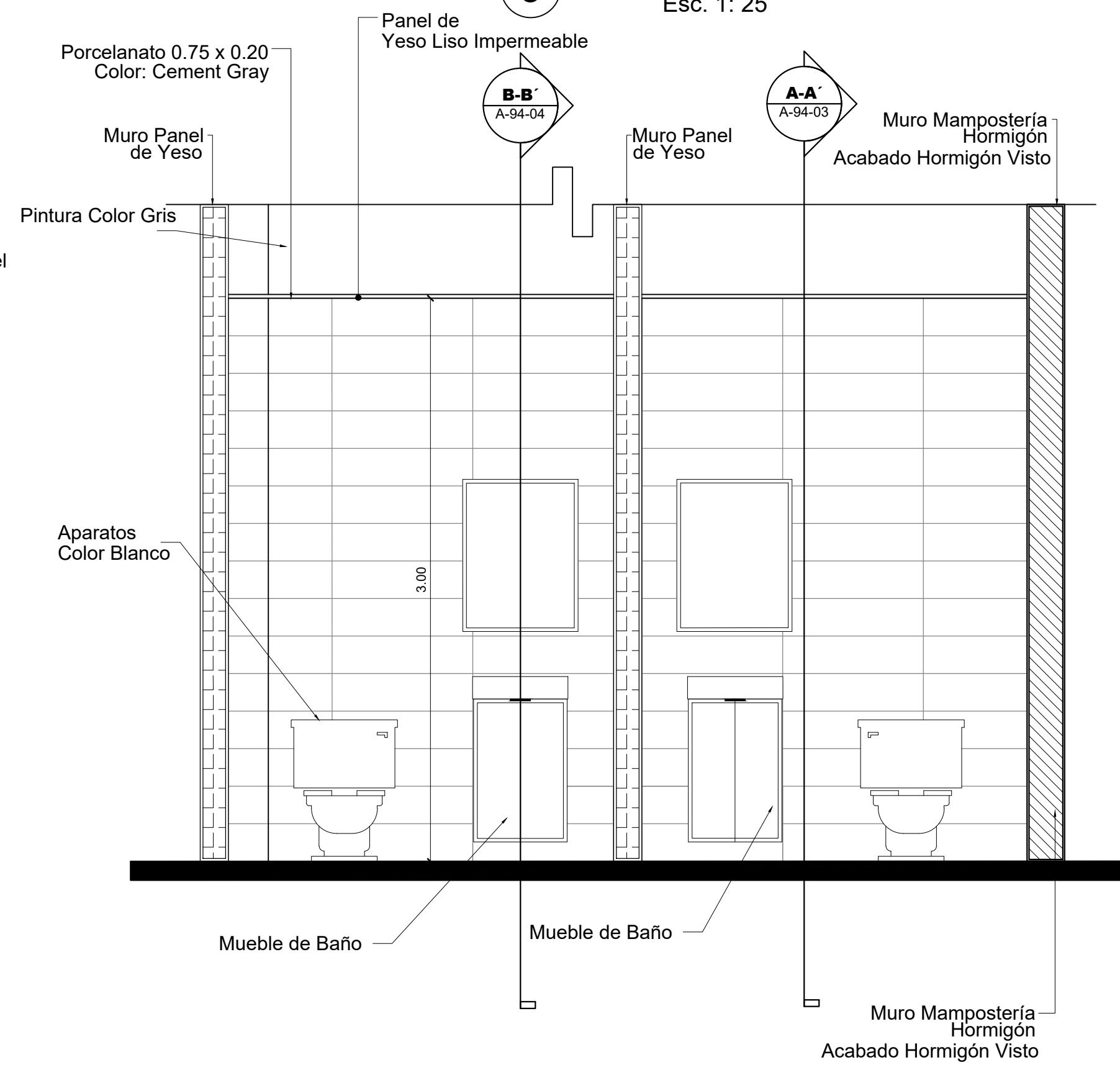
6 Sección D-D' Esc. 1: 25
