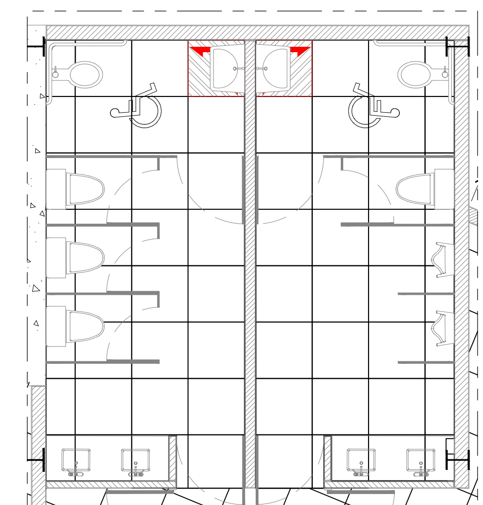
2 Detalle A Esc. 1:50
