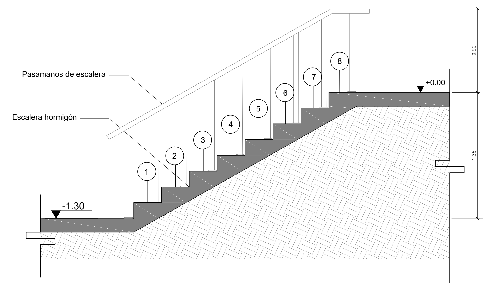
5 Sección Escalera Gran Plaza - N1 Esc. 1:20
