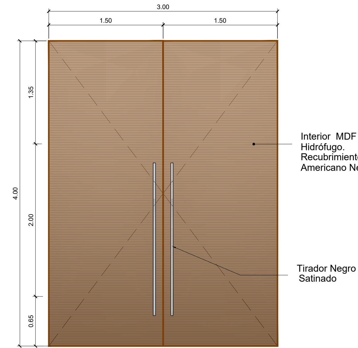
7 Puerta P06 ESCALA 1:30
