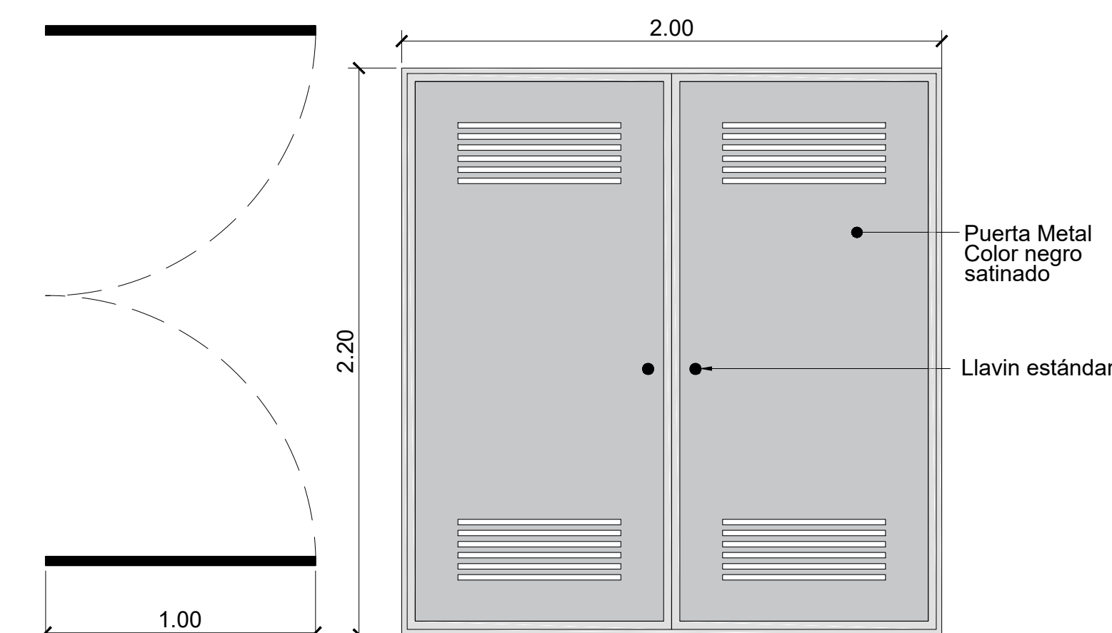
12 Puerta P09 ESCALA 1:20
