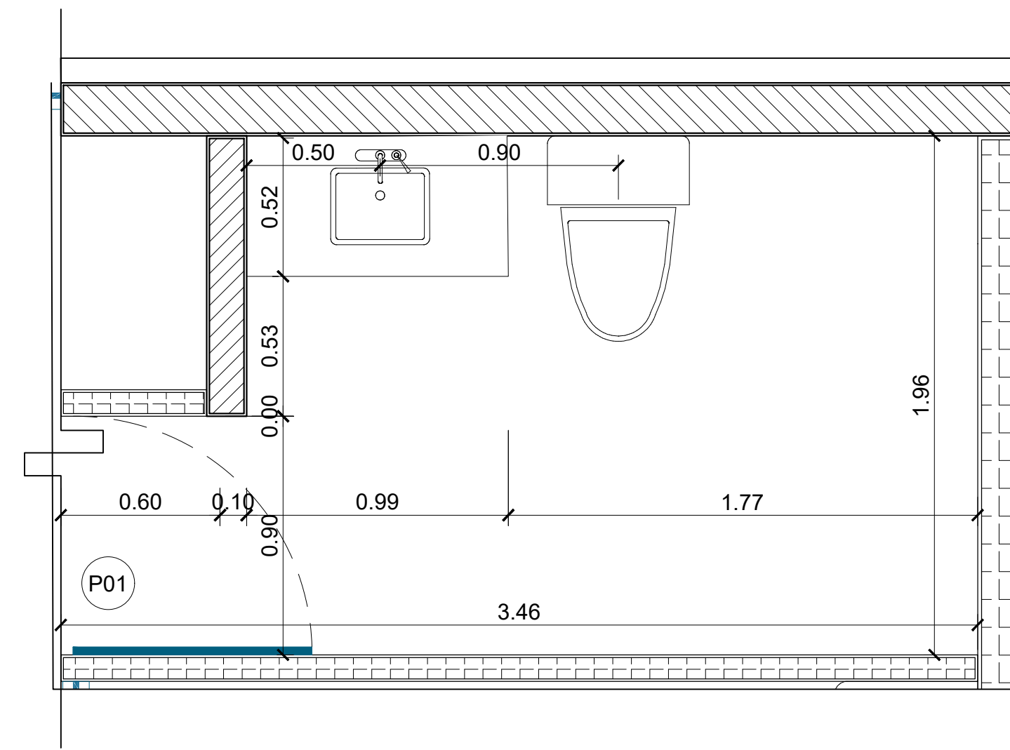
2 Planta Dimensionada - Baños Esc. 1: 20
