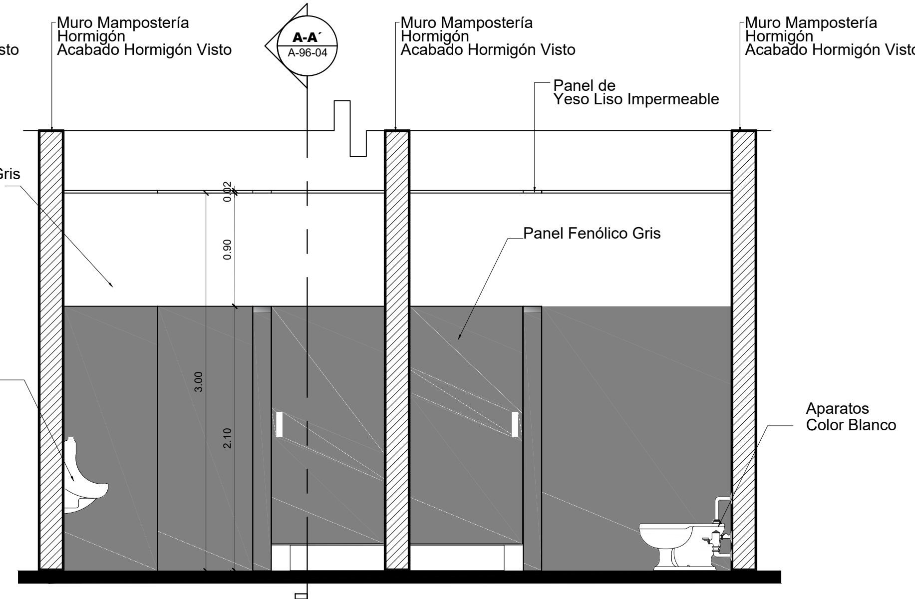
5 Sección B-B' Esc. 1: 30
