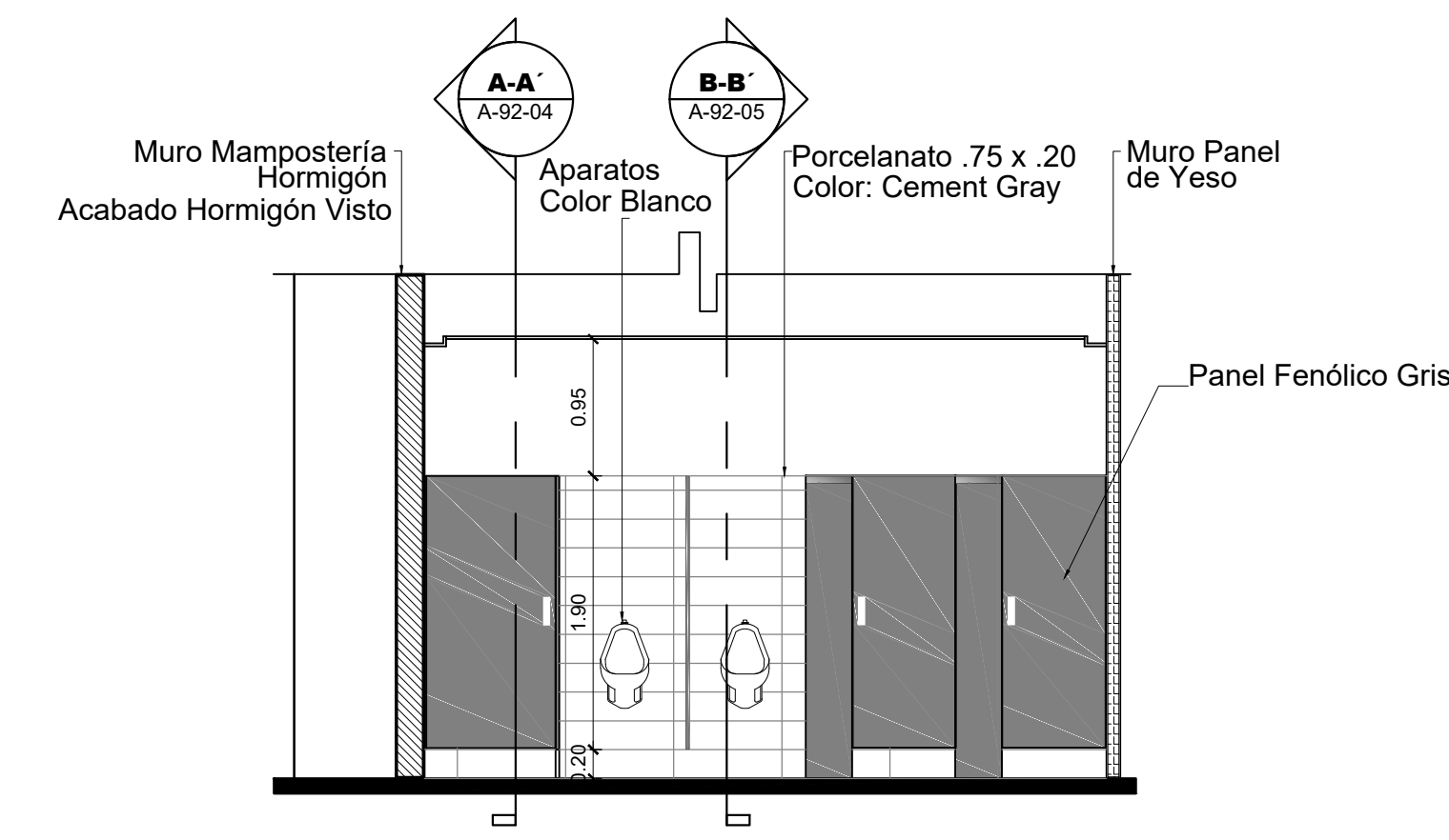
7 Sección D-D' Esc. 1: 50
