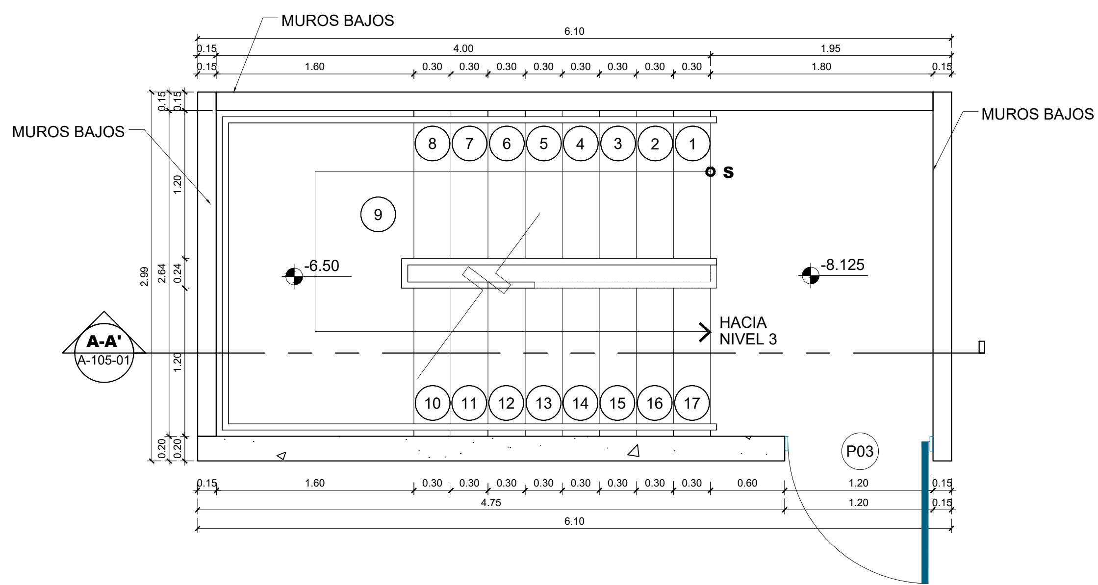
1 Planta Escalera Sala de Audiencia S3M - N3 Esc. 1:30
