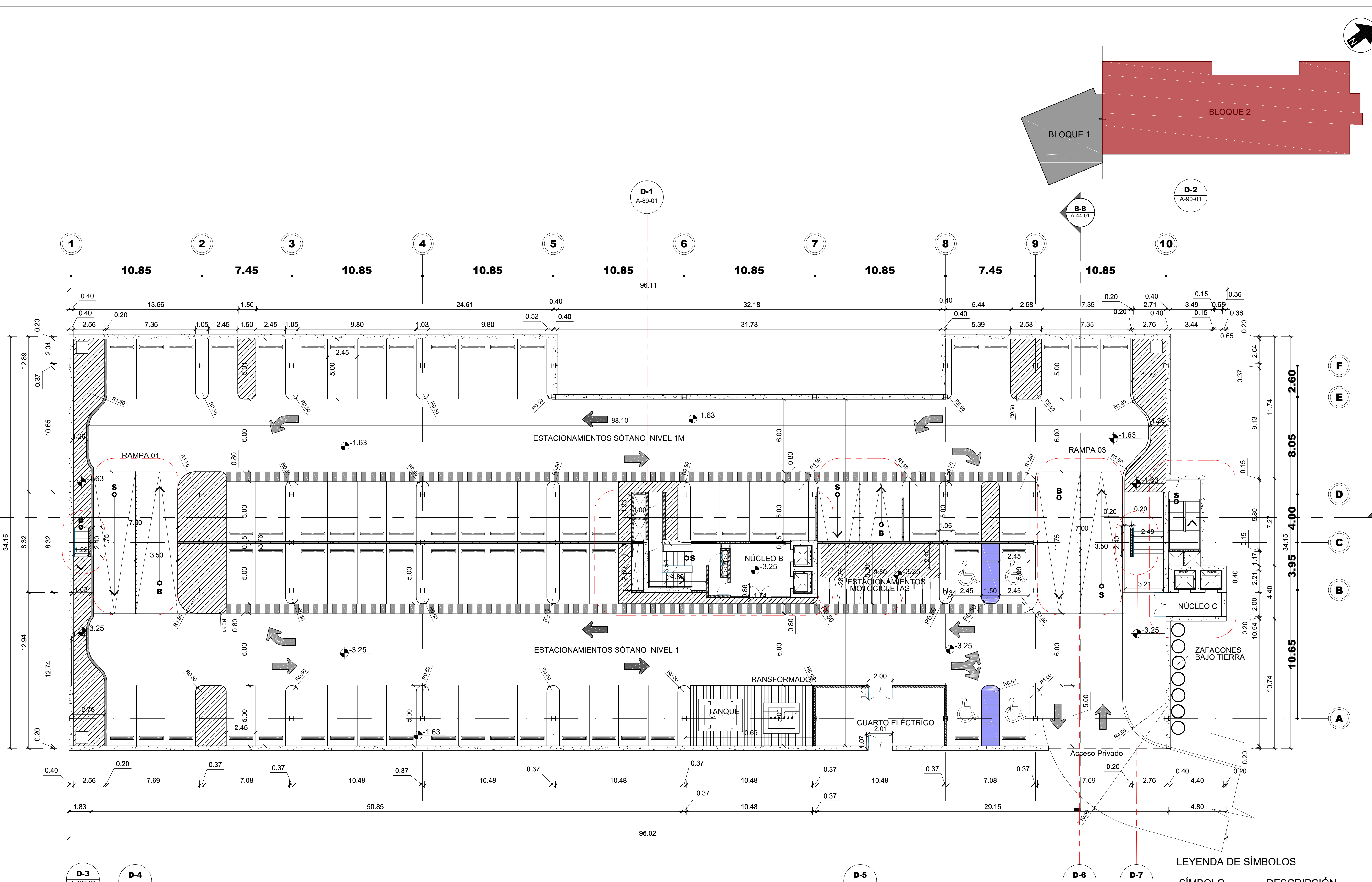
1 Planta Dimensionada - Sótano 1 Esc. 1:150
