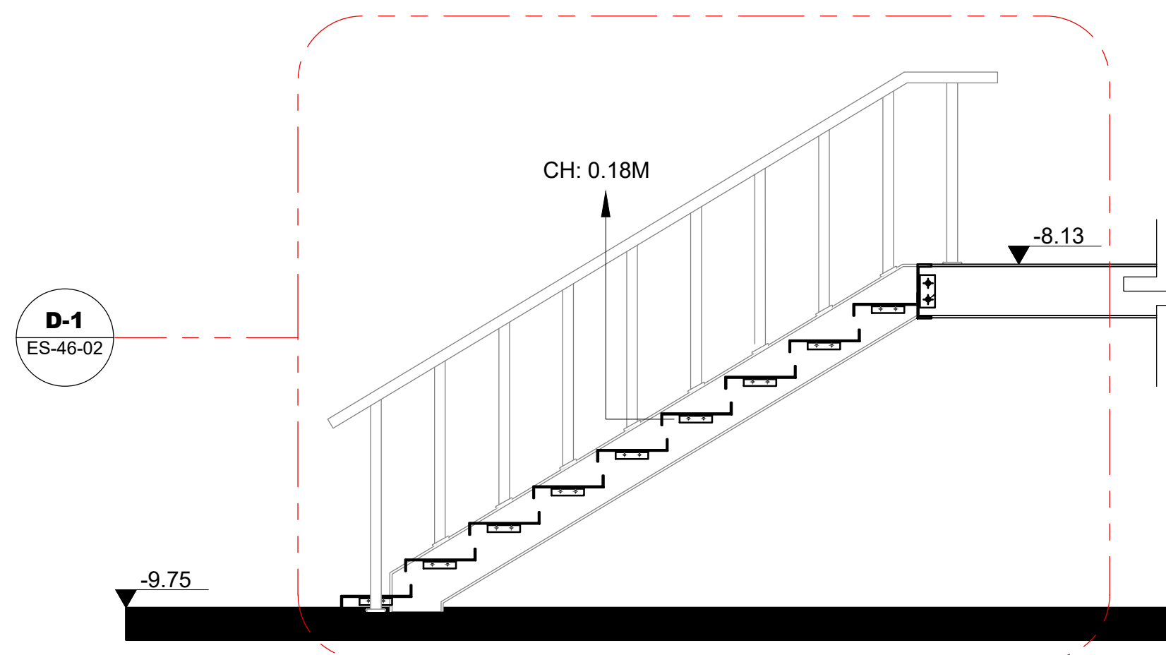
4 Detalle Escalera de acceso En niveles S3 y N2 Esc. 1:40
