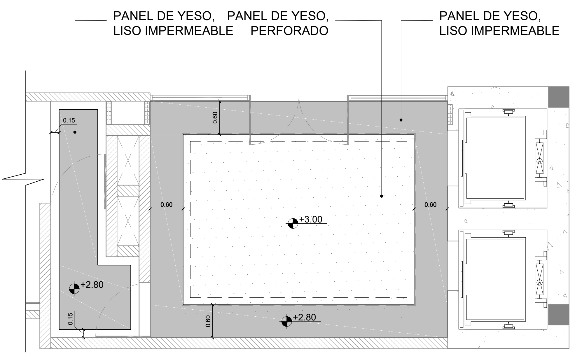
2 Detalle 1, Planta de Plafón, Nucleo B Esc. 1:40
