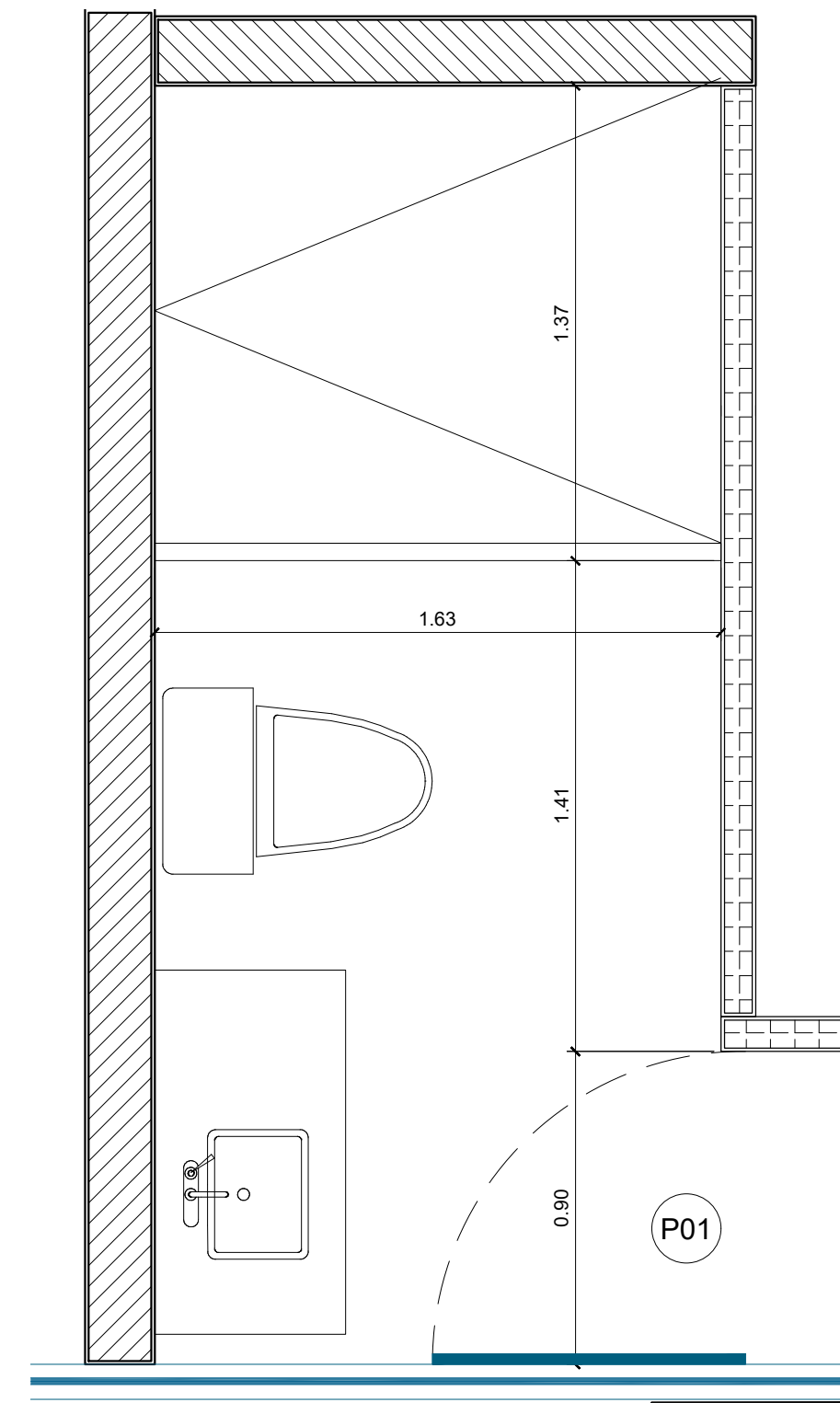
3 Planta Dimensionada - Baño Esc. 1: 20
