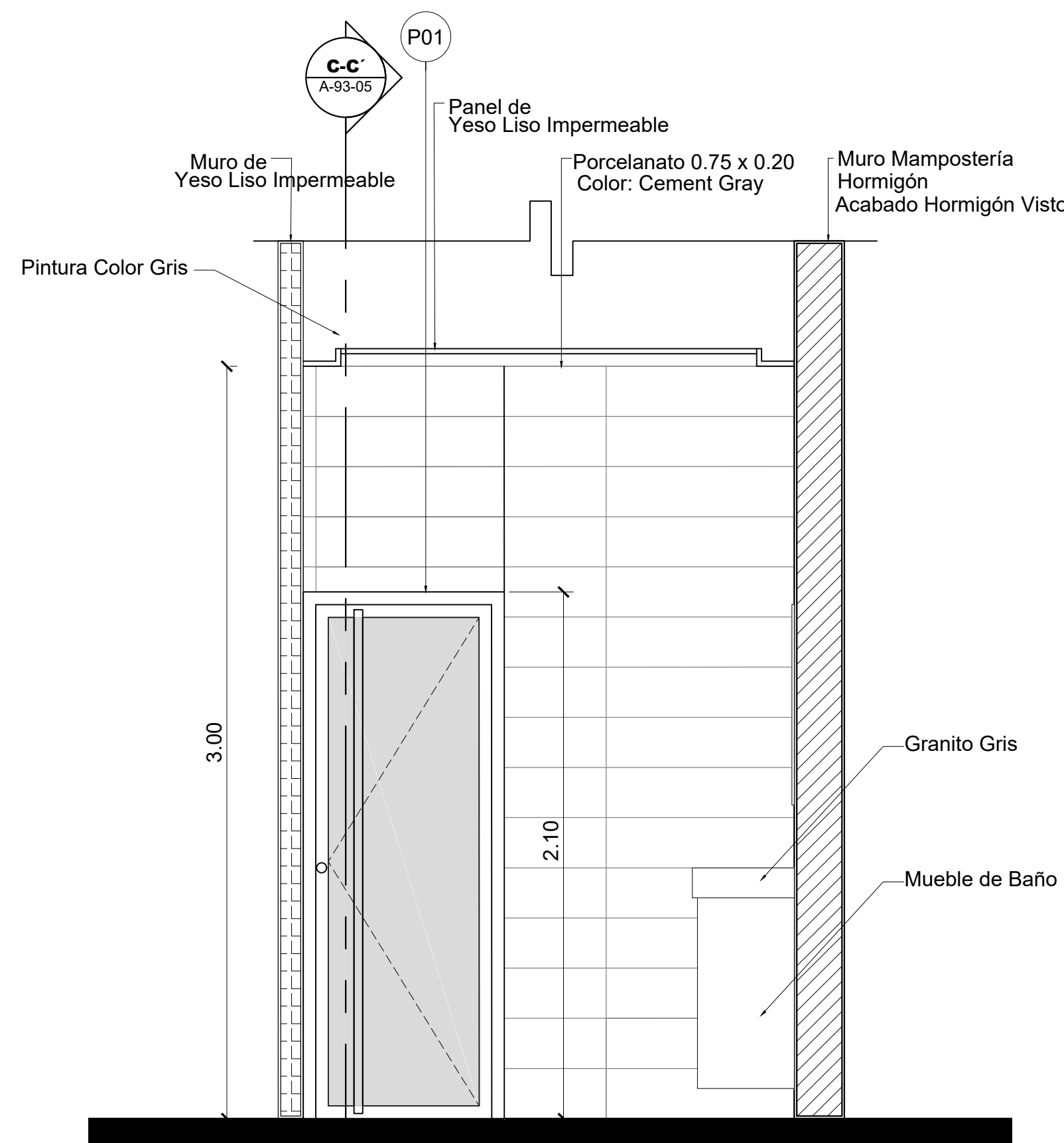
4 Sección B-B' Esc. 1: 20
