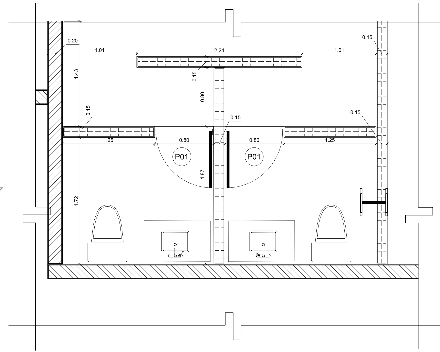
2 Planta Dimensionada - Baños Esc. 1: 25
