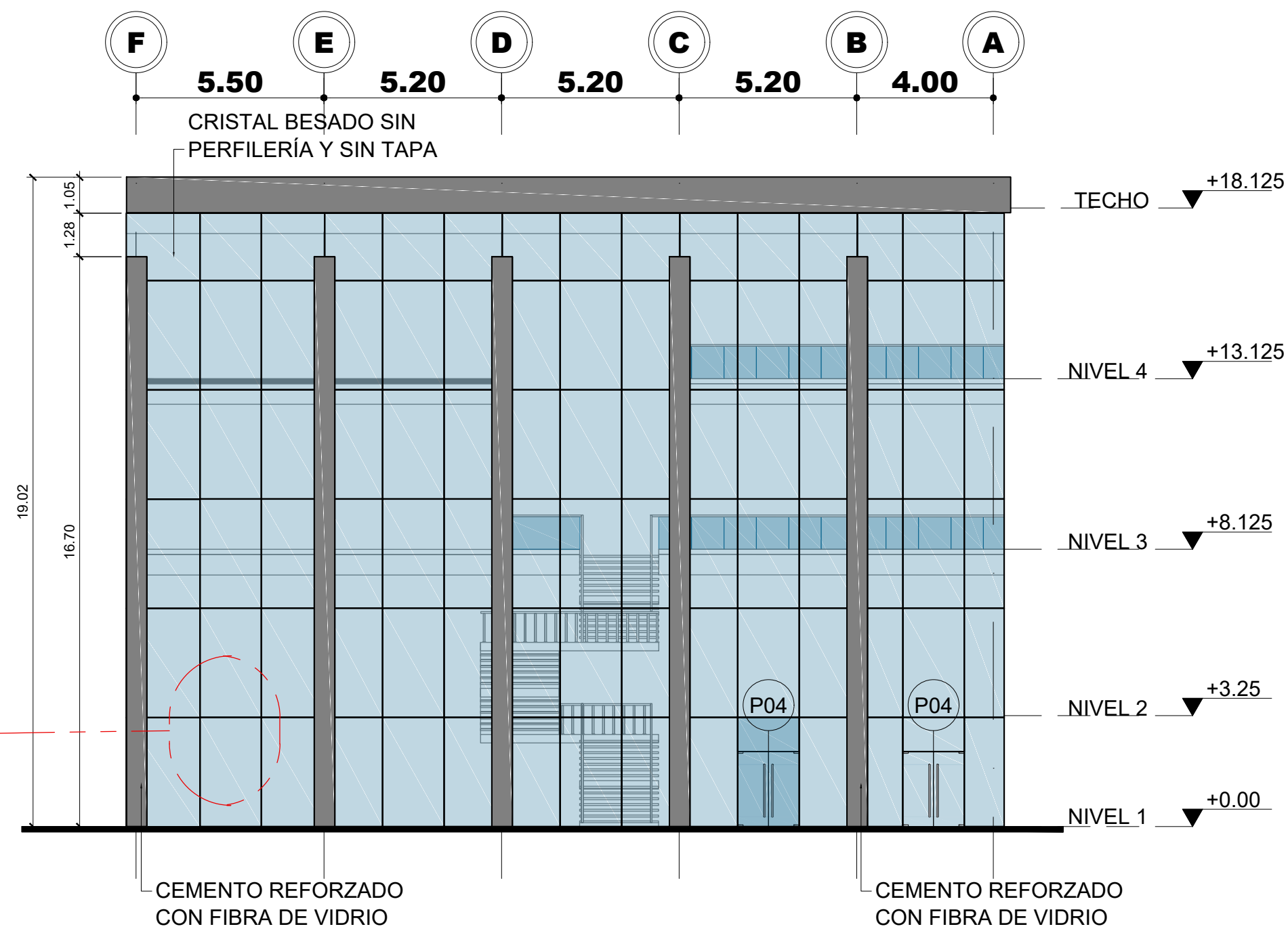
1 Elevación Frontal bloque 1 Esc. 1:150
