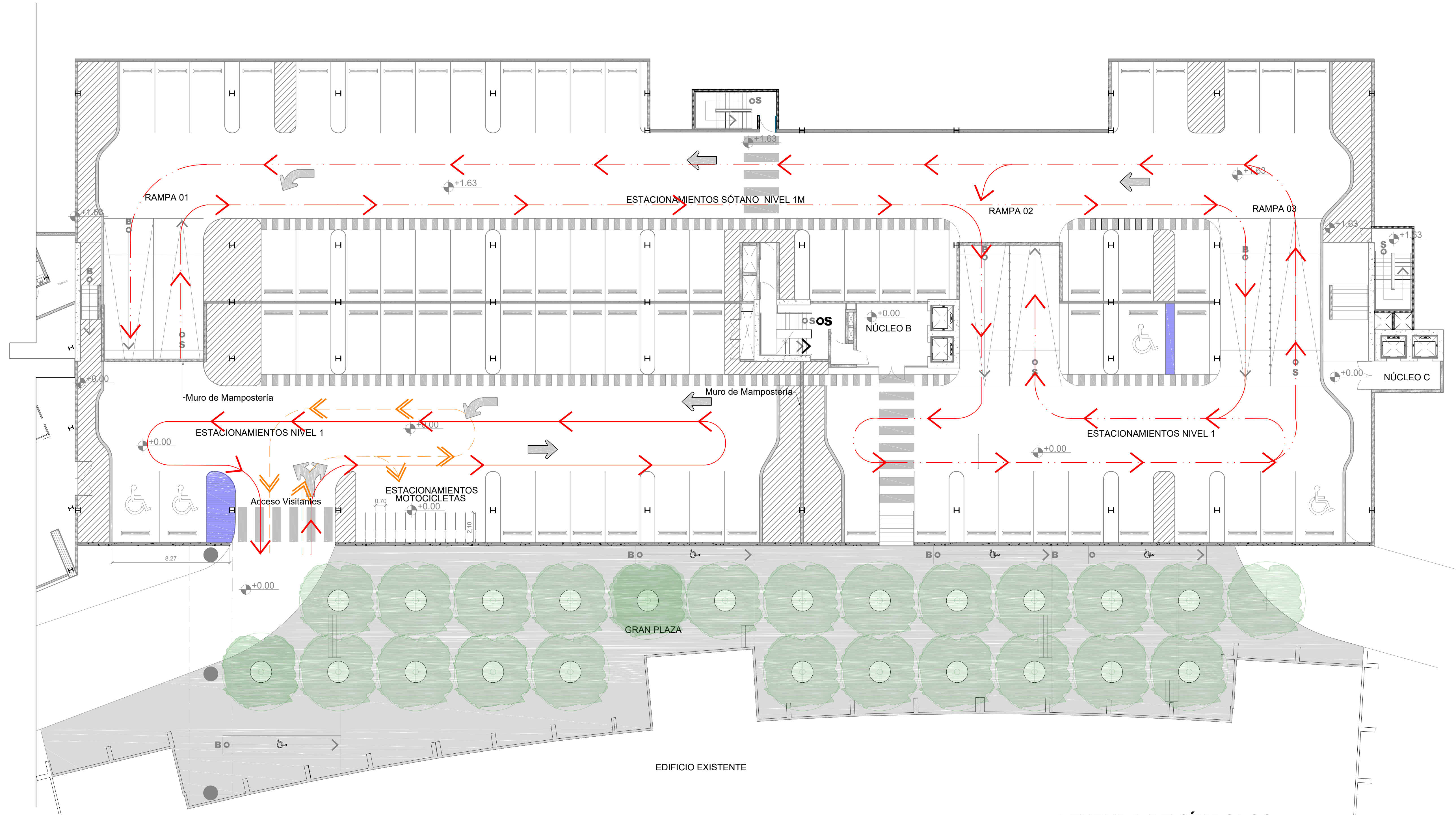
1 Planta de Accesos y Flujo Vehicular - Nivel 1 Esc. 1:150
