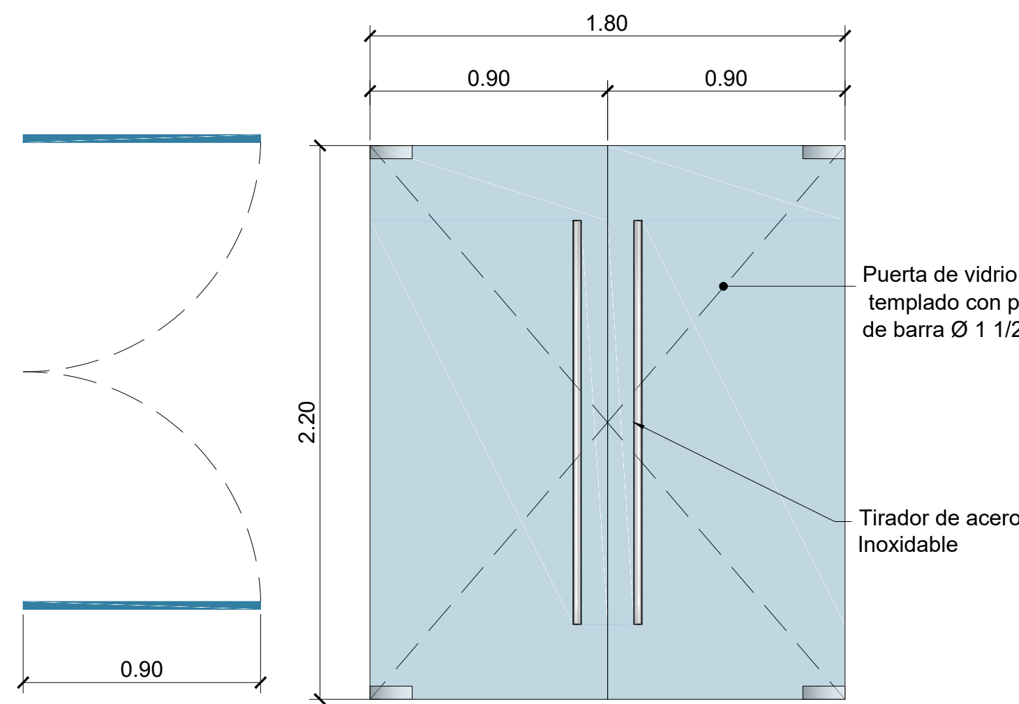
5 Puerta P04 ESCALA 1:20
