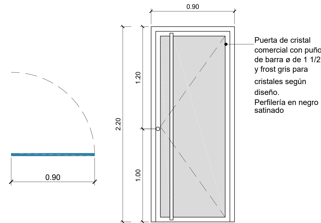
1 Puerta P01 ESCALA 1:20
