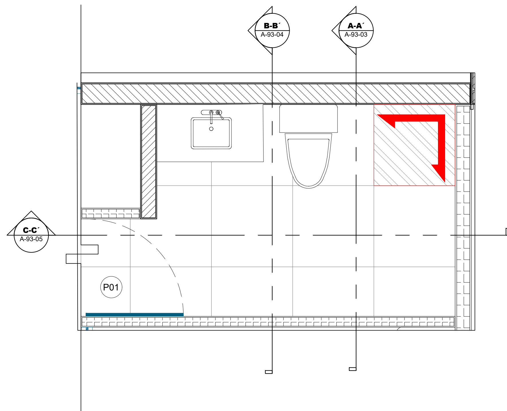
1 Planta Amueblada - Baños Esc. 1: 20
