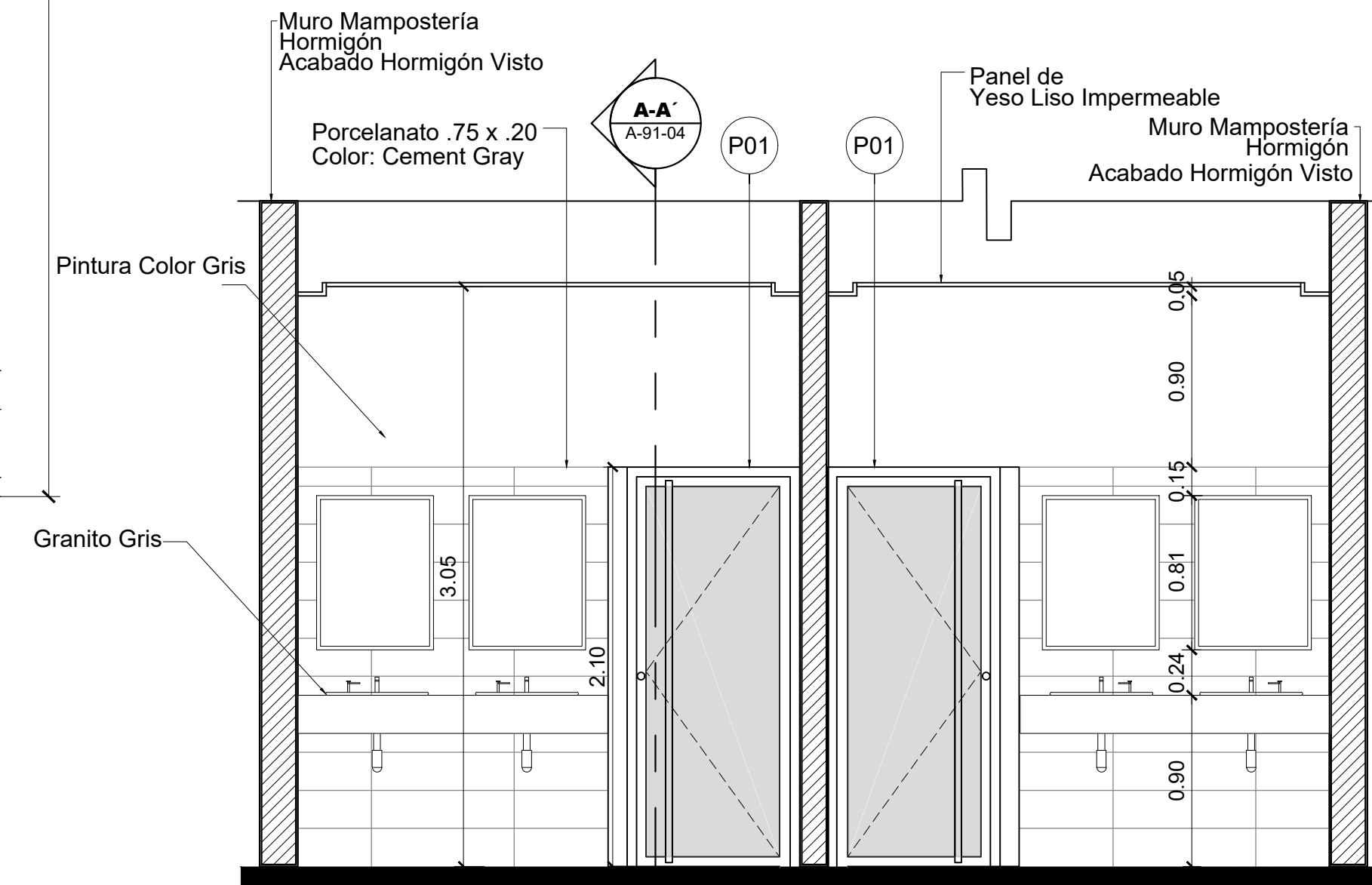
6 Sección C-C' Esc. 1: 30
