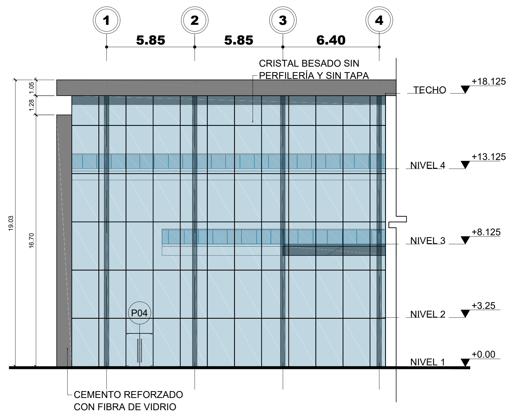
2 Elevación Lateral Derecha bloque 1 Esc. 1:150
