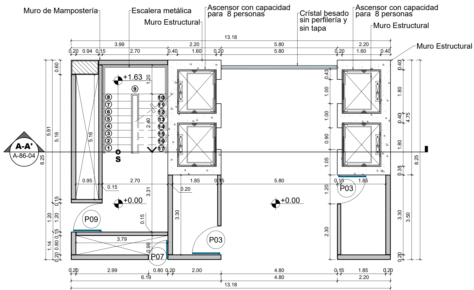
1 Planta Núcleo A - N1 a N2 Esc. 1:75
