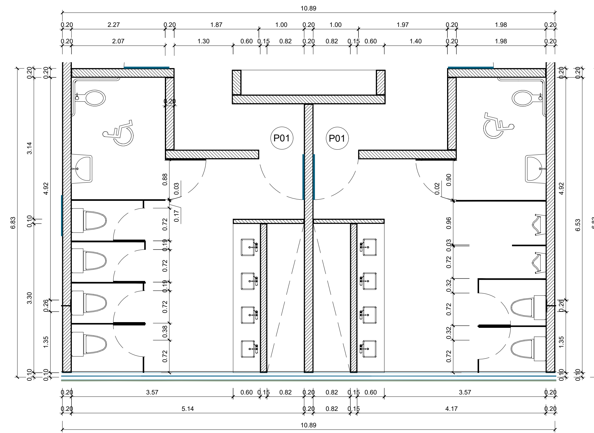
2 Planta Dimensionada - Baños Esc. 1: 50
