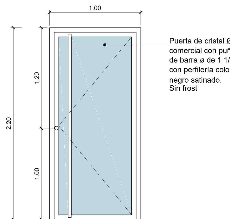
4 Puerta P10 ESCALA 1:30
