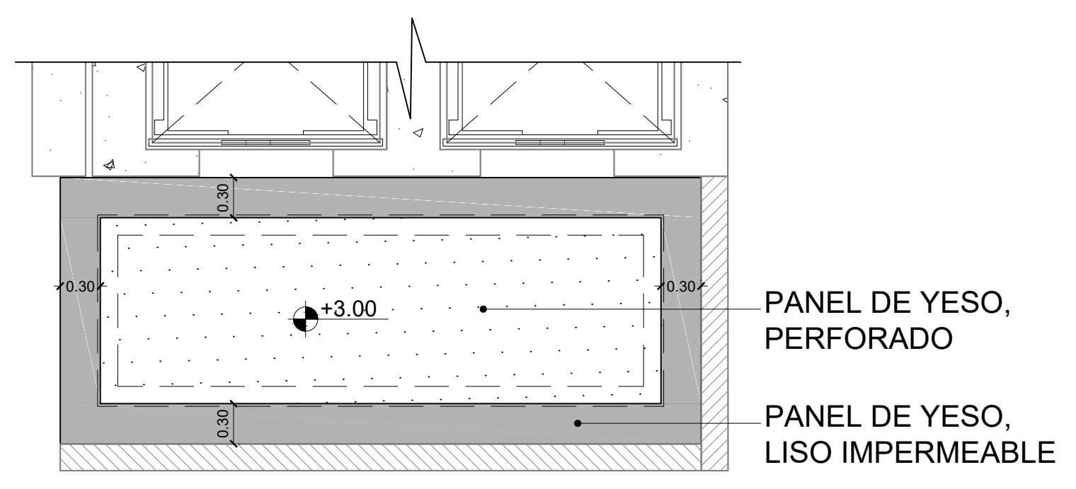
3 Detalle 1, Planta de Plafón, Nucleo C Esc. 1:40
