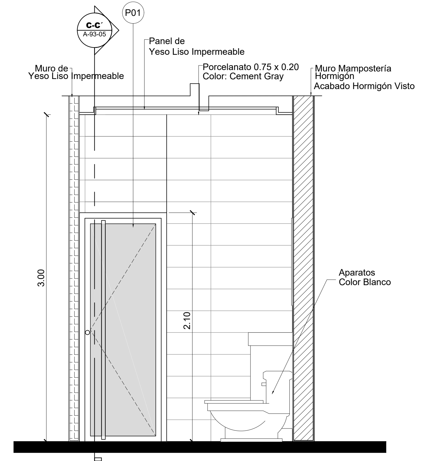
3 Sección A-A' Esc. 1: 20
