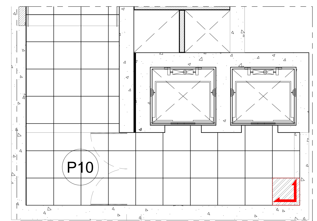
3 Detalle B Esc. 1:50
