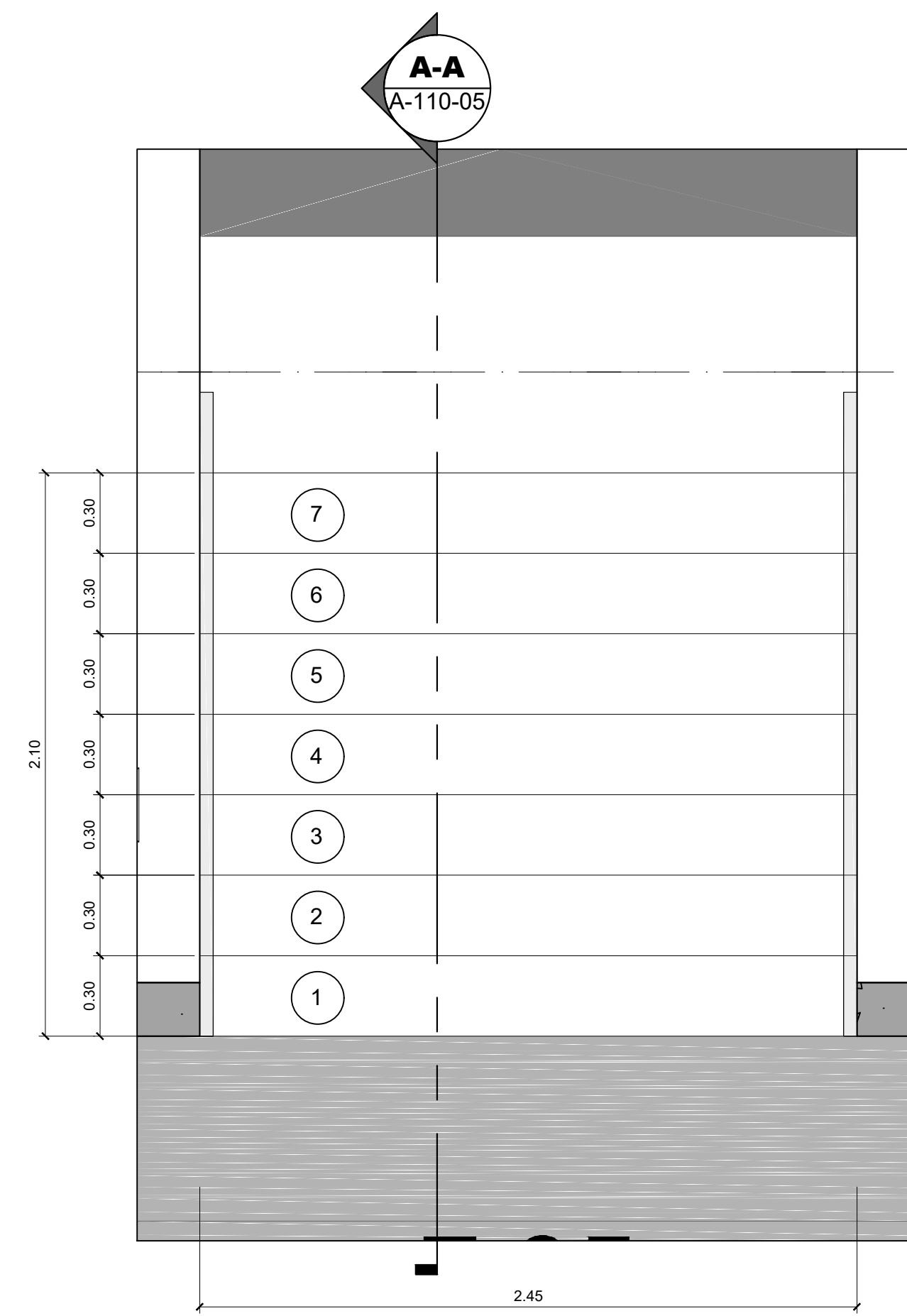
4 Planta Escalera Gran Plaza - N1 Esc. 1:20
