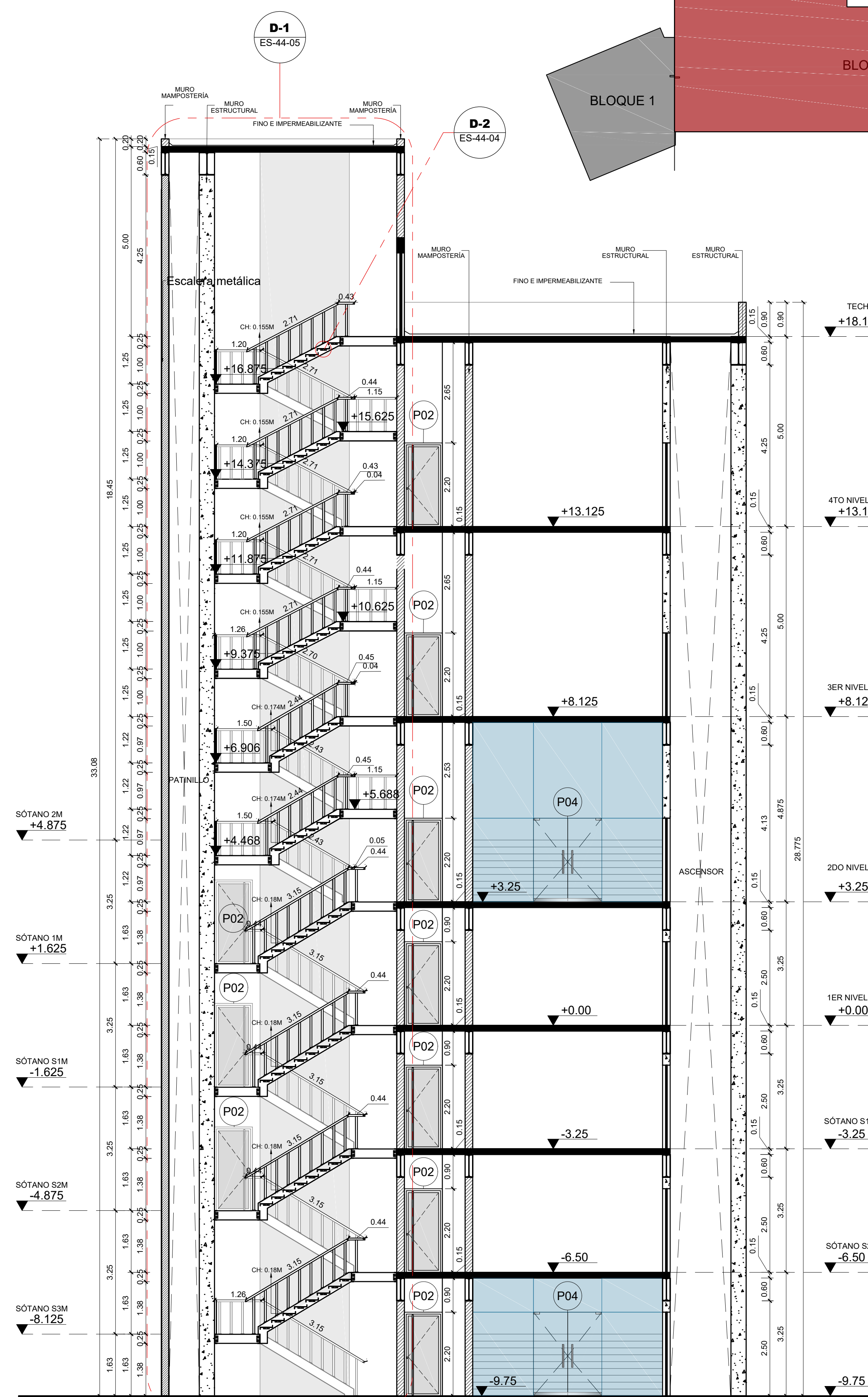
5 Sección A-A' Núcleo B - Sótano 3 a Techo Esc. 1:75
