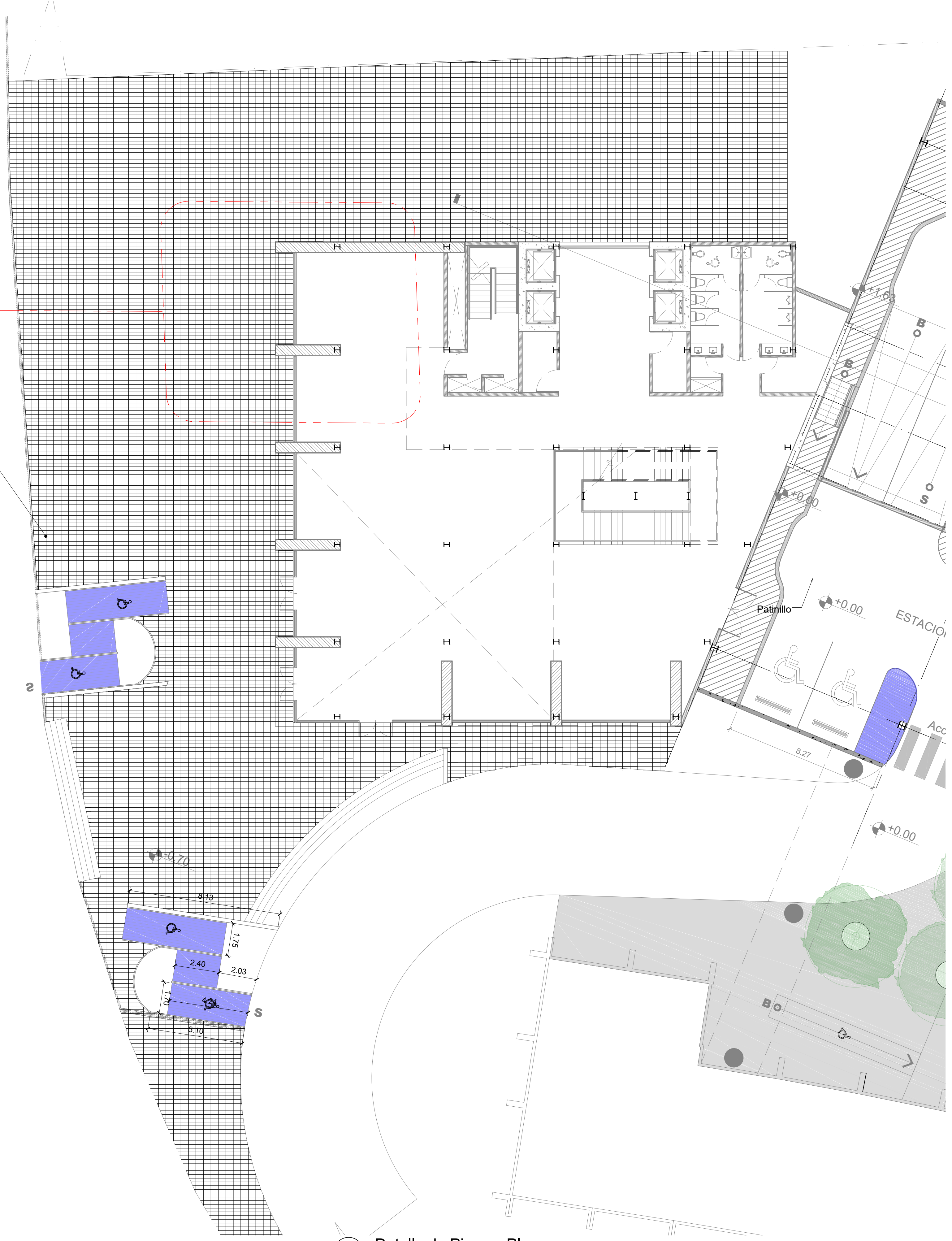
1 Detalle de Piso en Plaza Esc. 1:125
