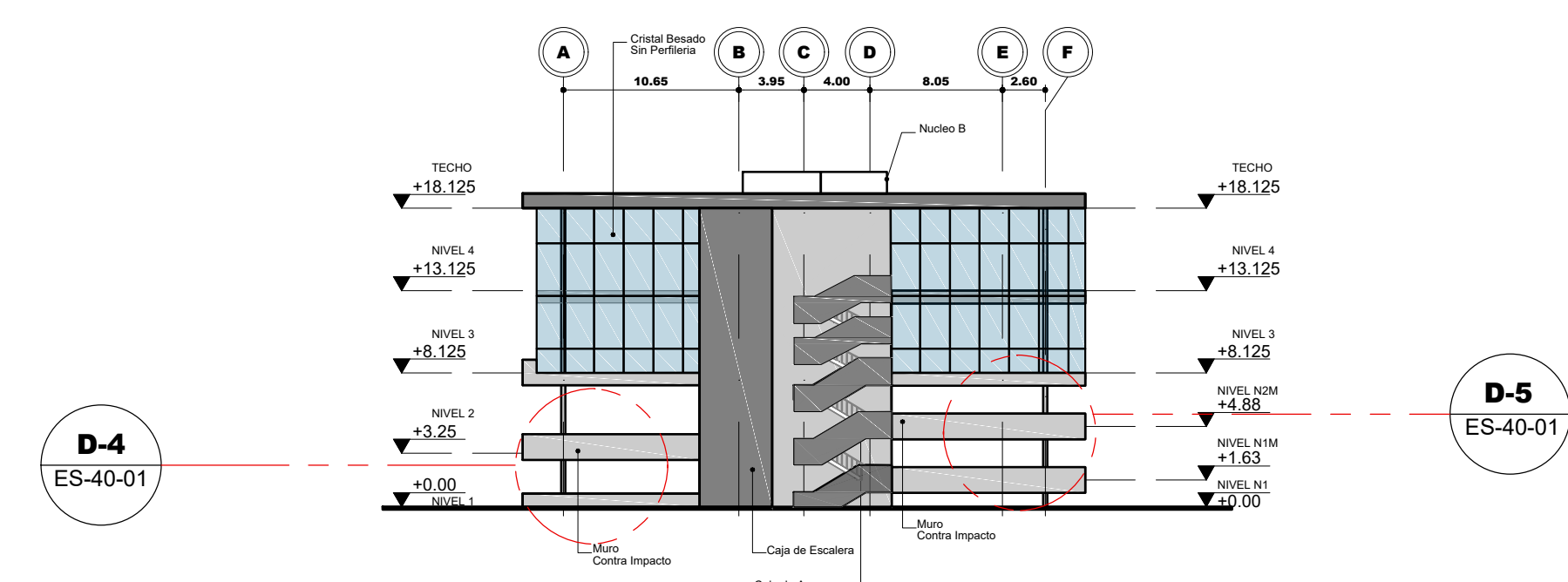
3 Elevación lateral Derecha bloque 2 Esc. 1:250
