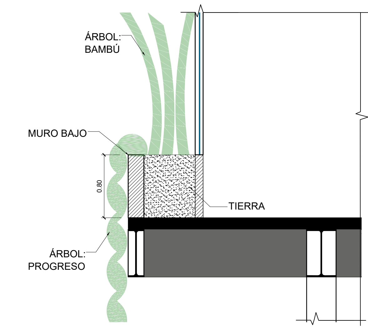
2 Detalle 1 Esc. 1:30
