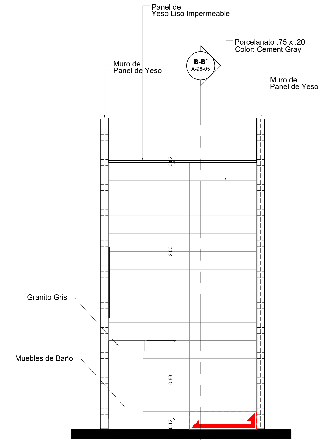
6 Sección C-C' Esc. 1: 20
