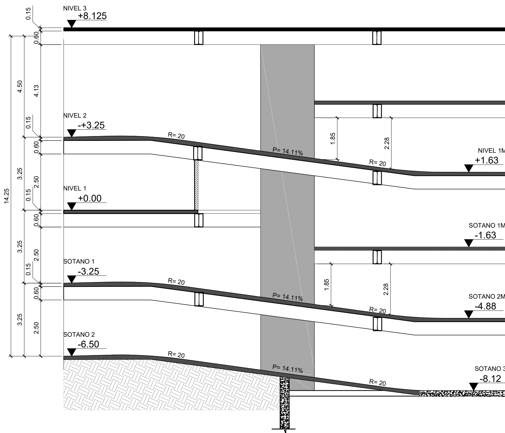
1 Sección de Detalle Rampa 1 - Bloque 2 Esc. 1:100
