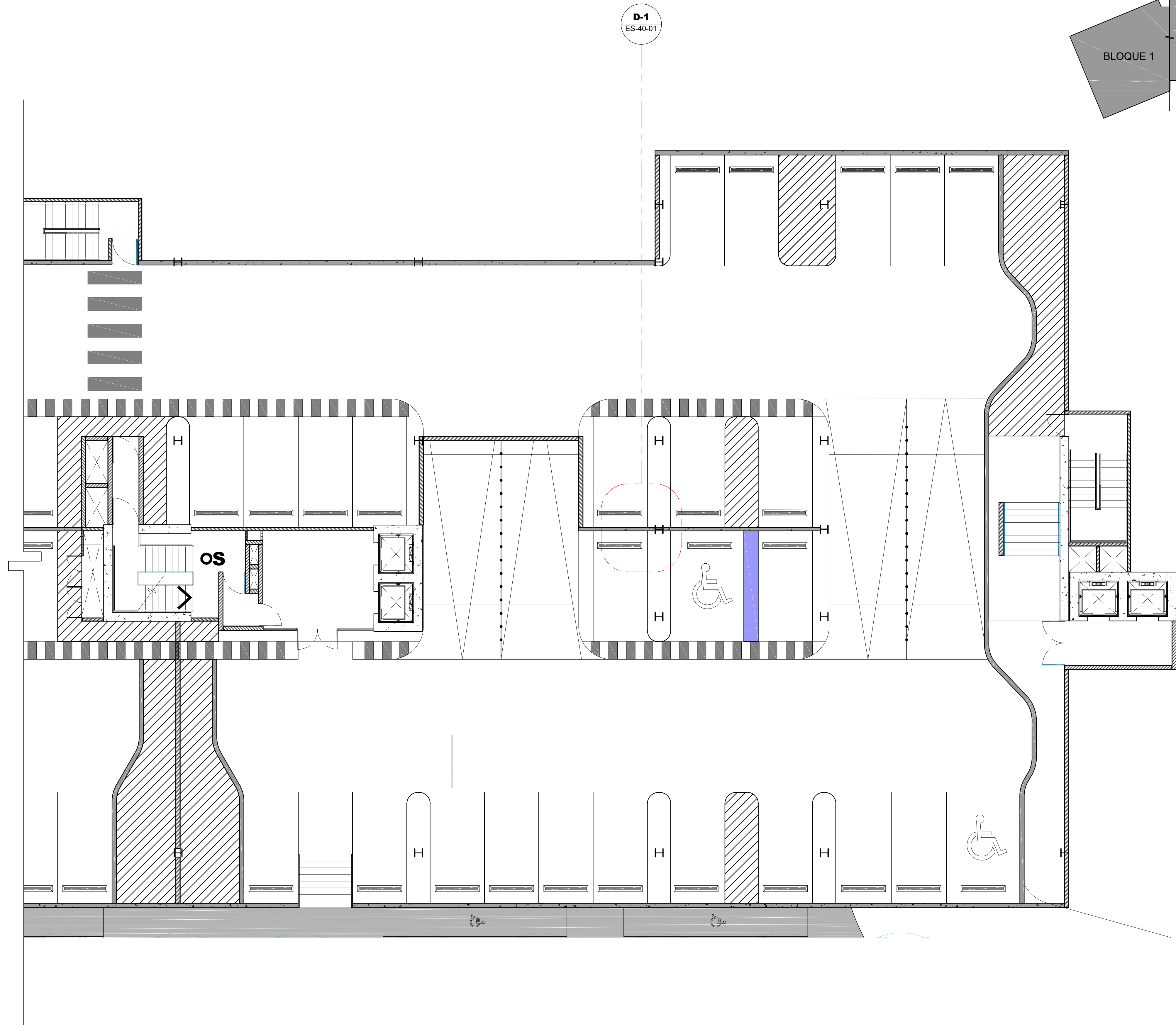
1 Planta Muros Bloque 2B - Nivel 1 Esc. 1:100
