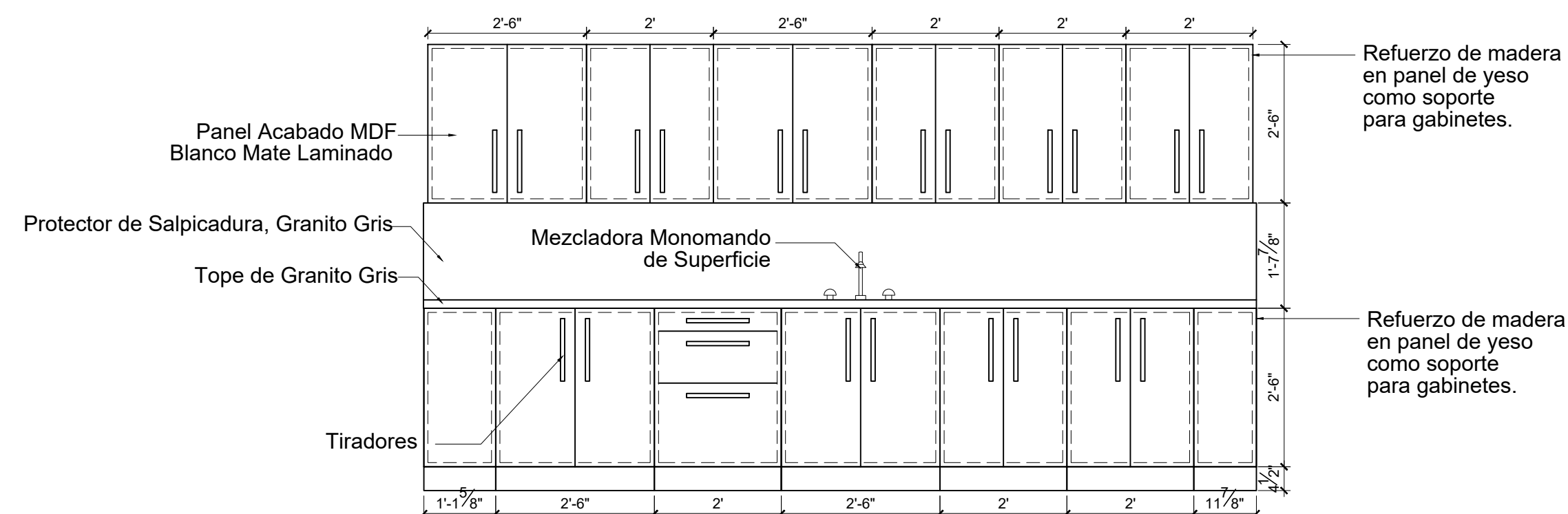
1 Detalle Cocineta Cafeteria - Bloque 2 - N3 Esc. 1:25
