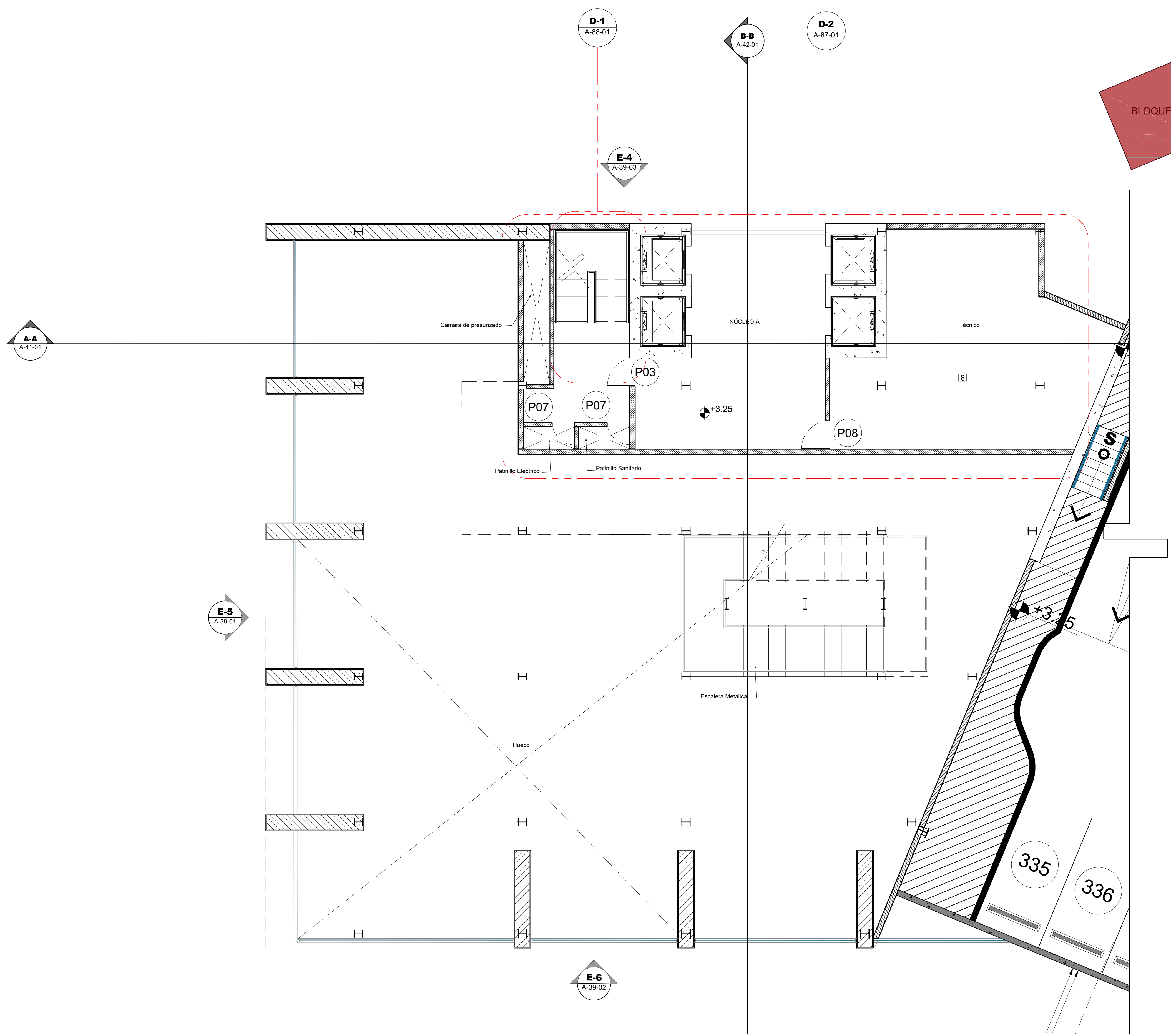
1 Planta Amueblada Nivel 2 - Bloque 1 Esc. 1:75
