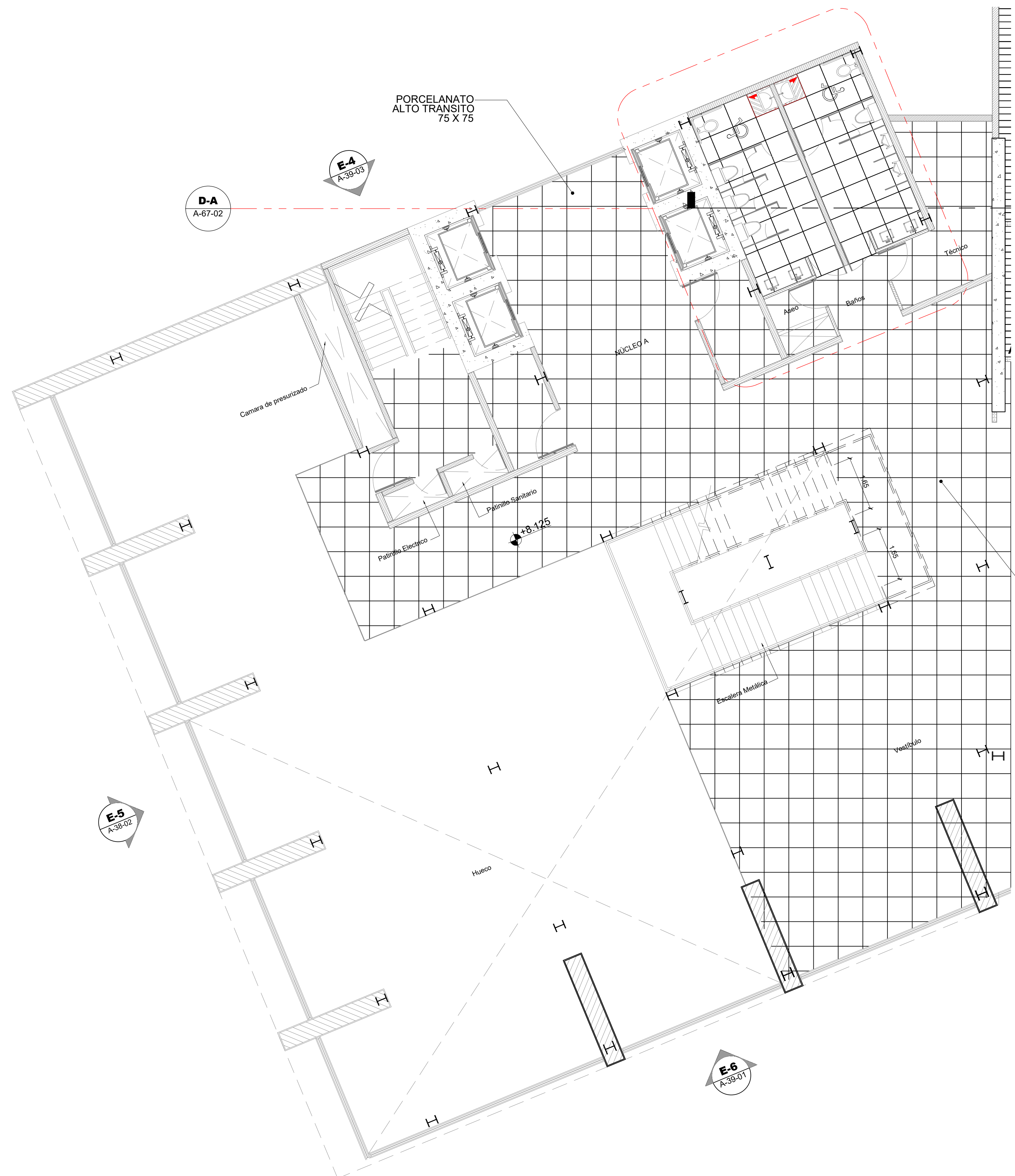
1 Planta Pisos - Bloque 1 - Nivel 3 Esc. 1:75
