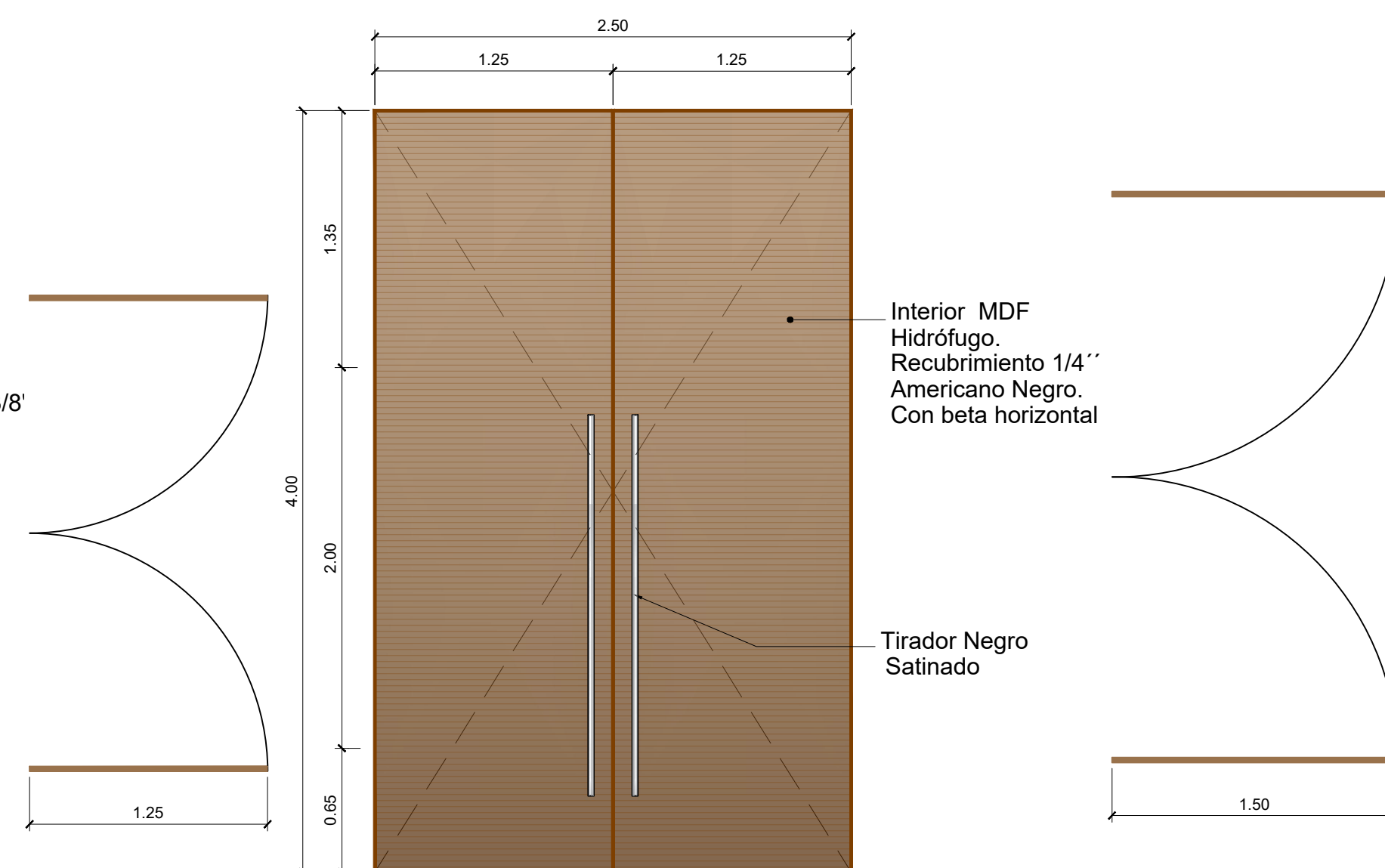
6 Puerta P05 ESCALA 1:30
