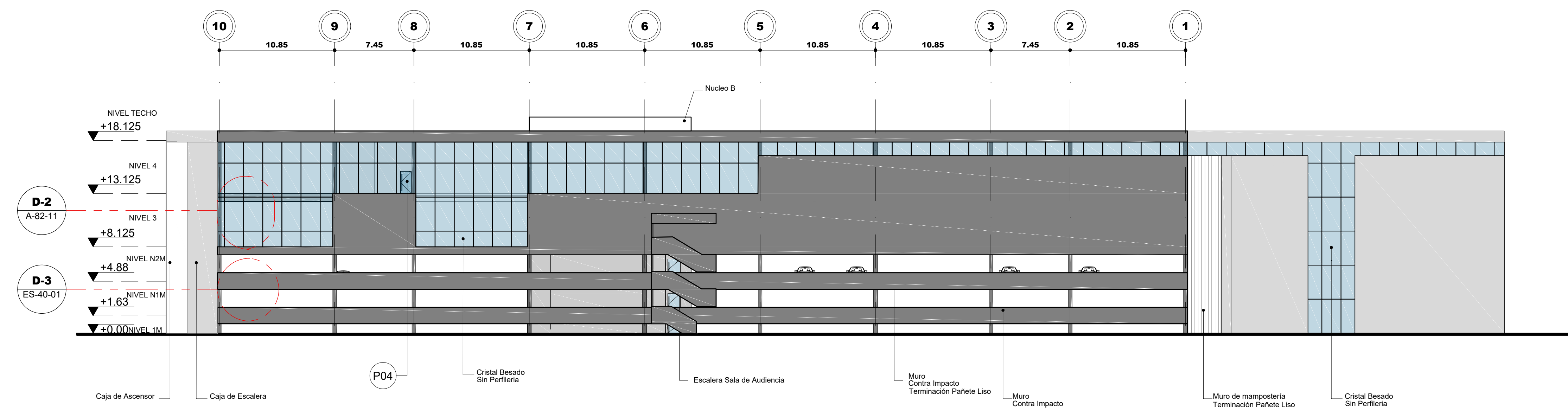
2 Elevación Posterior bloque 2 Esc. 1:250
