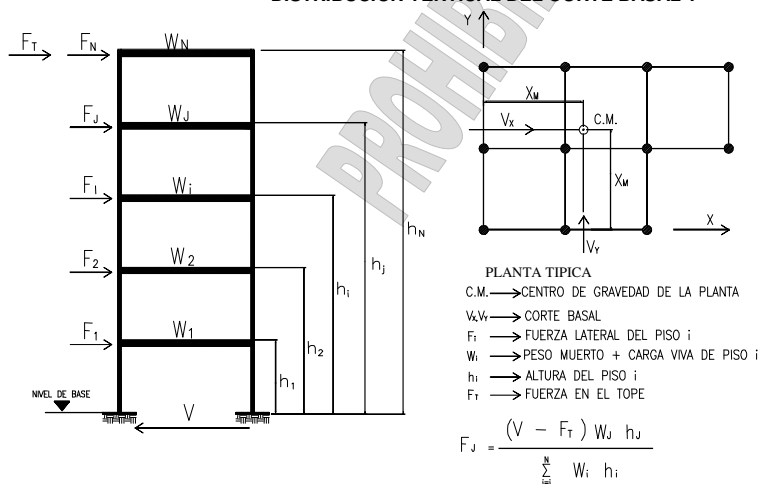
FIGURA 4 DISTRIBUCIÓN VERTICAL DEL CORTE BASAL V
