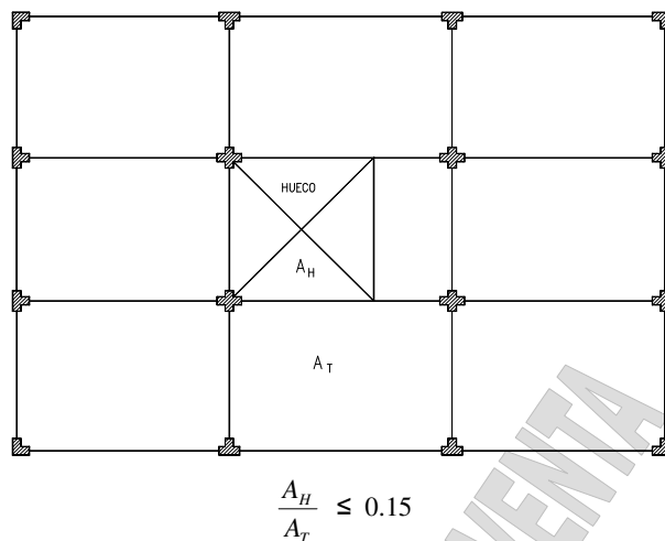
FIGURA 8 EJEMPLO DISCONTINUIDAD EN LOSAS
