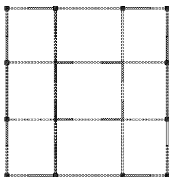
SISTEMA ESTRUCTURAL RECOMENDADO
