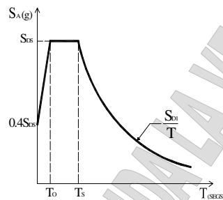
GRÁFICA 1 ESPECTRO SÍSMICO LINEAL ELÁSTICO
