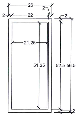
Elevación Frontal Dimensionada
