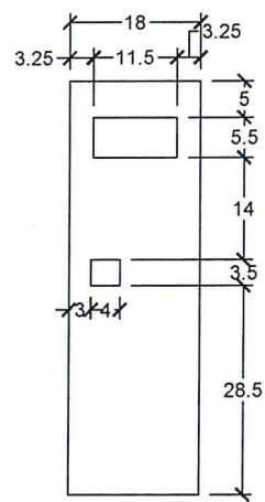
Elevación Lateral Dimensionada
