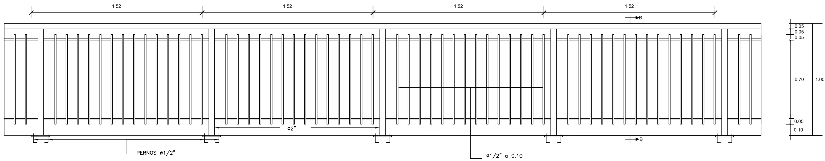
DETALLE BARANDILLA ESC. 1:20
