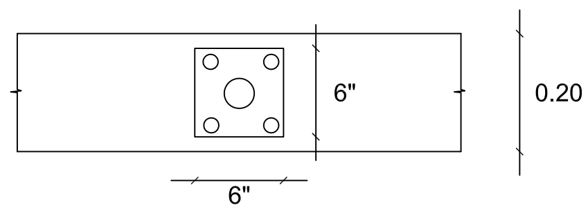
DETALLE ANCLAJE PLACA ESC. 1:10
