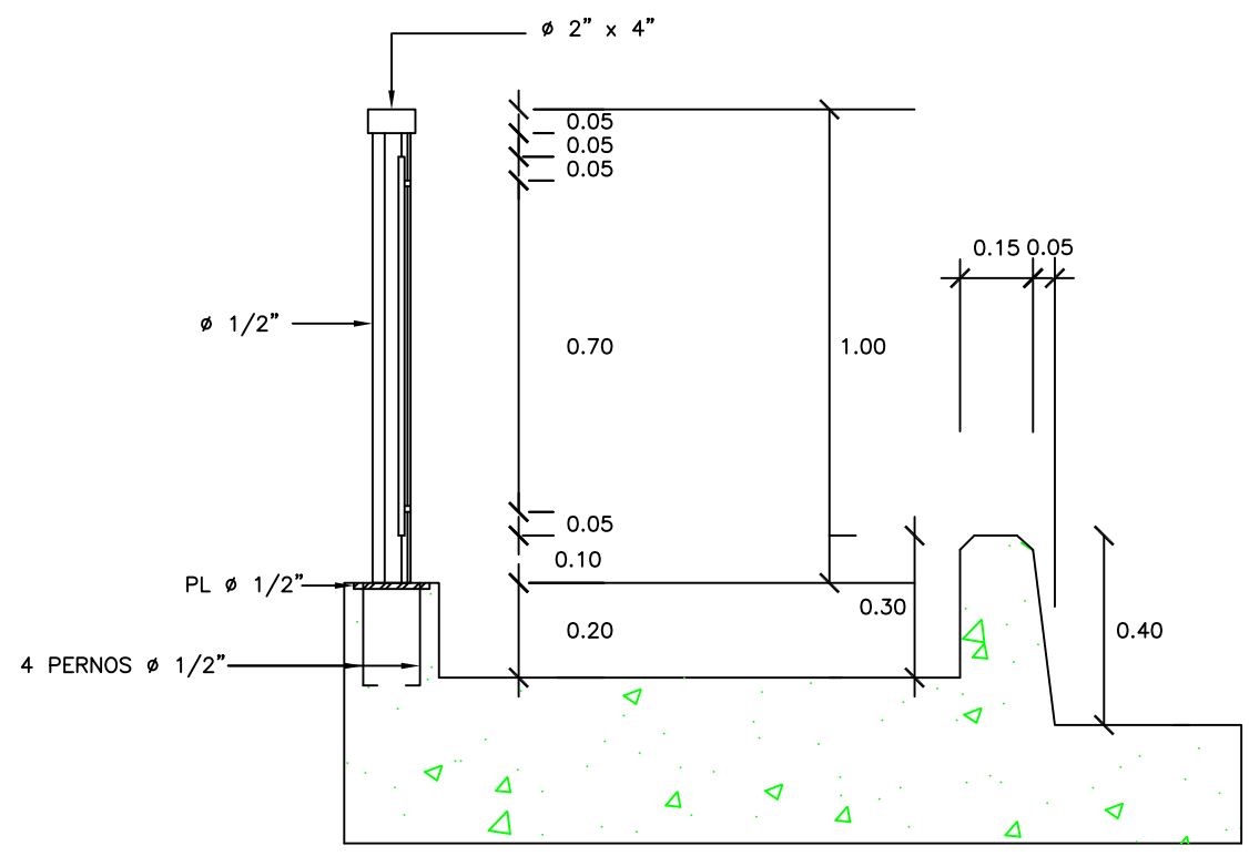
DIMENSIONES BARANDILLAS
