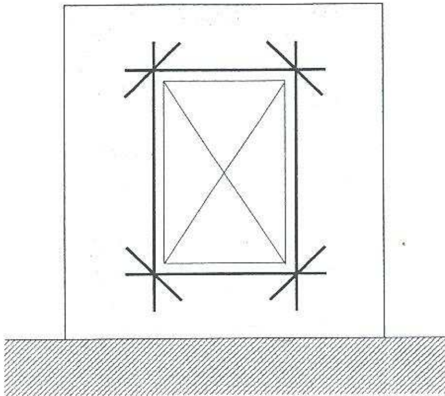
Figura 3.23 – Acero para contramarcos convencional
