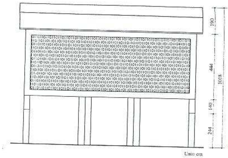
Figura G3 Elevación frontal
