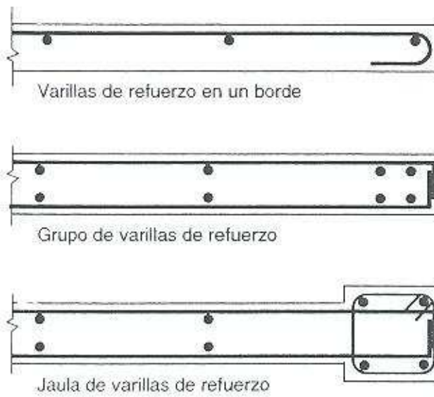
Figura 3.22 – Elementos ubicados en los límites
