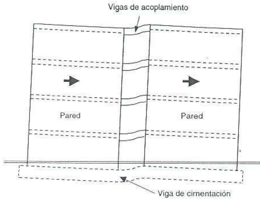
Figura 3.21- Paredes acopladas
