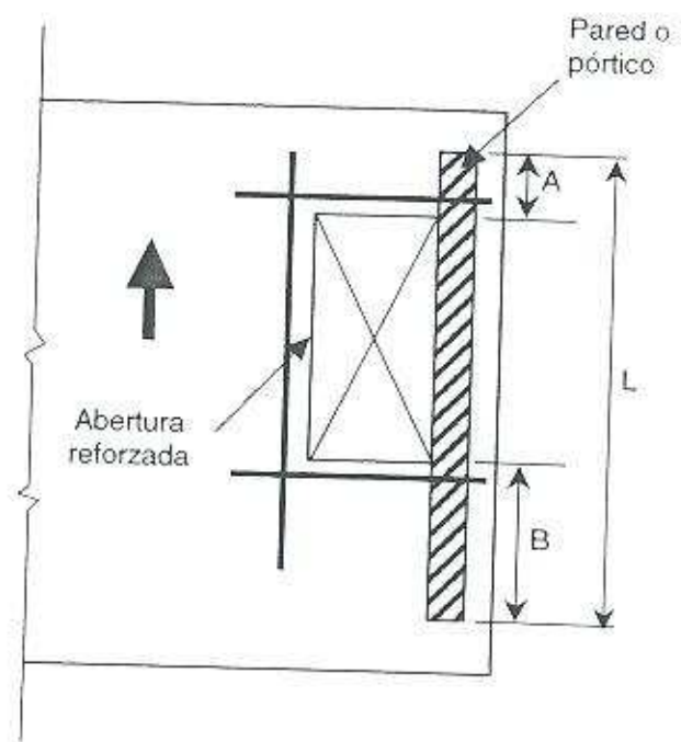
Figura 3.20 – Abertura de diafragma en una pared exterior
