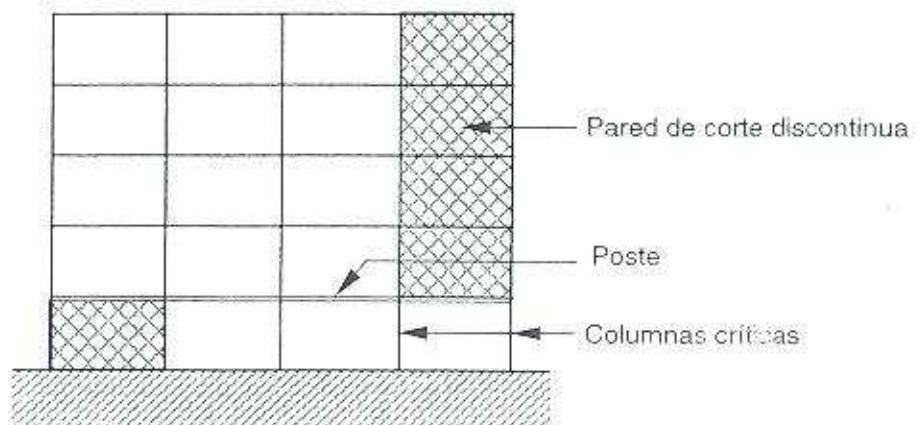
Figura 3.7- Discontinuidad vertical en el plano
