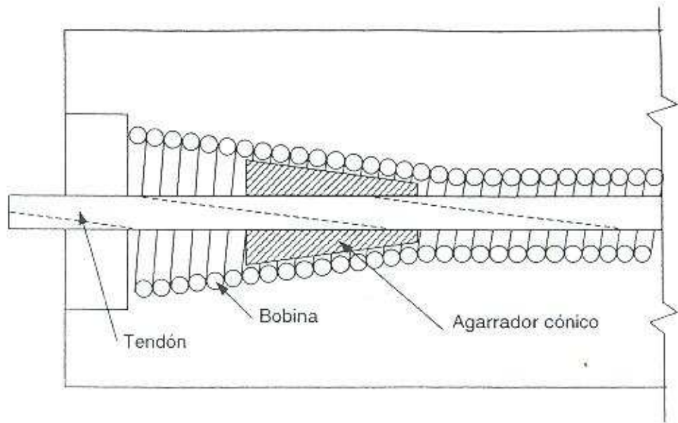
Figura 3.12 – Anclaje abobinado
