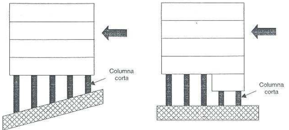
Figura 1.1 Columnas Cortas
