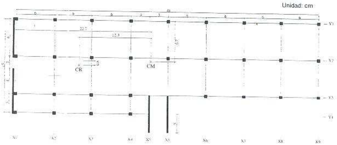
Figura G2 Ubicación del centro de masa y del centro de rigidez
