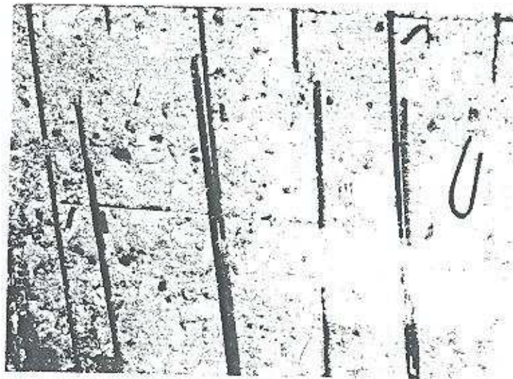
Parte inferior de la losa sin cubierta de hormigón. Refuerzo de acero expuesto
