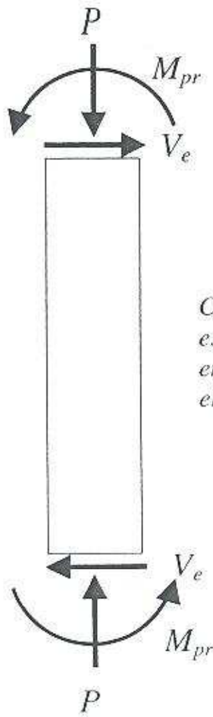
Figura 3.15 - M_{pr} y V_e
