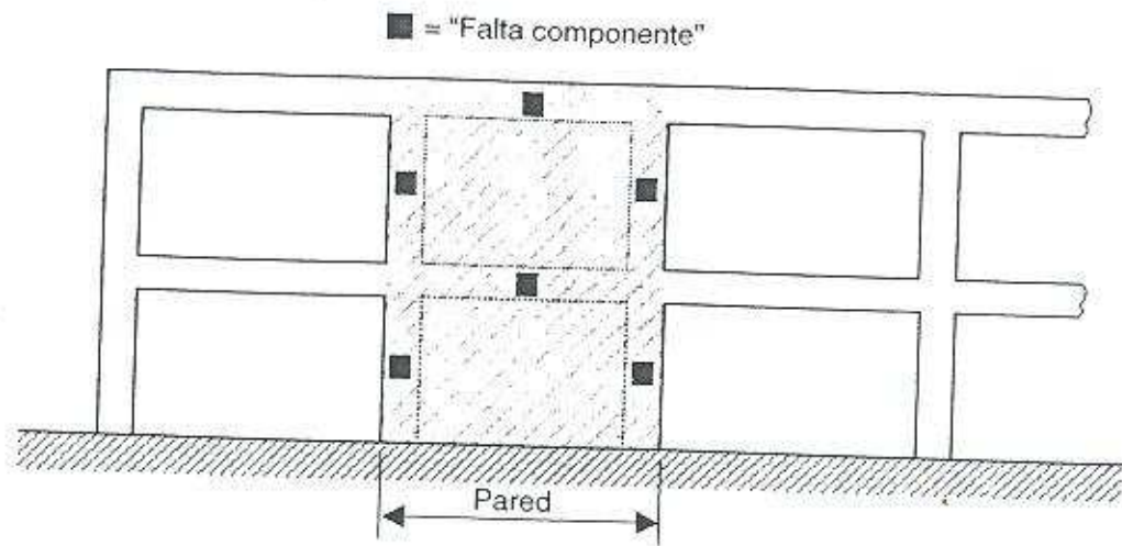
Figura 3.19 – Pórtico incompleto
