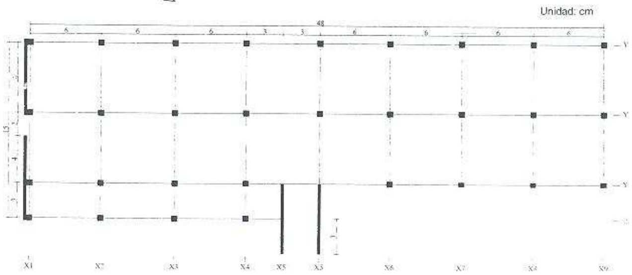
Figura G1 Planta y elevación de una ala del hospital
