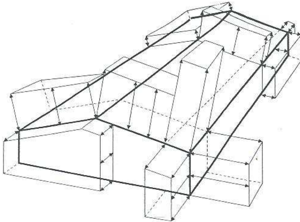
Figura 2.2— Distribución de presiones de viento localizadas
