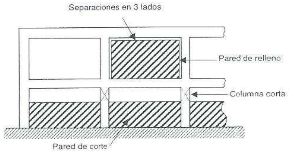
Figura 3.24 -Paredes de relleno
