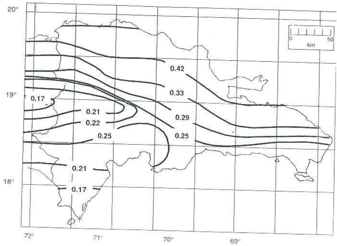
Figura 2.1 — Contornos de aceleración sísmica (Periodo de retorno de 50 años, 10 % probabilidad de ser excedida)
