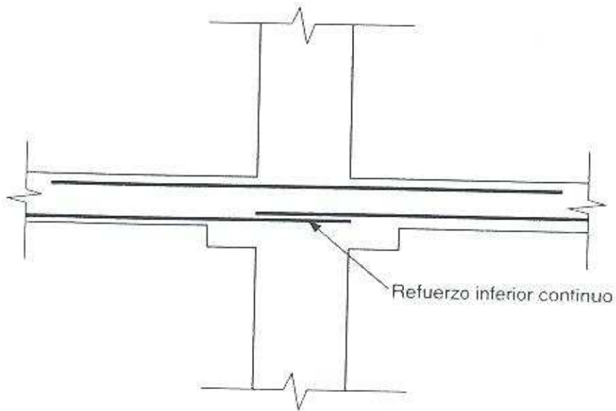
Figura 3.11 – Acero de refuerzo inferior continuo
