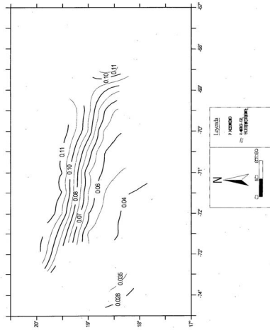
Mapa N°3. - Mapa de isoceleraciones espectrales S_1 para un 10% de Probabilidad de ser excedida en 5 años
