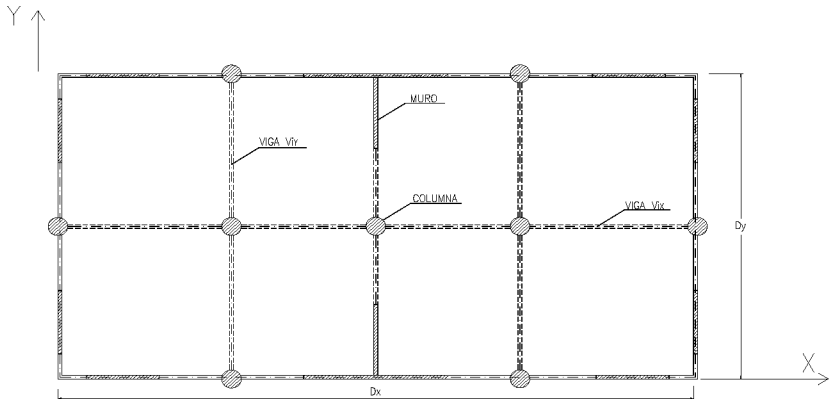
FIGURA 3 SISTEMA MIXTO (MUROS Y PÓRTICOS) SISTEMA DE MUROS ORTOGONALES (X,Y) (ESTRUCTURA SISTEMA 3)
