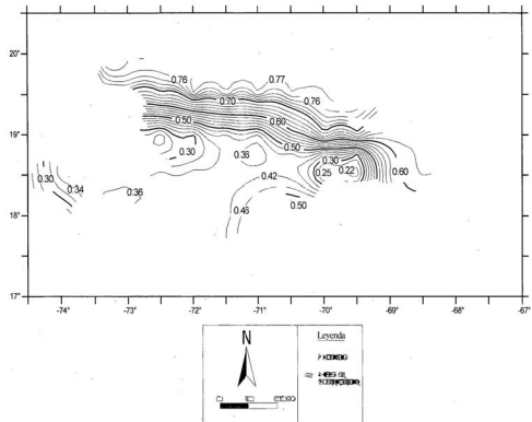
Mapa N°7. - Mapa de isoaceleraciones espectrales S_d para un 2% de Probabilidad de ser excedida en 50 años
