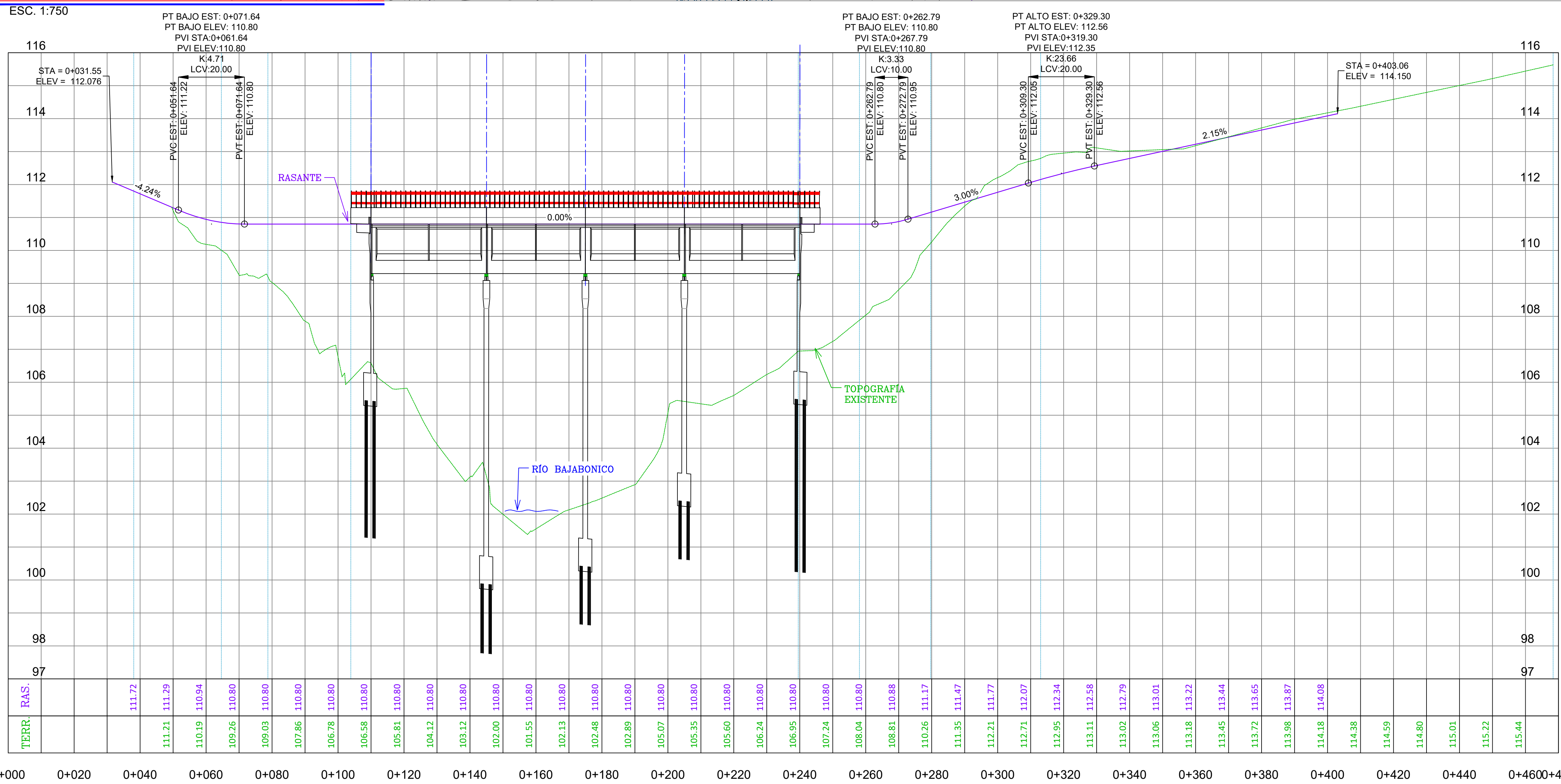
2 PERFIL LONGITUDINAL PUENTE BAJABONICO
