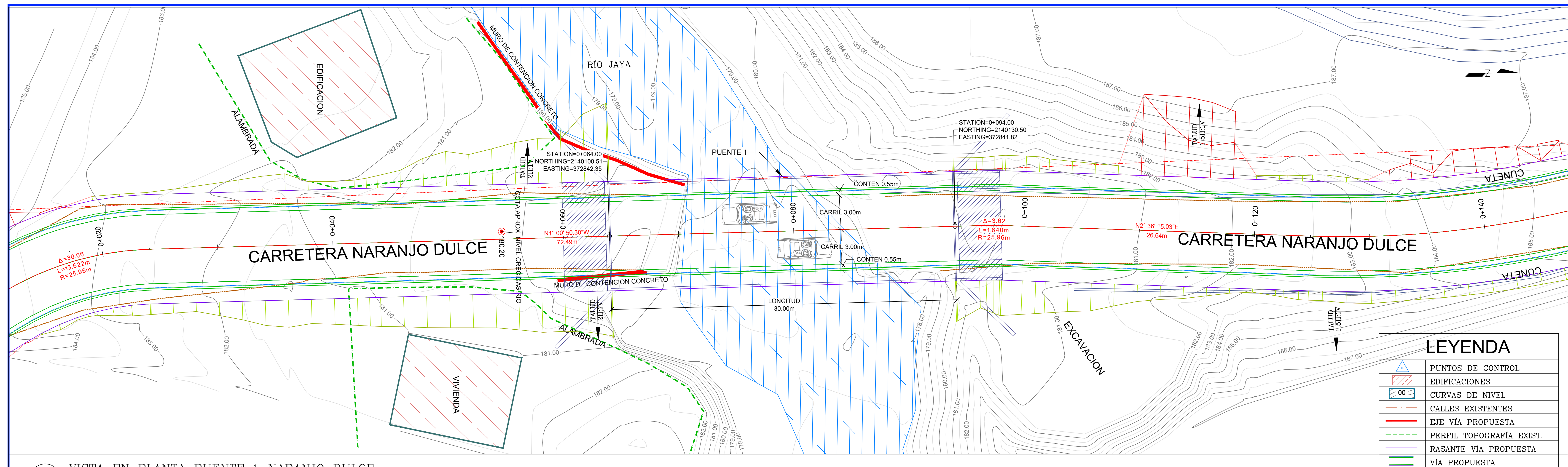
1 VISTA EN PLANTA PUENTE 1 NARANJO DULCE ESC. 1:150
