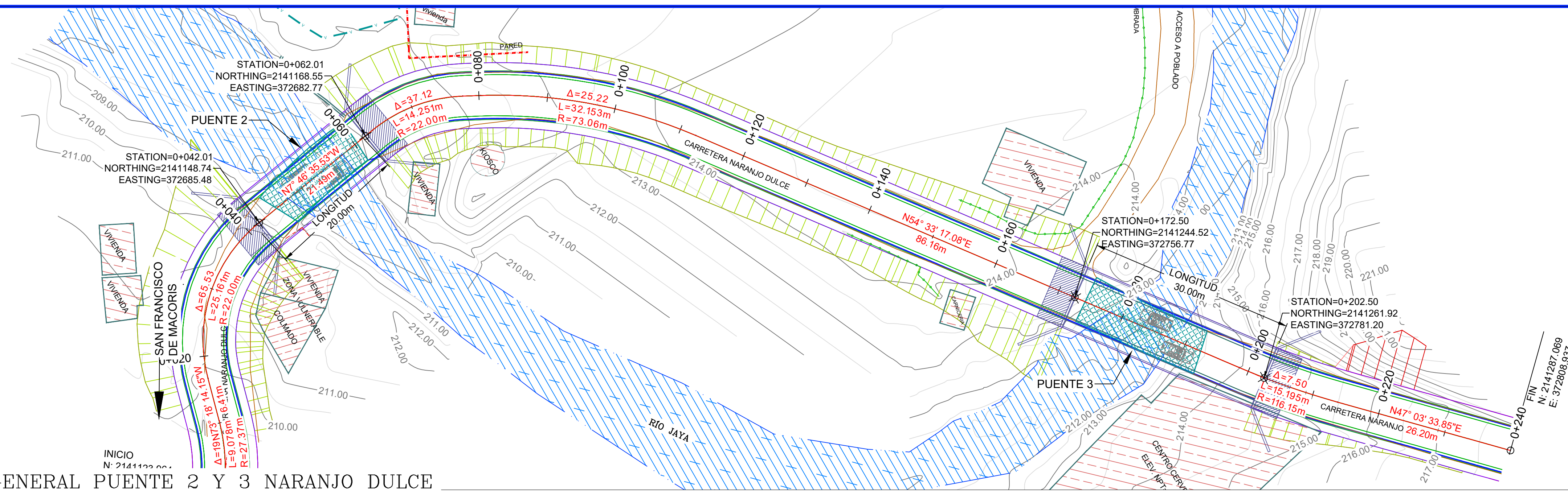
1 VISTA EN PLANTA GENERAL PUENTE 2 Y 3 NARANJO DULCE ESC. 1:400
