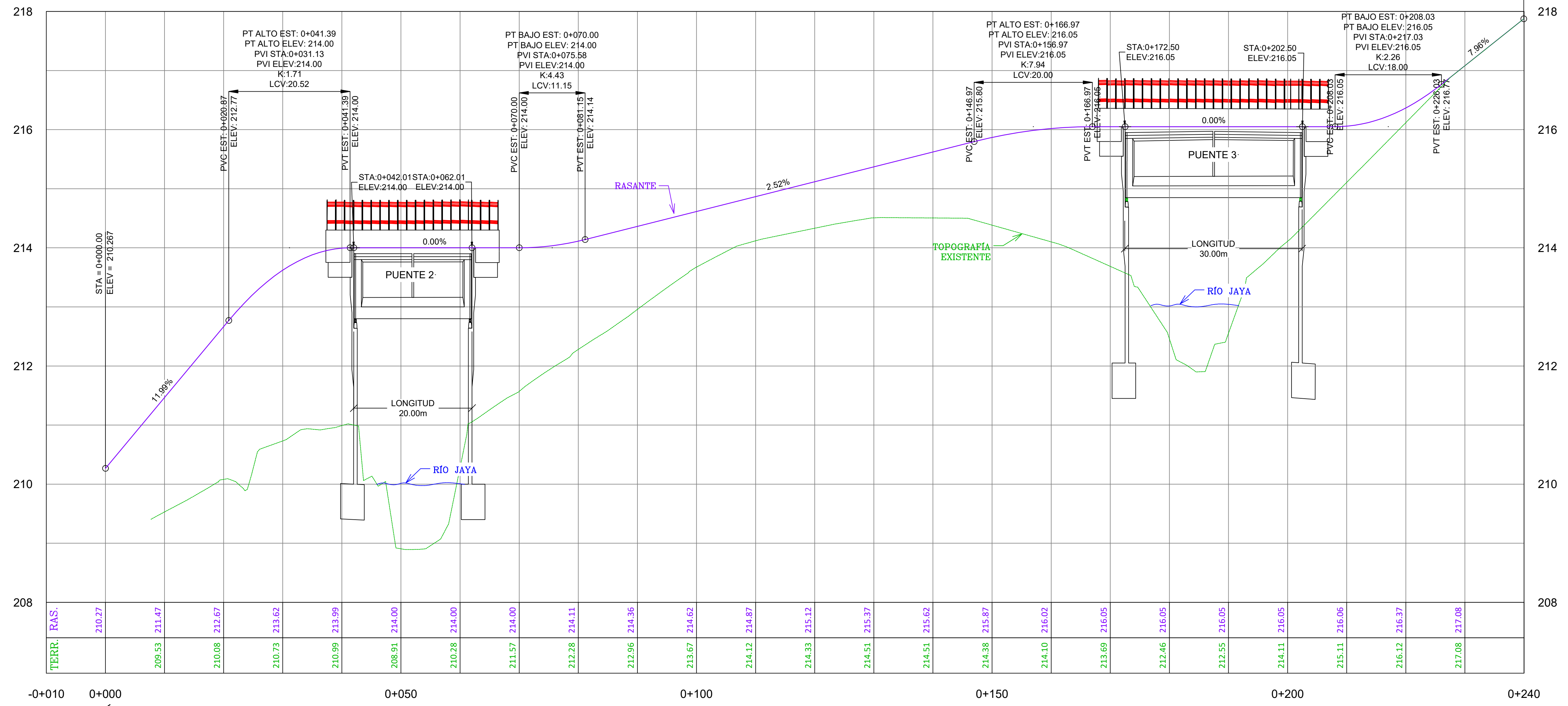
2 PERFIL LONGITUDINAL VIA DE ACCESO NARANJO DULCE ESC. H1:400 : V1:40
