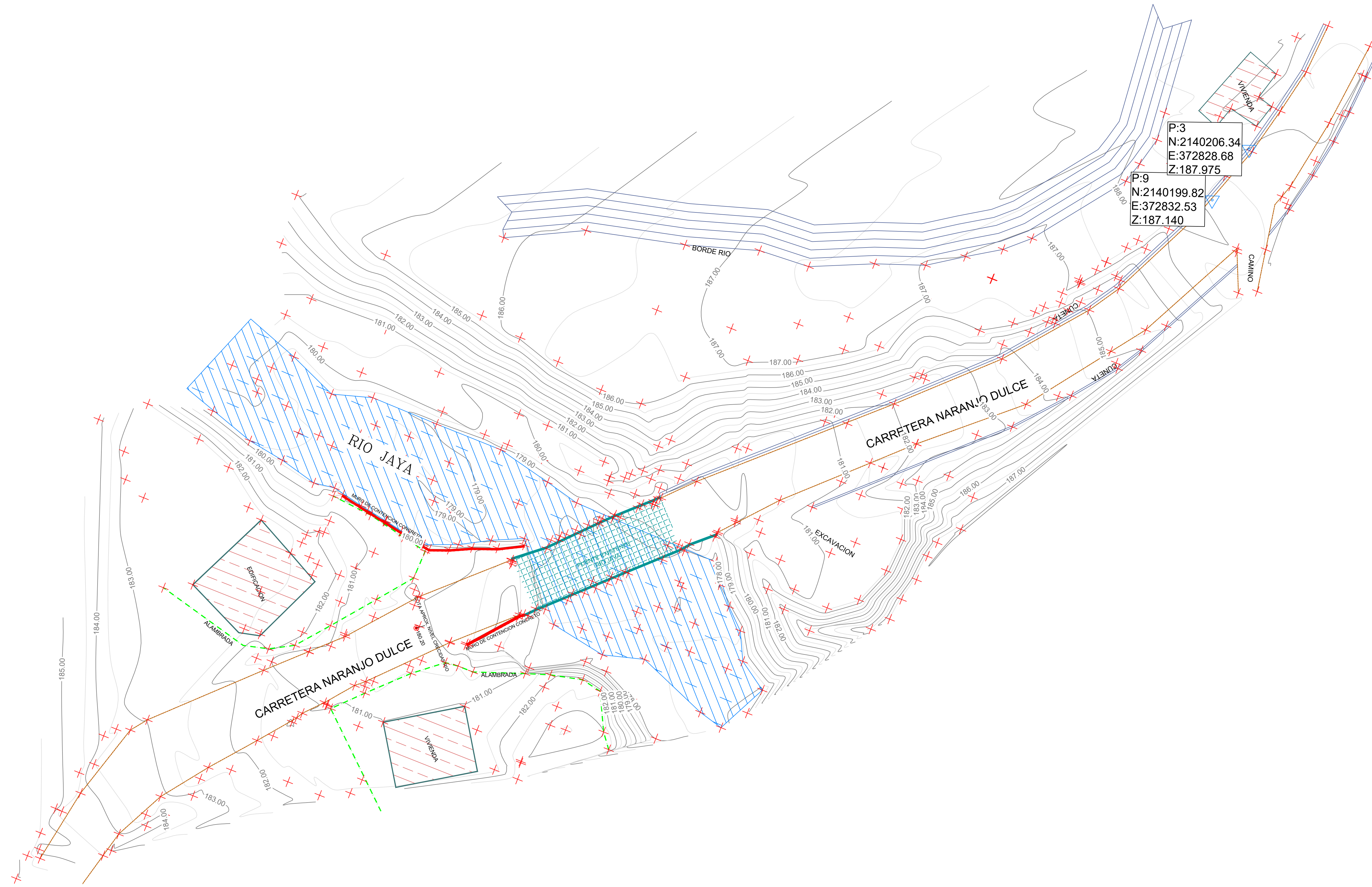
1 VISTA EN PLANTA TOPOGRAFÍA EXISTENTE ESC. 1:250
