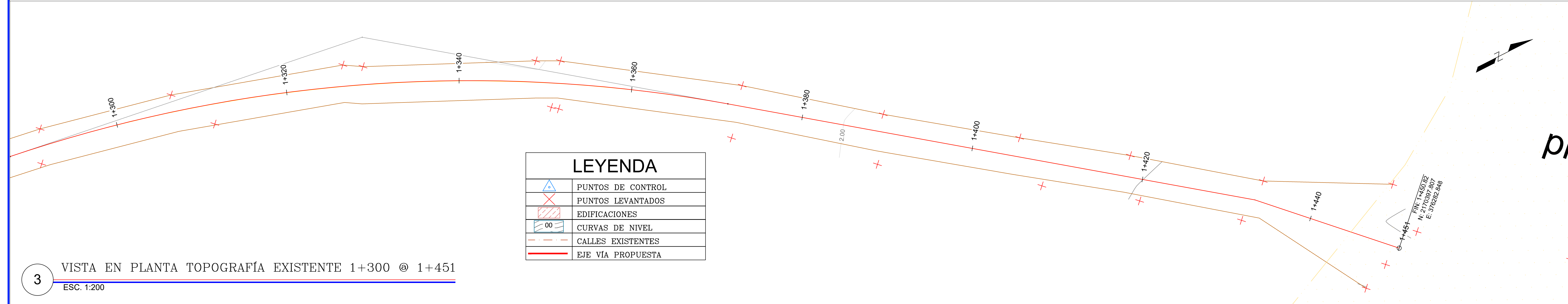
2 VISTA EN PLANTA TOPOGRAFÍA EXISTENTE 1+120 @ 1+280 ESC. 1:200
