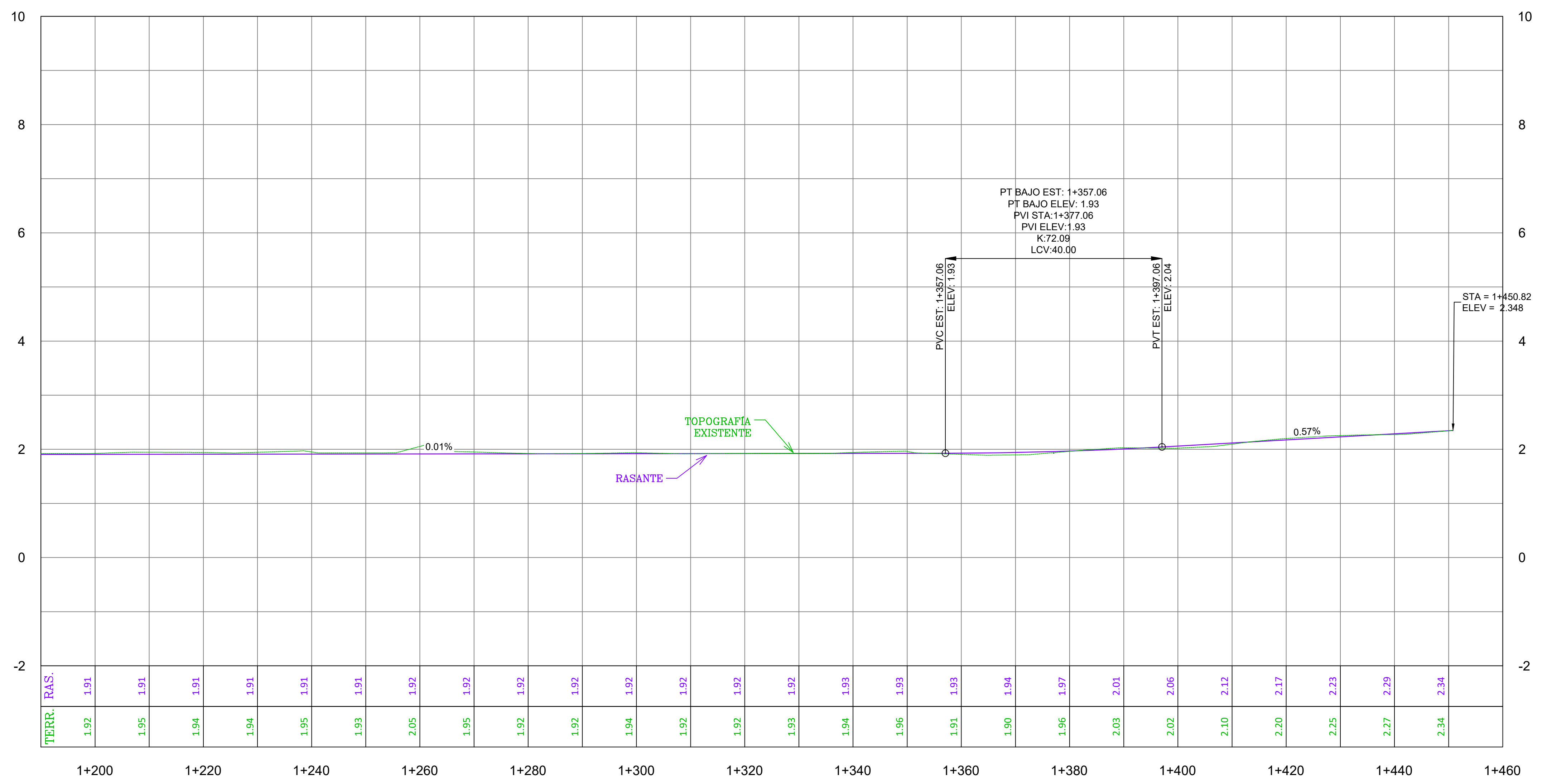
2 PERFIL LONGITUDINAL VÍA DE ACCESO PLAYA ROGELIO 1+200 @ 1+451 ESC. H1:500 ; V1:50
