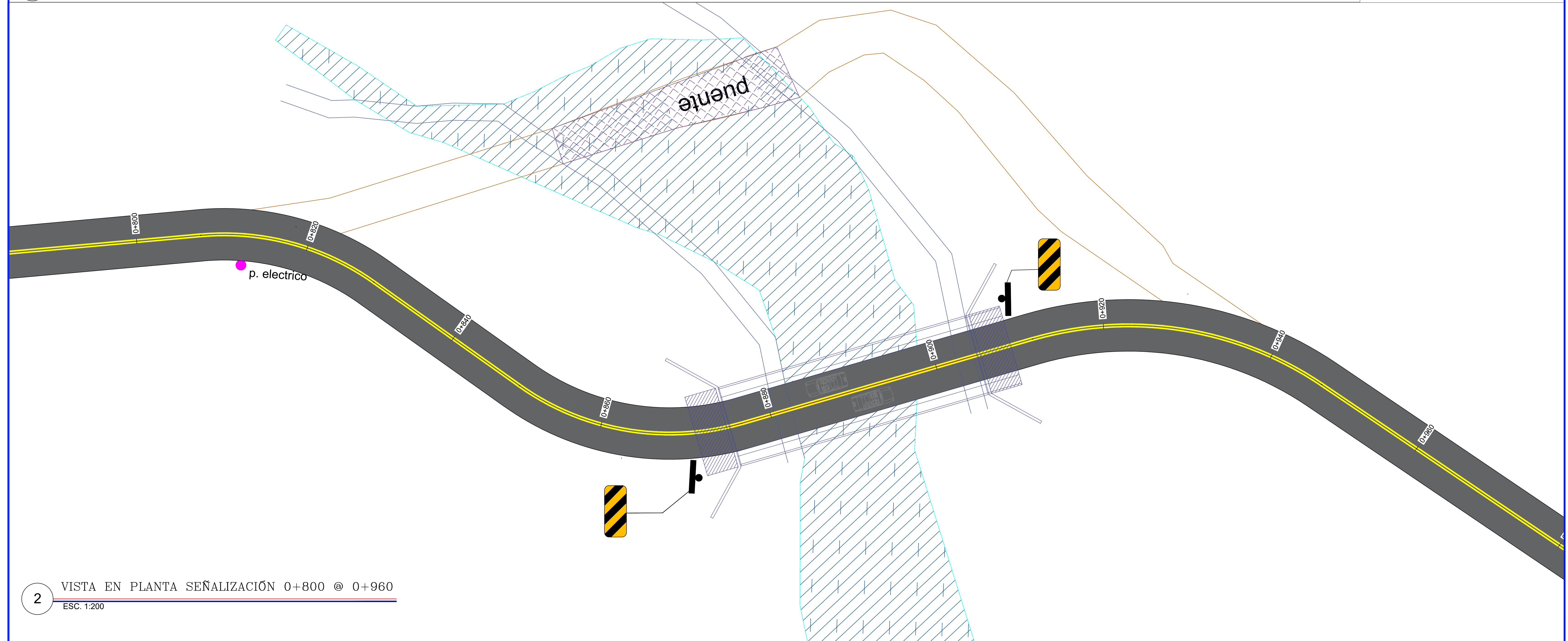
1 VISTA EN PLANTA SEÑALIZACIÓN 0+640 @ 0+800 ESC. 1:250
