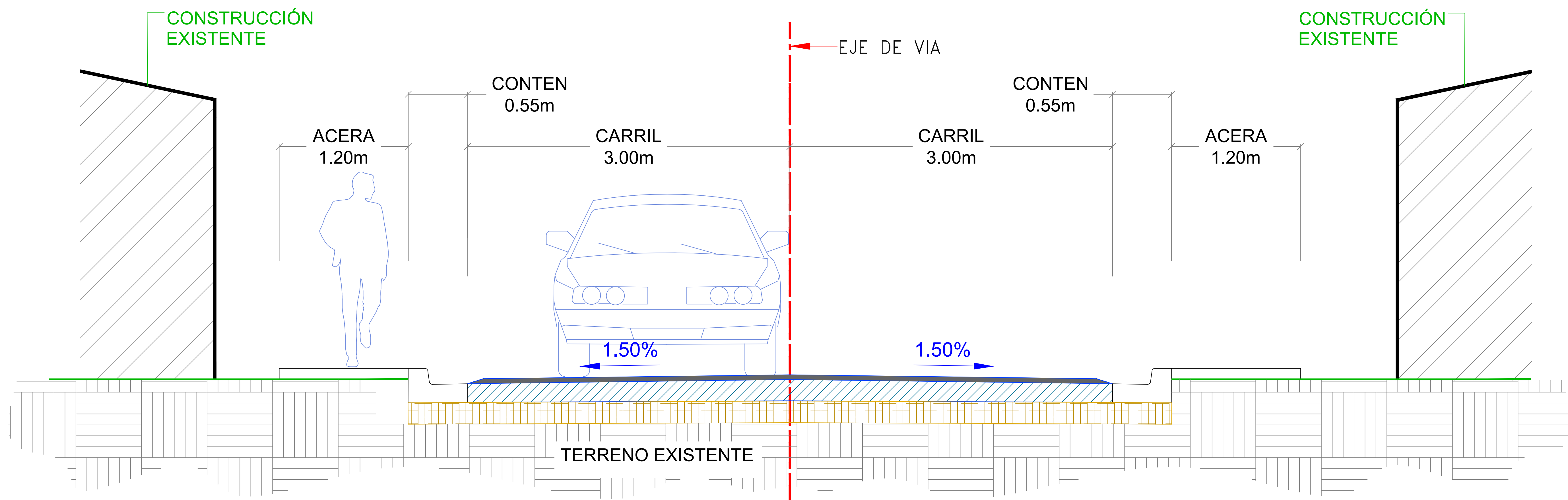
2 SECCIÓN TÍPICA 4+280 @ 5+280 ESC. 1:20
