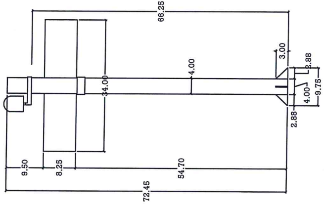
DISPLAY VISTA POSTERIOR
